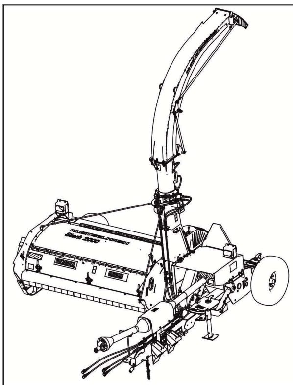
Рисунок 1.1 - Комбайн кормоуборочный полуприцепной КСД-2.0-01 «Sterh Plus»
