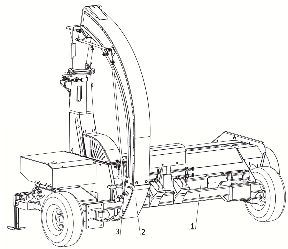
1 – сница; 2 – силосопровод; 3 – опора
