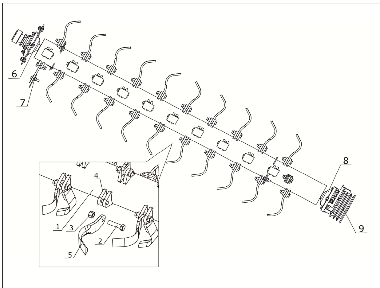
Рисунок 2.4 – Роторный режущий аппарат
