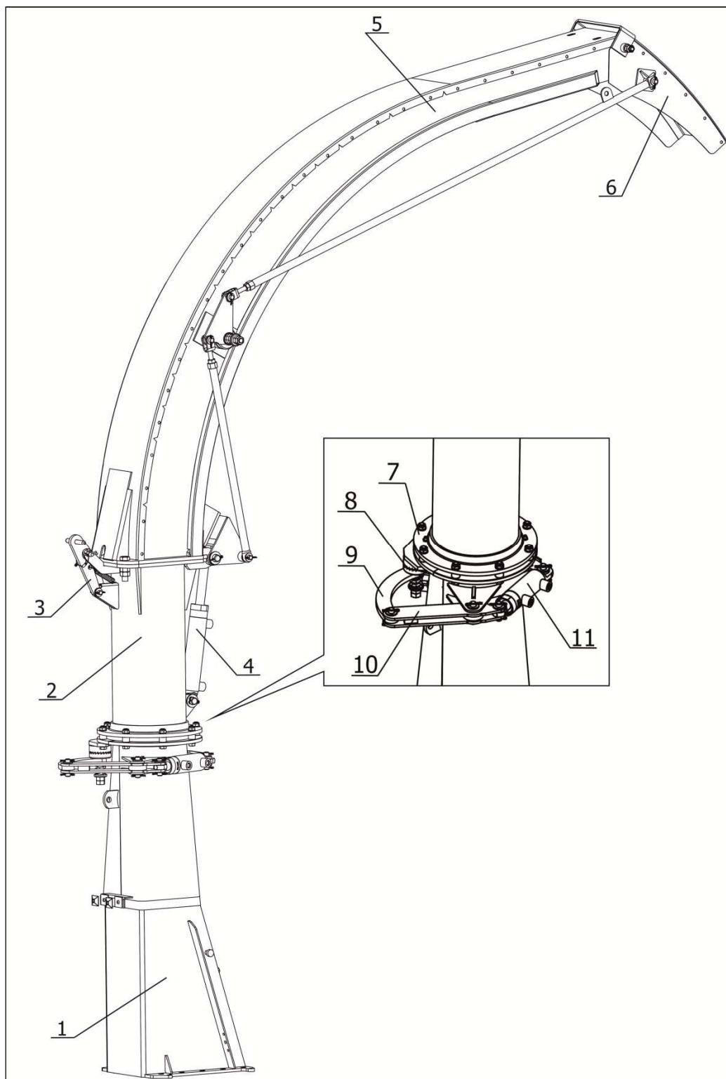
1 – основание силосопровода; 2 – опора; 3 – крючок; 4 – гидроцилиндр подъема силосопровода и управления козырьком; 5 – силосопровод; 6 – козырек; 7 – диски скользящие; 8 – муфта кулачковая; 9, 10 – рычаг; 11 – гидроцилиндр поворота силосопровода Рисунок 2.9 - Силосопровод
