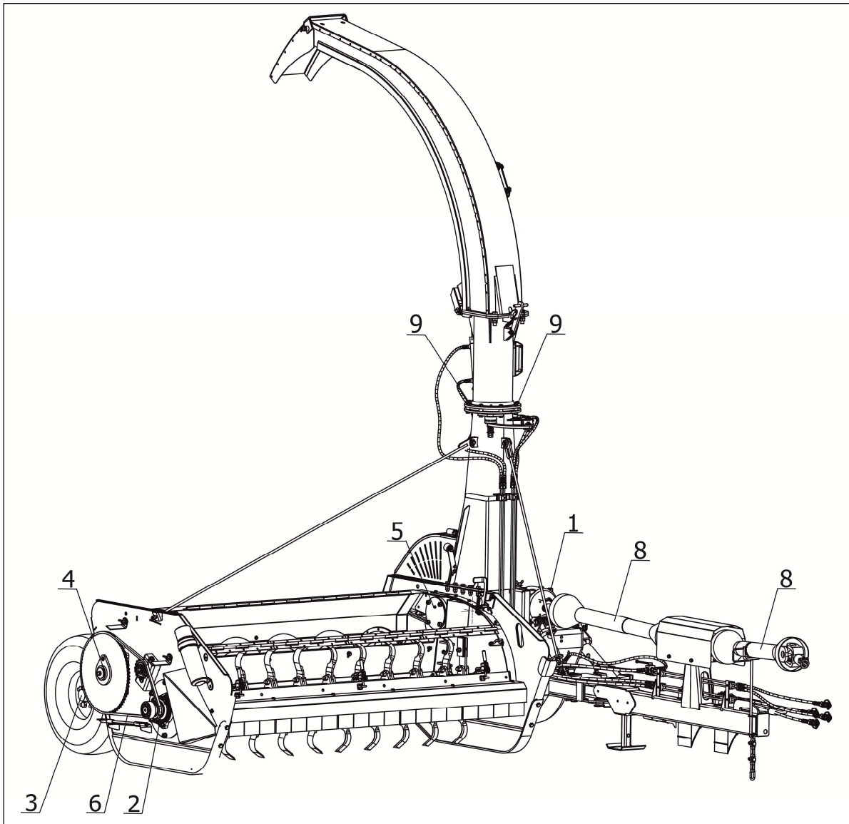
Рисунок 8.1 - Объекты смазки комбайна
