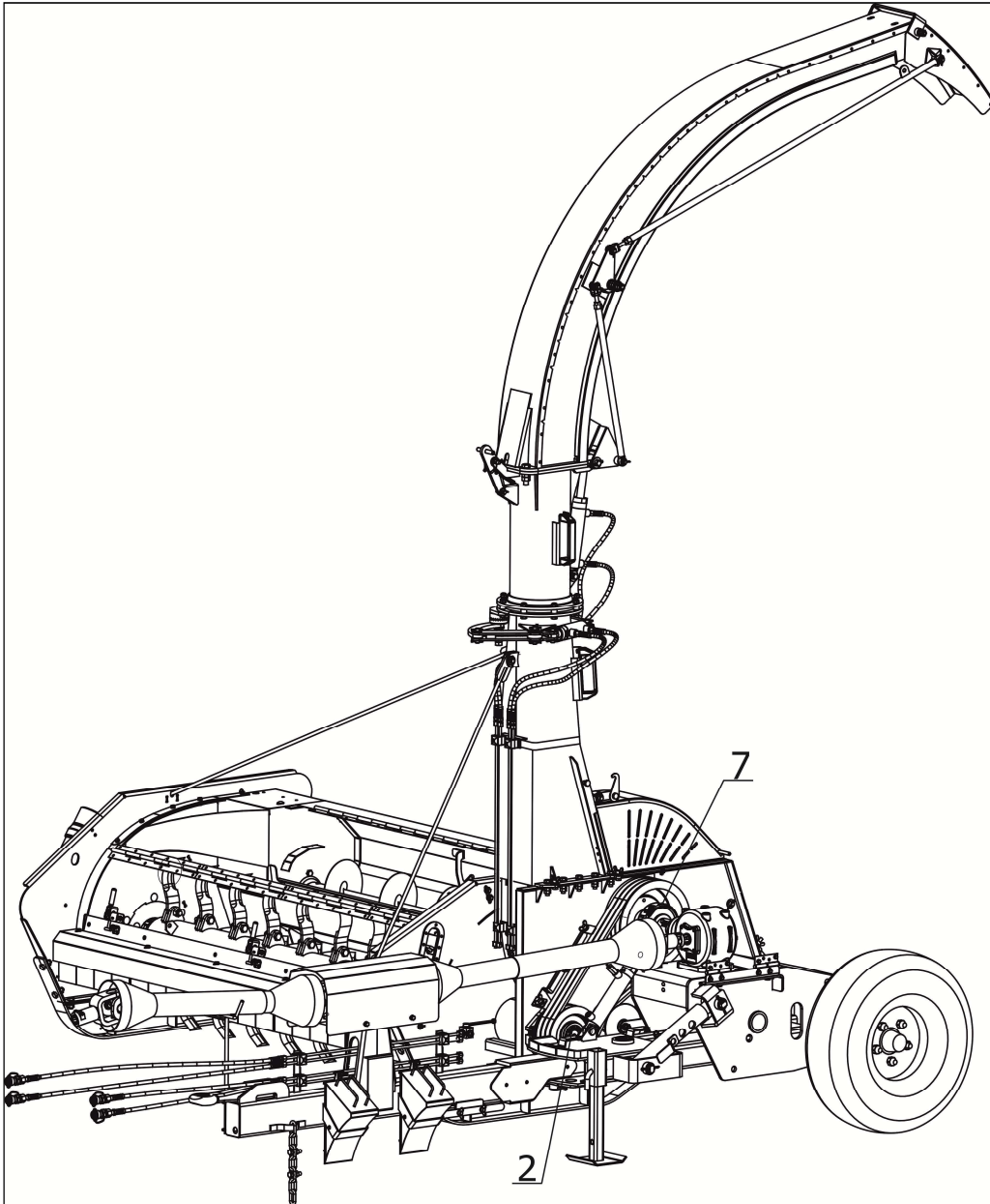
Рисунок 8.2 – Объекты смазки комбайна
