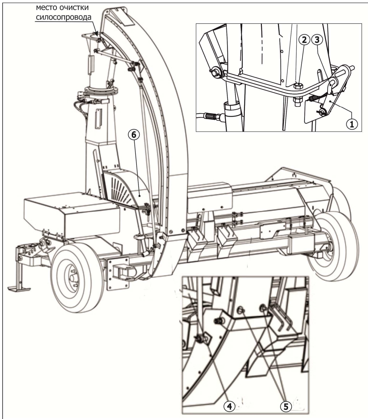
Рисунок 7.3 - Транспортное положение силосопровода
