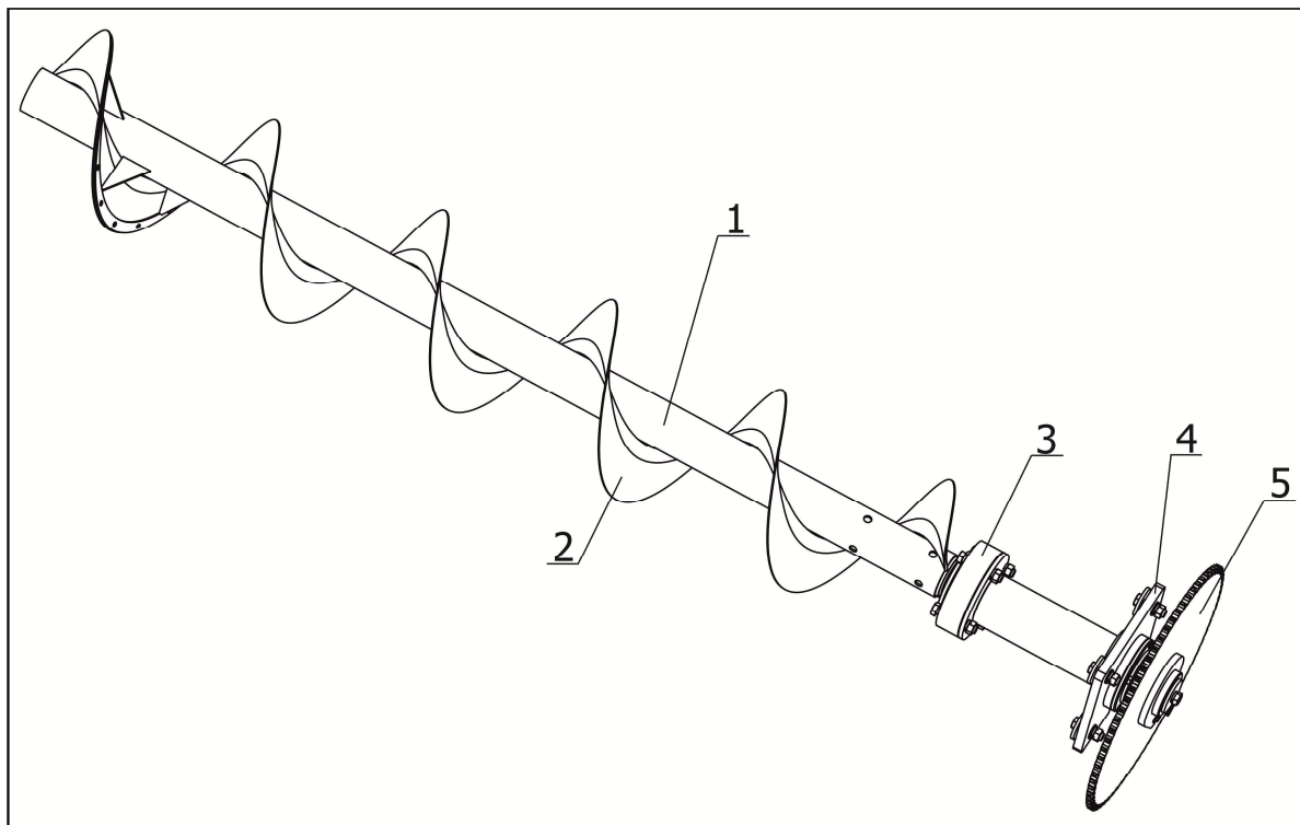
1 – труба; 2 – виток; 3, 4 – опора подшипниковая; 5 – звездочка привода
