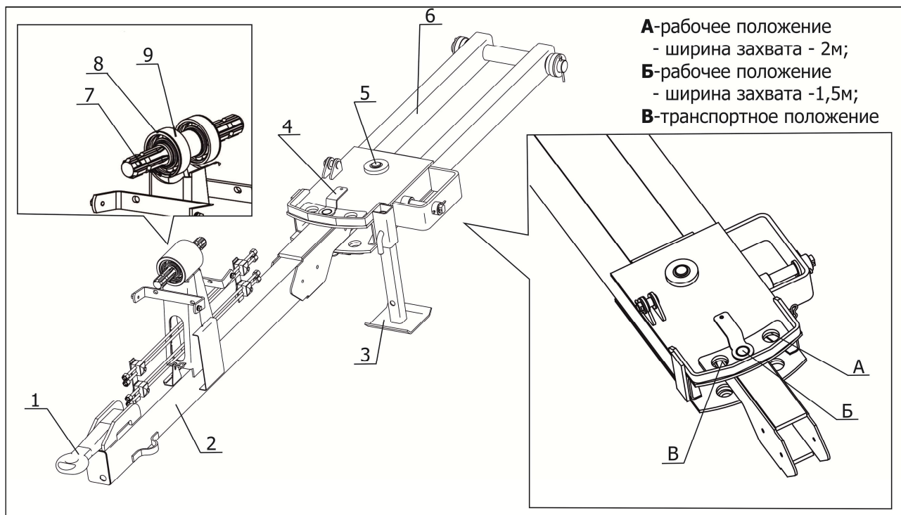
1 – зацеп; 2 – брус сницы; 3 – стояночная опора; 4 – палец; 5 – ось; 6 – опорная площадка; 7 – промежуточный вал; 8 – кольцо стопорное; 9 – подшипник
