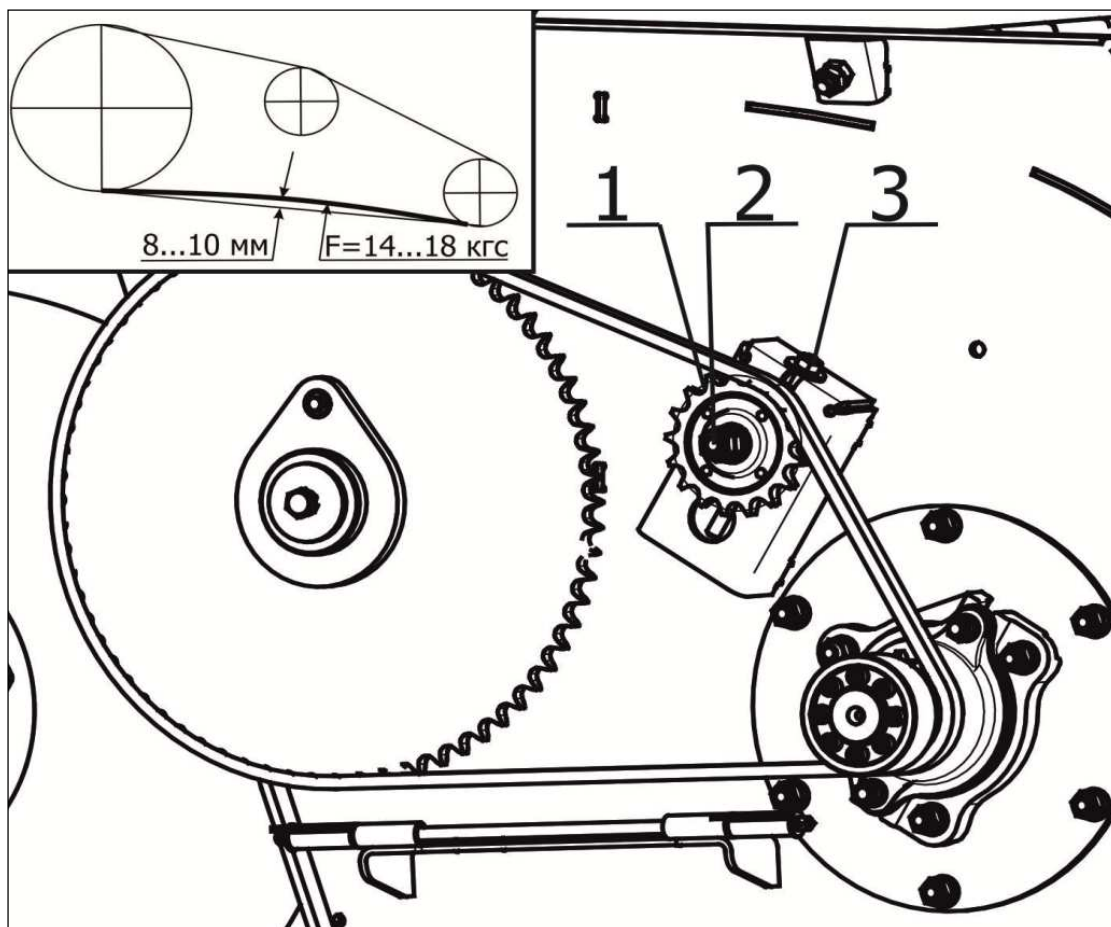
1 - звездочка натяжная; 2 – гайка; 3 - винт Рисунок 7.10 - Регулировка натяжения цепной передачи
