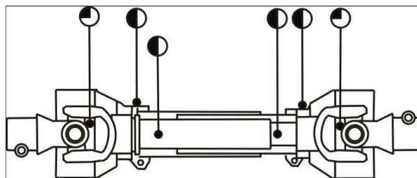
Рисунок 8.3 - Точки смазки карданного вала
