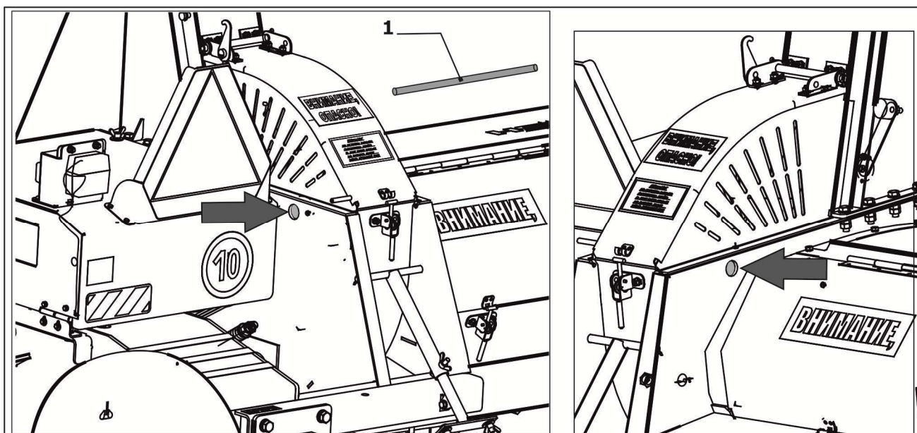
1 - монтажная лопатка
