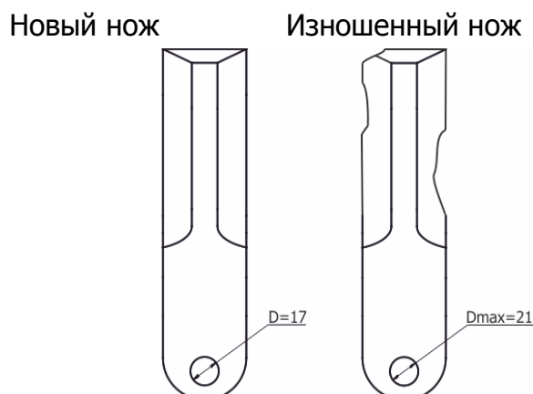
Рисунок 7.7 – Предельно допустимые размеры ножей
