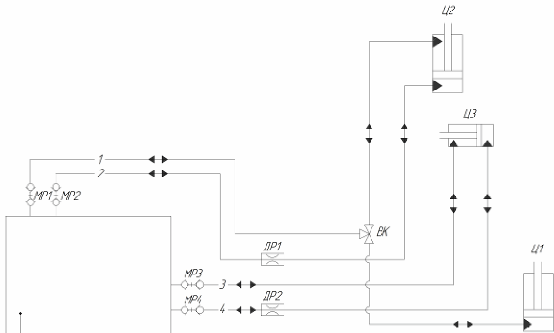
Гидравлическая система трактора для работы с навесными машинами
