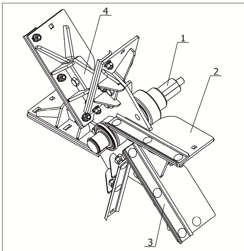
1 – вал; 2 – швыряющая лопатка; 3 – нож измельчителя; 4 – диск
