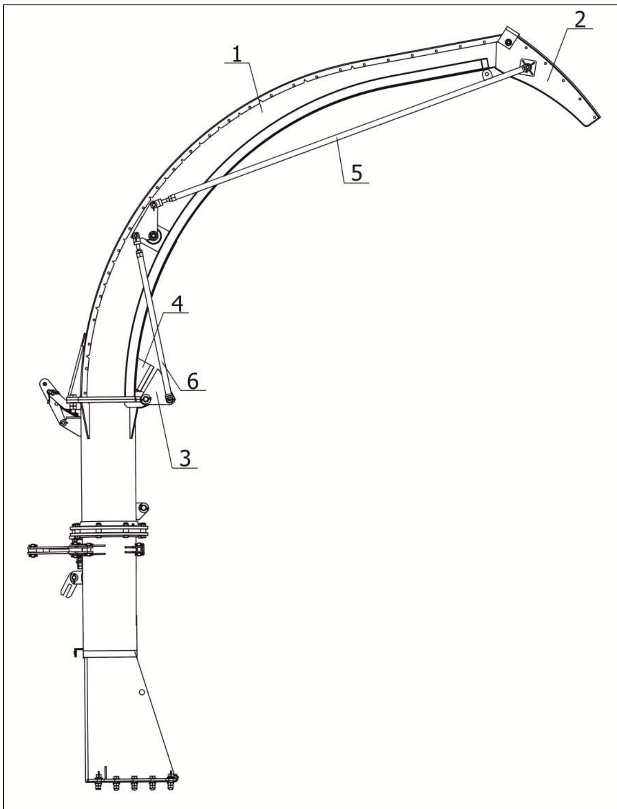
1 – верхняя часть силосопровода; 2 – козырек; 3 – кронштейн; 4 – упор силосопровода; 5, 6 – тяга Рисунок 7.8 – Силосопровод
