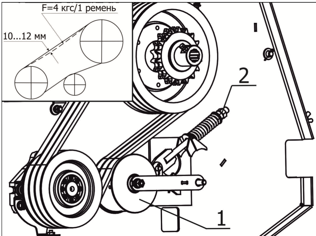
1 - ролик натяжной; 2 - гайка Рисунок 7.9 - Регулировка натяжения ременной передачи
