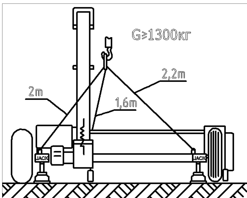
Рисунок 11.1 - Схема строповки
