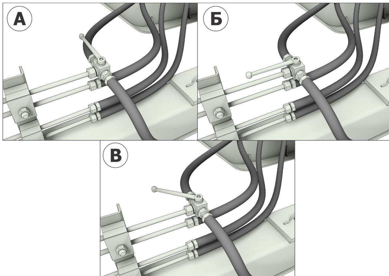
Рисунок 7.2 - Положения рукоятки гидрокрана
