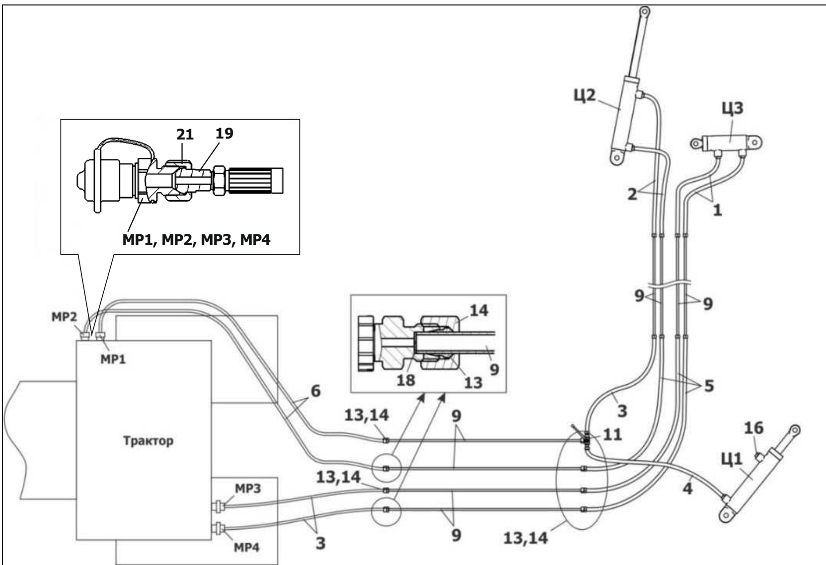
Рисунок А.2 – Схема гидравлических соединений
