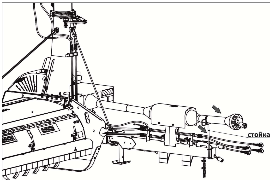
Рисунок 7.4 - Стойка для поддержки карданного вала
