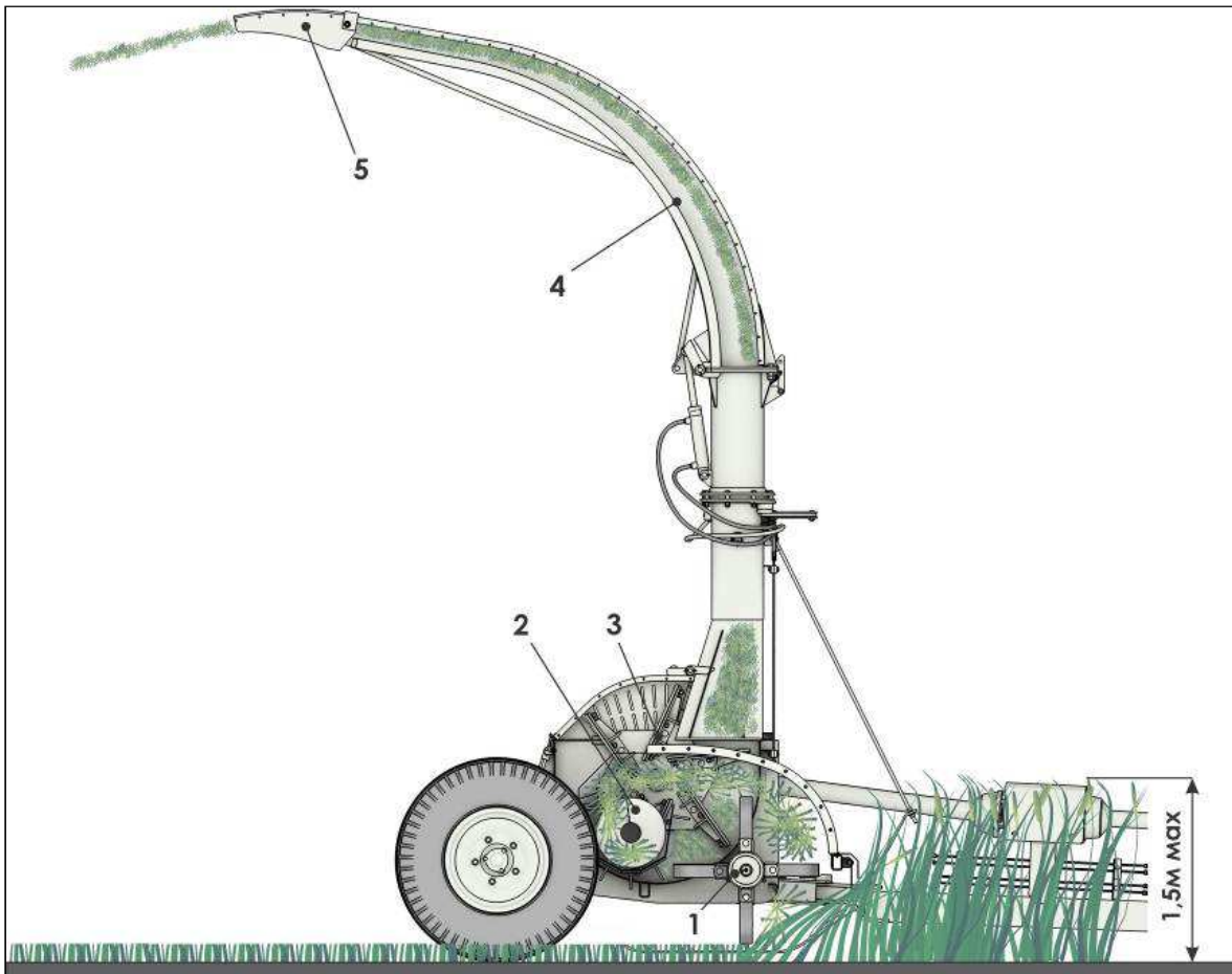
1 – ротор; 2 – шнек; 3 – измельчающий аппарат; 4 – силоспровод; 5 – козырек Рисунок 2.2 - Технологическая схема работы комбайна
