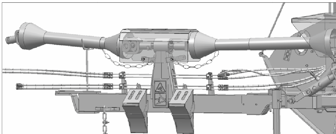
Рисунок 6.5 – Фиксация кожуха карданного вала
