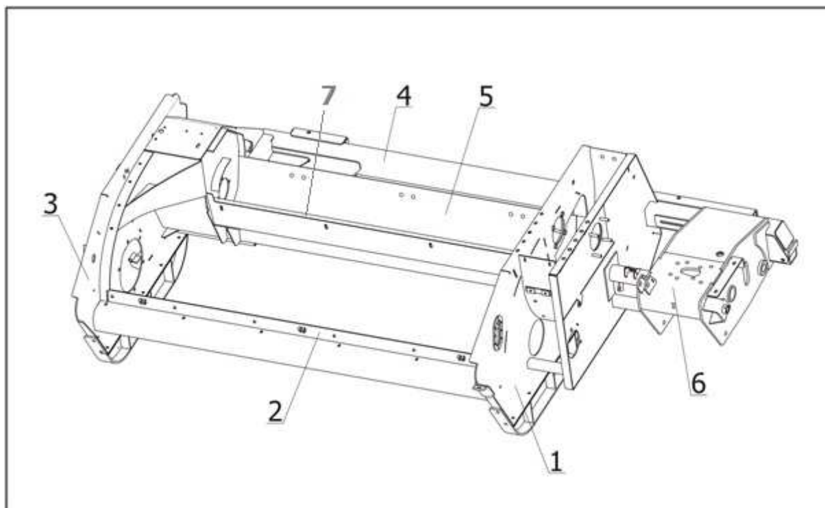
1 – боковина левая; 2 – брус передний; 3 – боковина правая; 4 – труба ходовой части; 5 – корыто шнека; 6 – площадка для установки мультипликатора; 7 – чистик (уголок)
