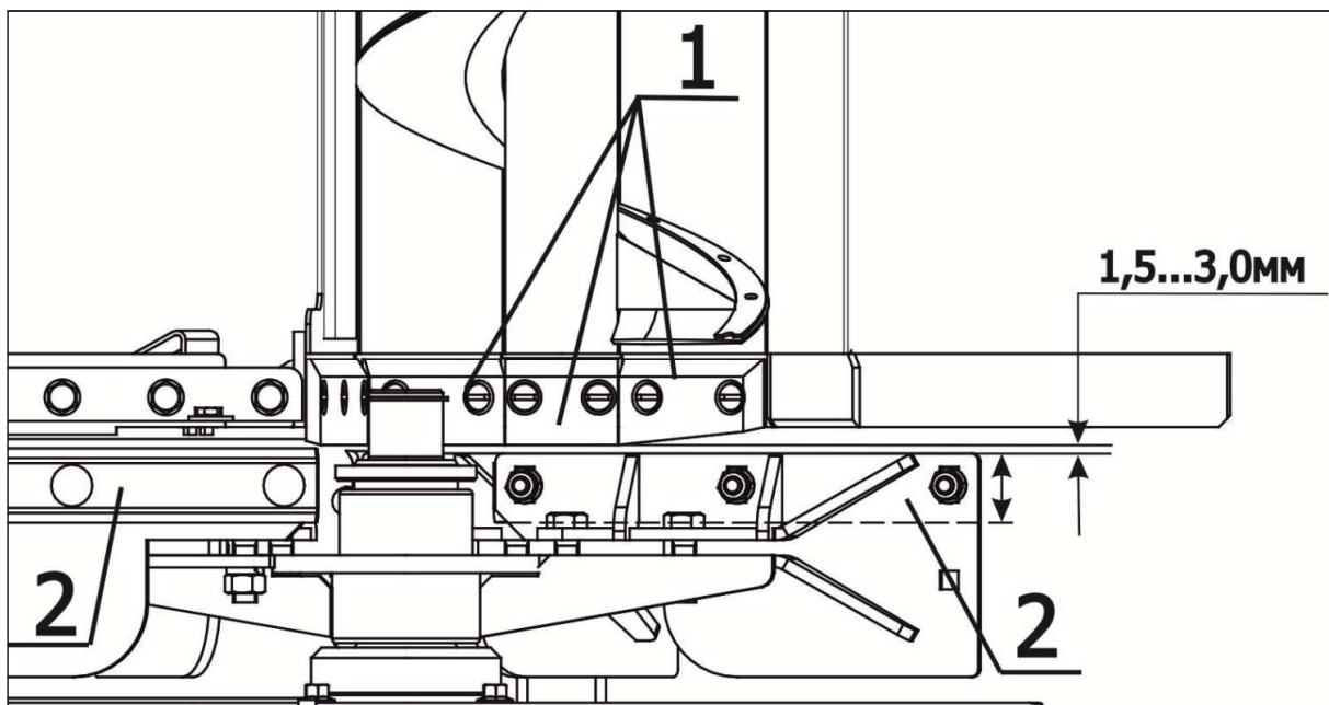
1 – противорежущие пластины; 2 – нож Рисунок 2.8 – Регулировка измельчителя
