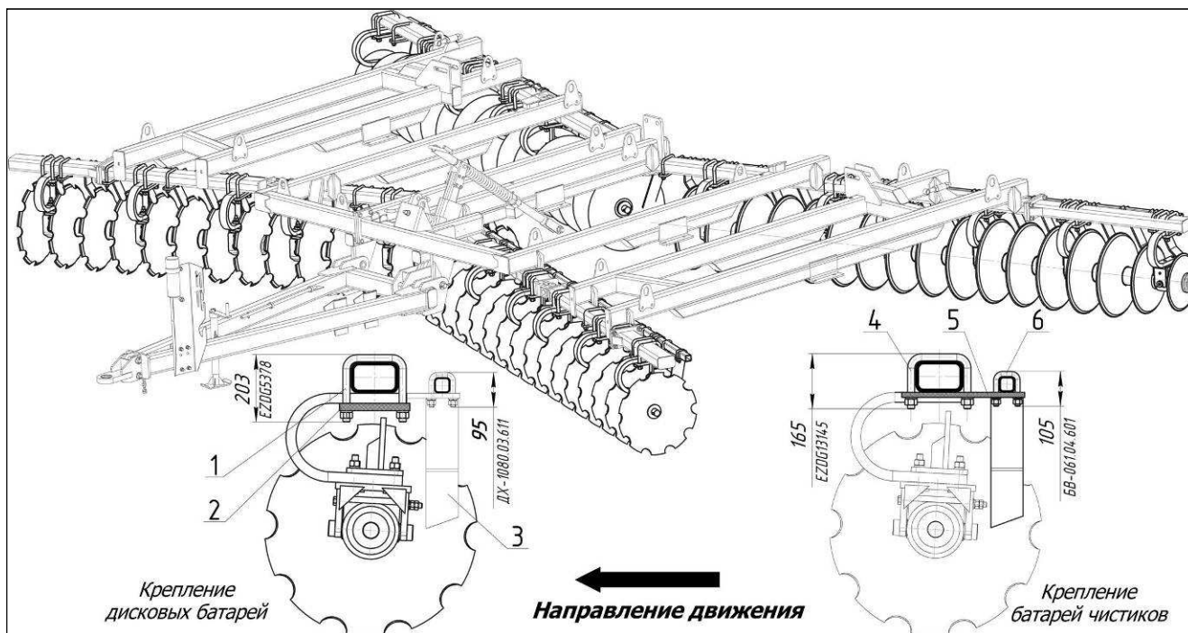
1 – U-болт 7/8×6" EZDG5378; 2 – плита (БВ-061.03.090); 3 – скоба крепления М12 ДХ-1080.03.611; 4 – U-болт 3/4×6-7/8" EZDG13145; 5 – плита крепления чистиков (ДХ-971.04.418); 6 – скоба крепёжная М16 БВ-061.04.601
