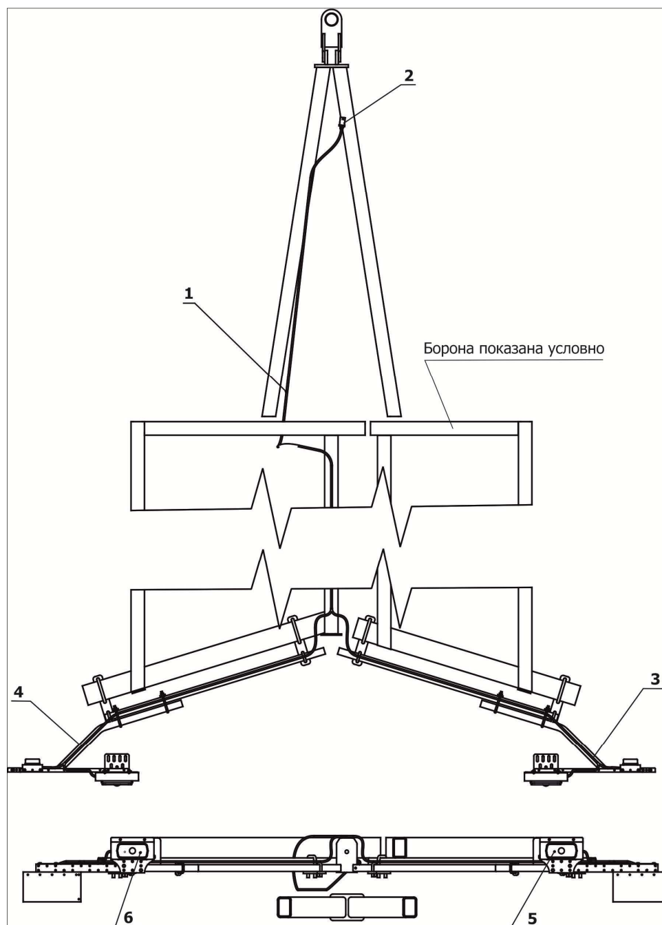
1 – жгут кабельной проводки; 2 – вилка; 3, 4 – кронштейн фонарей; 5,6 – фонарь Рисунок 5.20 – Коммуникации электрические
