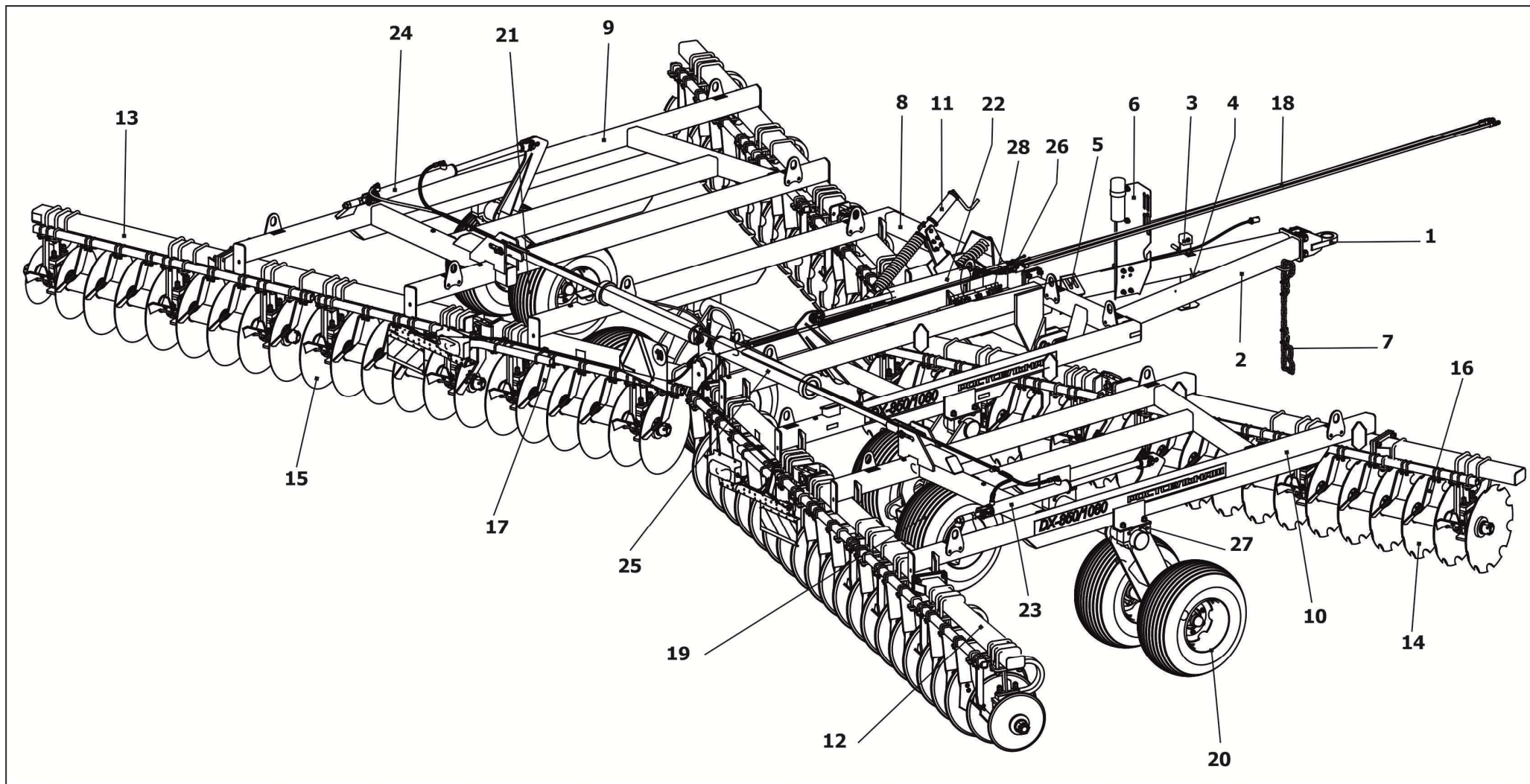
1 – прицеп; 2 - сница; 3 – опорная стойка; 4 – чистик; 5 – противооткатные упоры; 6 – стойка; 7 – страховочная цепь; 8 – рама; 9 – крыло левое; 10 – крыло правое; 11 – регулятор горизонта; 12 – удлинитель крыла передний; 13 – удлинитель крыла задний; 14 – дисковые батареи переднего ряда; 15– дисковые батареи заднего ряда; 16 – чистик переднего ряда; 17 – чистики заднего ряда; 18 – коммуникации электрические; 19 – шасси центральной рамы; 20, 21 – шасси крыла; 22 – гидроцилиндр подъёма центральной рамы; 23, 24 – гидроцилиндр подъёма крыла; 25 – гидроцилиндр подъёма крыла; 26 – кран гидравлический; 27 – подшипниковая опора шасси; 28 – набор стоп-сегментов
