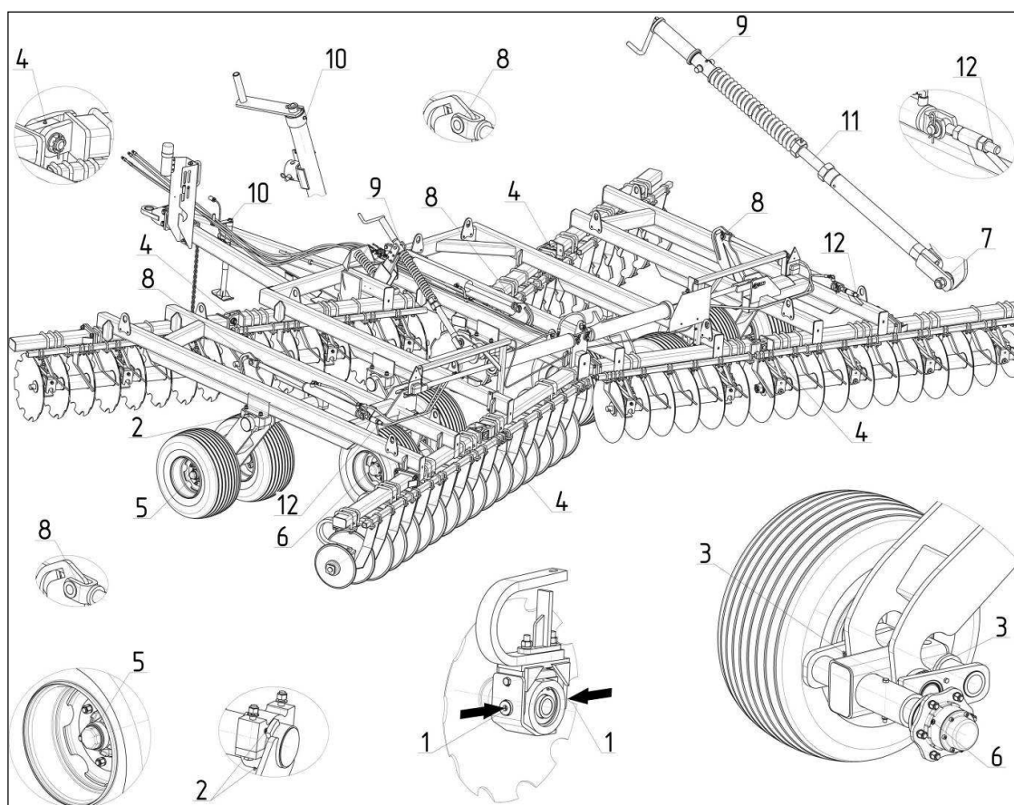
1 – подшипниковые опоры дисковых батарей; 2 – подшипниковые опоры шасси; 3 – балансиры шасси рамы; 4 – шарнирное соединение рамы и крыльев; 5 – ступица колеса крыла; 6 – ступица колеса шасси рамы; 7 – шаровая опора регулятора горизонта; 8 – шаровая опора гидроцилиндра шасси; 9 – регулятор горизонта; 10 – домкрат; 11 – резьбовая часть регулятора горизонта; 12 – резьбовая часть регулятора глубины на крыле Рисунок 7.1 - Места смазки бороны
