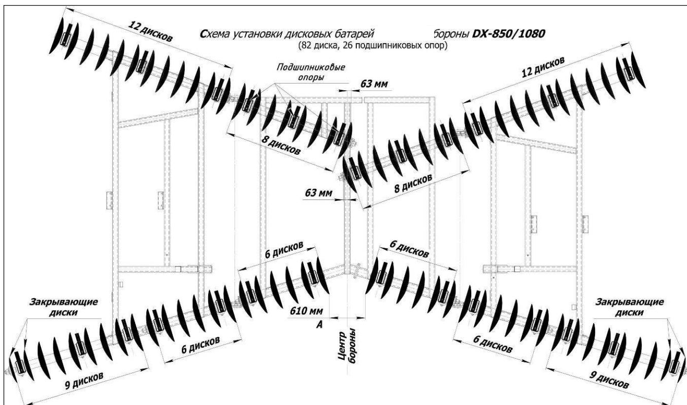
Рисунок 5.11 – Схема установки дисковых батарей для борона DX-850/1080
