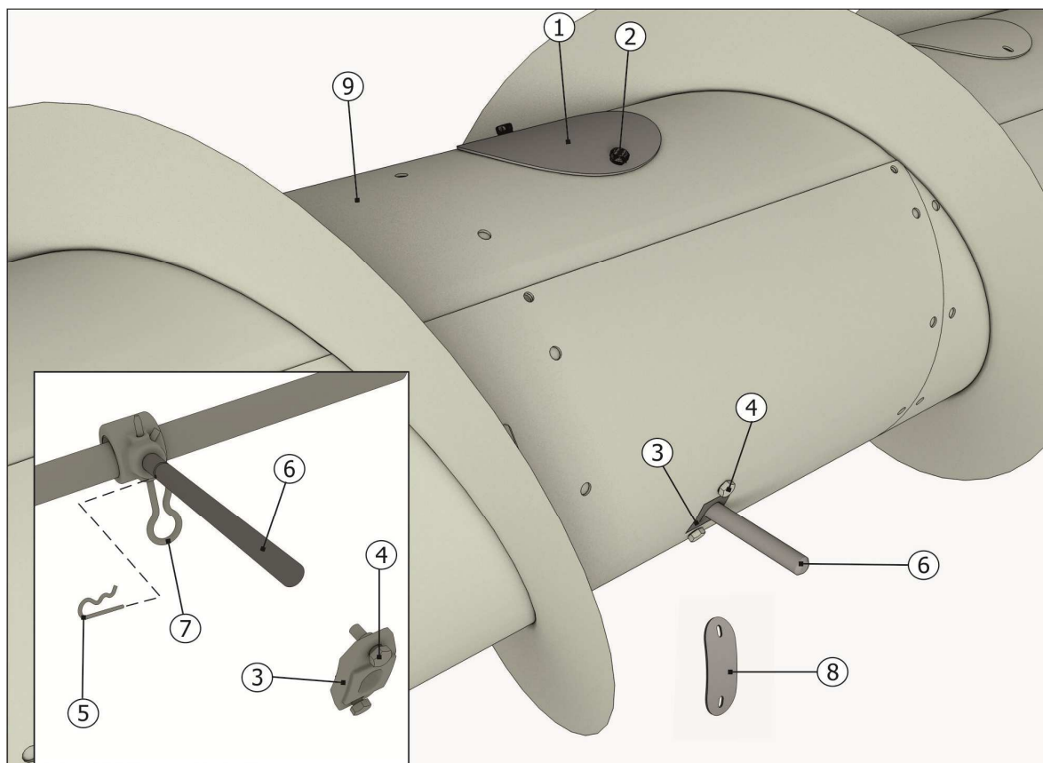
1 - крышка; 2,4 - болтокрепеж; 3 - глазок; 5 – шплинт; 6 - палец; 7 – фиксатор; 8 – крышка; 9 - шнек Рисунок 6.11
