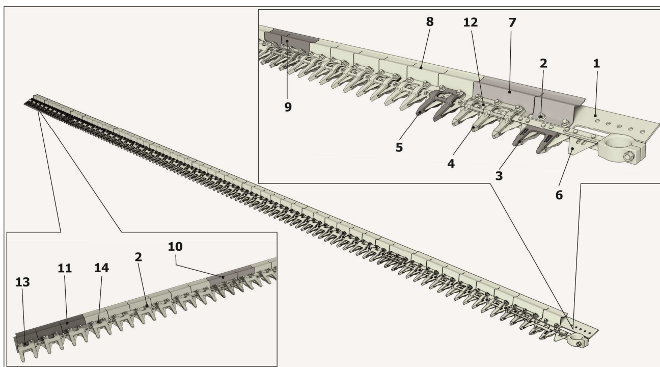
1 - брус; 2 - болтокрепеж; 3, 4, 5 – палец; 6 – нож; 7, 8, 9, 10, 11 – камнеотбойник; 12, 13, 14 – пластина трения
