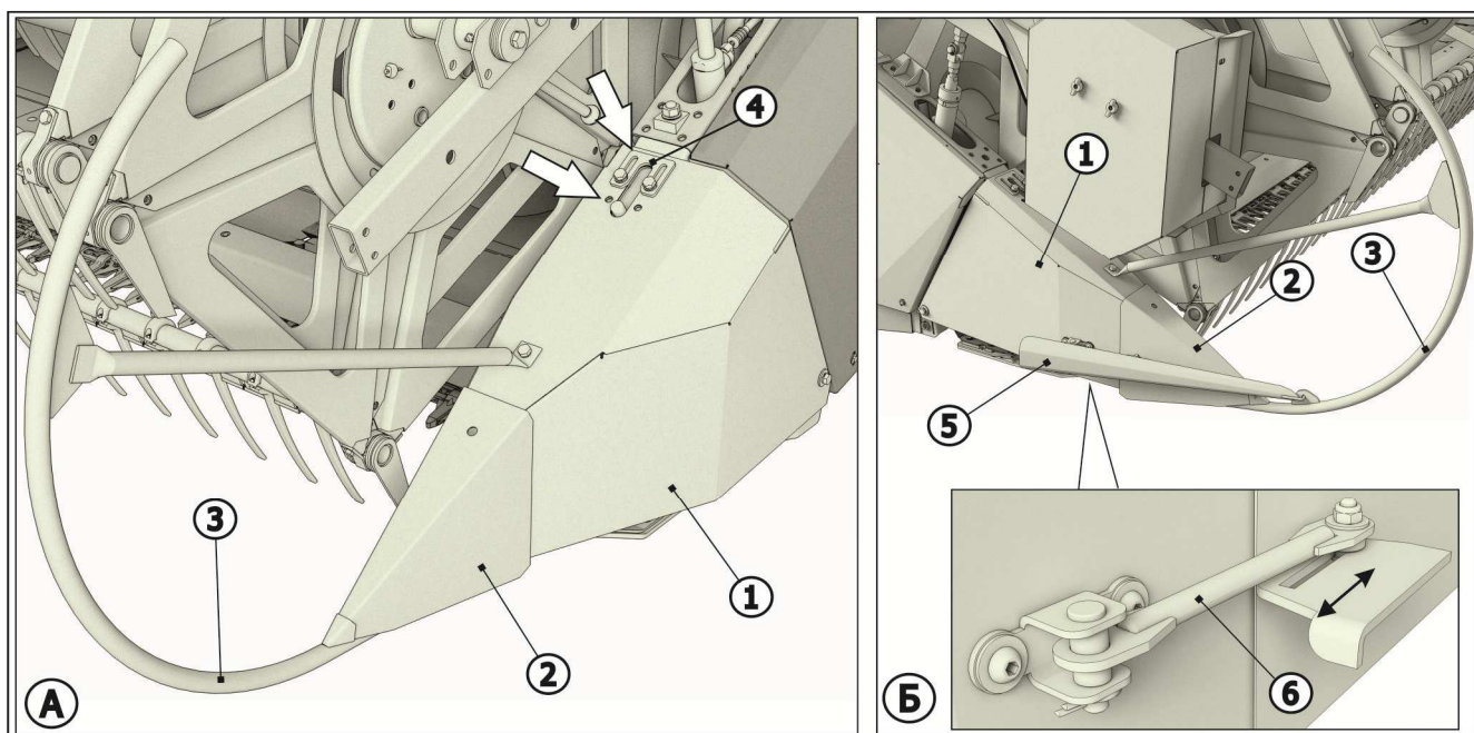
А - левый делитель; Б - правый делитель 1 – корпус делителя; 2 – носок делителя; 3 – труба делителя; 4 - пластина регулировочная; 5 - отсека- тель; 6 - тяга
