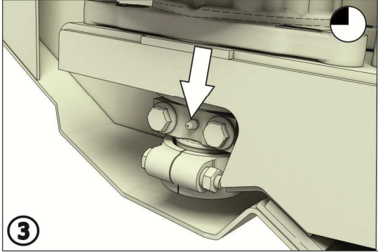
Рисунок 7.1 - Точки смазки жатки
