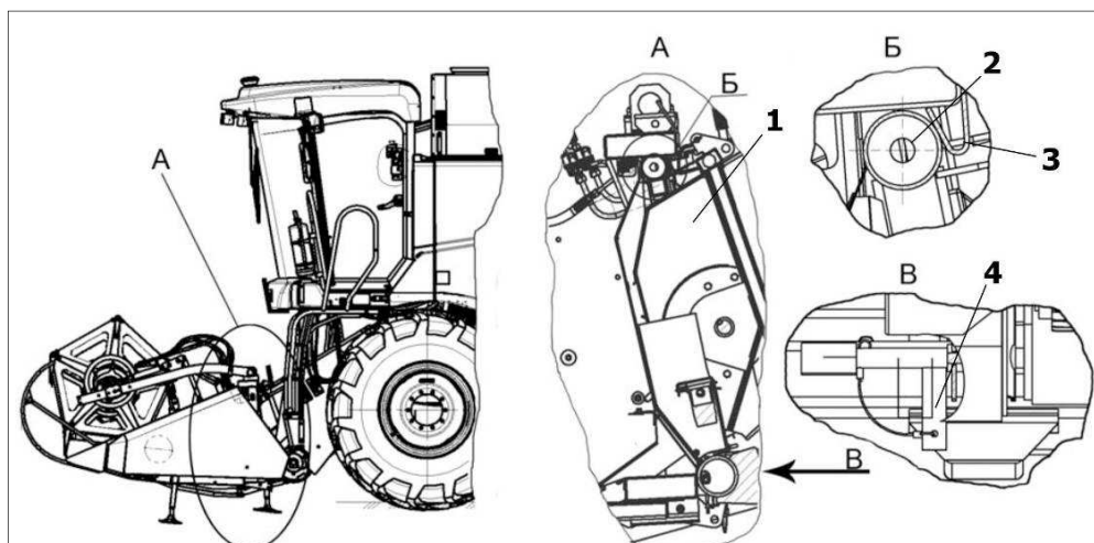
1 - наклонная камера; 2 - верхняя труба переходной рамки наклонной камеры; 3 – ловитель; 4 – фиксатор Рисунок 5.5 - Монтаж жатки на комбайн
