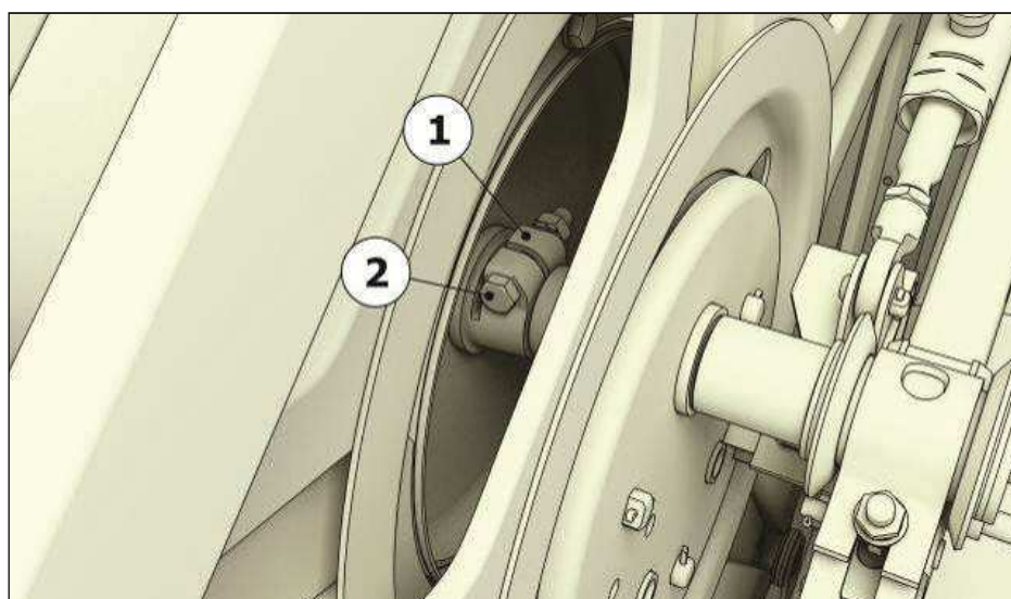
1 – клемма; 2 - болт Рисунок 6.7 - Контроль затяжки клеммы мотовила
