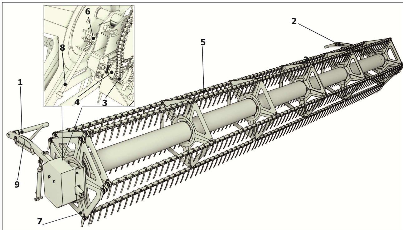
1, 2 - поддержка; 3 – цепная передача; 4 – гидромотор; 5 - граблина; 6 - сектор; 2 - рукоятка; 4 - крестовина; 5 - труба мотовила; 6 - палец; 7 – эксцентрик; 8 – рукоятка; 9 - опора Рисунок 2.4 – Мотовило
