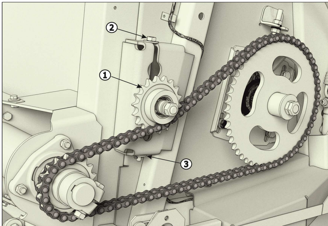
1 - звездочка натяжная; 2 – болт; 3-шайба
