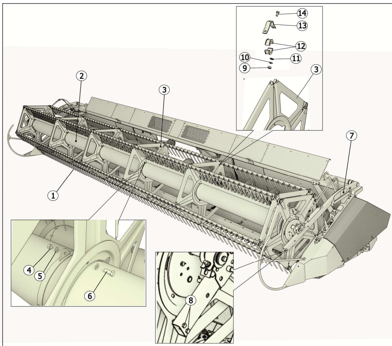
1 - граблина; 2 - труба; 3 - крестовина; 4, 9 - гайка; 5, 10, 11 - шайба; 6, 8, 14 - болт; 7 - труба поддержки мотовила; 12 - полуподшипник; 13 - скоба
