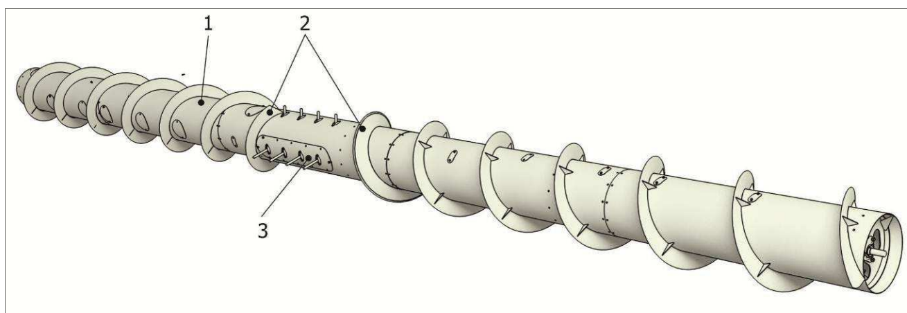
1 - труба; 2 - правая и левая винтовая лента; 3 - аппарат пальчиковый Рисунок 2.5 – Шнек
