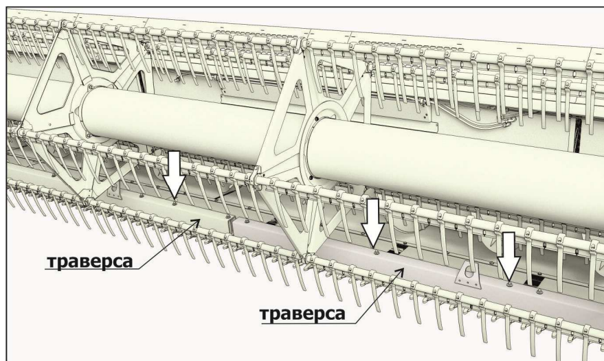
Рисунок – 8.1 Установка траверс на жатку
