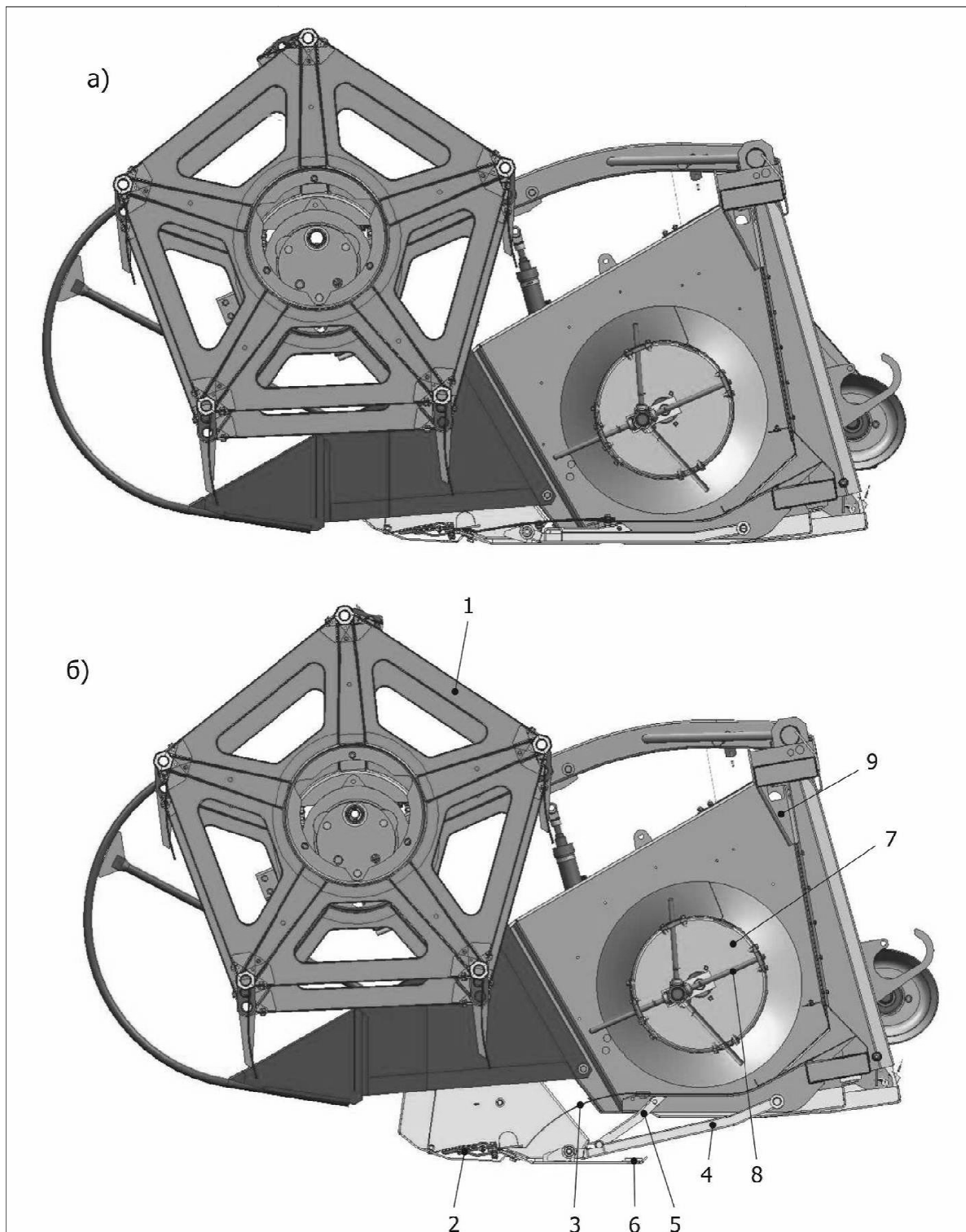
а) «с жестким ножом»; б) «с плавающим ножом» 1 – мотовило; 2 – режущий аппарат; 3 – пружинный щиток днища; 4.5 – рычаг; 6 – башмак режущего аппарата; 7 – шнек; 8 – палец шнека; 9 – корпус жатки Рисунок 2.2 - Схема работы жатки
