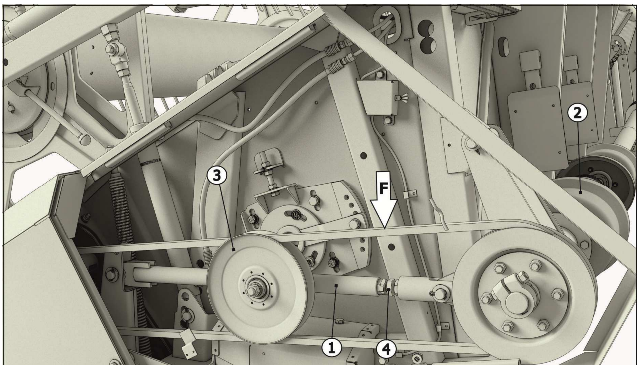
1 – тяга; 2 – контрпривод; 3 – шкив; 4 - винт регулировочный; F – усилие Рисунок 6.21 - Регулировка натяжения ремня
