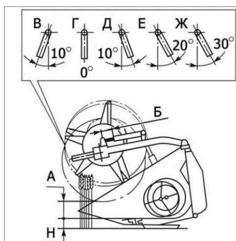
Рисунок 6.5 - Положения граблин мотовила
