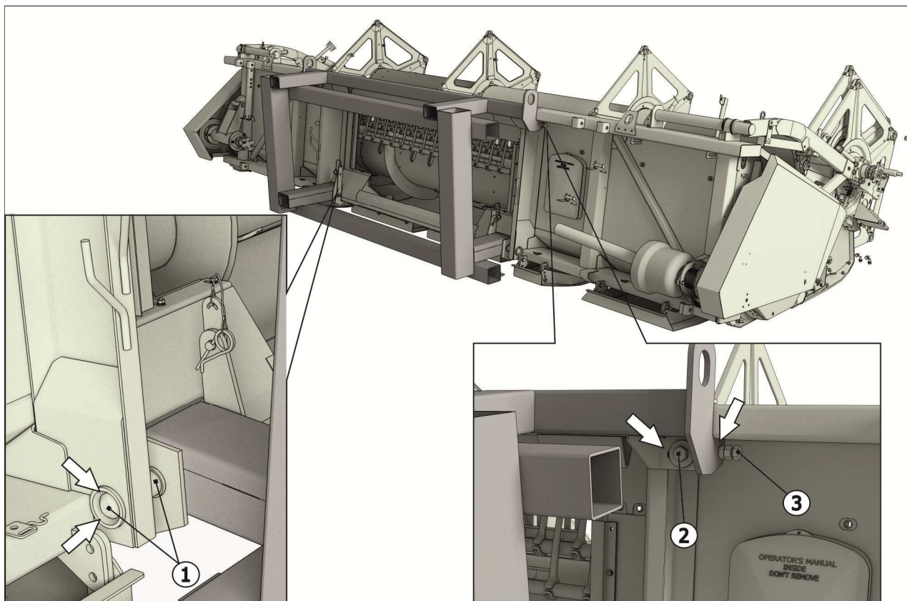
1 – фиксатор погрузочной рамки; 2 – болтокрепёж; 3 – болт Рисунок 8.10
