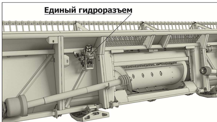
Рисунок 2.8 - Единый гидроразъем
