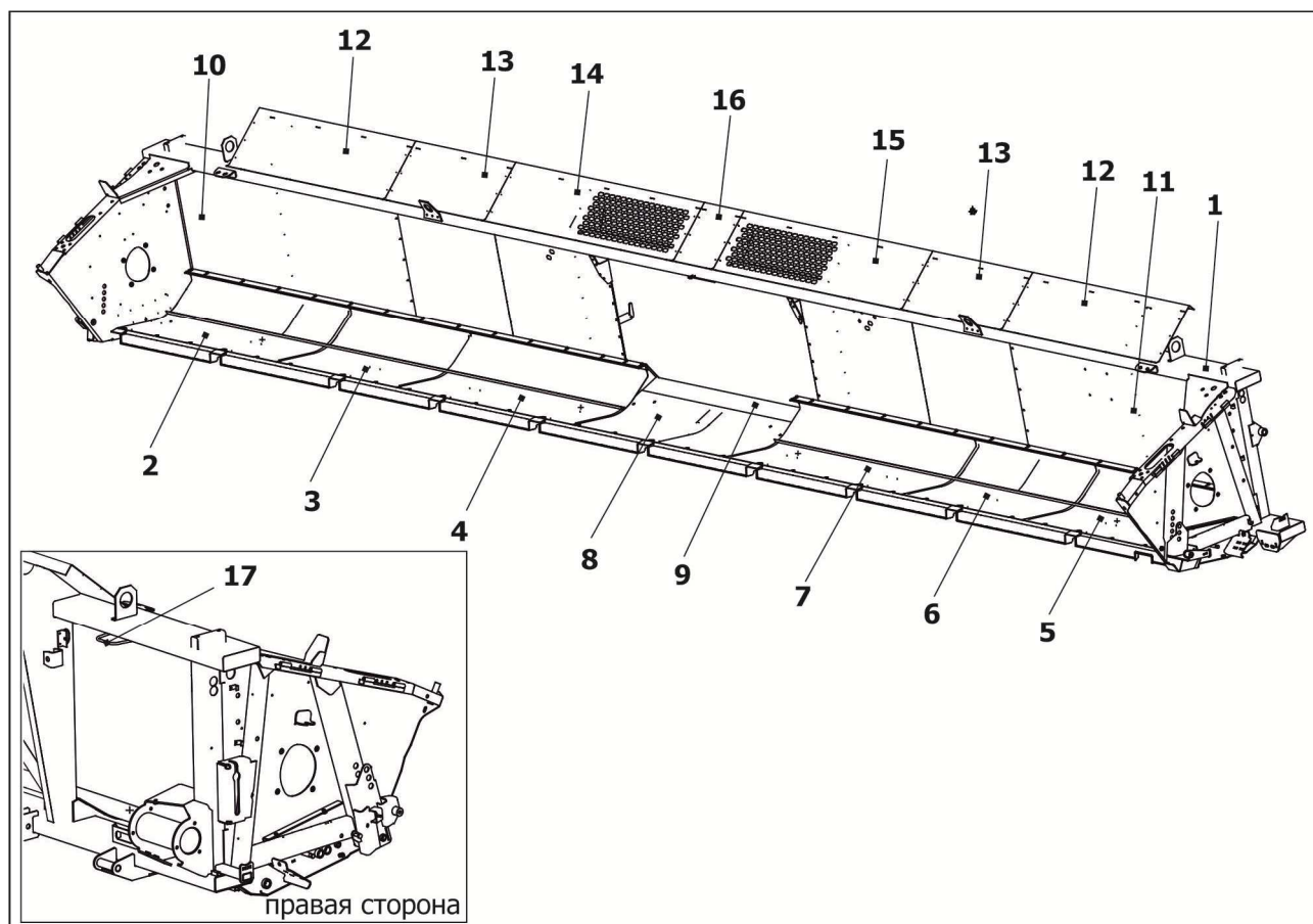
1 – рама; 2, 3, 4 – правое днище; 5, 6, 7 – левое днище; 8 – центральное днище; 9 – упор; 10, 11 – задний лист; 12, 13, 14, 15, 16 – щит; 17 - кронштейн
