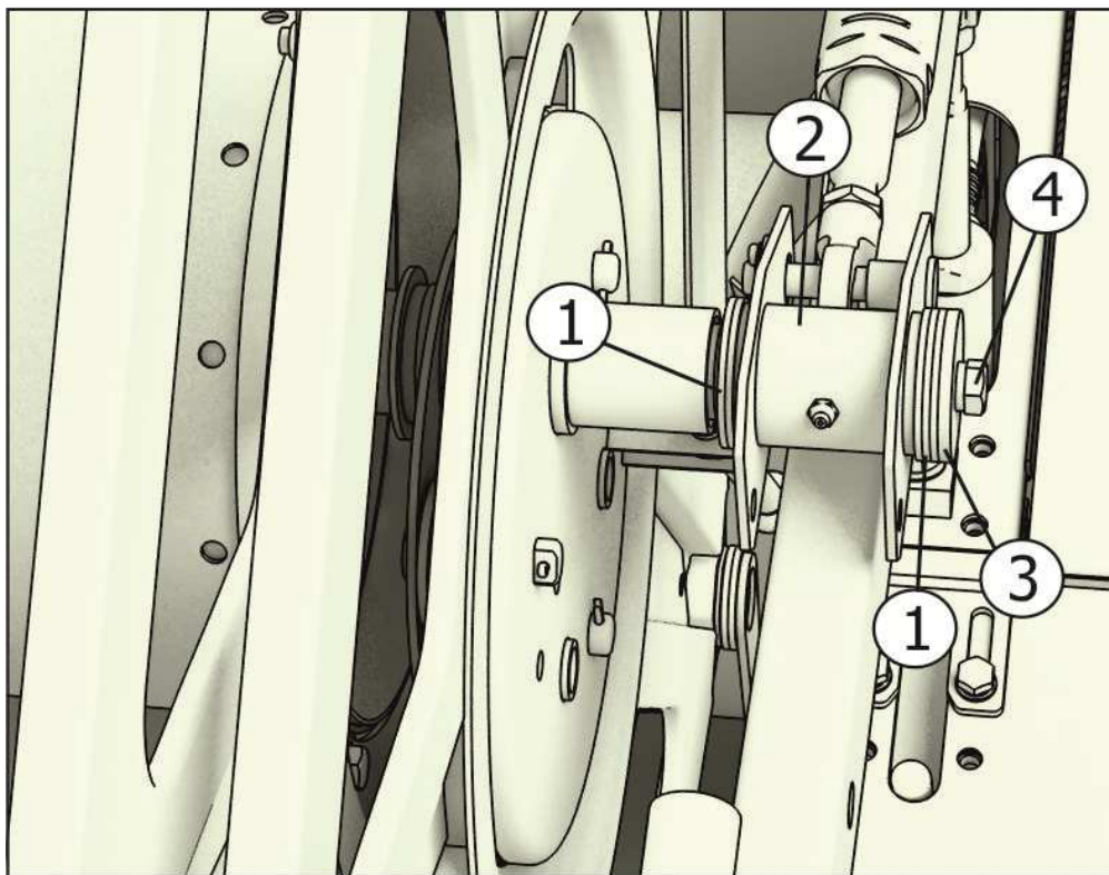
1 - шайба регулировочная; 2 – подшипник; 3 - шайба специальная; 4 - болт торцевой Рисунок 6.8 - Регулировка положения мотовила относительно боковин каркаса жатки
