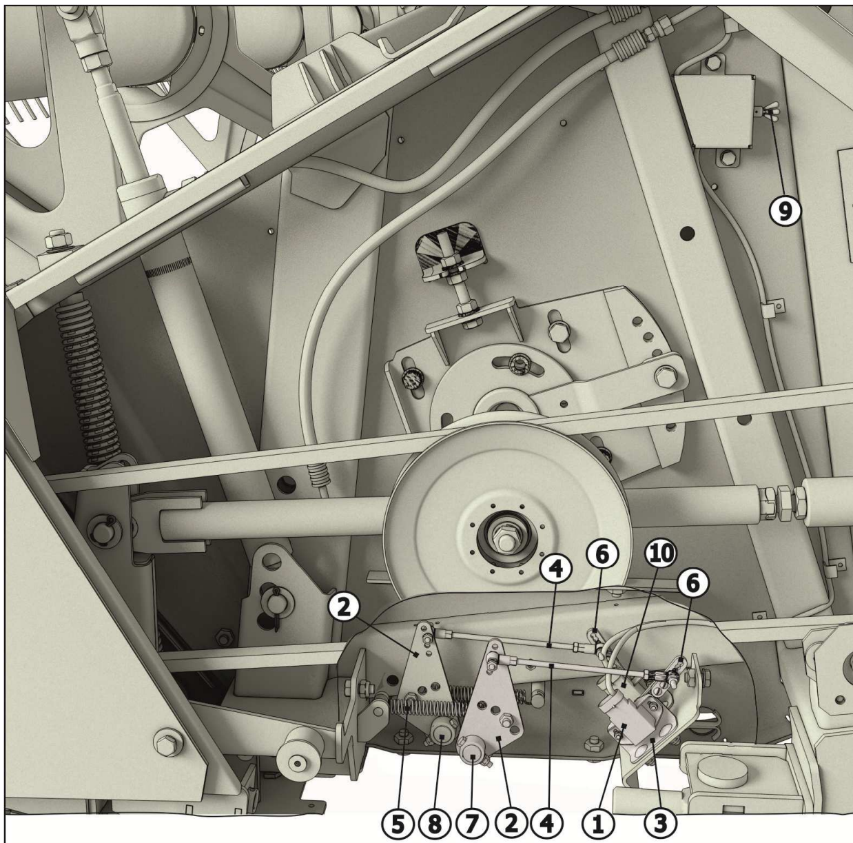
Рисунок 2.9 – Установка датчиков автоконтура. Правая боковина жатки
