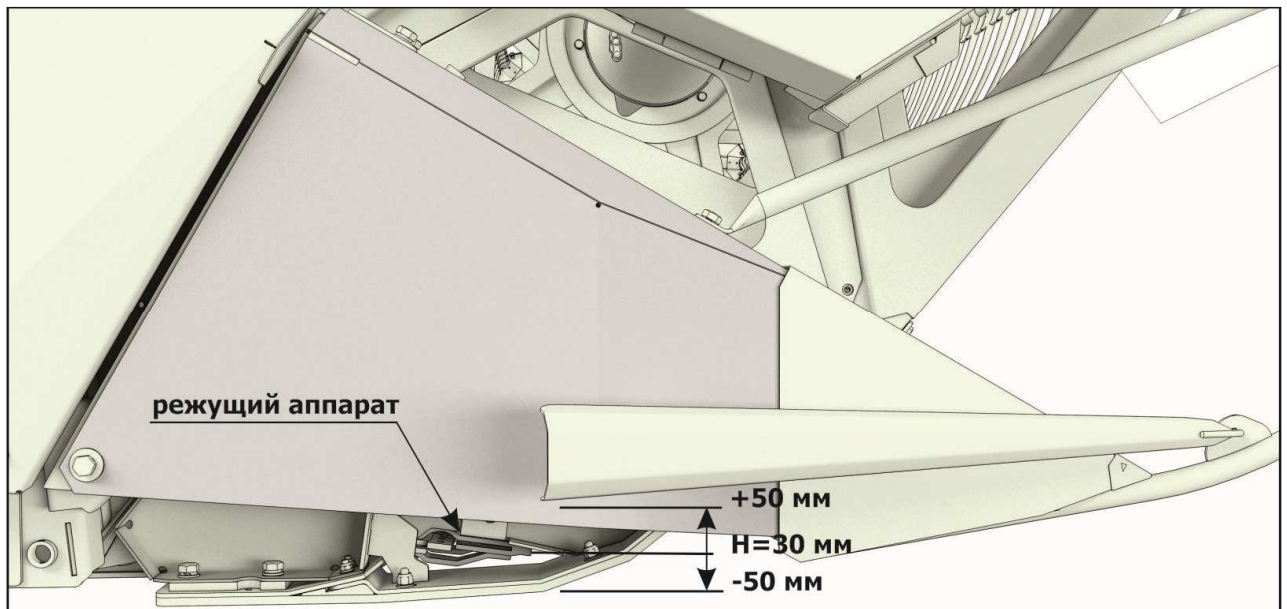
Рисунок 6.14 - Положение режущего аппарата при уборке сои в режиме «с плавающим ножом»
