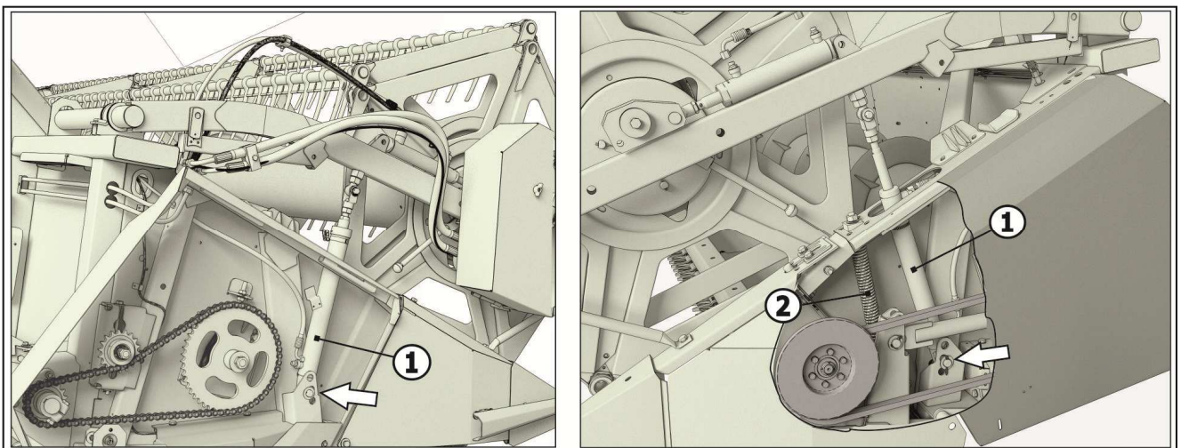
1 – гидроцилиндр; 2 – вертикальная пружина Рисунок 5.2 – Пружина уравновешивания редуктора привода ножа
