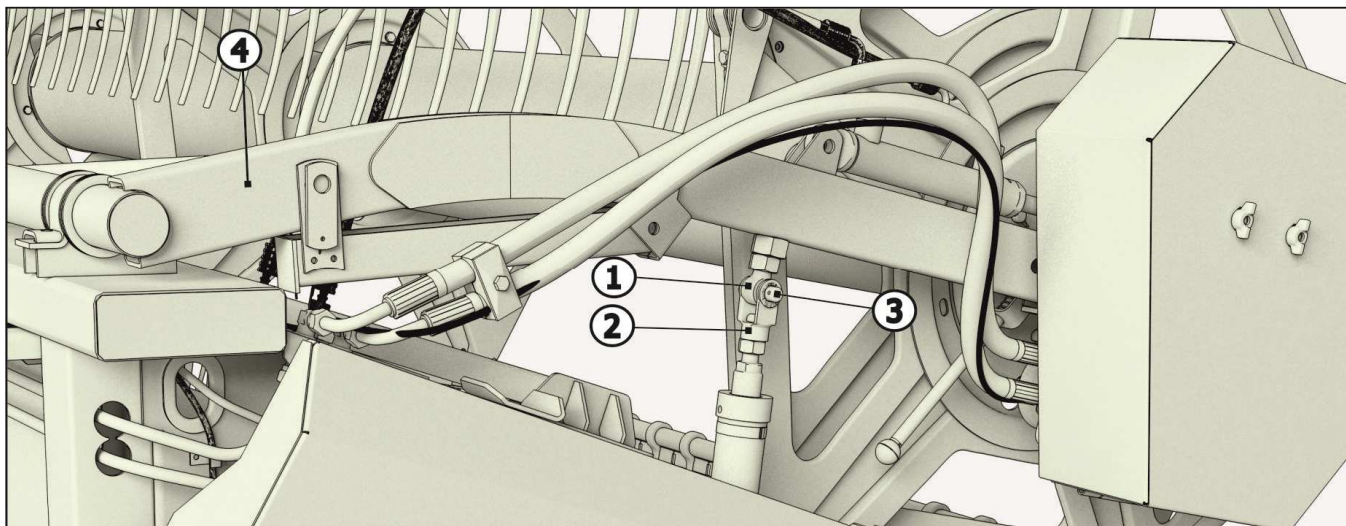
1 – винт; 2 - вилка гидроцилиндра; 3 – ось; 4 – поддержка Рисунок 6.6 - Регулировка положения мотовила
