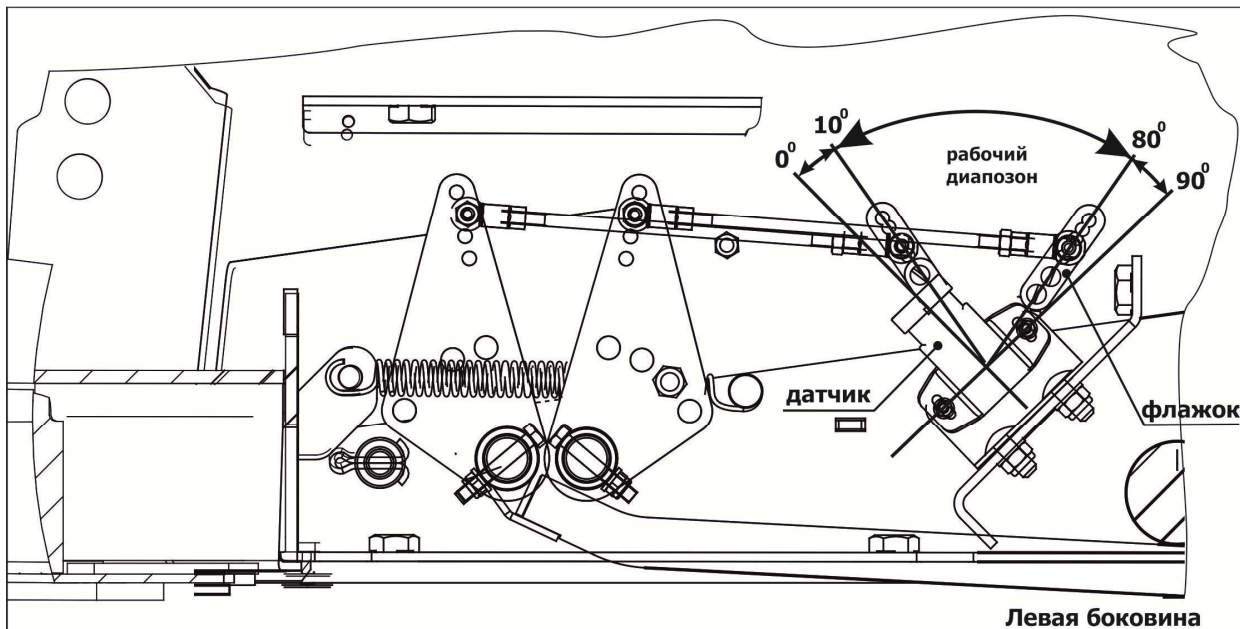
Рисунок 6.19 – Рабочий диапазон датчика положения
