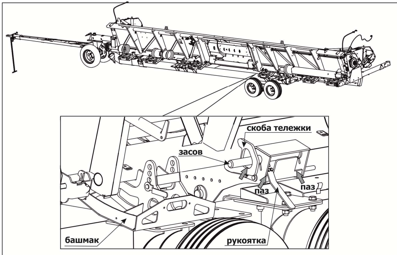
Рисунок 8.7 – Установка жатки на тележку
