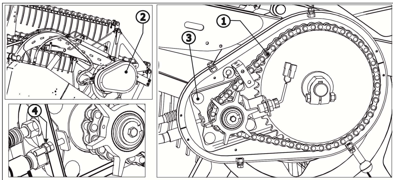
1-цепная передача мотовила; 2-щиток; 3-болт; 4-контгайка
