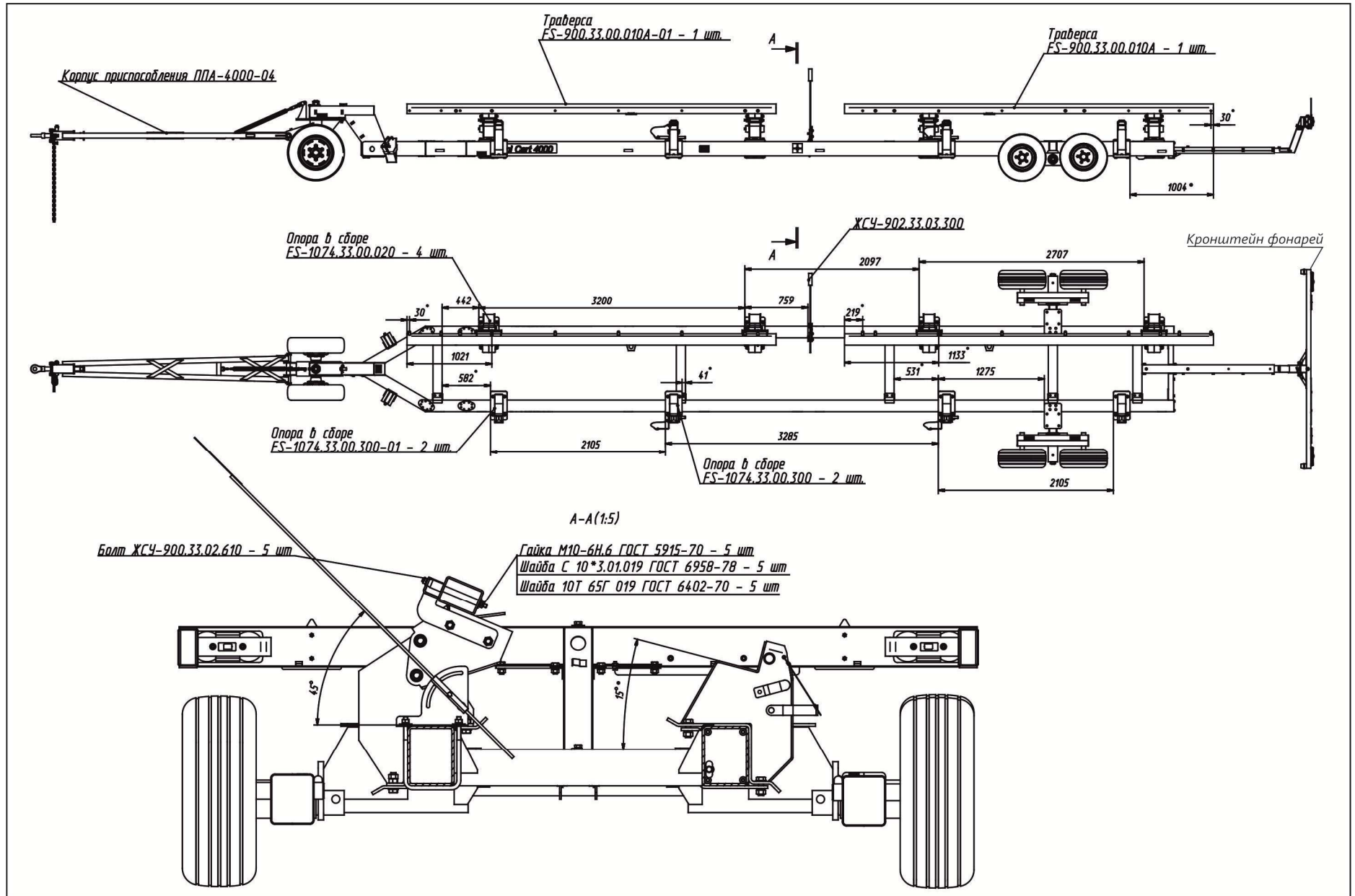
Рисунок 8.2 – Схема установки комплектов на тележку
