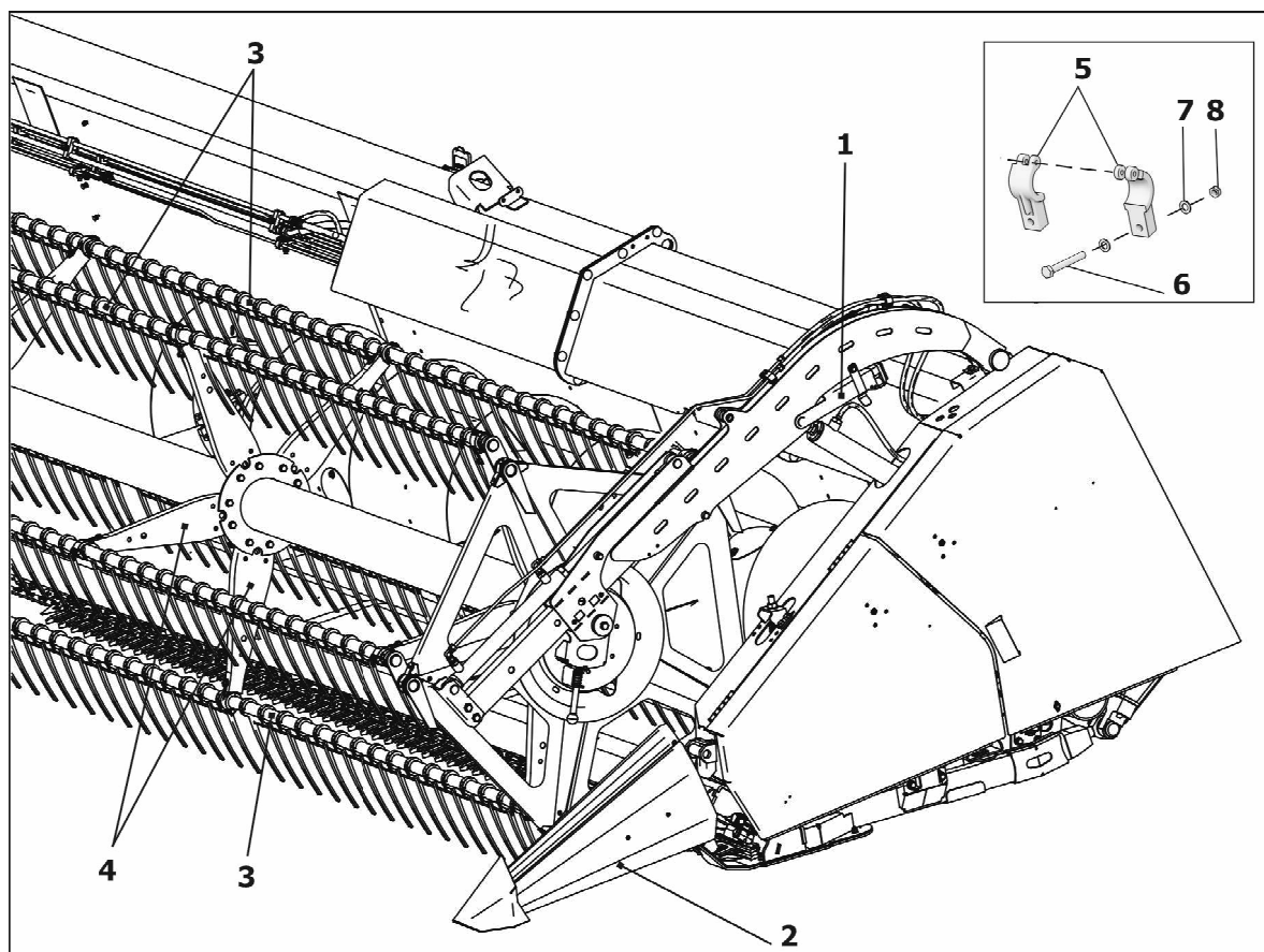
1-транспортная опора; 2-делитель; 3-граблина; 4-лопость 5-полуподшипник; 6-болт; 7-шайба; 8-гайка Рисунок 5.1 – Сборка
