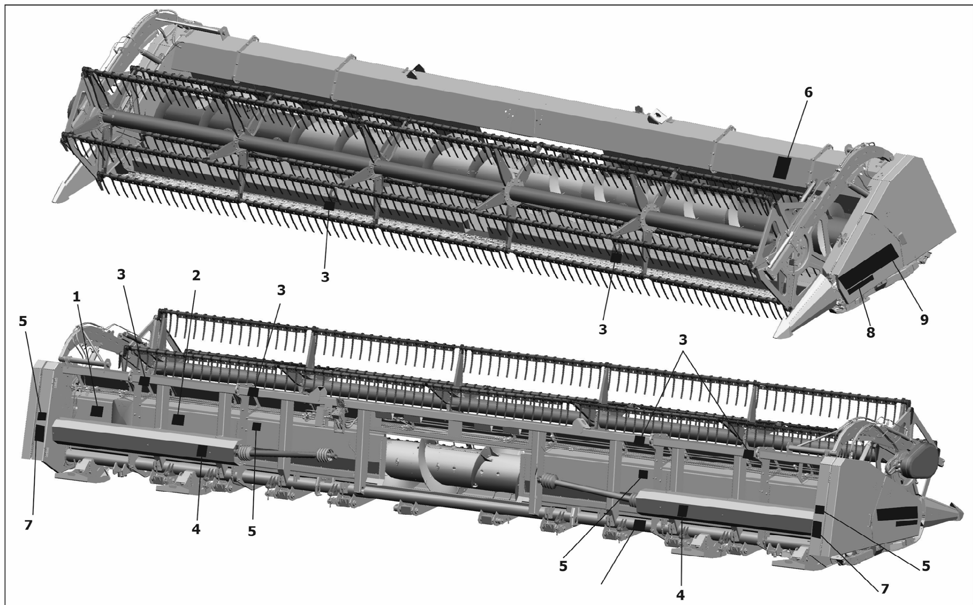
Рисунок 4.1 – Места расположения табличек и аппликаций на жатке
