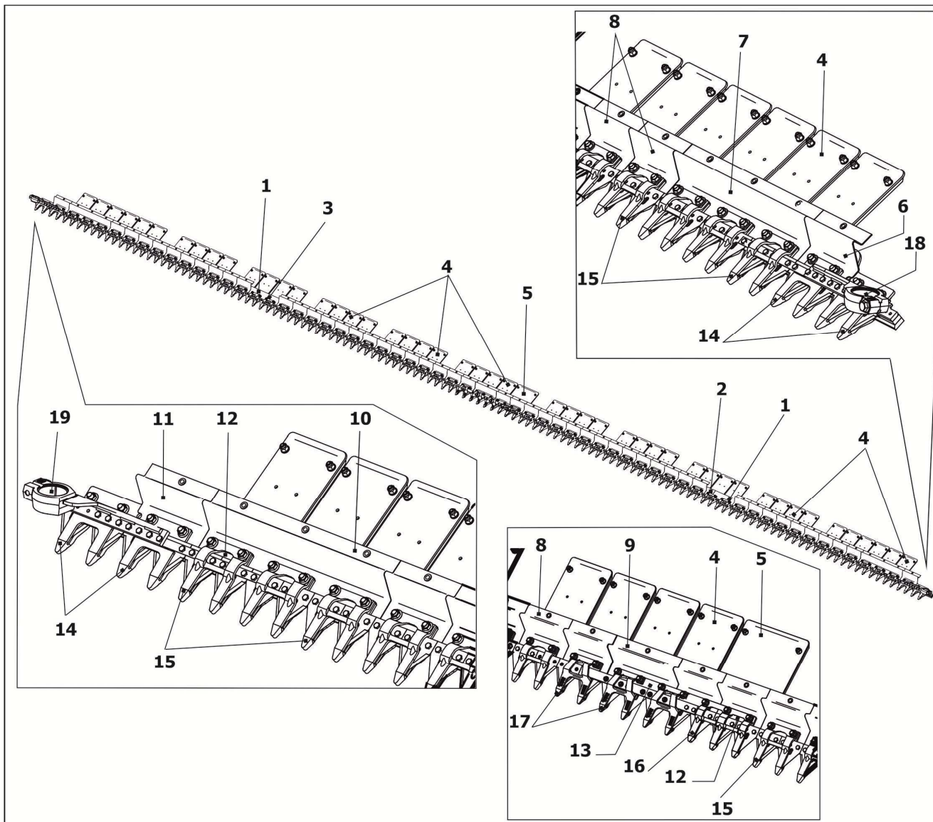
1, 2, 3—брус; 4, 5—опора; 6, 7, 8, 9, 10, 11—камнеотбойник; 12, 13—пластина трения; 14—палец двойной открытой; 15—палец двойной закрытой; 16—палец тройной закрытой; 17—палец двойной закрытой; 18, 19—нож Рисунок 2.5 – Режущий аппарат
