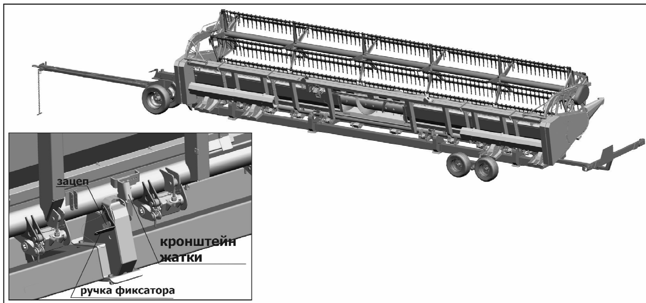
Рисунок 8.3 - Установка жатки на тележку ППА-4000-04
