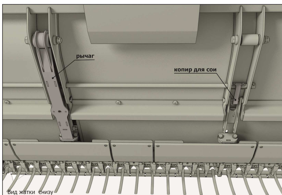
Рисунок 6.12 – Положение копирных дуг для уборки сои в режиме «с плавающим ножом»
