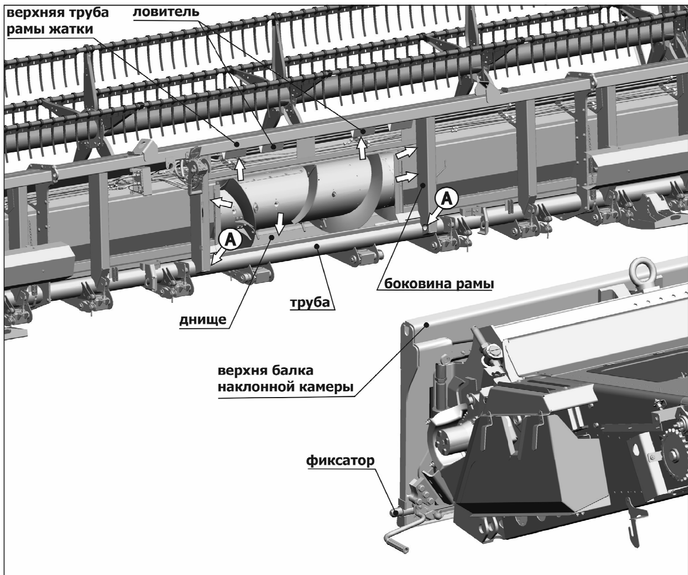
Рисунок 5.2 - Монтаж жатки на комбайн
