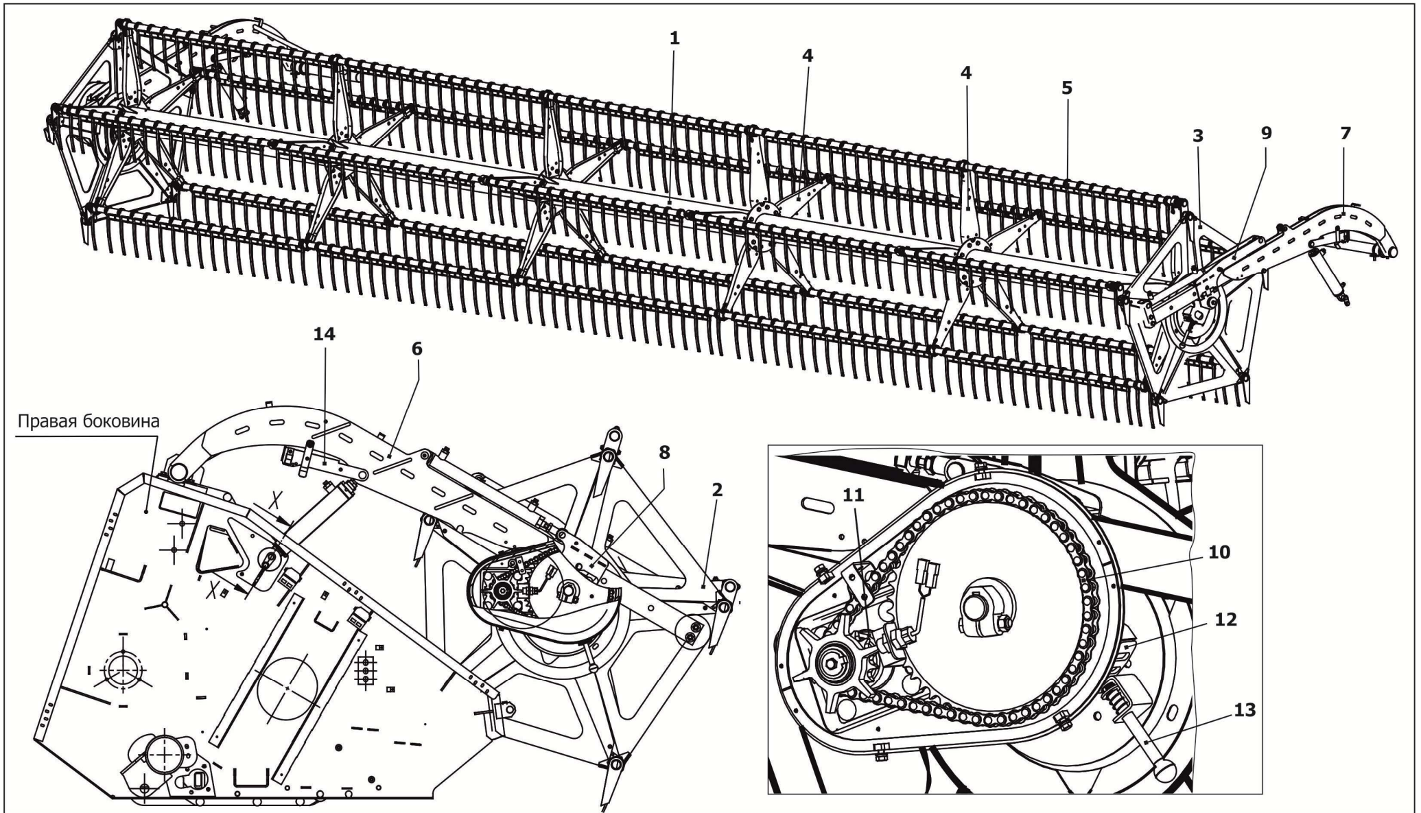
1-труба; 2, 3-эксцентрик; 4-лопасть; 5-граблина; 6, 7-поддержки; 8, 9-ползун; 10-цепная передача; 11-гидромотор; 12-сектор; 13-рукоятка; 14 - транспортная опора
