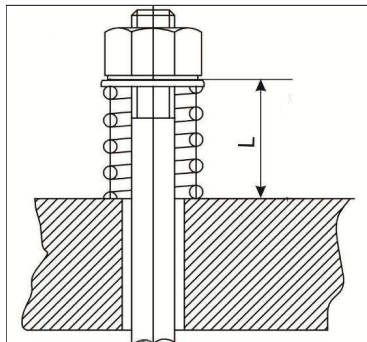
L – длина пружины
