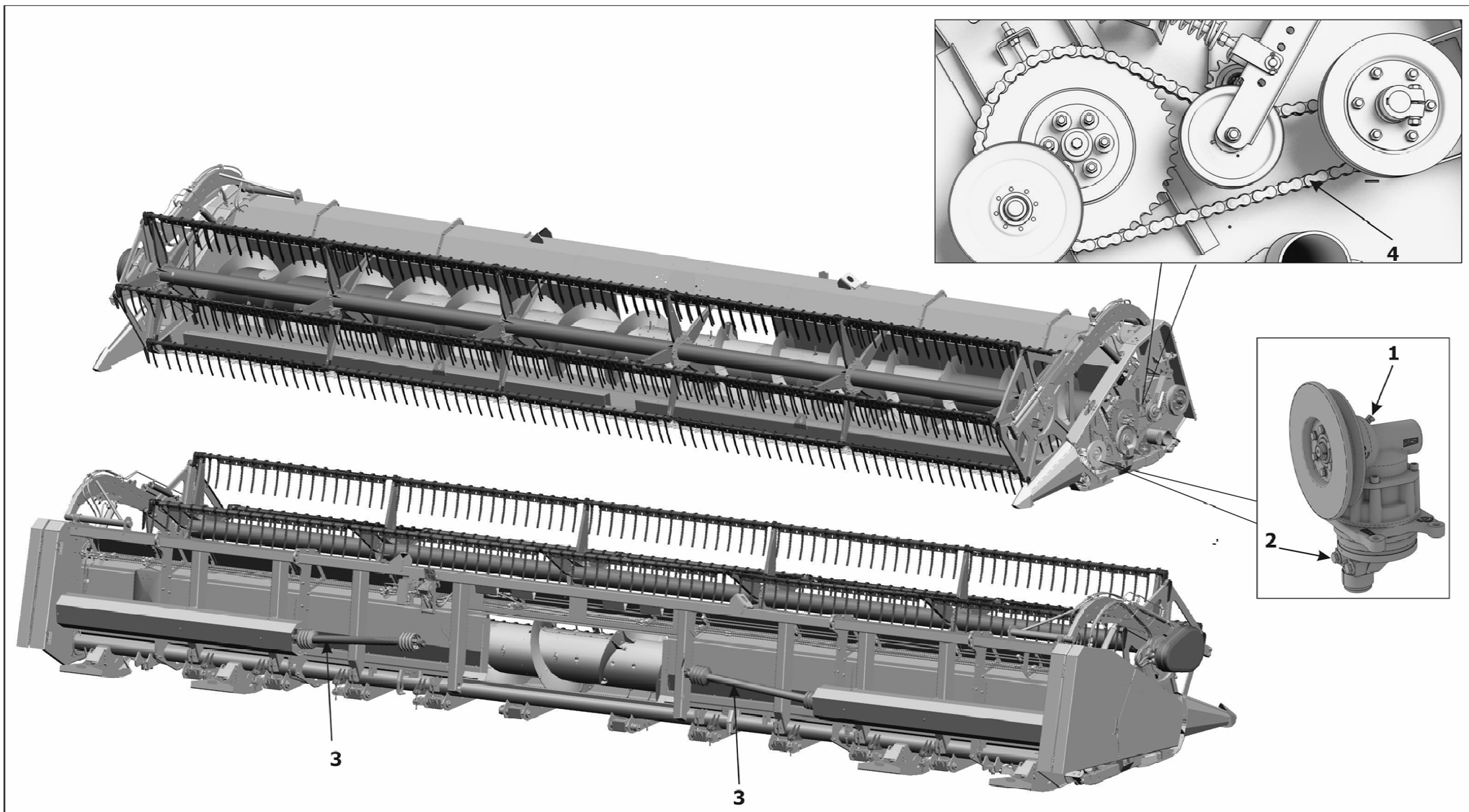
Рисунок 7.1 - Точки смазки жатки
