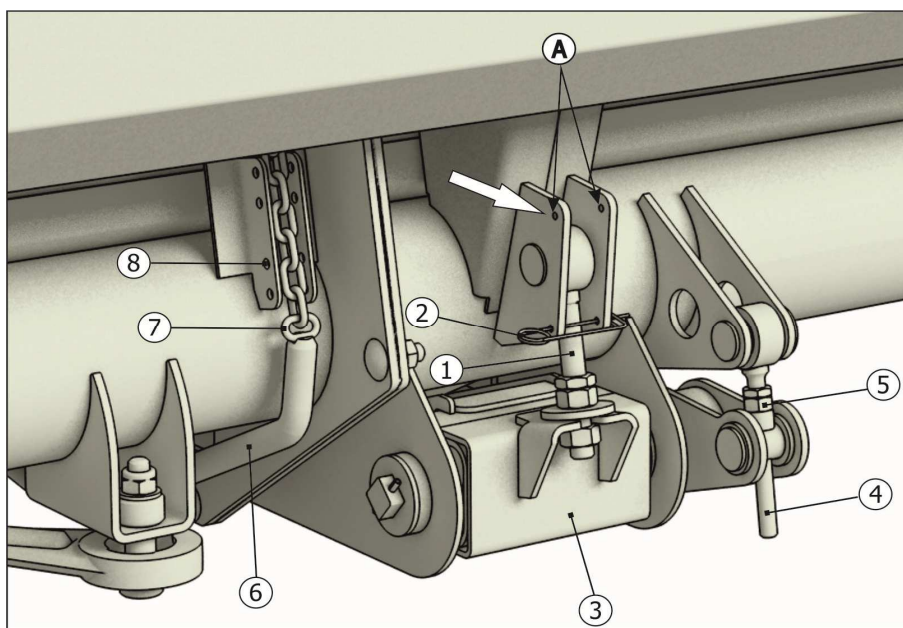
1-тяги; 2-защелка; 3-торсион; 4-тяги; 5-гайка; 6-копирная дуга; 7-цепь; 8-болтокрепеж А-отверстие
