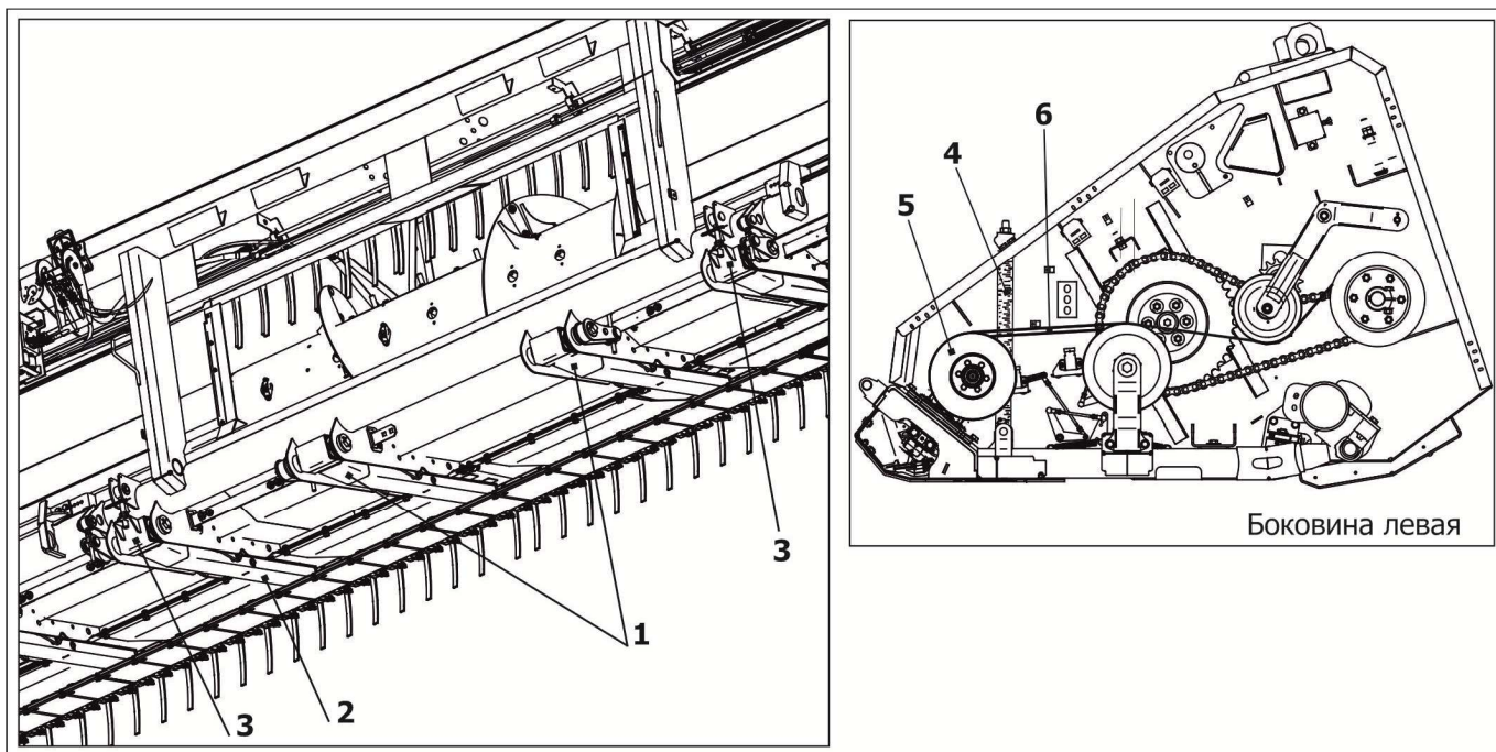
1, 2-центральный рычаг; 3-торсион; 4-пружина вывешивания; 5-редуктор Pro-Drive; 6-клиноременная передача
