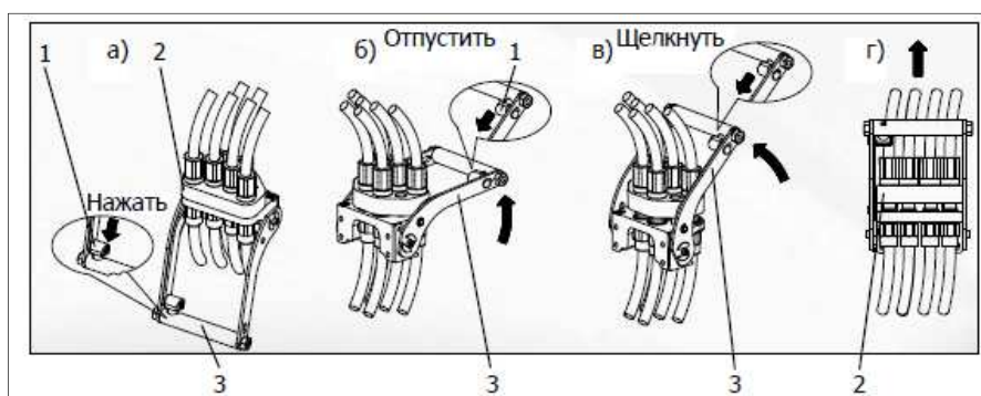
1-предохранительная кнопка; 2-подвижная часть единого гидроразъема; 3-рукоятка
