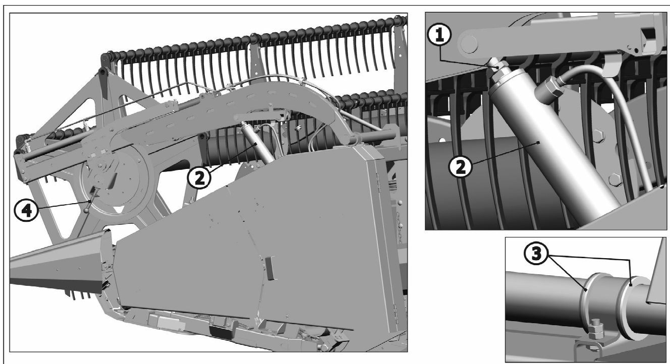
1-гайка; 2-гидроцилиндр подъема мотовила; 3-шайба; 4-рукоятка
