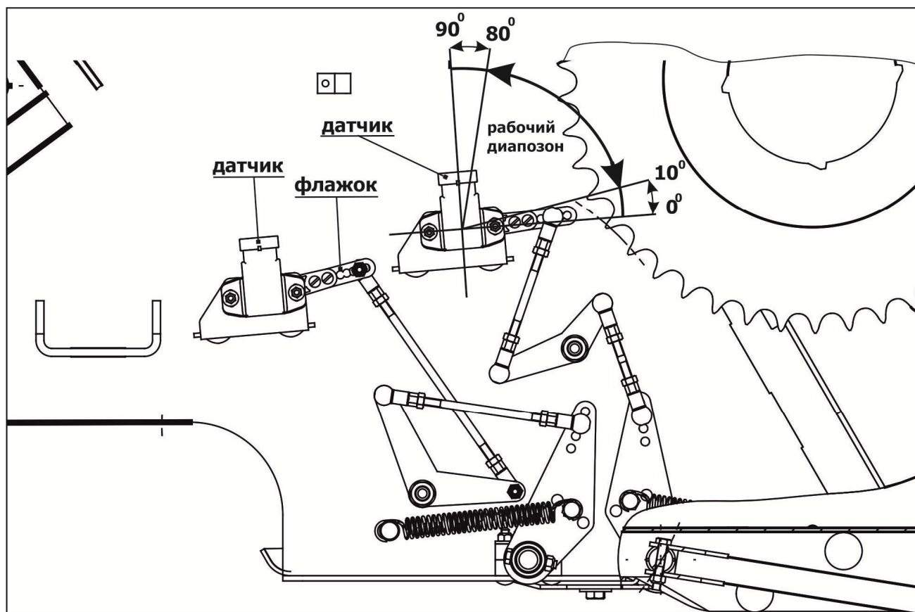
Рисунок 6.9 – Рабочий диапазон датчика
