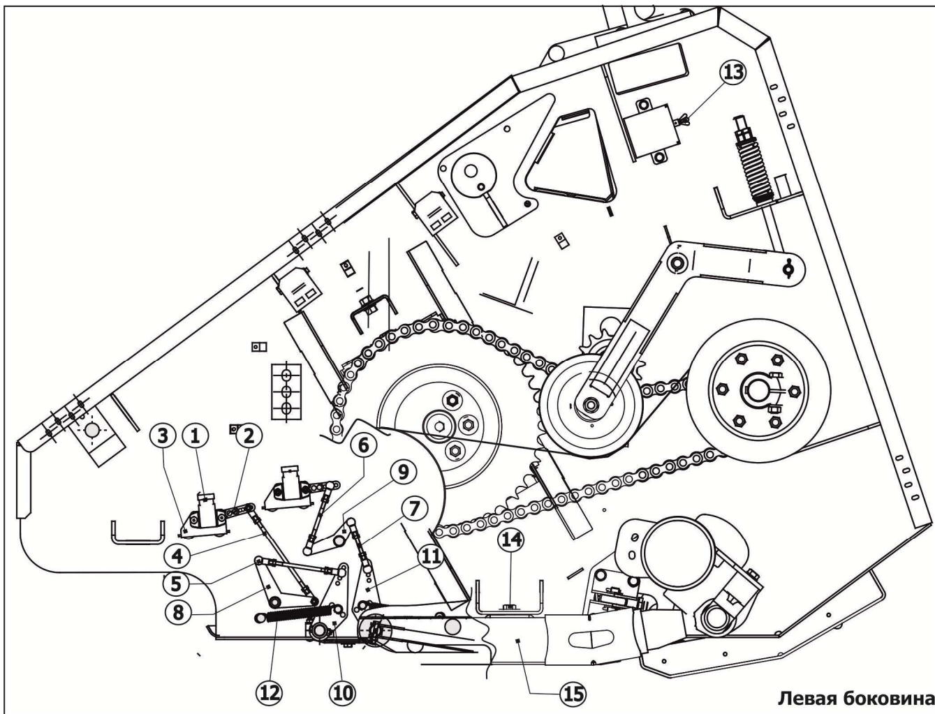
1-датчик; 2-флажок; 3-кронштейн; 4, 5, 6, 7-тяги; 8, 9-коромысло; 10, 11-кронштейн; 12-пружина; 13 –переключатель; 14-болткрепеж; 15-боковой рычаг
