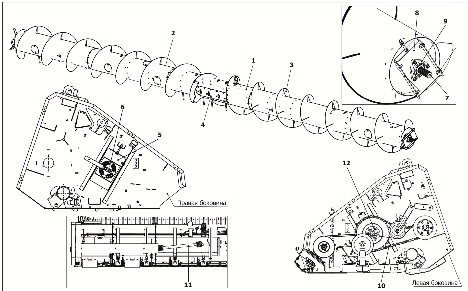
1-труба; 2, 3- правая и левая винтовая лента; 4-пальчиковый механизм; 5, 8-плита; 6 – втулка; 7-вал; 9-подшипниковая опора; 10-цепная передача; 11-вал карданный; 12-муфта
