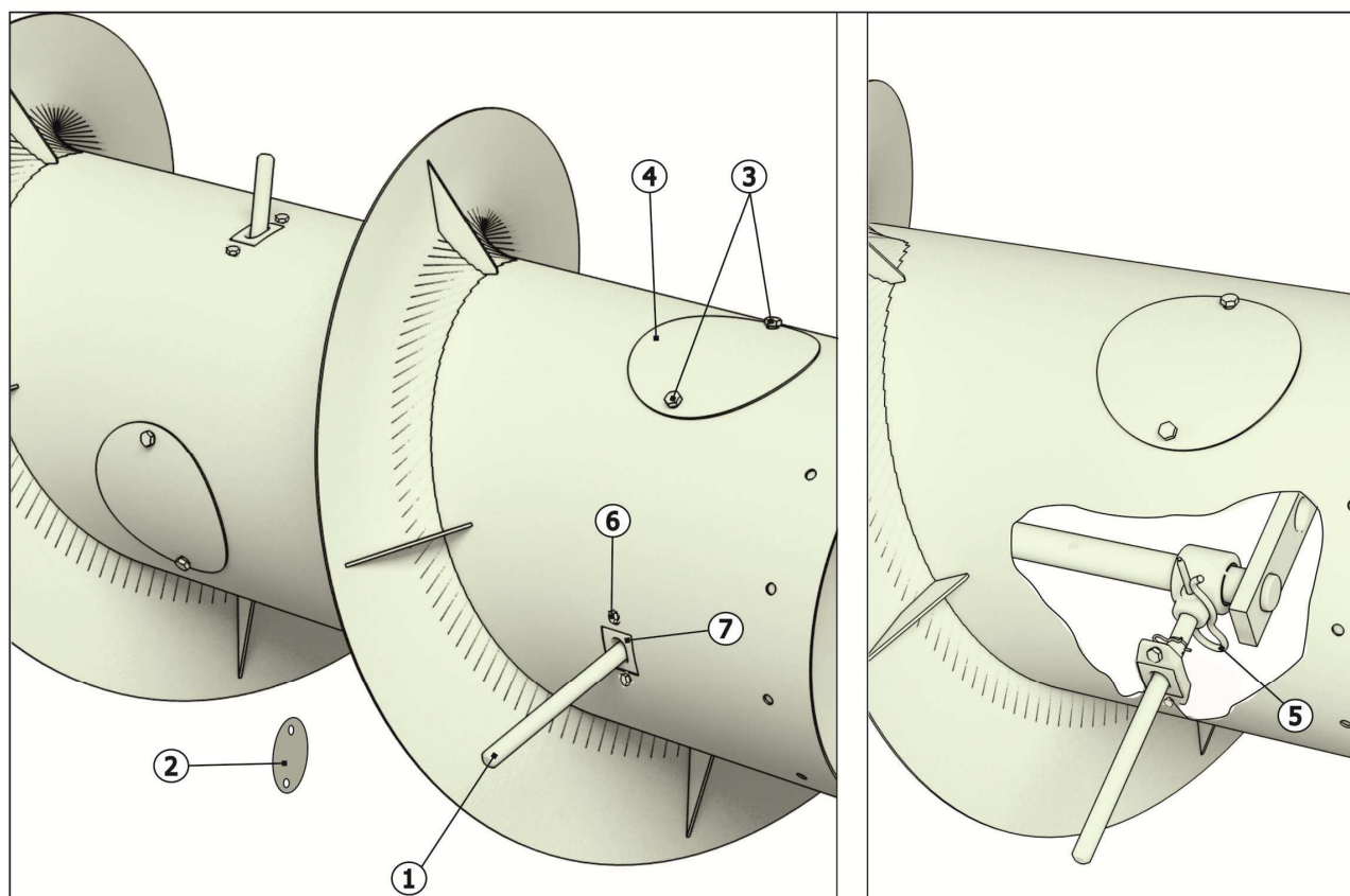
1-палец шнека; 2-крышка из комплекта ЗИП; 3, 6-болтокрепеж; 4-крышка; 5-фиксатор; 7-глазок пальца Рисунок 6.8 – Демонтаж пальцев на шнеке
