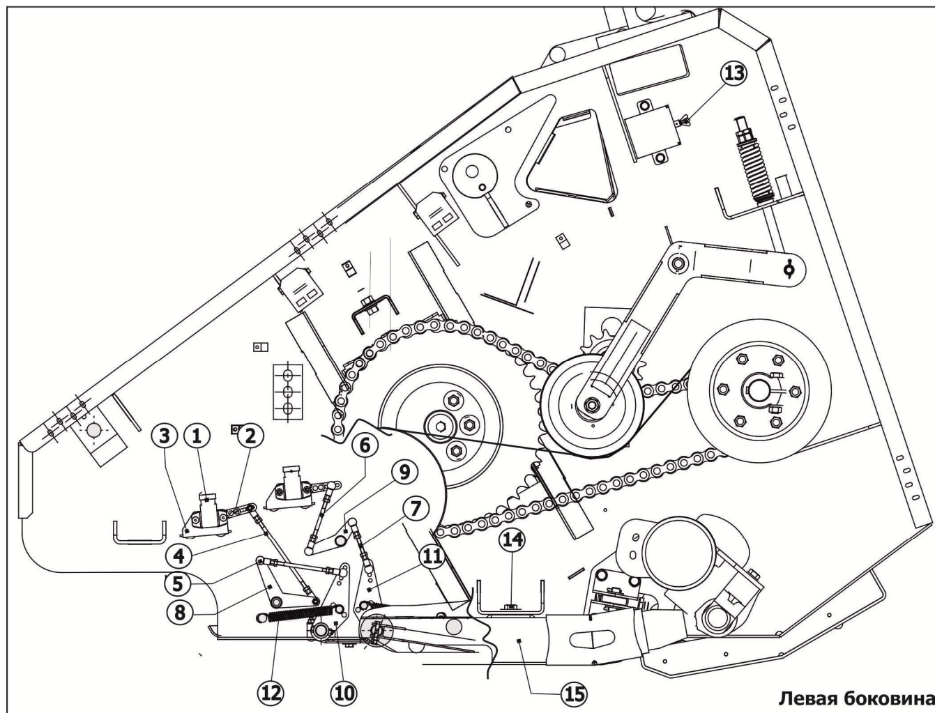
Рисунок 6.10 – Система датчиков автоконтура. Левая боковина
