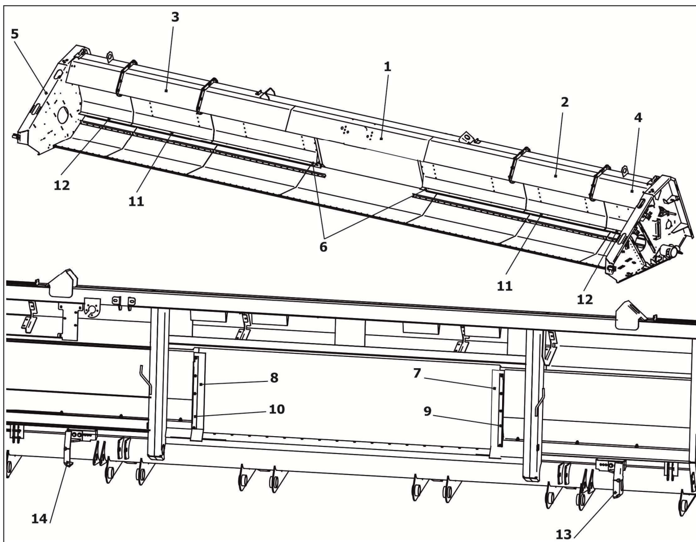
1—рама центральная; 2,3—средняя рама; 4—правая боковая рама; 5—левая боковая рама; 6, 9, 10, 11, 12—чистик; 7, 8—ремень; 13, 14—кронштейн
