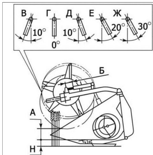
Рисунок 6.4 - Положения граблин мотовила
