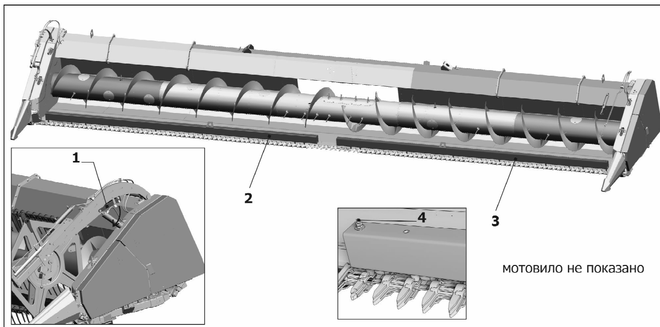
1-транспортная опора; 2, 3-траверса; 4-болтокрепеж
