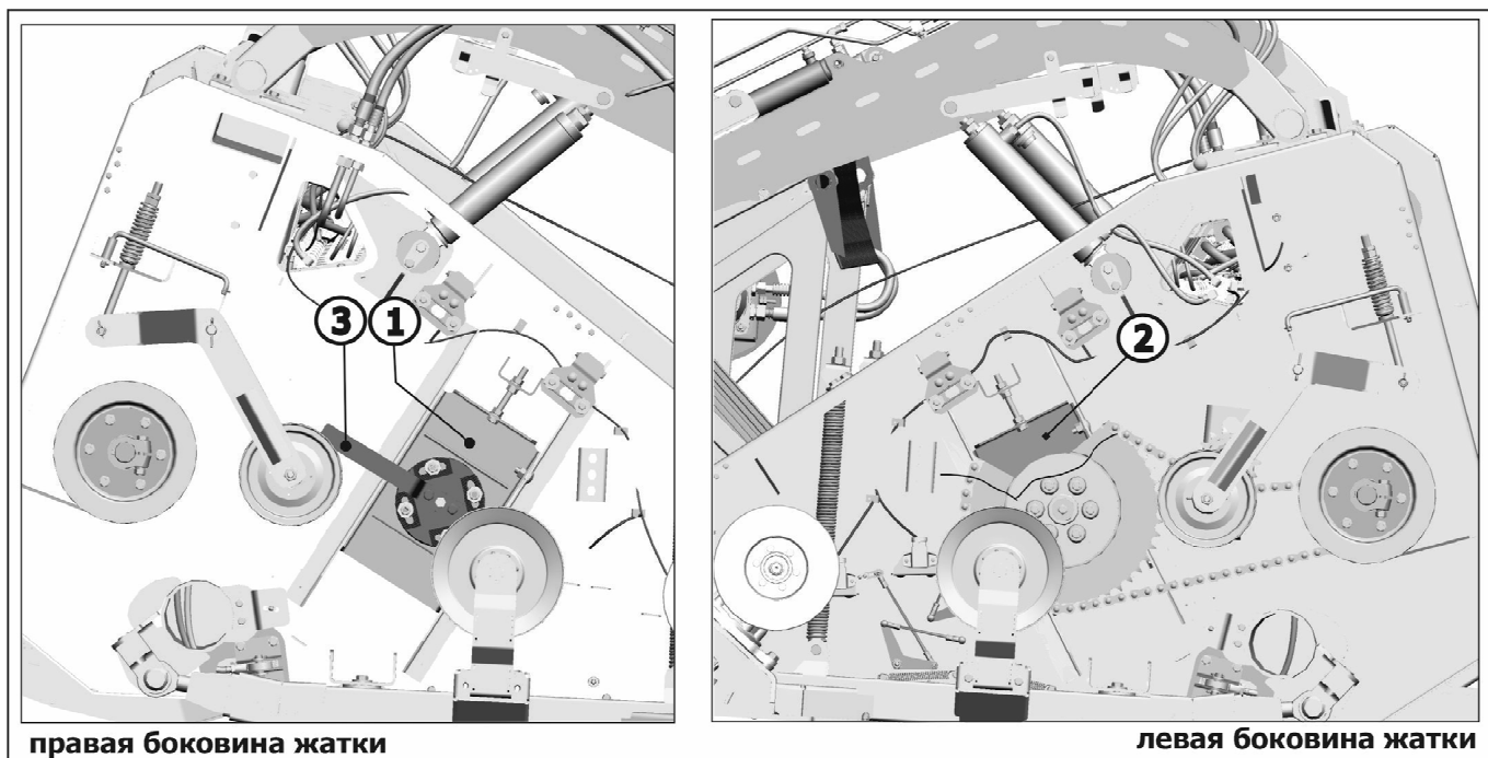
Рисунок 6.6 – Регулировка шнека
