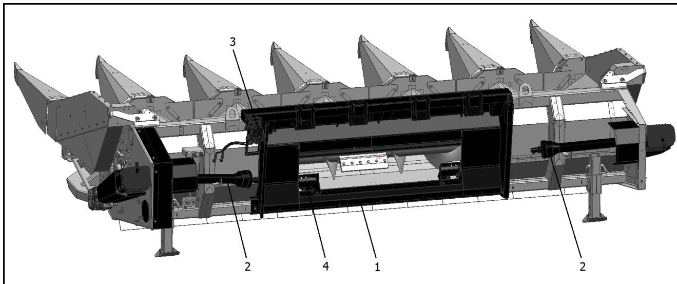
1 – Рамка; 2 – Приводной карданный вал; 3 – ЕГР; 4 – Кронштейн Рисунок 2.19 – Комплект для агрегатирования RSM CS-670-50
