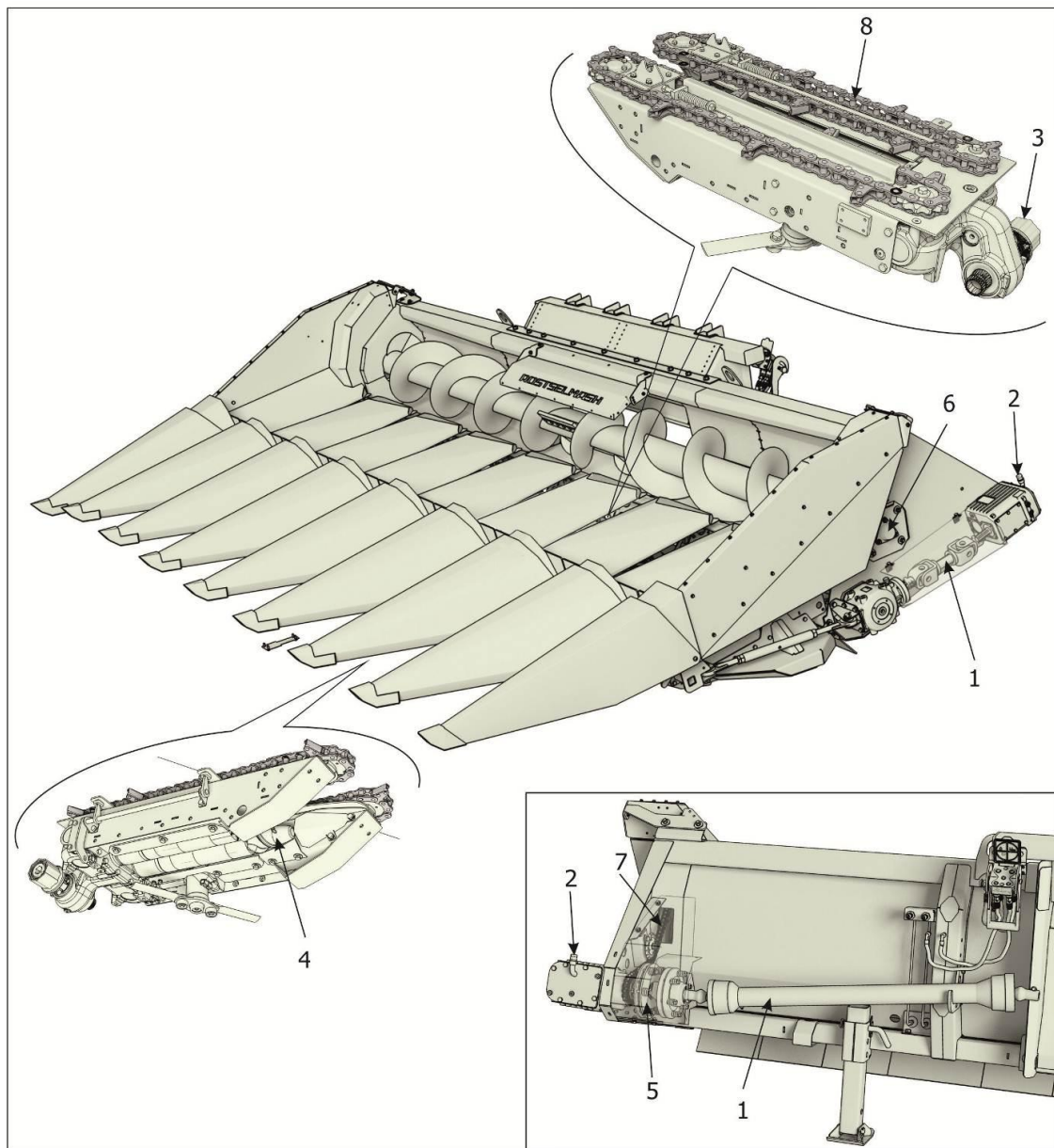
Рисунок 9.1 – Смазка жатки
