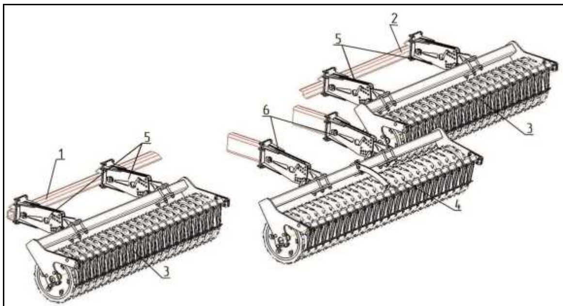
1 – крыло левое; 2 – крыло правое; 3 – каток МД-880.30.200, 4 – каток МД-880.30.200; 5 – подвеска МД-880.30.300-01, 6 – подвеска МД-880.30.300
