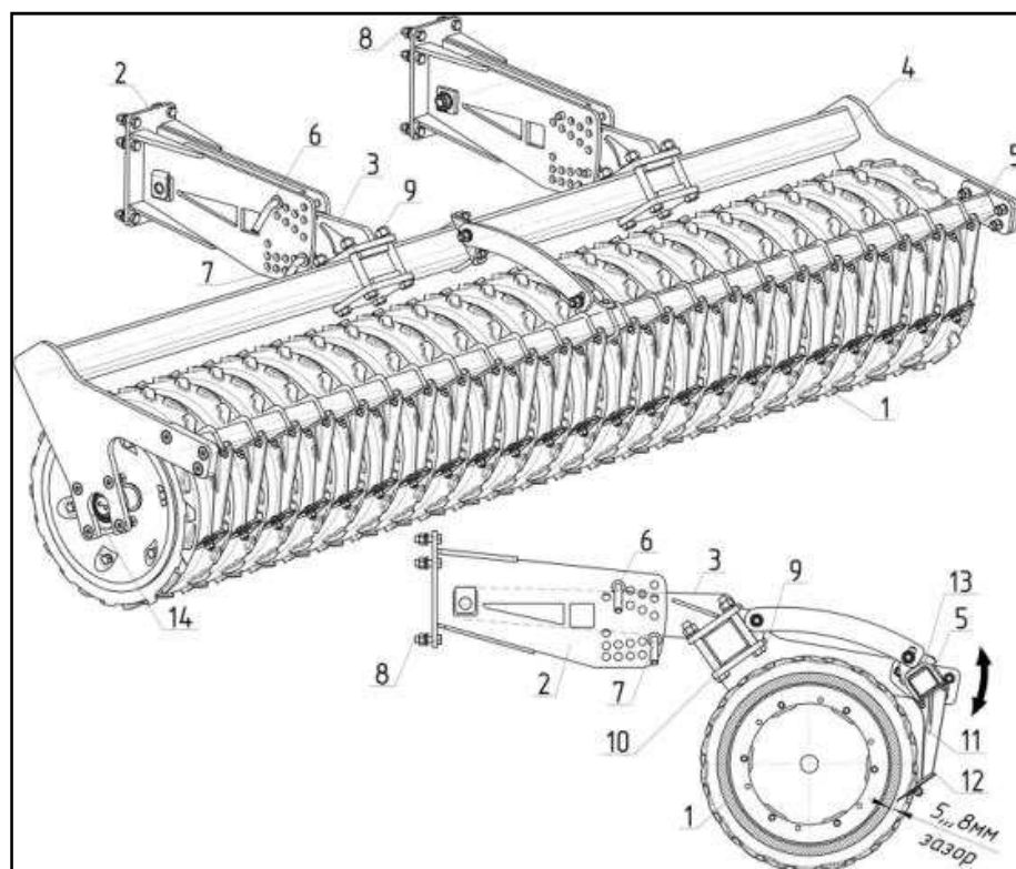
1 – каток 540x2900; 2 – кронштейн МД-800.30.040; 3 – стойка МД-880.30.020; 4 – рама МД-880.30.110; 5 – труба чистиков МД-880.30.130; 6 – штырь (верхний) МД-800.30.060; 7 – штырь (нижний) МД-800.30.060; 8 – болт М16-6gx55.88.35.019 ГОСТ 7798-70; 9 – болт М20-6gx150.88.019 ГОСТ 7798-70; 10 – плита МД-800.30.030; 11 – стойка чистика; 12 – чистик; 13 – хомут чистика; 14 – подшипниковая опора
