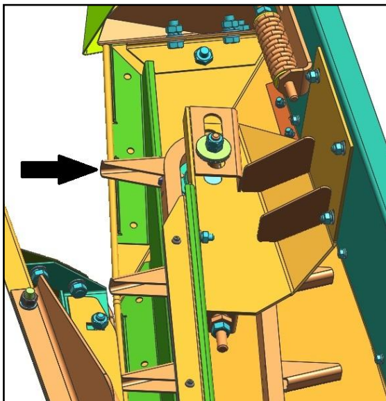
Рисунок 2.3 – Транспортёр стеблей
