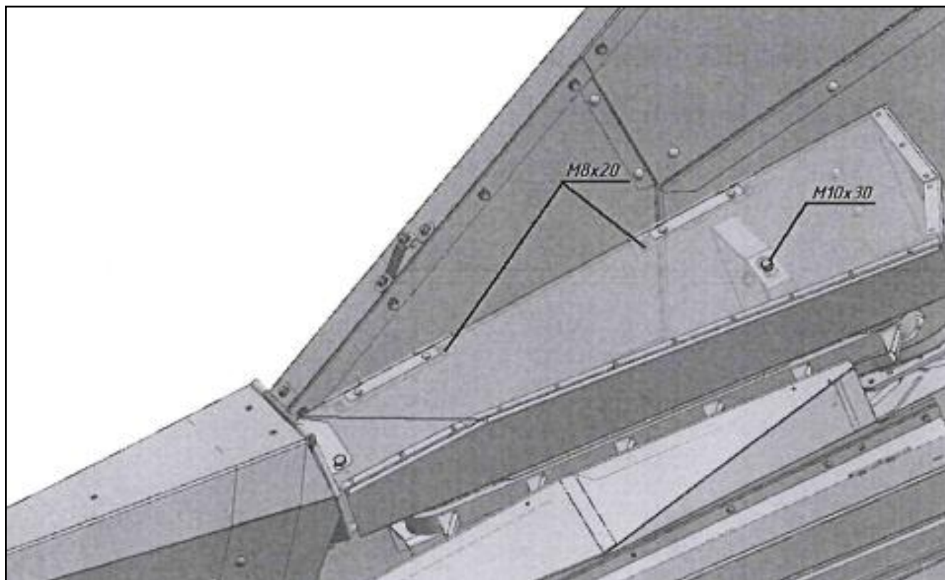
Рисунок 2.7 – Демонтаж скатков
