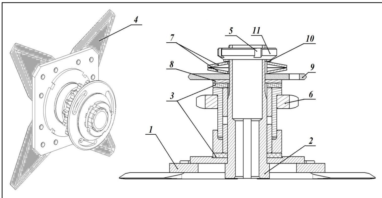
1 – Диск ножевой; 2 – Втулка шлицевая; 3 – Фрикционная накладка; 4 – Нож; 5 – Шайба стопорная; 6 – Звездочка транспортера стеблей; 7 – Тарельчатая пружина; 8, 9 – Шайба упорная; 10 – Шайба; 11 – Гайка
