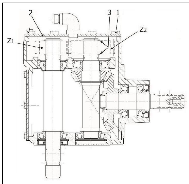
1 – Болт; 2 – Съемная задняя крышка; 3 – Стопорное кольцо Z1, Z2 – Сменные зубчатые колеса Рисунок 8.6 – Редуктор боковой (коробка передач)
