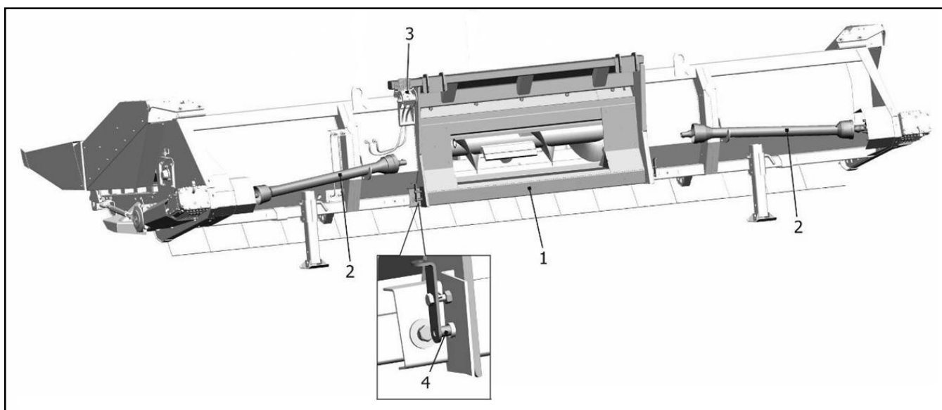
Рисунок 2.15 – Комплект для агрегатирования RSM CS-870-49
