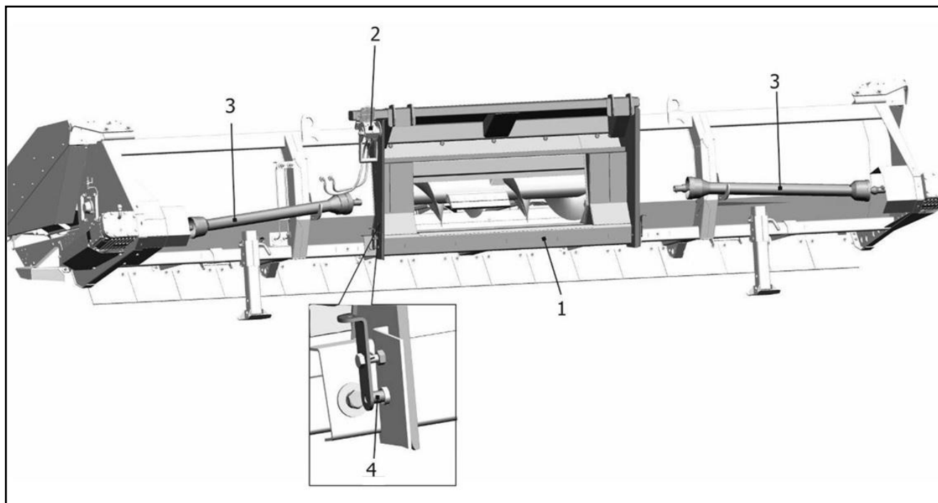
Рисунок 2.14 – RSM CS-870-47 Комплект для агрегатирования
