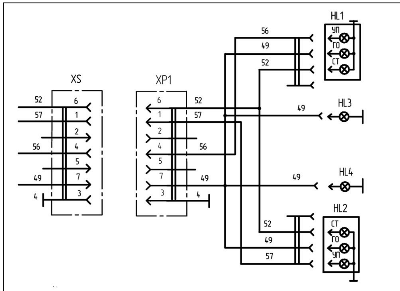
XP1– вилка; XS – розетка ПС300А3; HL1, HL2 – Фонарь задний; ФП-132; HL3, HL4 – Фонарь передний16.3712 Рисунок Г.1 – Схема электрическая принципиальная
