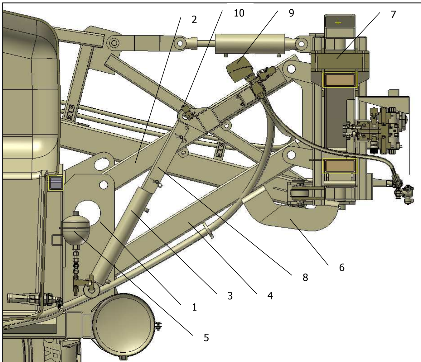
1 – Рама; 2 – Верхний рычаг; 3 – Гидроцилиндры подъема; 4 – Нижний рычаг; 5 – Пневмогидроаккумулятор; 6 – Фиксатор штанги в верхнем положении от раскочки; 7 – Штанга; 8 – Стопор гидроцилиндров подъема; 9 – Блок секционных клапанов; 10 – Блок электропневмоклапанов отключения концевых форсунок Рисунок 3.3 – Механизм подъема штанги
