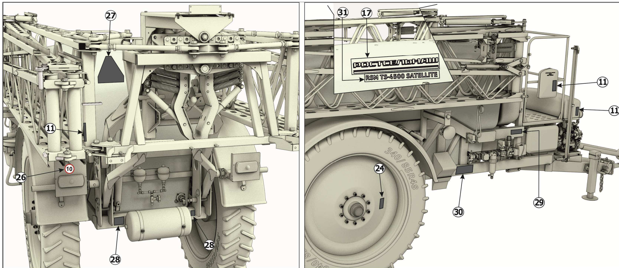
Рисунок 4.2 – Месторасположение табличек на опрыскивателе
