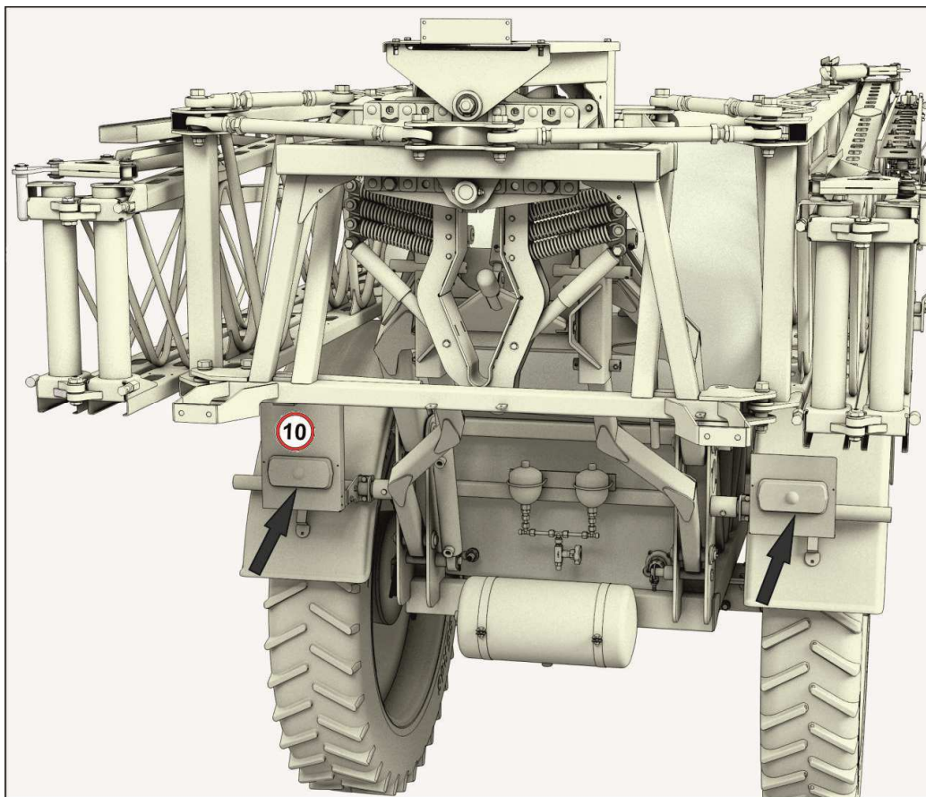
Рисунок 3.18 – Задние фонари
