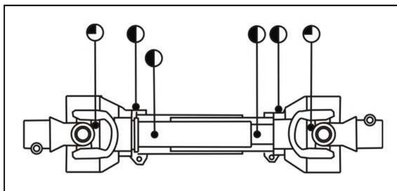
Рисунок 7.1 – Точки смазки карданного вала
