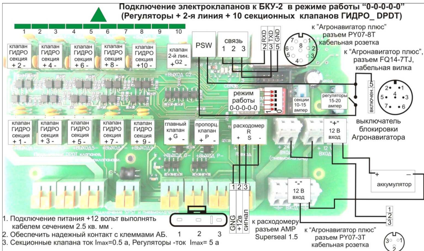
Рисунок 3.14 – Принципиальная электрическая схема системы управления нормой расхода рабочей жидкости
