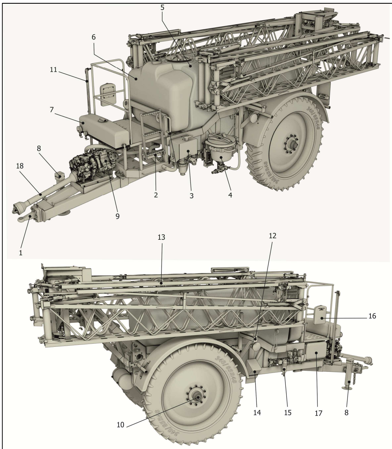
1 – Сница; 2 – Лестница площадки для обслуживания; 3 – Панель управления; 4 – Миксер; 5 – Основная емкость; 6 – Промывочная емкость; 7 – Емкость для мытья рук; 8 – Домкрат; 9 – Насос; 10 – Мост колес; 11 – Уровень наполнения основной емкости; 12 – Ложемент; 13 – Штанга; 14 – Противооткатный упор; 15 – Регулятор-распределитель рабочей жидкости; 16 – Пенал для документации; 17 – Ящик для СИЗ и ЗИП; 18 – Вал карданный Рисунок 3.1 – Общий вид опрыскивателя RSM TS-4500/36
