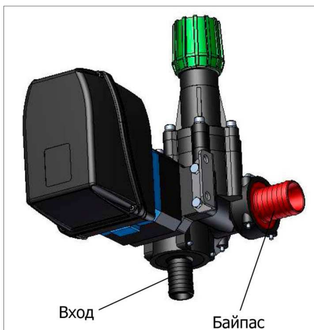
Рисунок 3.12 – Главный клапан
