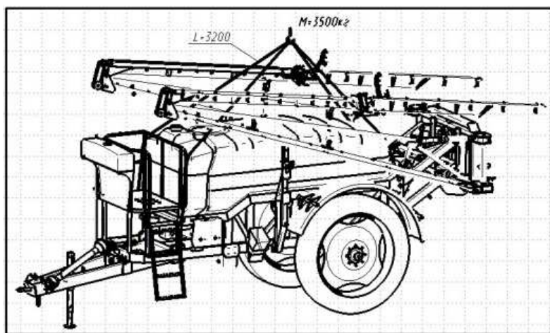
Рисунок 8.1 – Схема строповки
