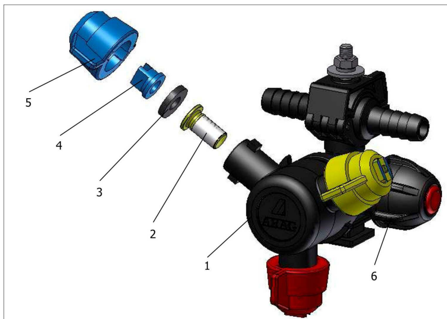
1 – Соплодержатель; 2 – Фильтр; 3 – Прокладка; 4 – Форсунка; 5 – Колпачек; 6 – Отсечной клапан
