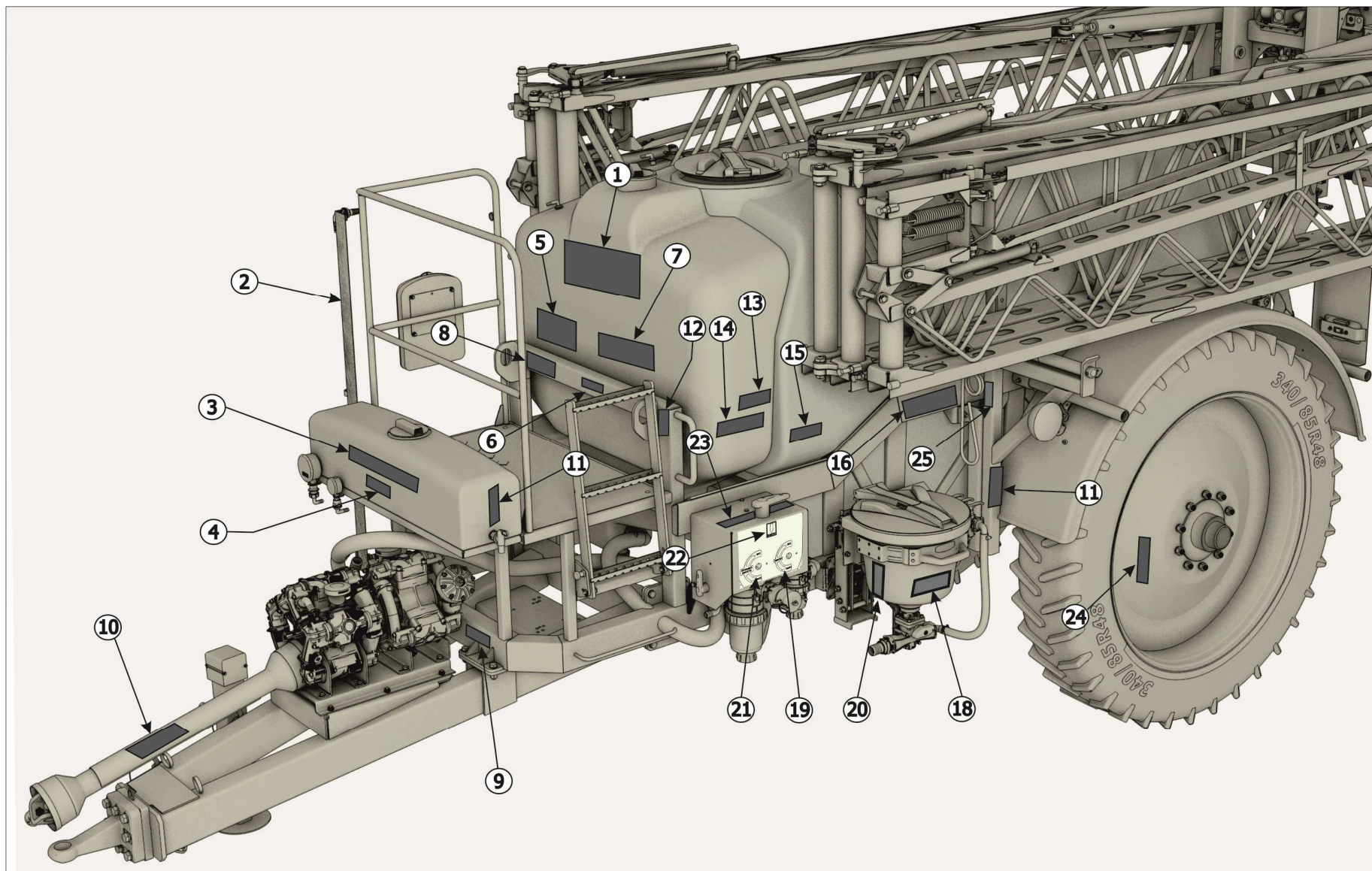
Рисунок 4.1 – Месторасположение табличек на опрыскивателе
