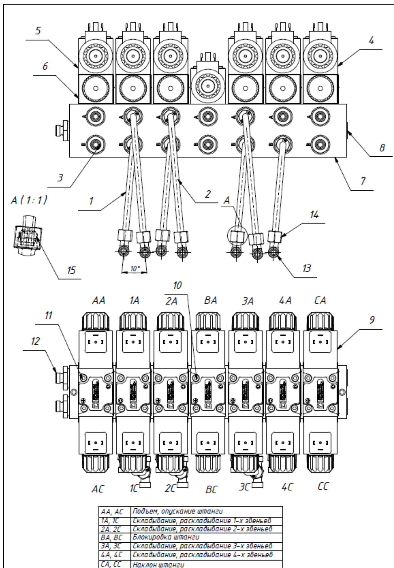
Рисунок Б.3 – Гидроблок
