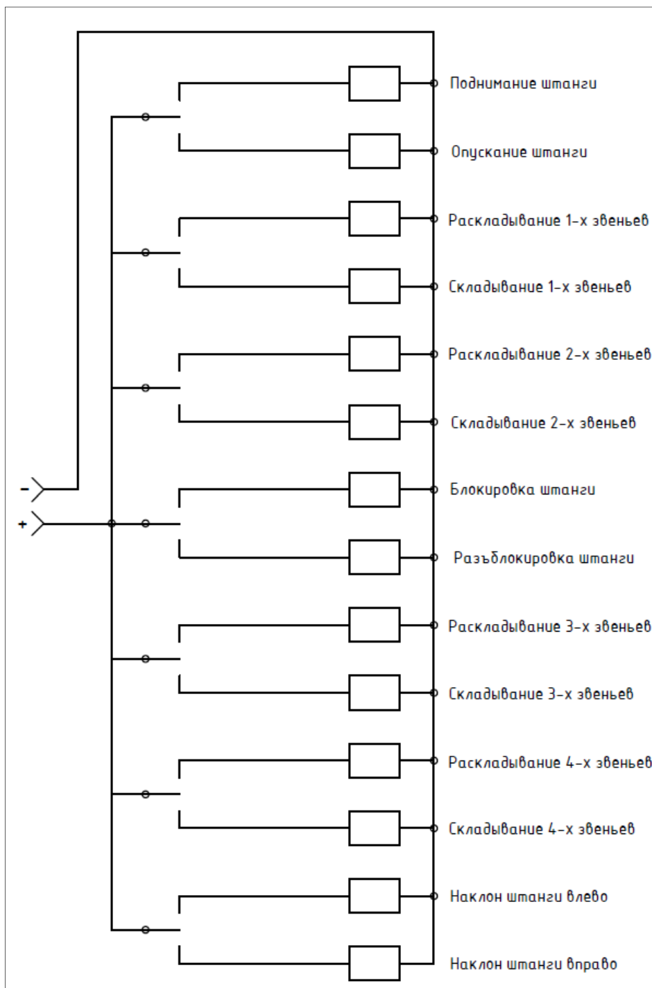
Рисунок 3.15 – Принципиальная электрическая схема гидравлической системы управления штангой
