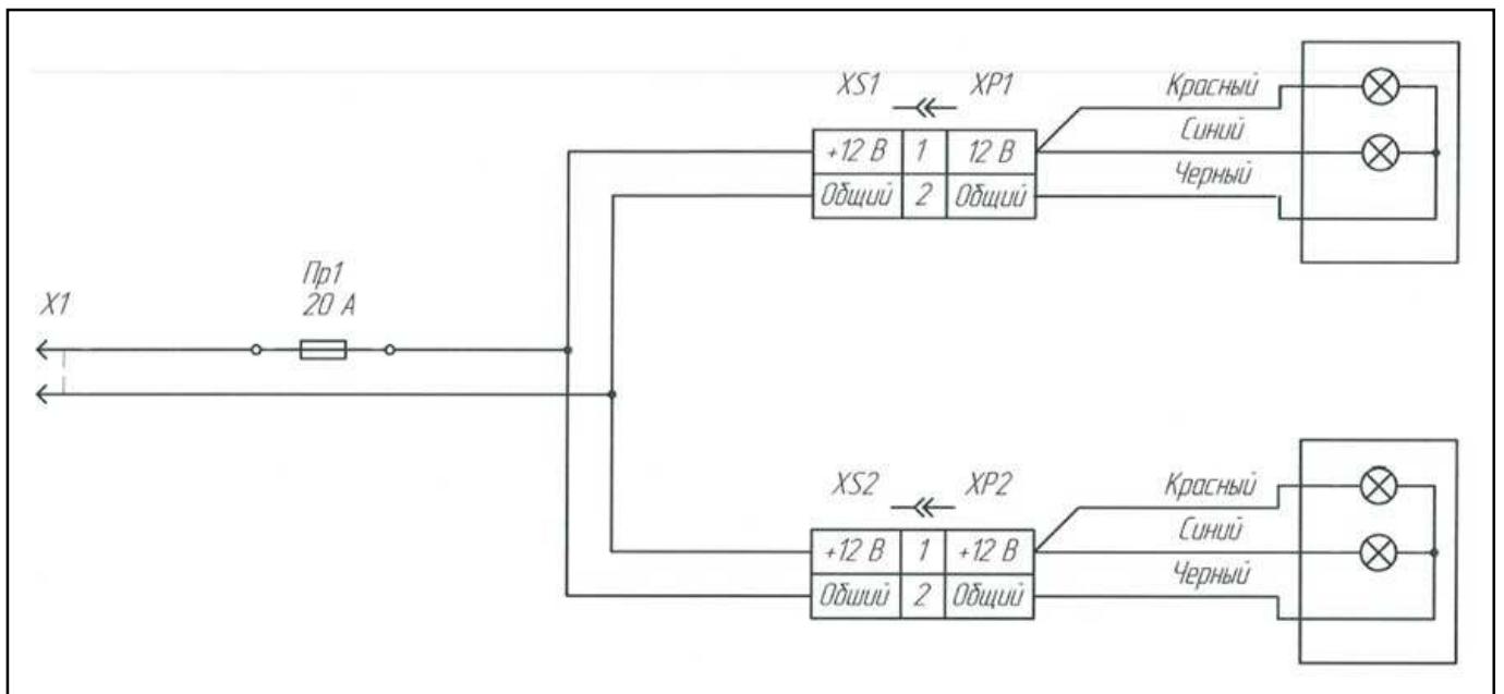
Рисунок 3.22 – Схема жгута фар для освещения штанги
