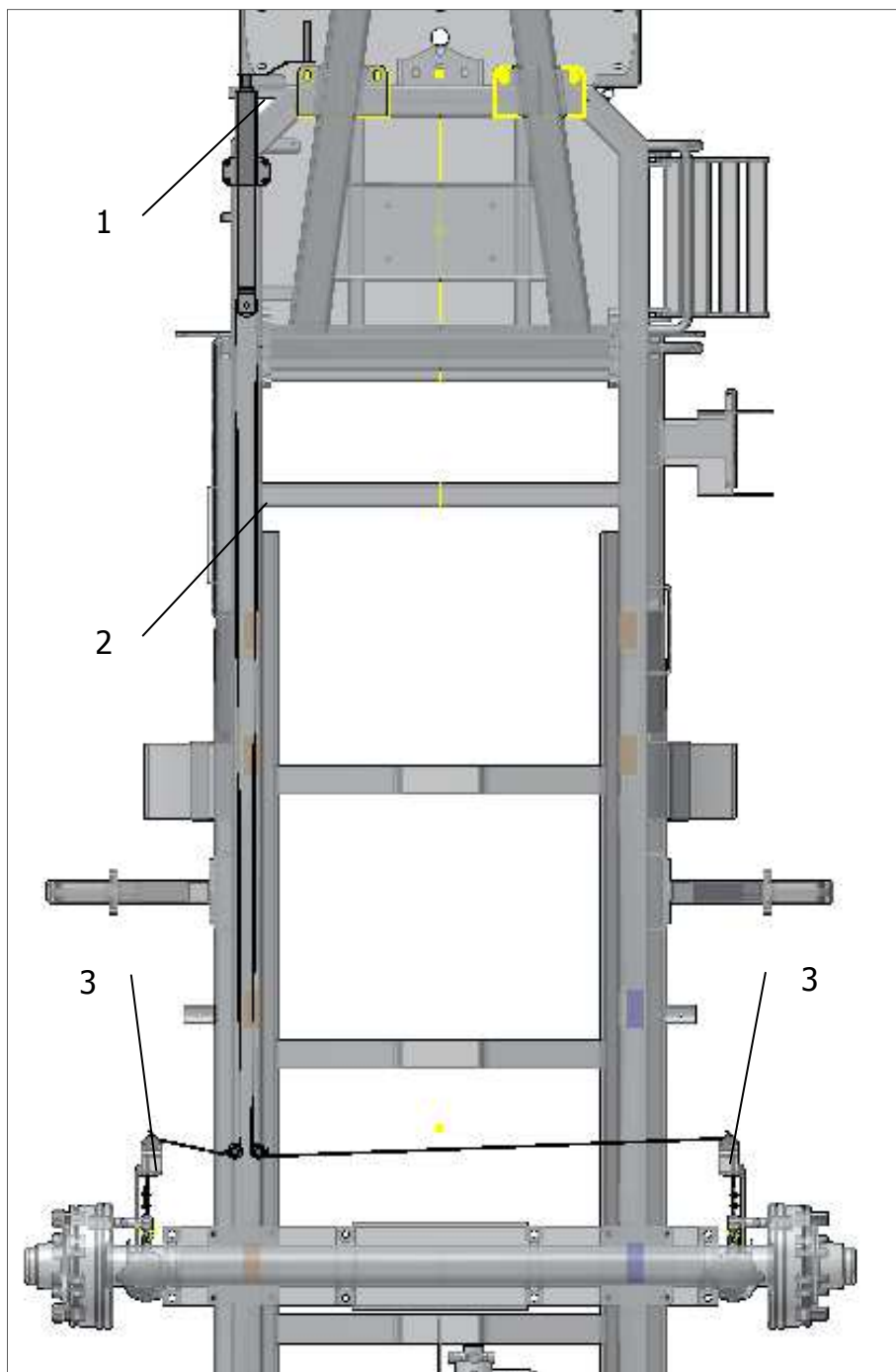
1 – Привод стояночного тормоза; 2 – Трос; 3 – Ролик Рисунок 3.17 – Стояночная тормозная система
