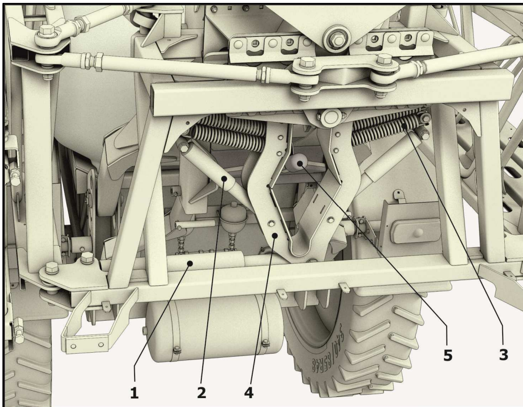
1 – Гидроцилиндр наклона штанги; 2 – Амортизатор; 3 – Пружина; 4 – Маятник; 5 – Замок Рисунок 3.2 – Штанга. Центральное звено
