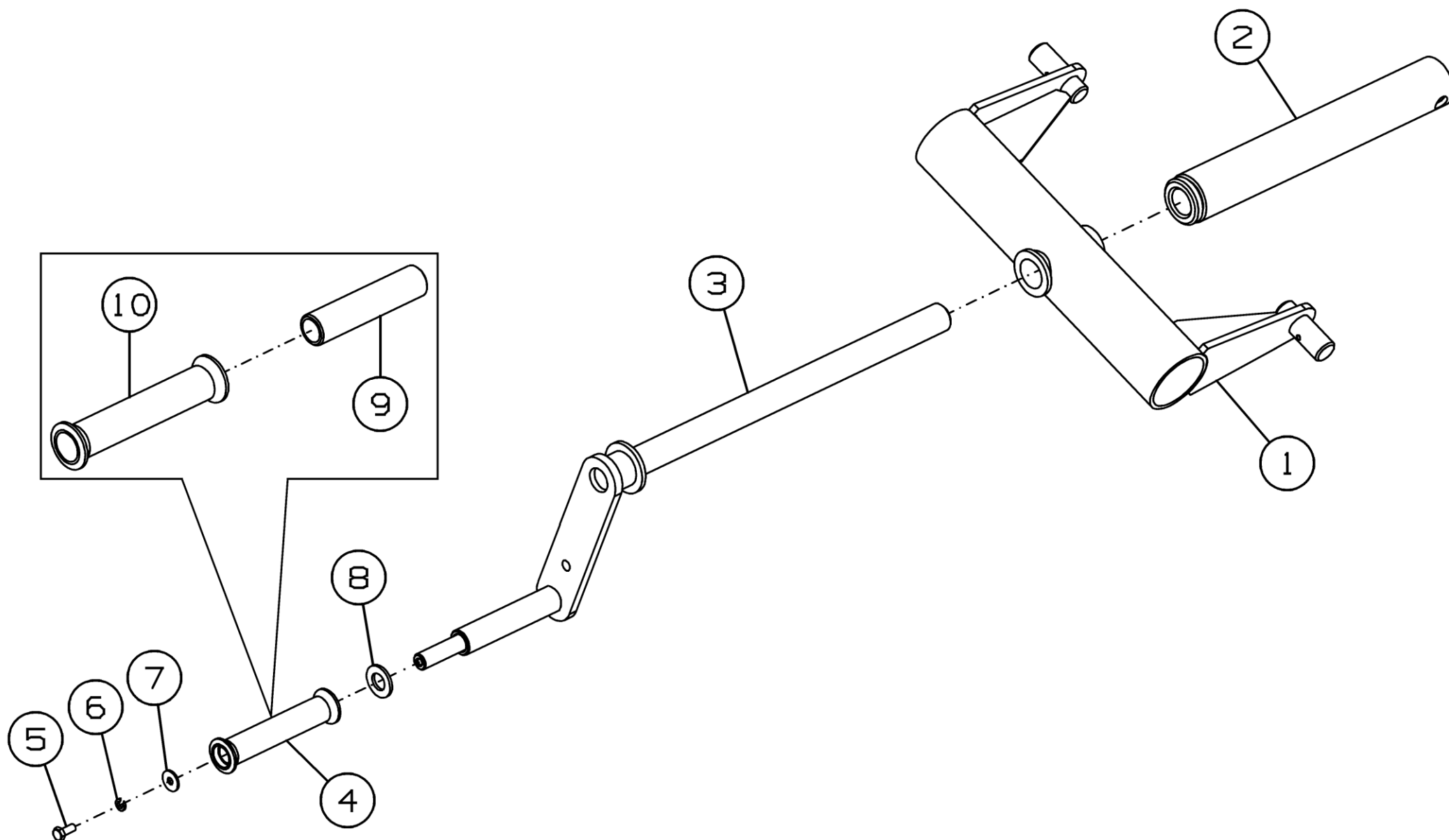
Рисунок 8 - Механизм подъема МЗС-150.01.740А
