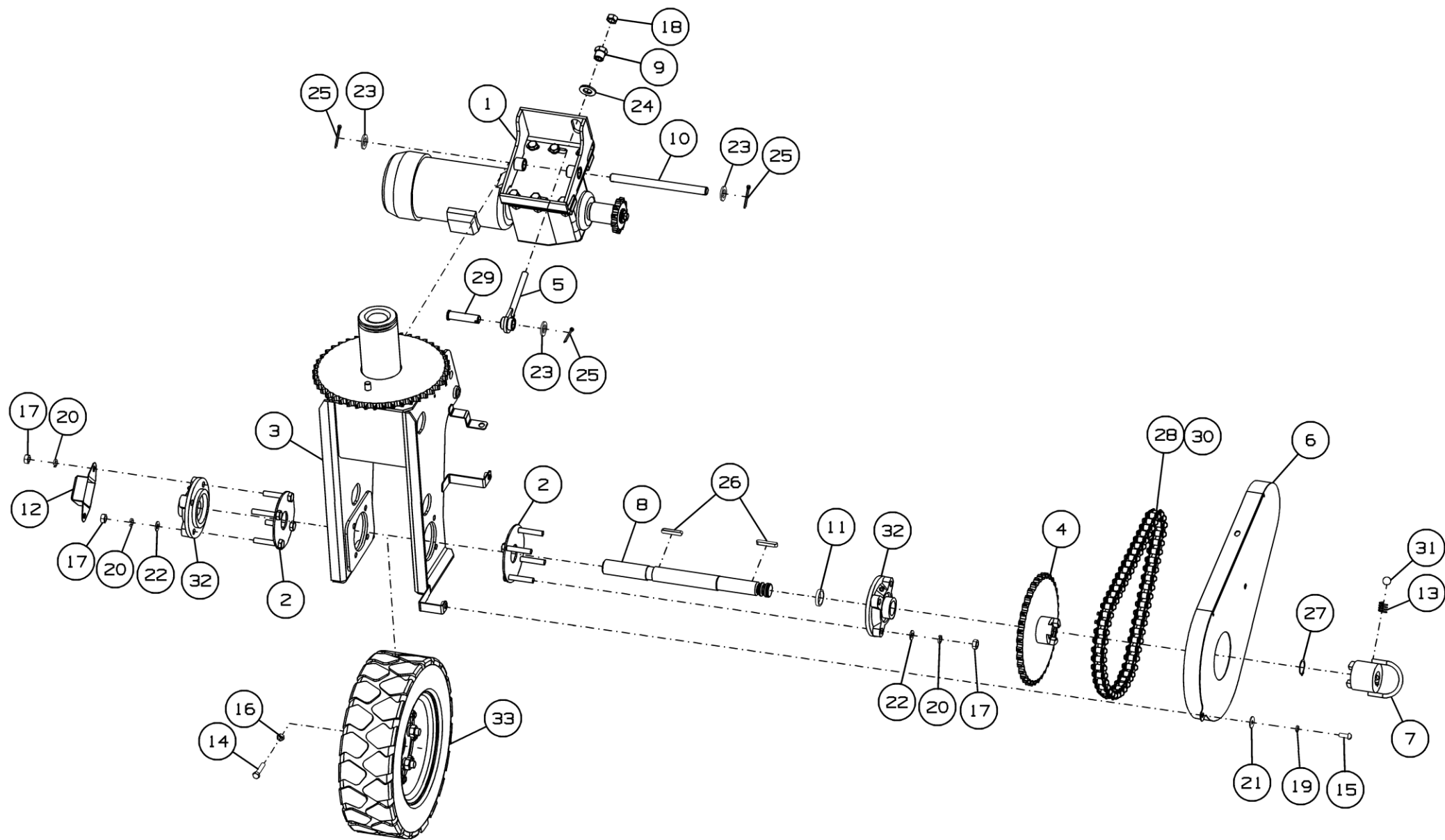
Рисунок 5 - Ход передний МЗМ-150.01.090
