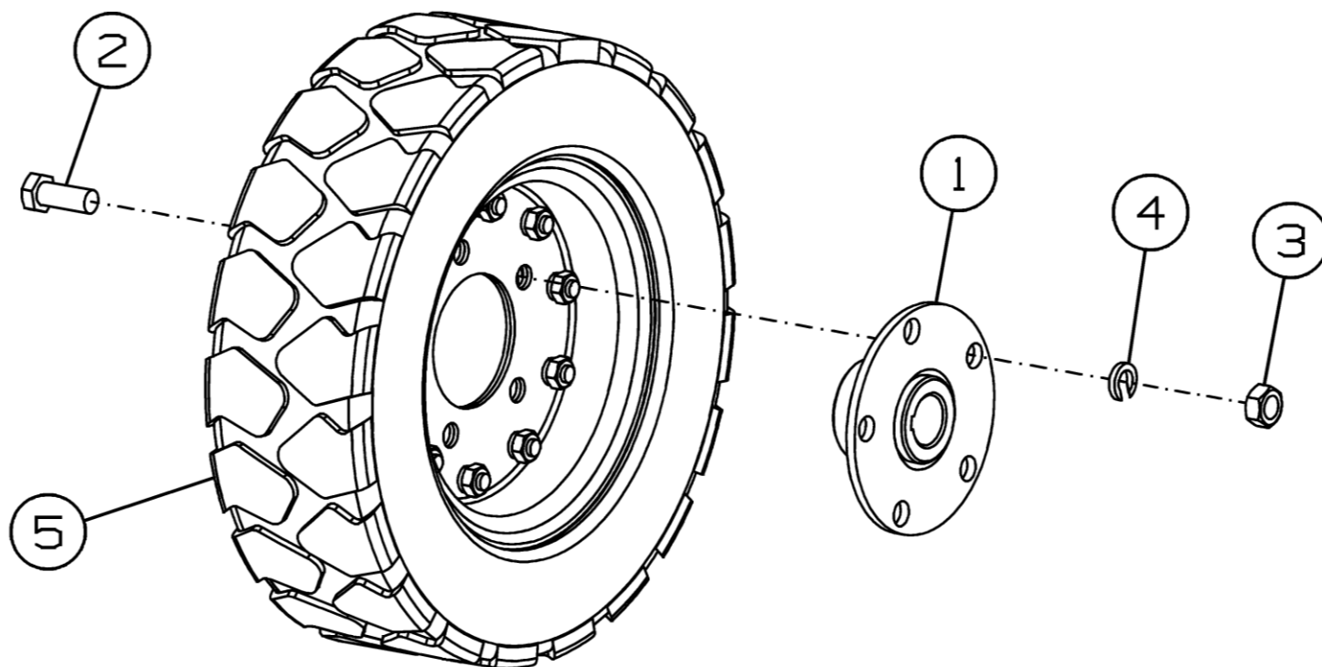
Рисунок 7 - Колесо переднее МЗС-150.01.270
