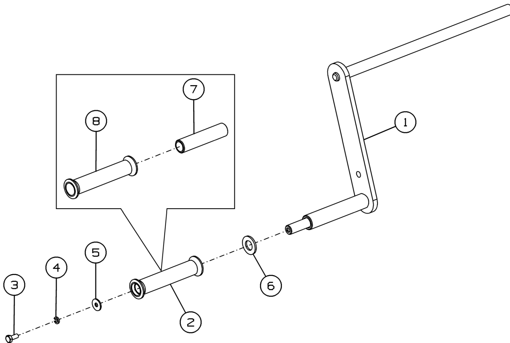
Рисунок 29 -Рукоятка МЗС-150.04.100
