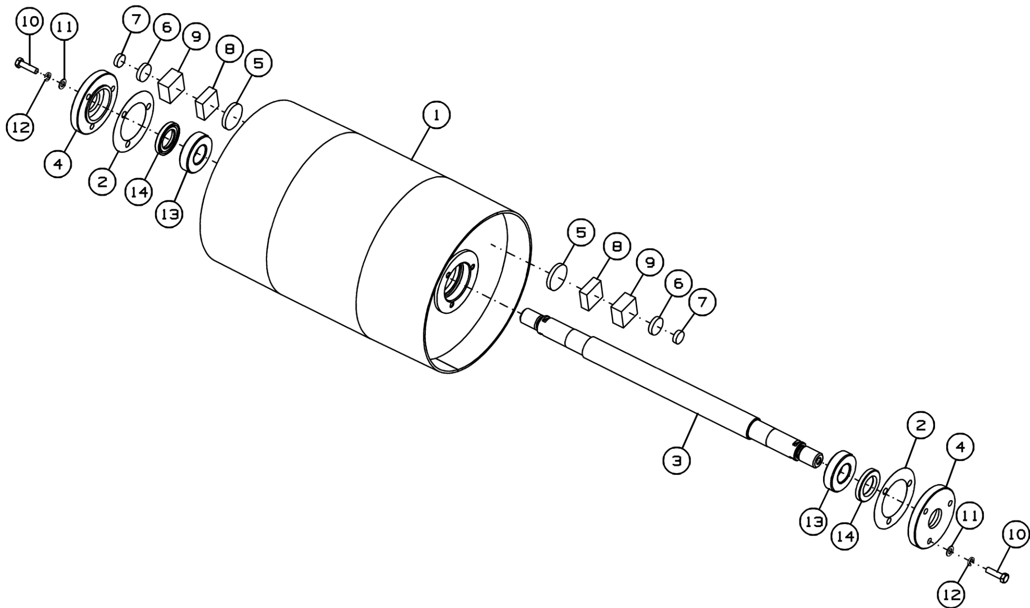
Рисунок 14 - Барабан натяжной МЗС-150.02.080А
