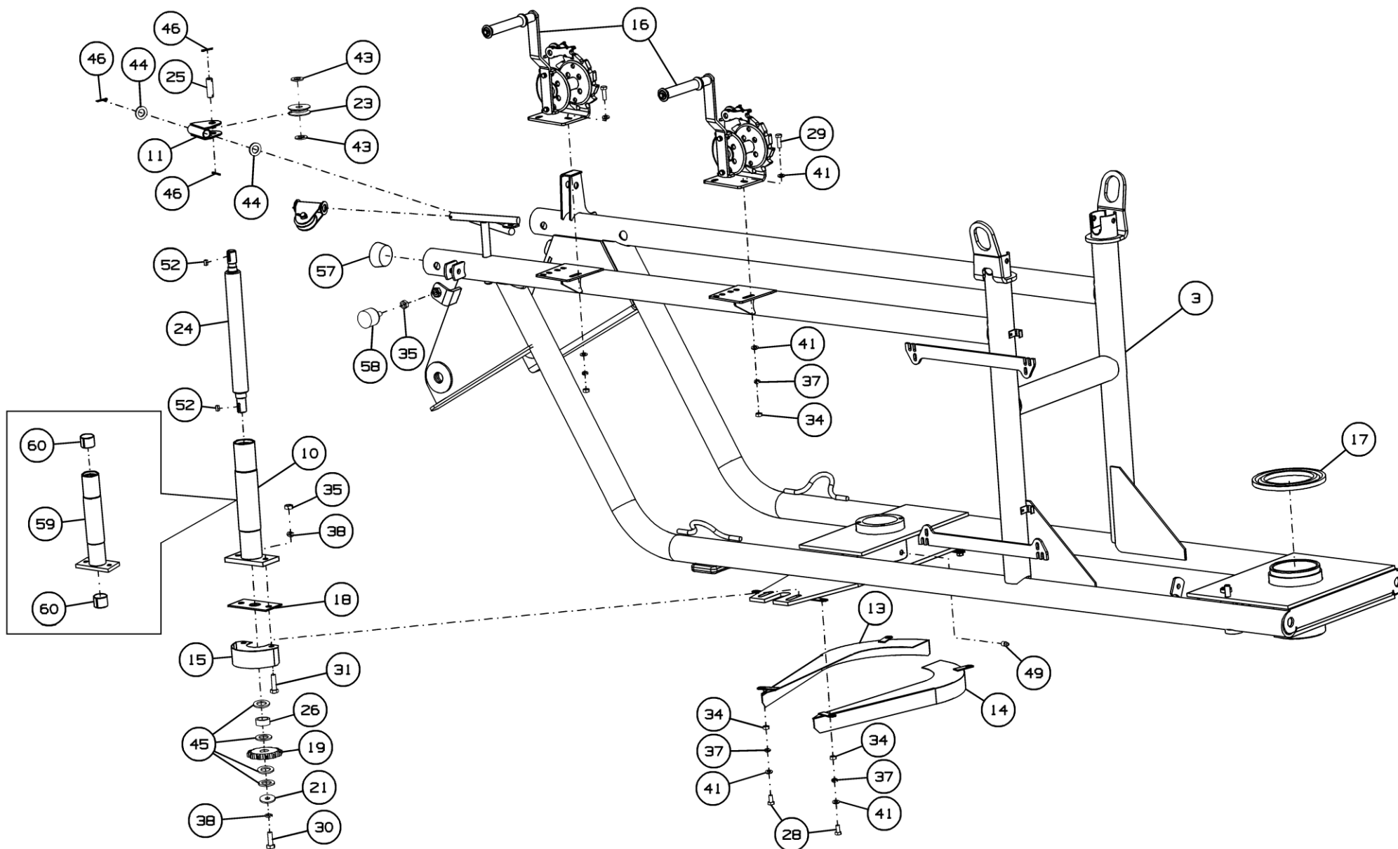
Рисунок 3 - Рама МЗС-150.01.000
