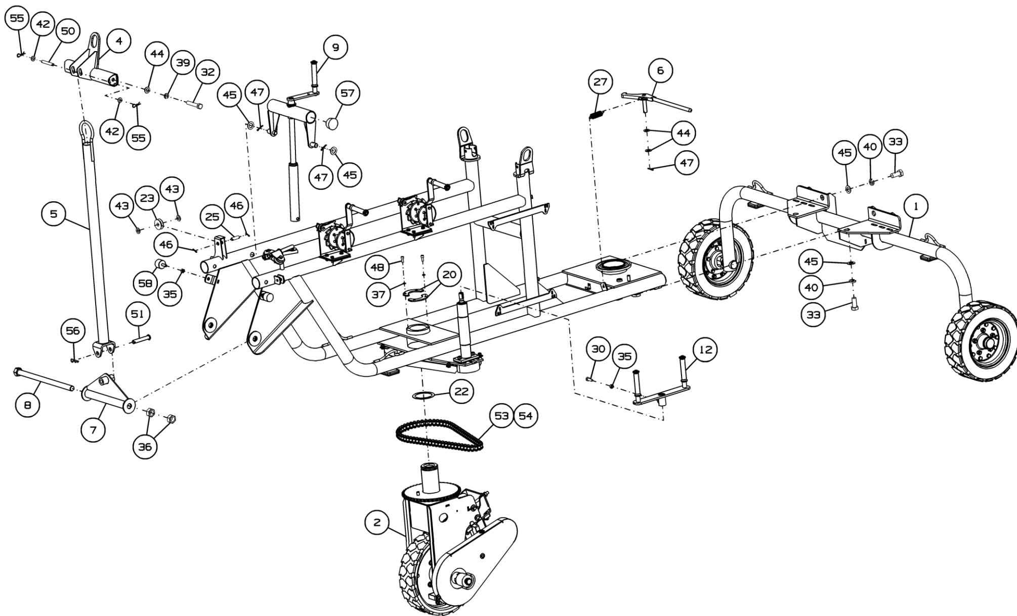
Рисунок 2 - Рама МЗС-150.01.000
