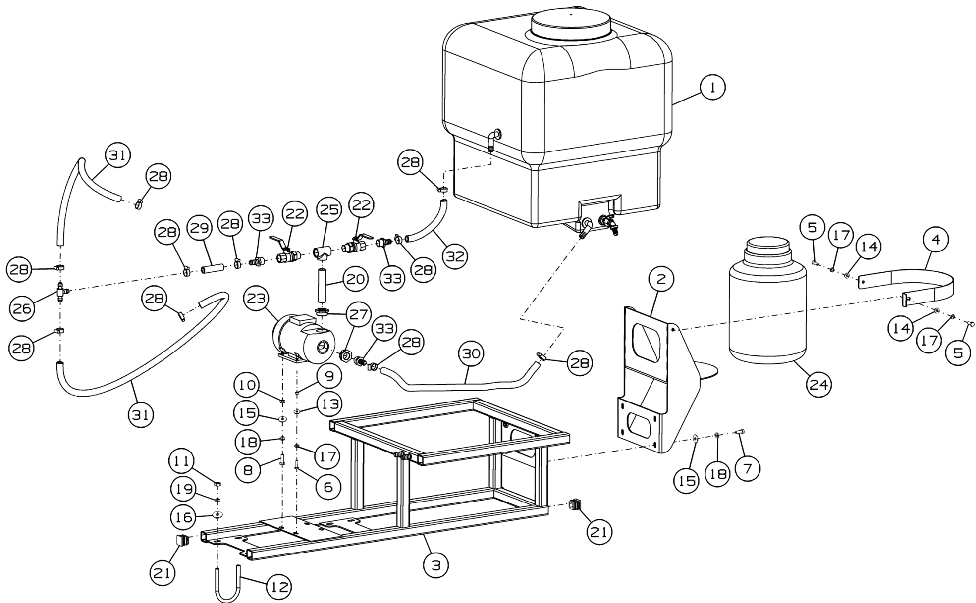
Рисунок 38 - Сборка насосной установки МЗС-150.08.200
