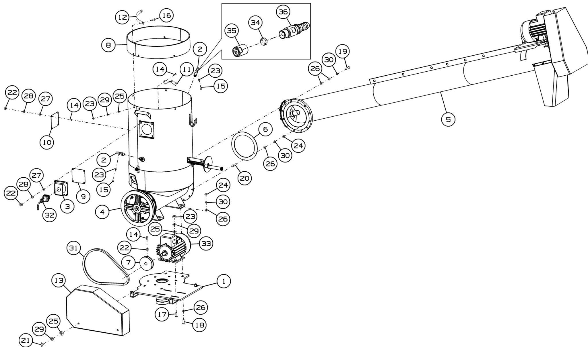
Рисунок 31 - Приставка протравливающая МЗС-150.08.100
