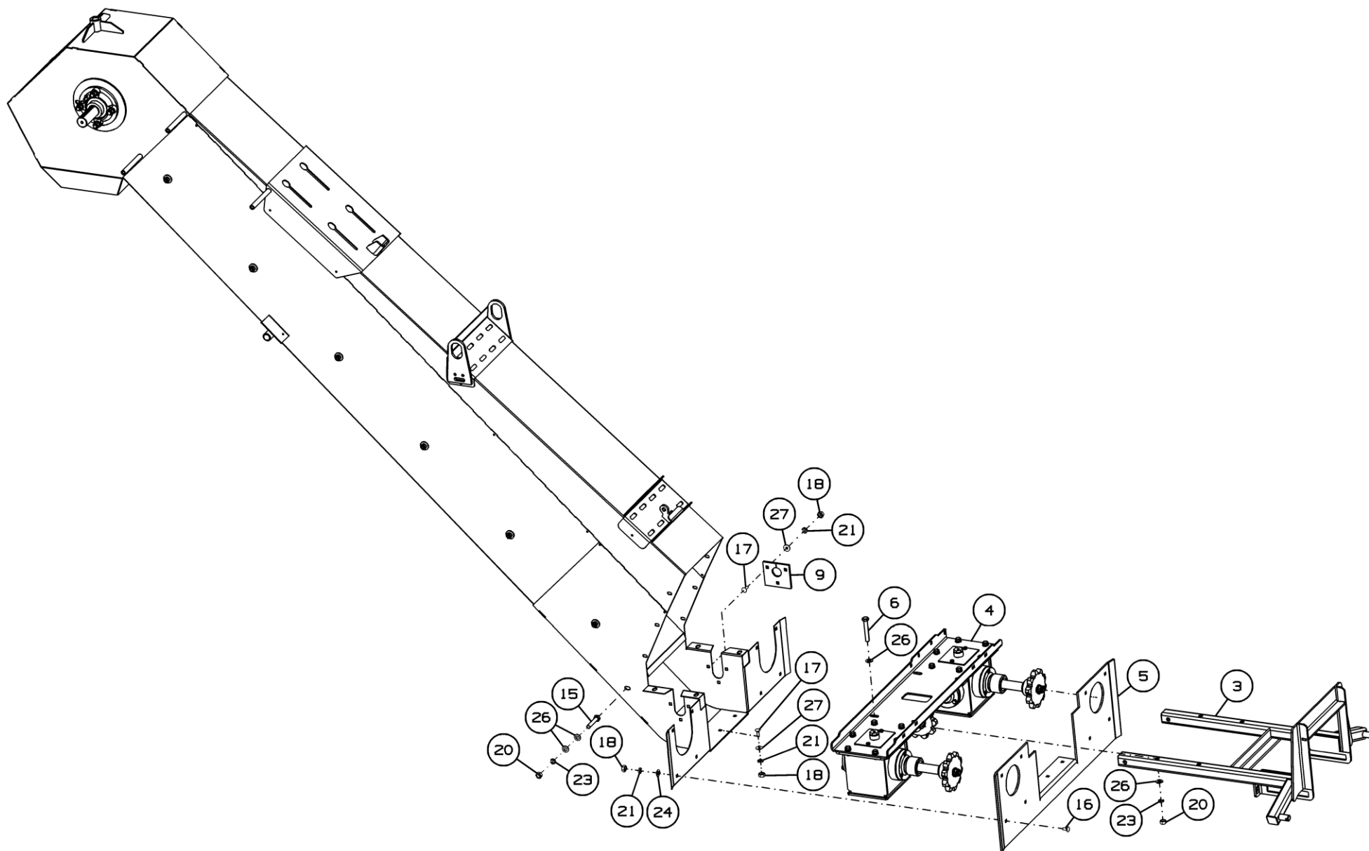
Рисунок 19 - Короб в сборе МЗС-150.03.020
