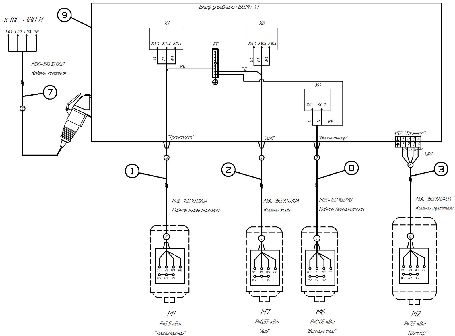
Рисунок 40 - Пульт управления МЗС-150.10.000А (Схема электрическая подключений)
