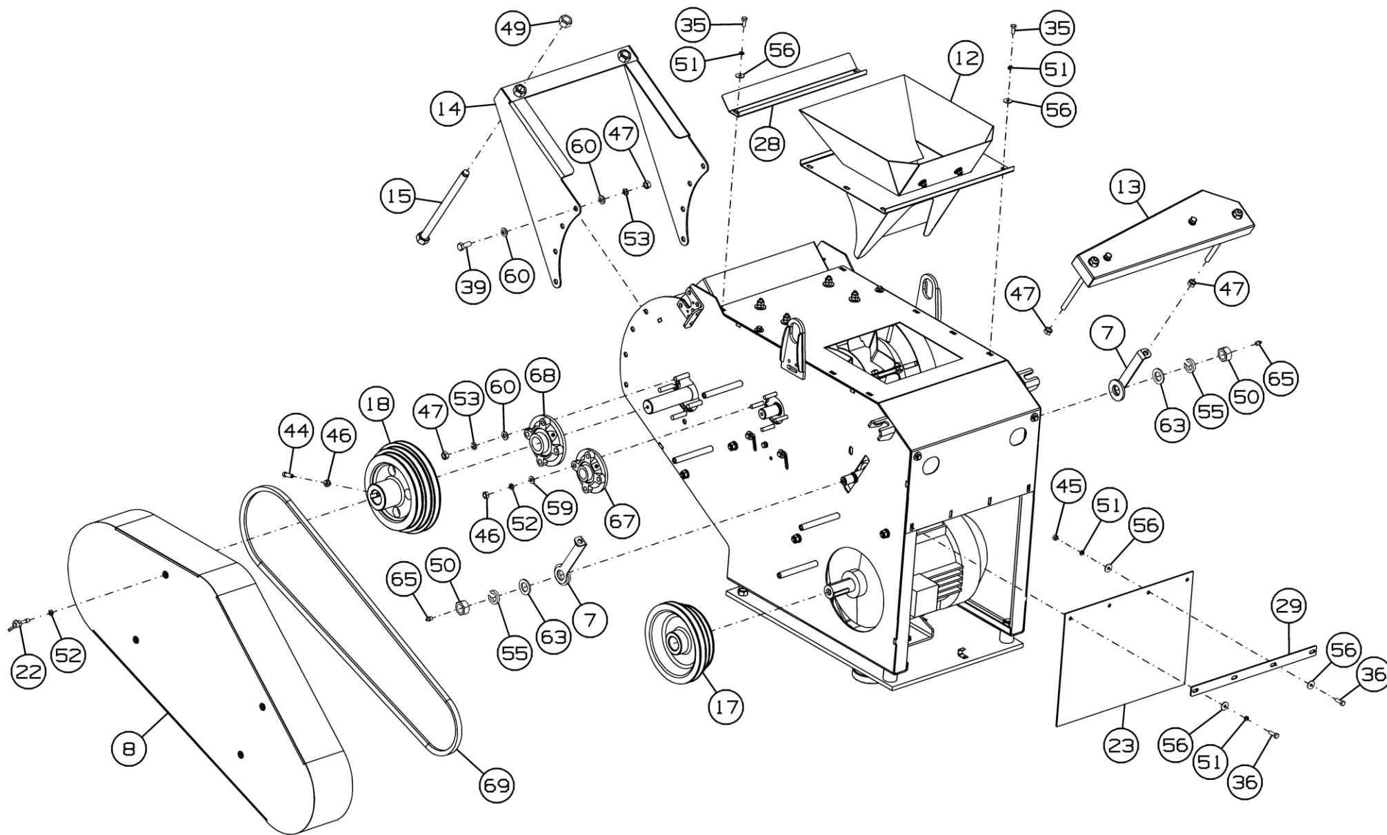
Рисунок 12 - Триммер МЗС-150.02.000
