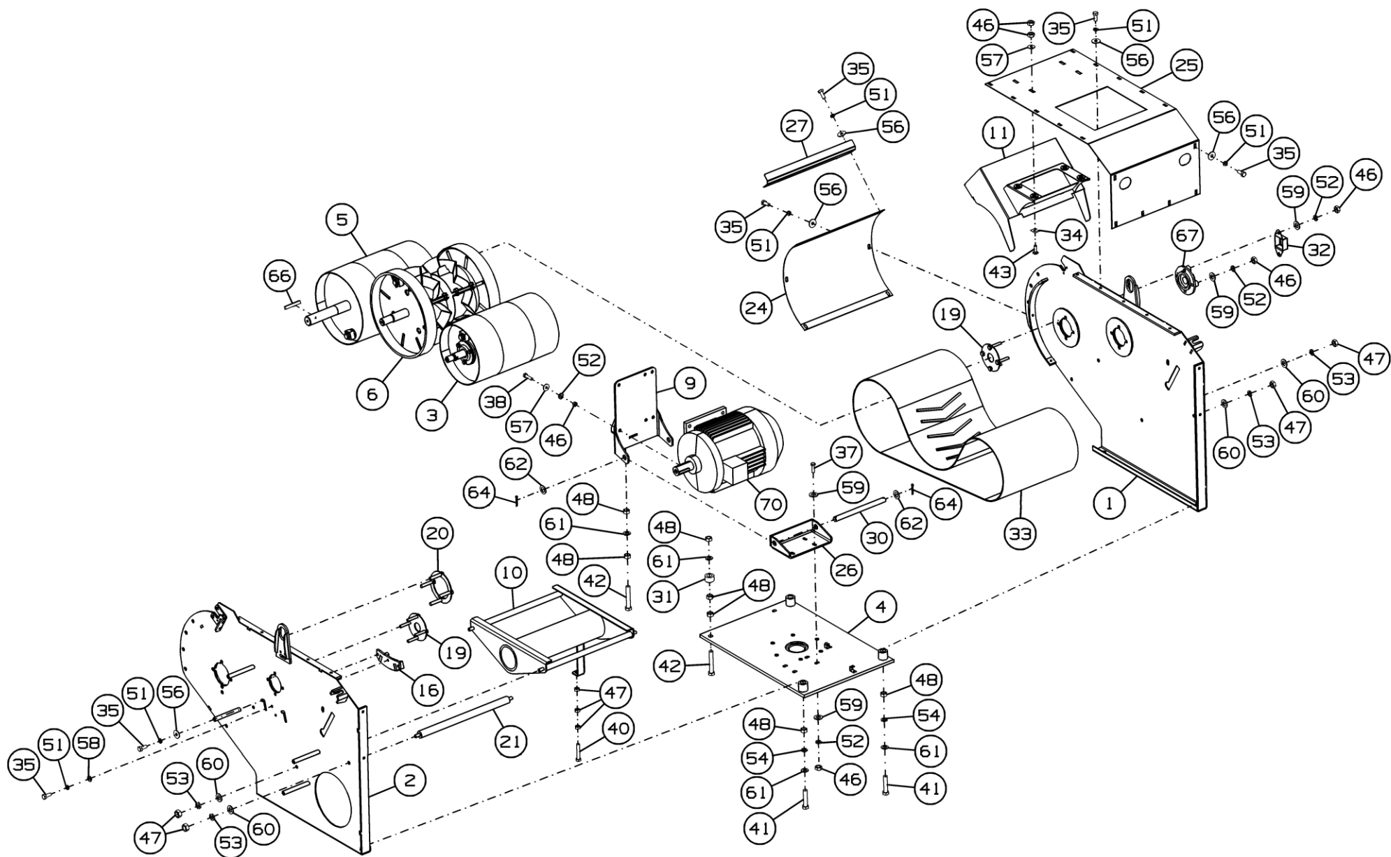
Рисунок 13 - Триммер МЗС-150.02.000
