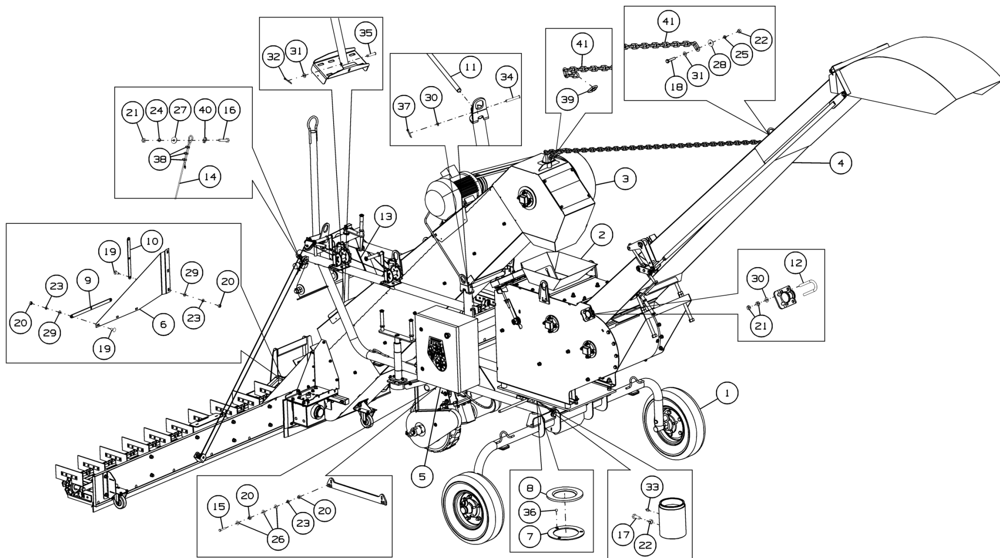
Рисунок 1 - Метатель зерна самопередвижной МЗС-150.00.000А и МЗС-150.00.000А-02
