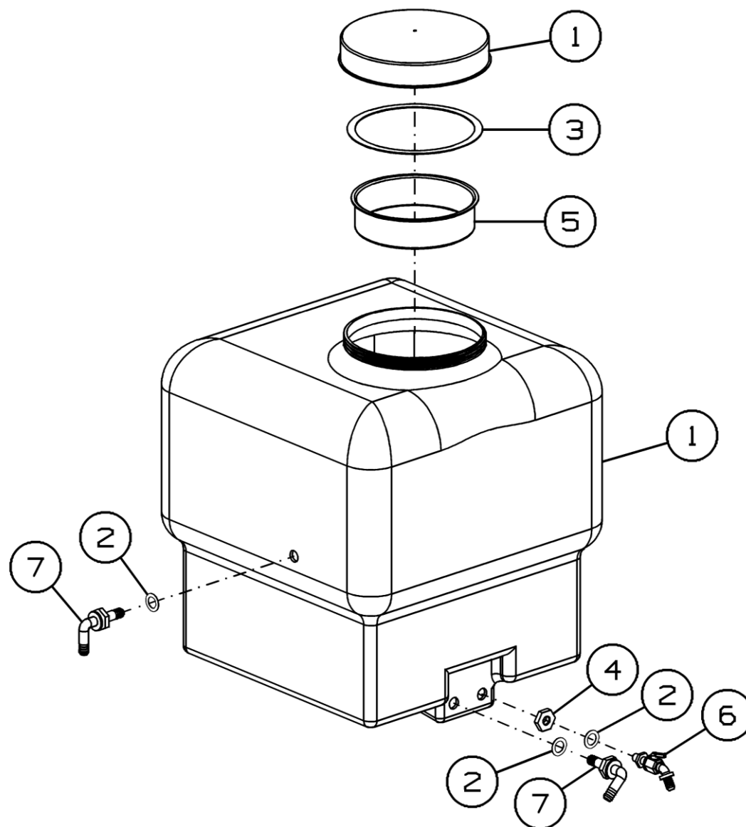
Рисунок 39 - Бак в сборе МЗС-150.08.210
