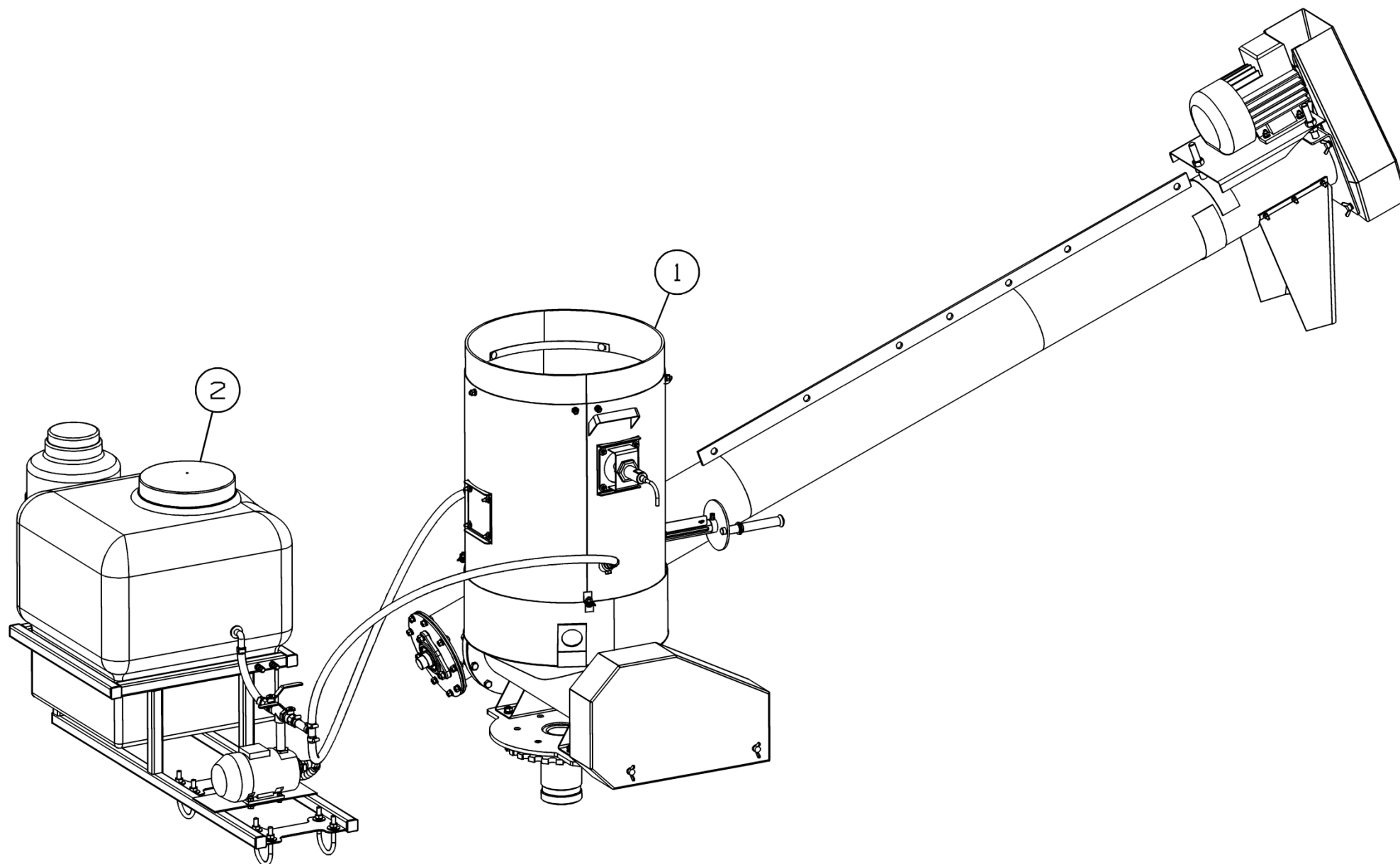
Рисунок 30 - Установка протравливающей приставки МЗС-150.08.000
