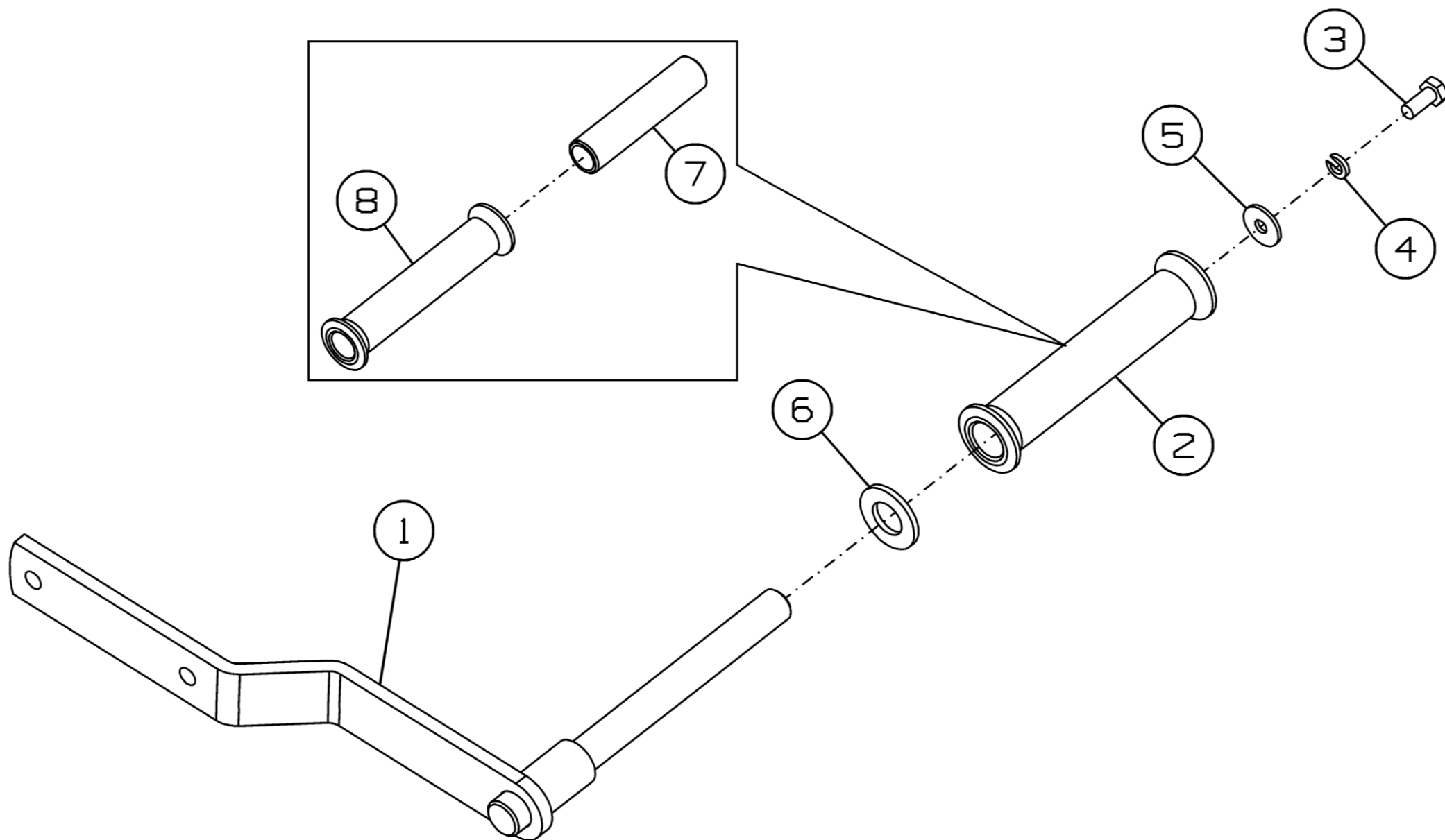
Рисунок 11 - Рукоятка МЗС-90.01.690А
