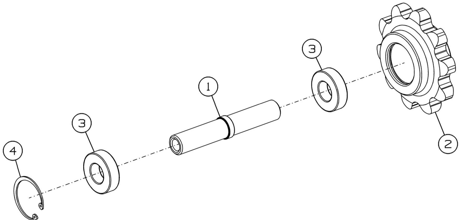
Рисунок 23 - Ось натяжная со звездочкой МЗС-150.03.230
