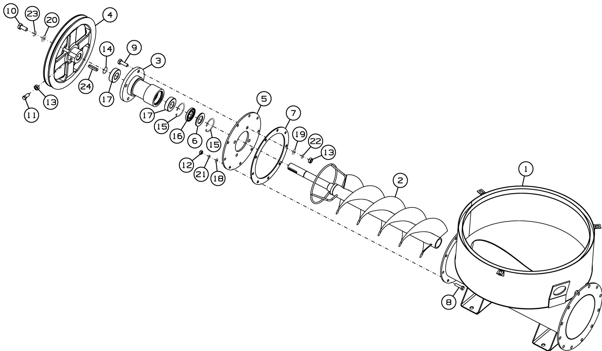
Рисунок 35 - Камера нижняя в сборе ПСМ-25.08.890
