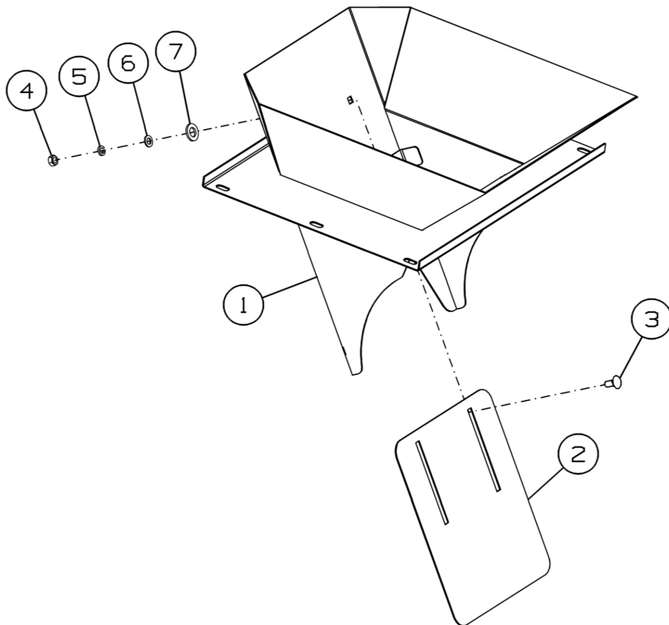
Рисунок 16 - Горловина засыпная МЗС-150.02.380
