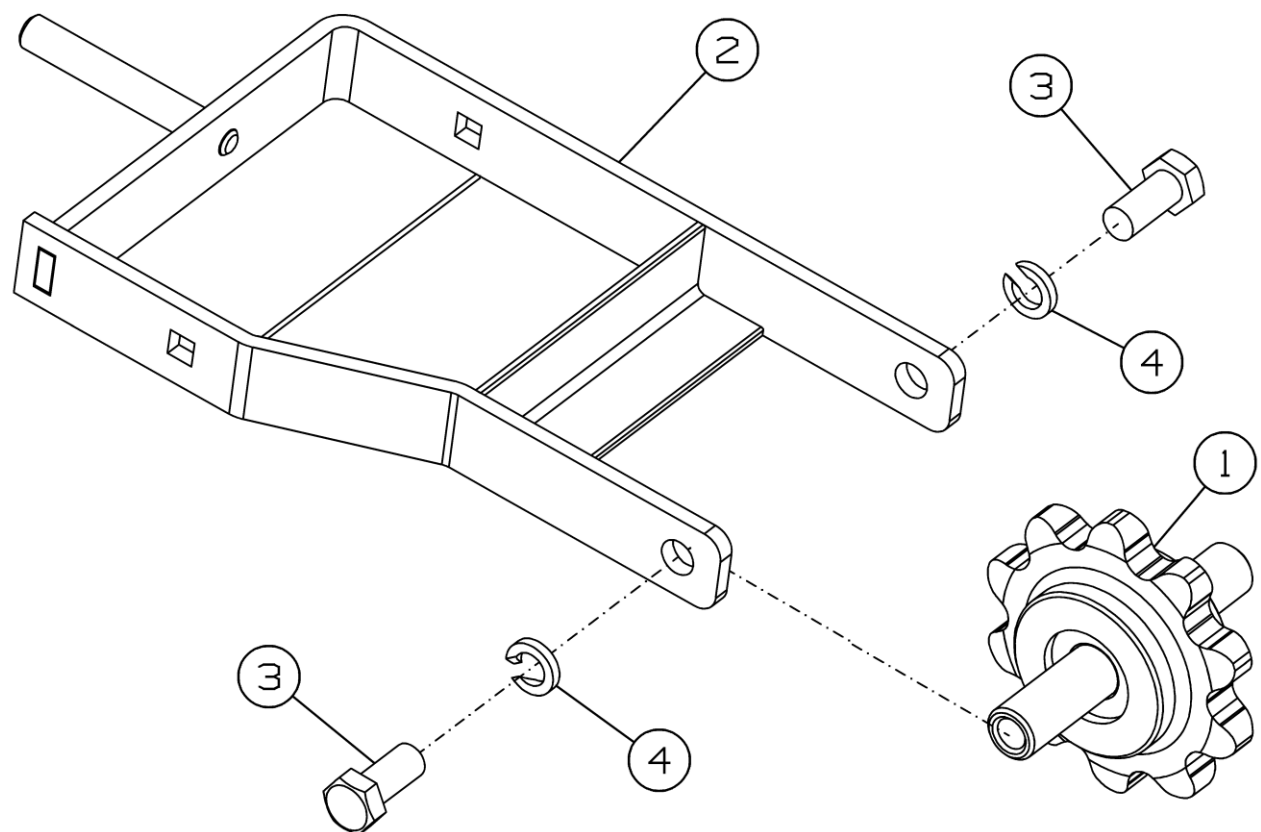
Рисунок 22 - Устройство натяжное МЗС-150.03.210
