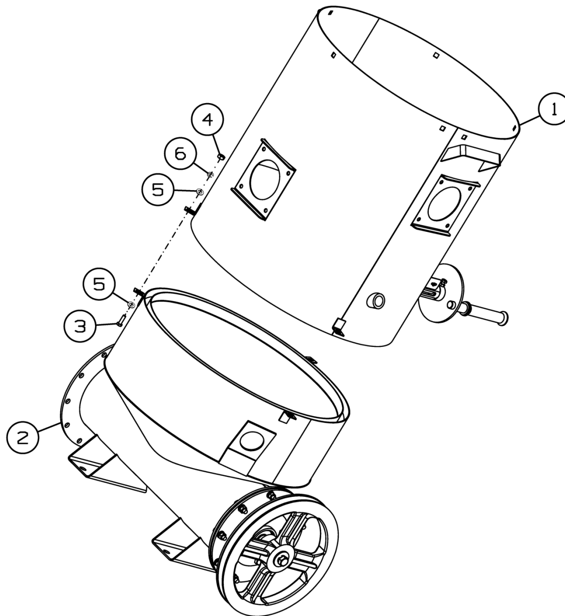
Рисунок 32 - Бункер в сборе ПСМ-25.08.840
