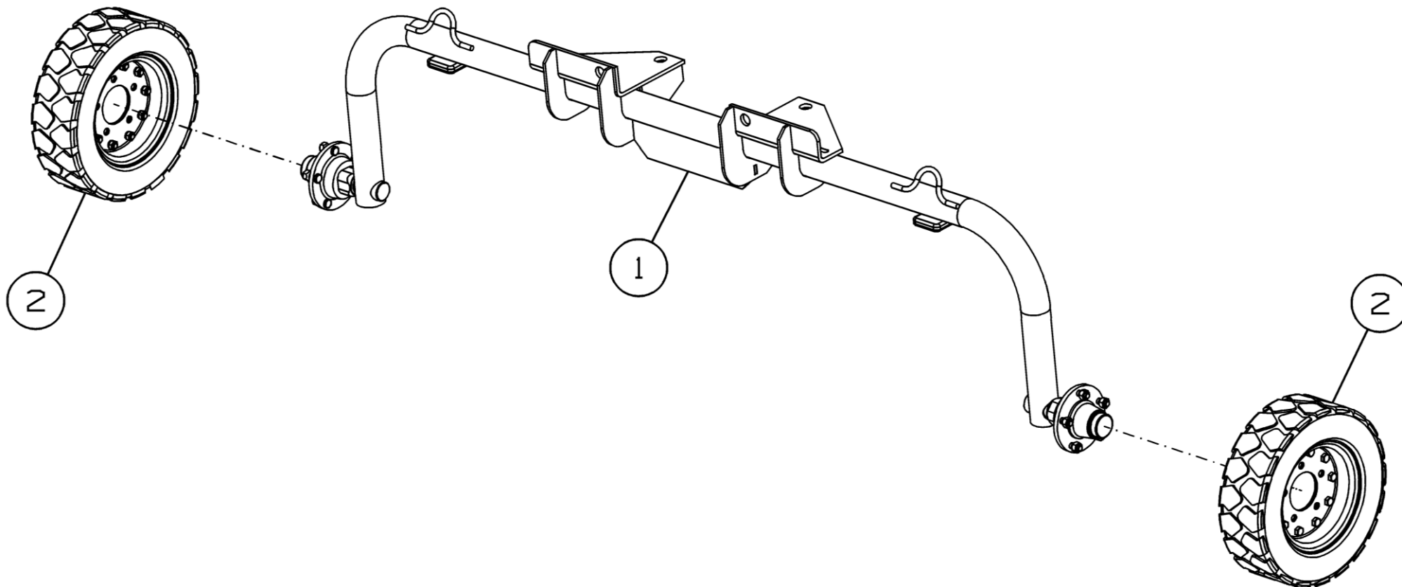
Рисунок 4 - Балка задняя в сборе МЗС-150.01.030
