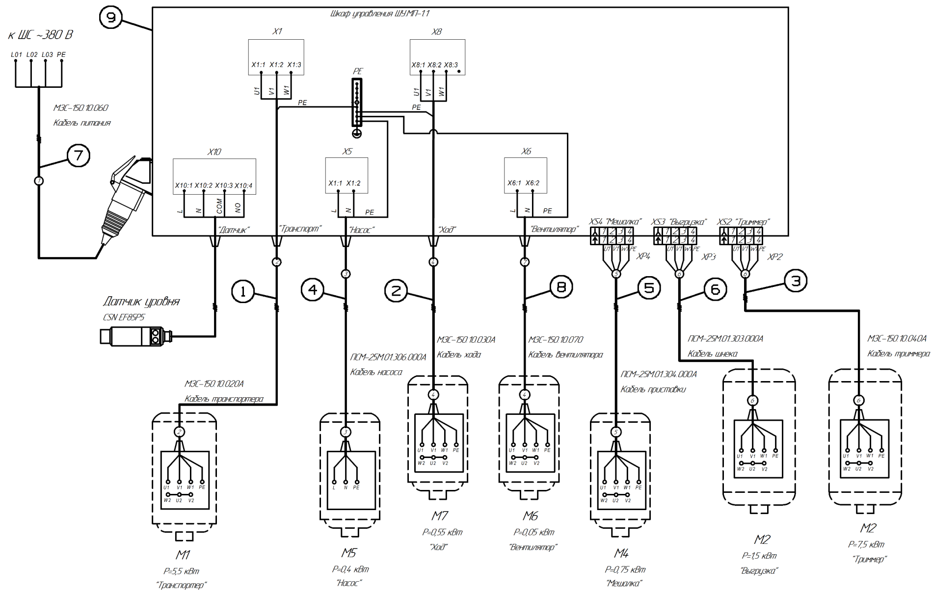
Рисунок 41 - Пулт управления МЗС-150.10.000А-01 (Схема электрическая подключений)
