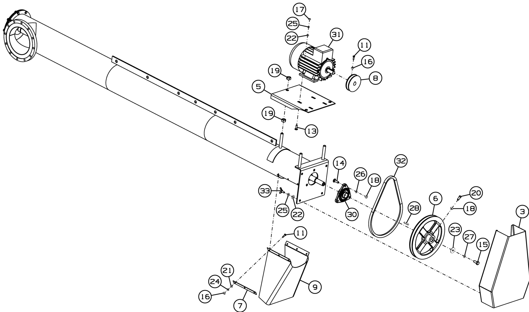
Рисунок 36 - Устройство выгрузное ПСМ-25.08.910
