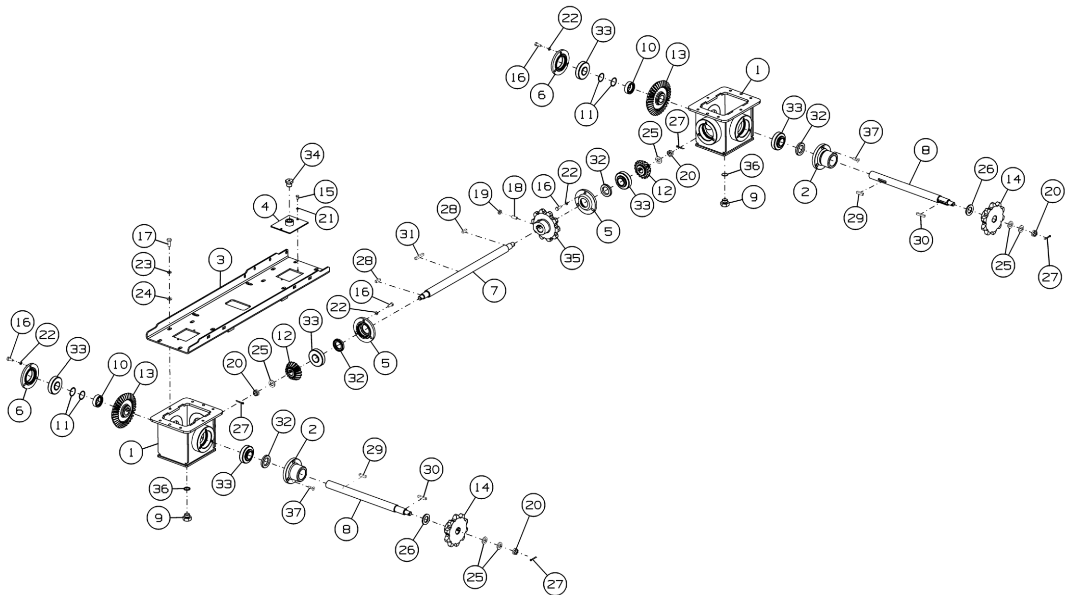
Рисунок 21 - Крышка со сварными редукторами МЗС-150.03.160А
