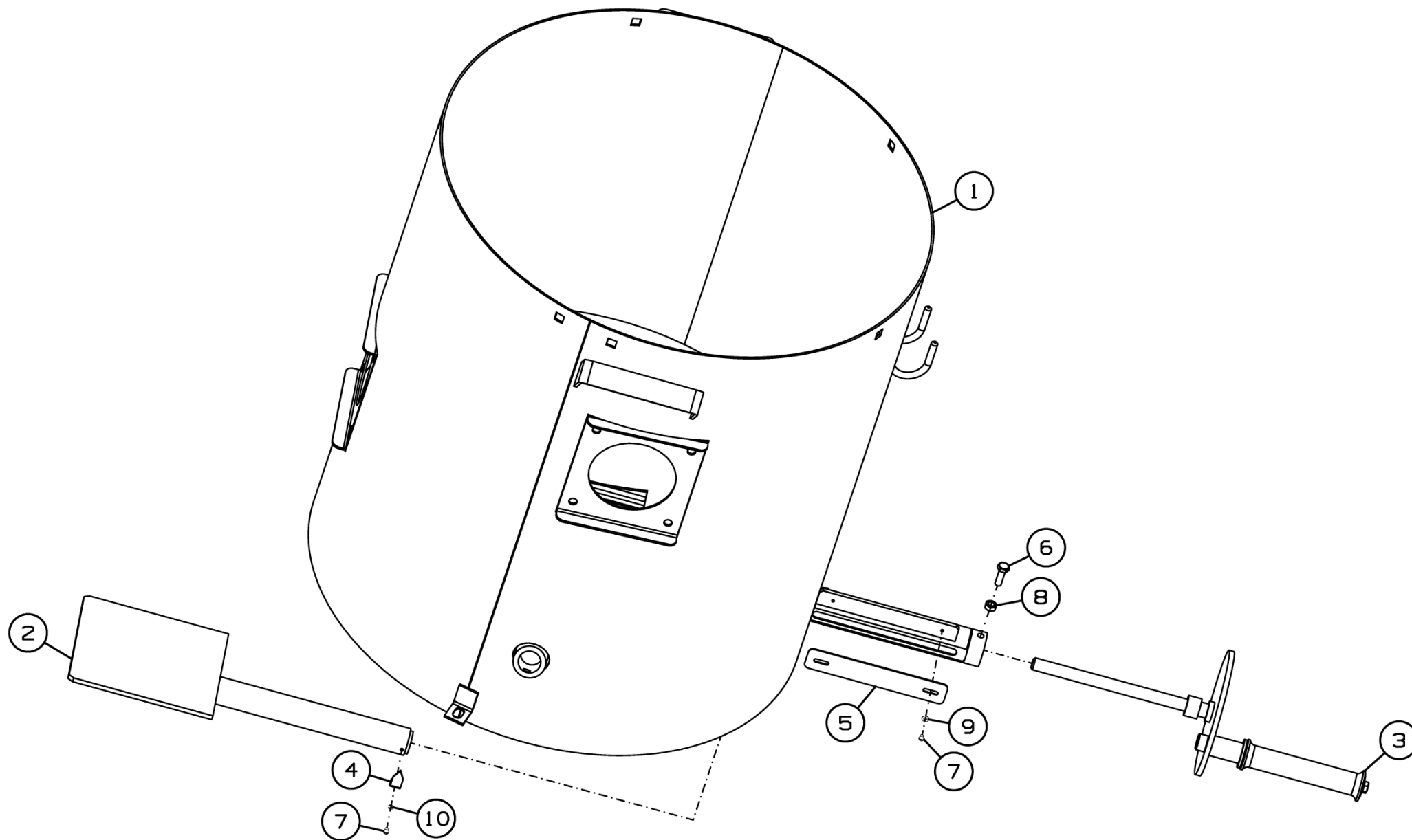
Рисунок 33 - Бункер семян в сборе ПСМ-25.08.850
