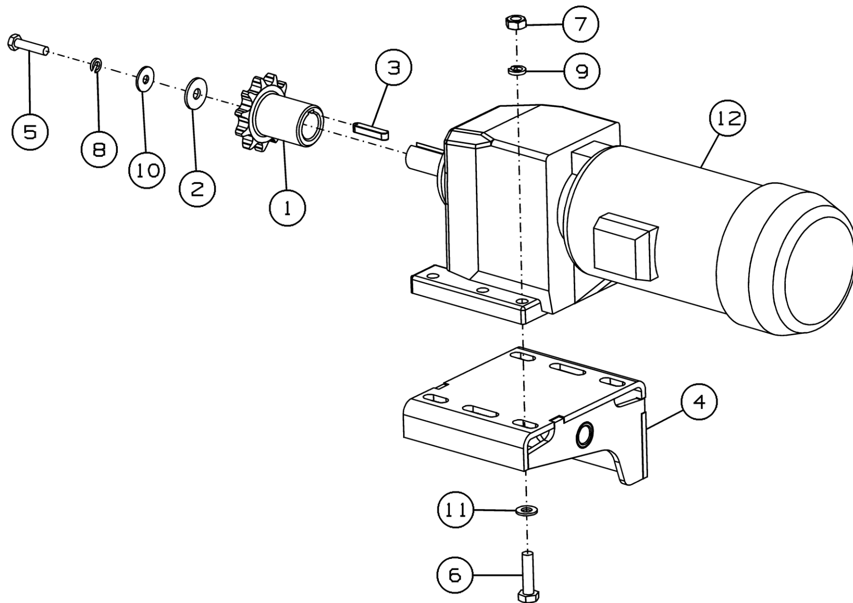
Рисунок 6 - Установка мотор-редуктора МЗС-150.01.260
