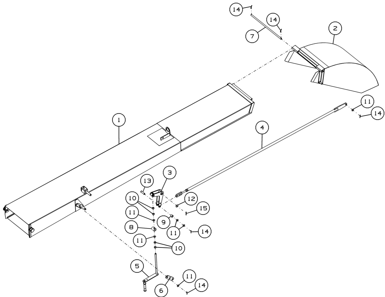
Рисунок 27 - Желоб выгрузной МЗС-150.04.000
