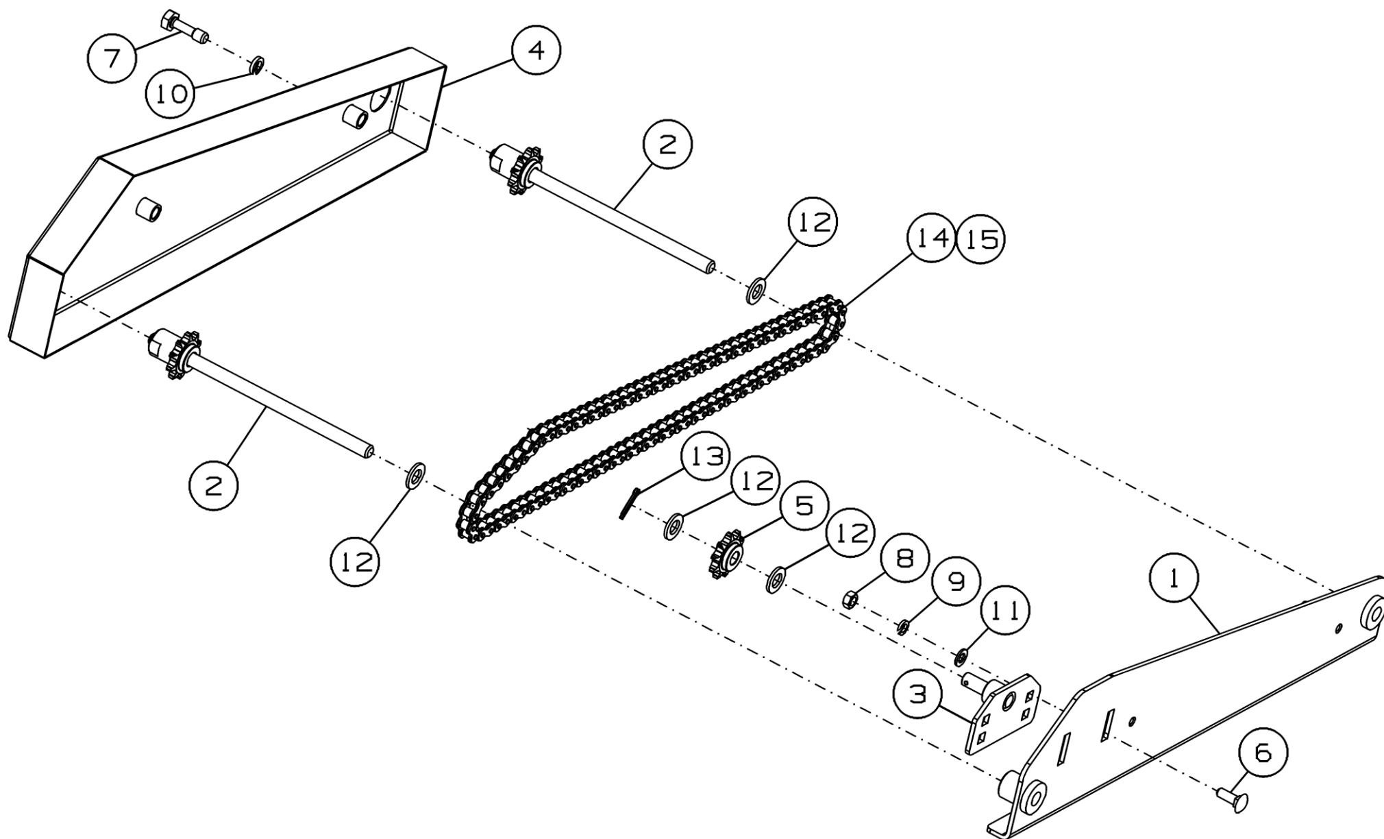
Рисунок 17 - Механизм натяжной МЗС-150.02.400
