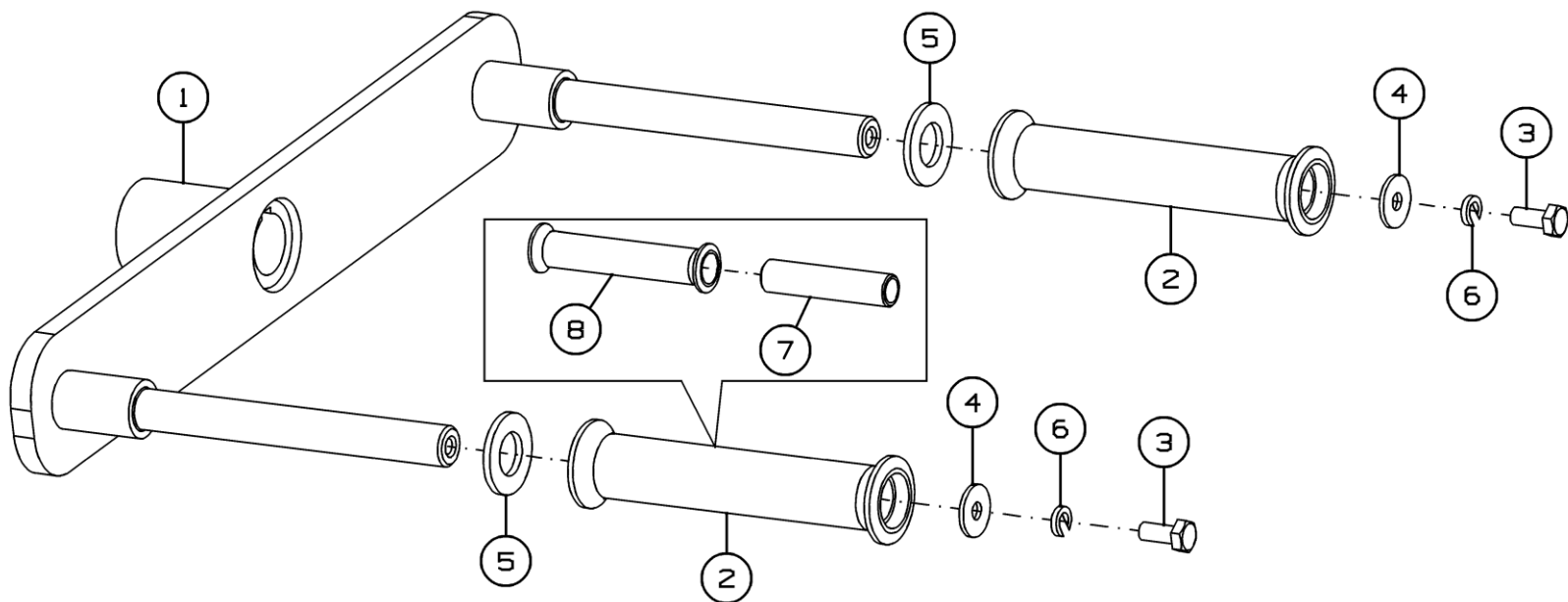
Рисунок 9 - Руль МЗС-150.01.530
