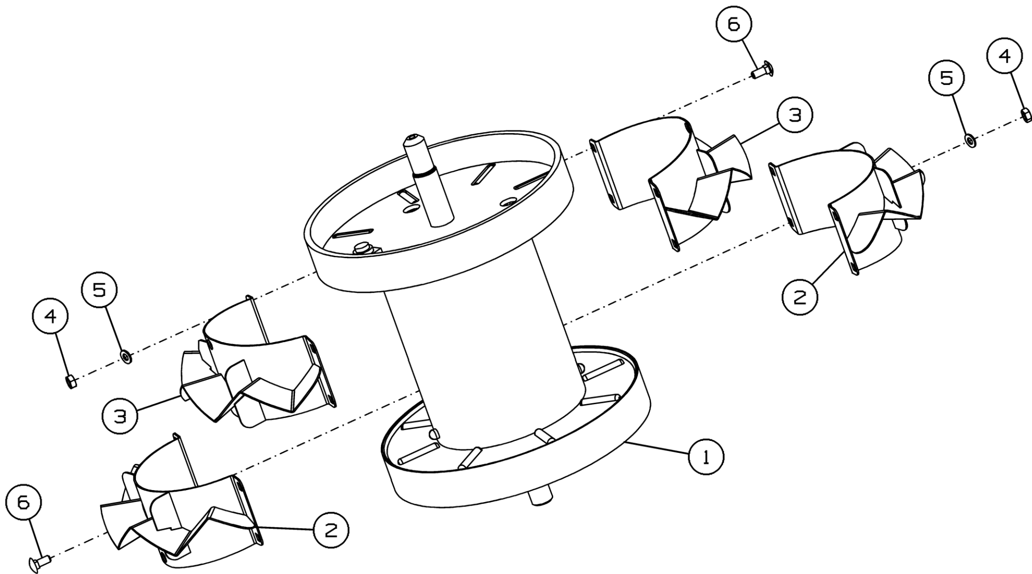
Рисунок 15 - Барабан-катушка МЗС-150.02.120-03
