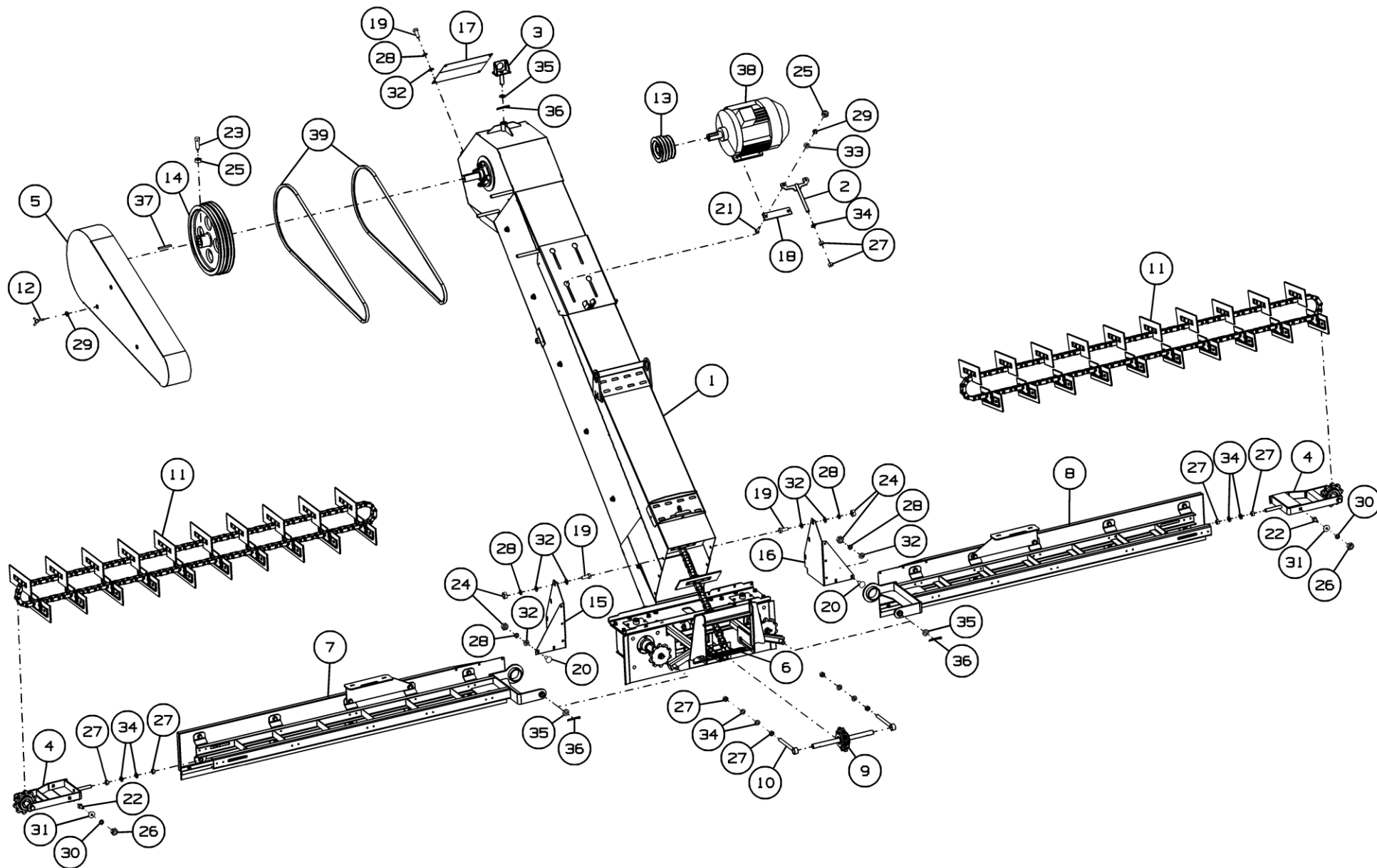
Рисунок 18 - Транспортер загрузочный МЗС-150.03.000
