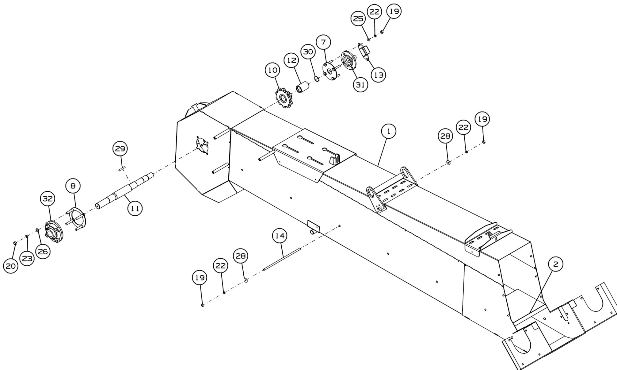
Рисунок 20 - Короб в сборе МЗС-150.03.020
