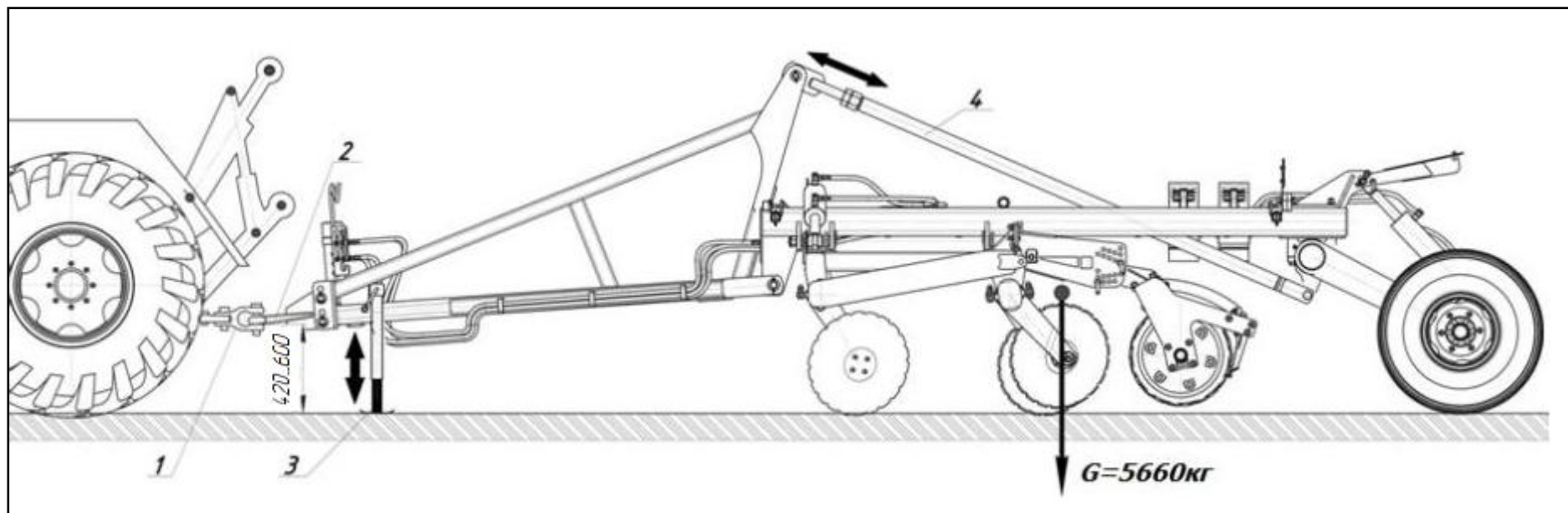
Рисунок Б.1 – Схема агрегатирования мульчировщика HD-800/600 при краткосрочном и длительном хранении
