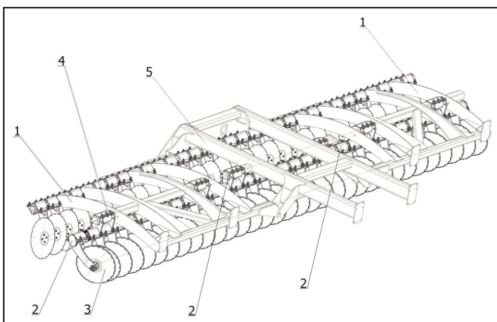
1 – крыло; 2 – брус; 3 – рабочий орган; 4 – хомут; 5 – рама Рисунок 3.10 – Брус рабочих органов мульчировщика HD-800/800
