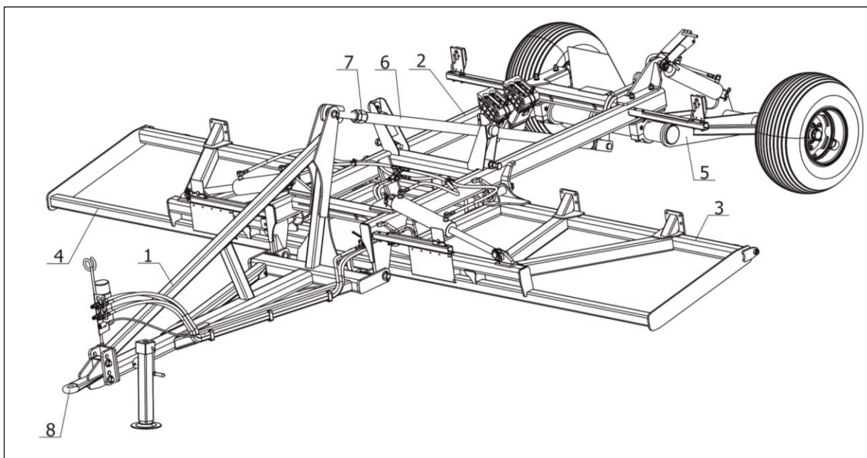
1 – сница; 2 – рама; 3 – крыло левое; 4 – крыло правое; 5 – рама шасси; 6 – тяга; 7 – контргайка; 8 – прицеп
