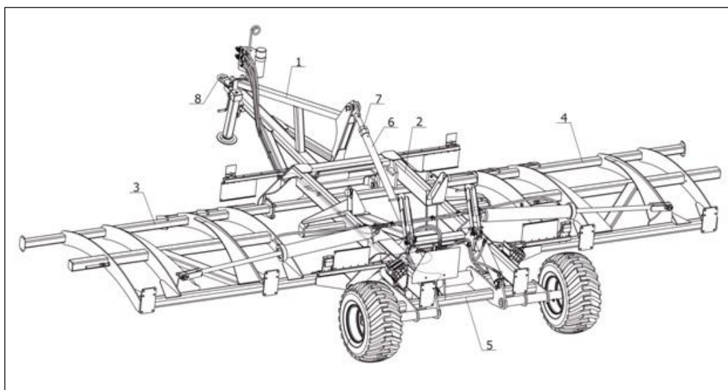
1 – сница; 2 – рама; 3 – крыло левое; 4 – крыло правое; 5 – рама шасси; 6 – тяга; 7 – контргайка; 8 – прицеп
