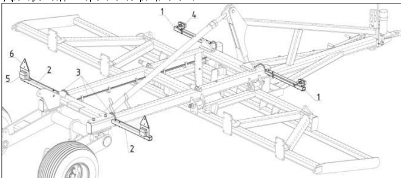
Рисунок 3.15 – Электрооборудование мульчировщика HD-800/600,
