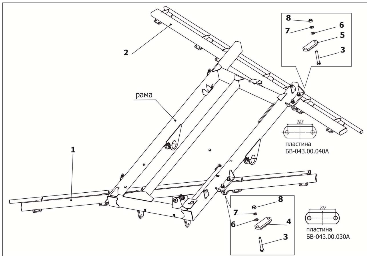
1 – брус передний (L=6742 мм); 2 – брус задний (L=7112 мм); 3 – болт; 4 – пластина (БВ-430.00.030А); 5 – пластина (БВ-430.00.040А); 6 – шайба; 7 – шайба; 8 – гайка
