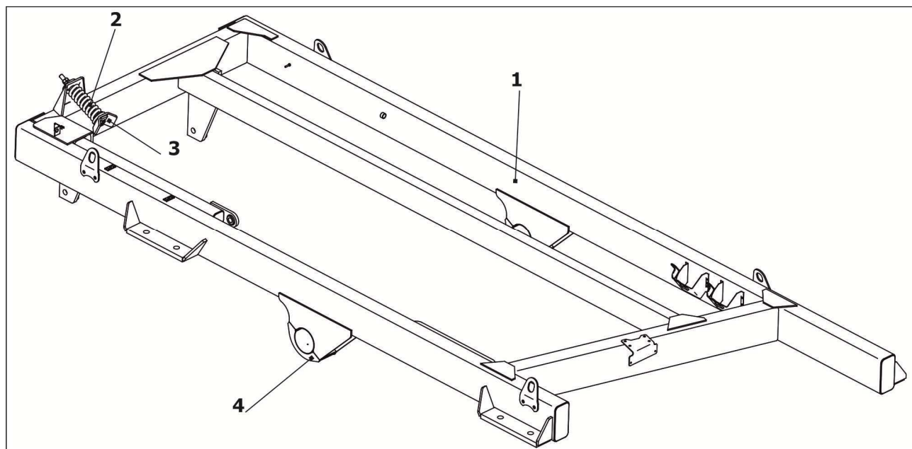
1 – рама; 2 – пружина; 3 – упор; 4 - обойма
