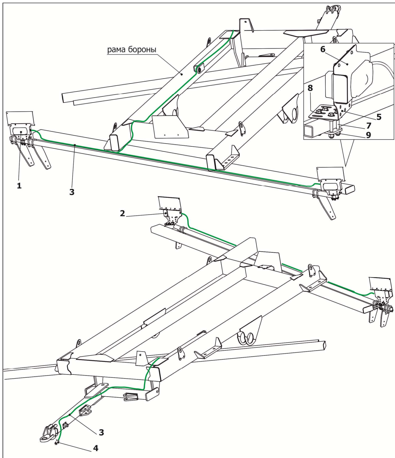
1 – фонарь задний; 2 – фонарь передний; 3 – жгут электропроводки; 4 – вилка; 5, 6 – кронштейн фонарей Рисунок 3.10 – Коммуникации электрические
