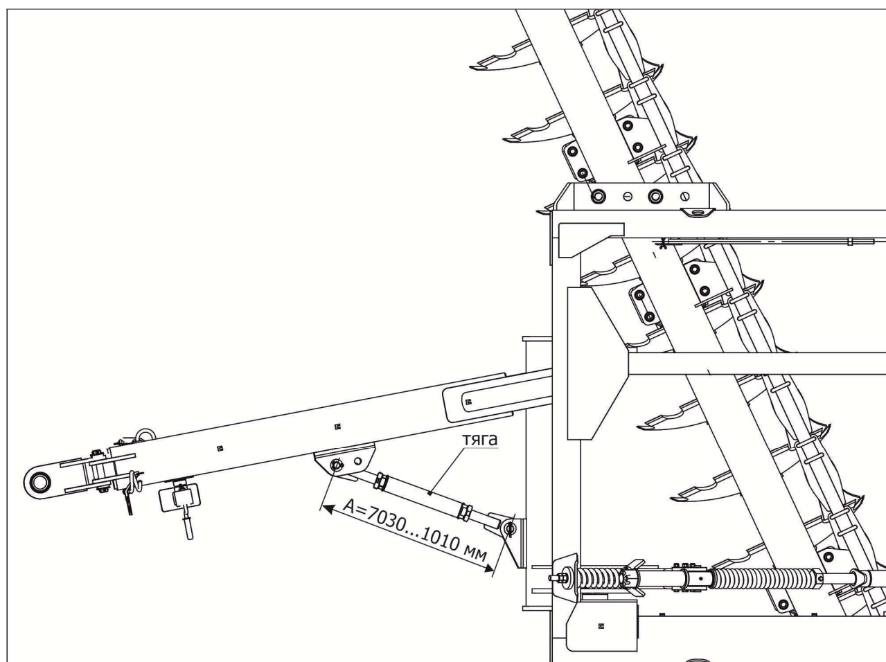
Рисунок 6.4 – Регулировка сннца бороны
