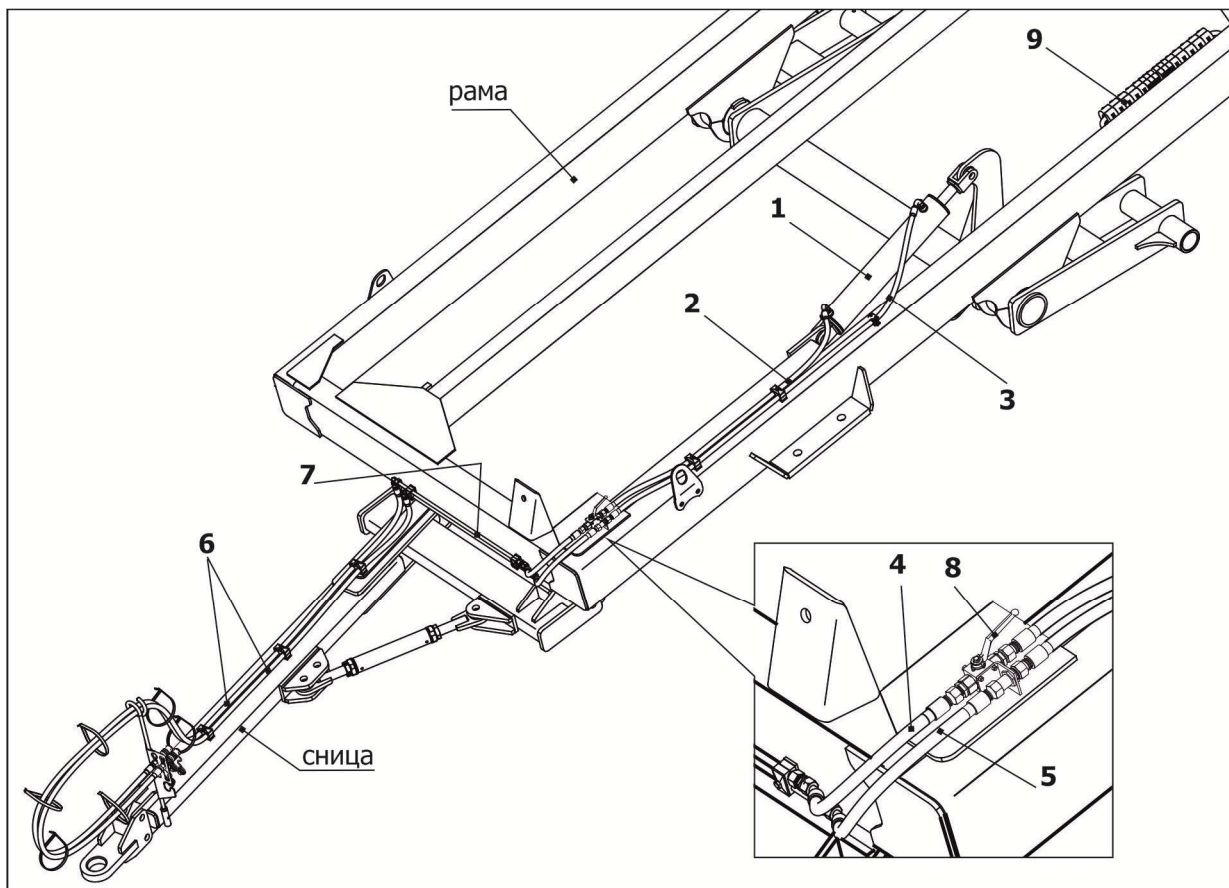
1 – гидроцилиндр; 2, 3, 4, 5, 6 – РВД; 7 – трубопровод; 8 – кран; 9 – набор стоп-сегментов Рисунок 3.9– Гидрооборудование
