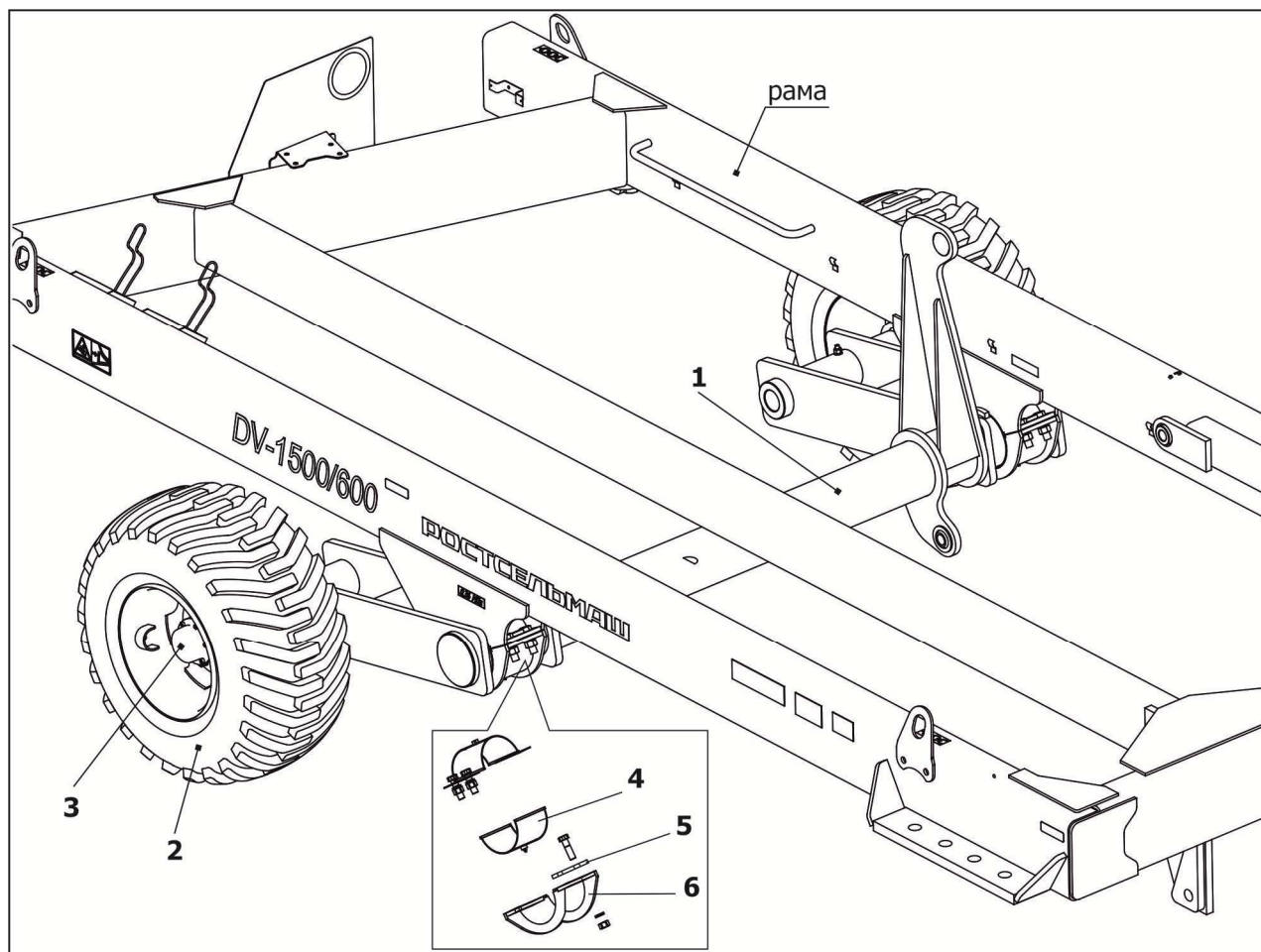
1 - балка шасси; 2 - колесо в сборе; 3 – ступица; 4 – вкладыш; 5 – прокладка; 6 - обойма Рисунок 3.4 – Шасси
