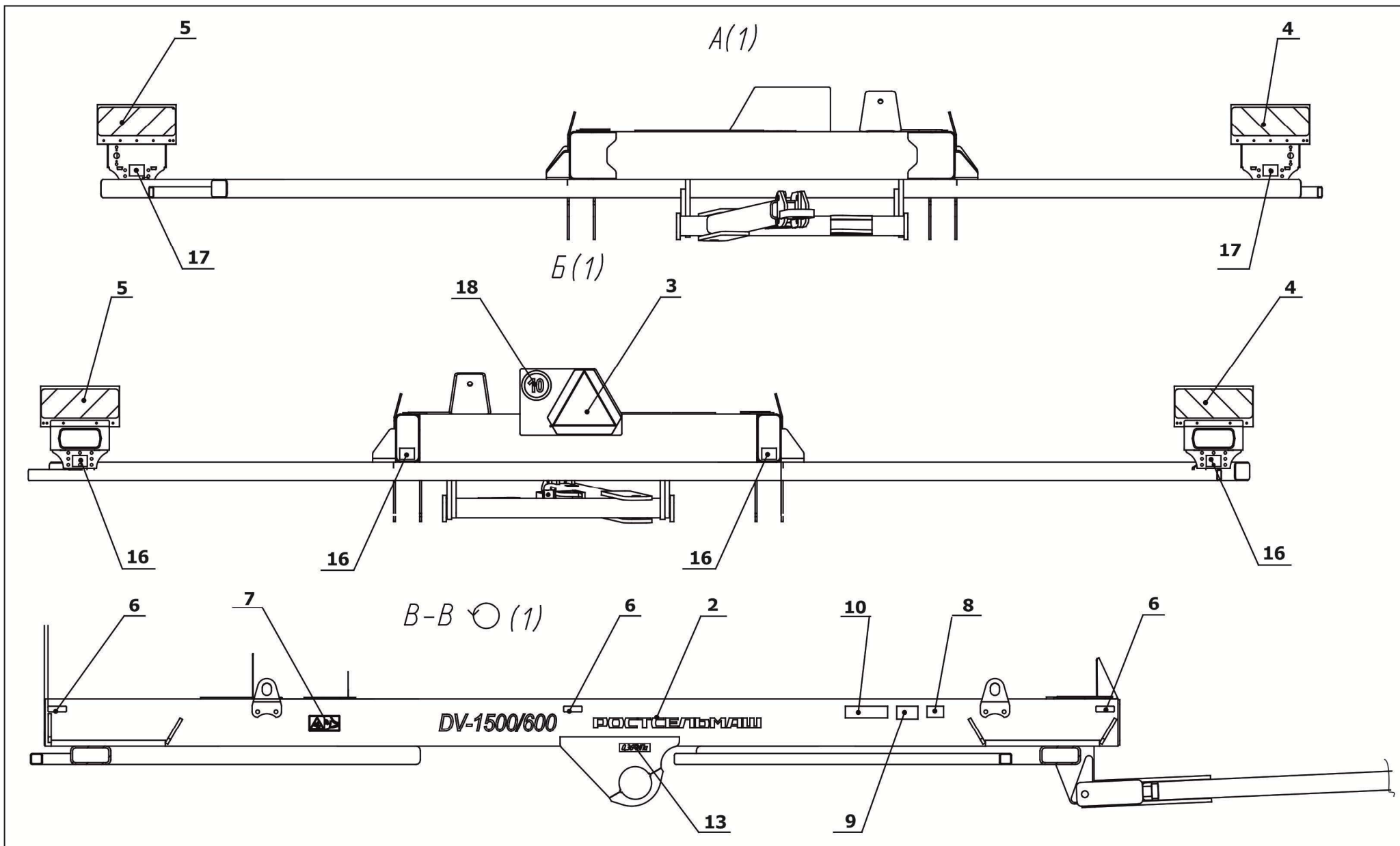
Рисунок 4.2 – Месторасположение табличек и аппликаций на бороне
