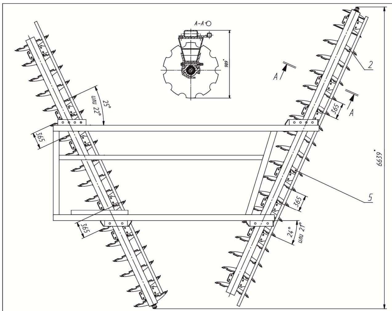
Рисунок 6.3 – Углы установки дисковых батарей. Схема
