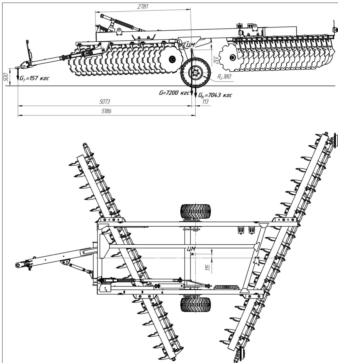
Рисунок В.1 – Схема расположения центра масс борона при транспортировании
