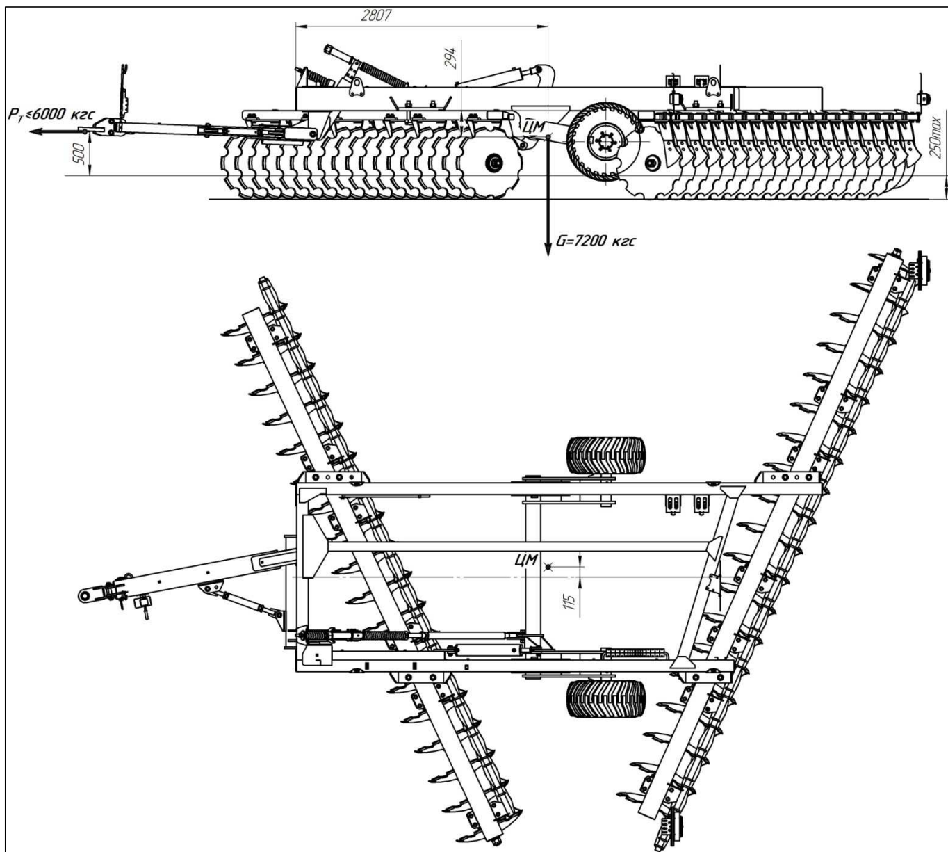
Рисунок В.2 – Схема расположения центра масс бороны при работе
