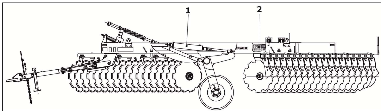
1 - стоп-сигменты; 2 - гидроцилиндр Рисунок 5.2 – Транспортное положение бороны
