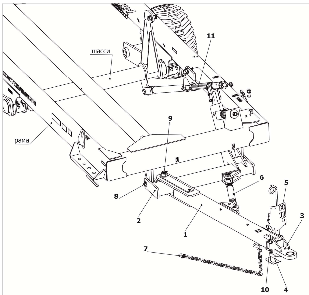
1 – сница; 2 – перемычка; 3 – прицеп; 4 – домкрат; 5 – держатель РВД; 6 – тяга; 7 – цепь страховочная; 8 – ось крепления сницы к раме; 9 – палец; 10 – ось крепления прицепа; 11 – регулятор горизонта
