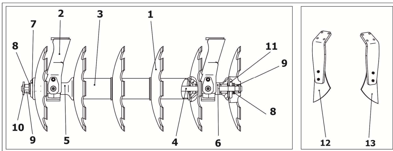
1 – диск; 2 – стойка; 3 – шпилька; 4 – ось; 5, 6 – проставка; 7 – прижим; 8, 11 – шайба; 9-гайка; 10 – штифт; 12, 13 – чистик
