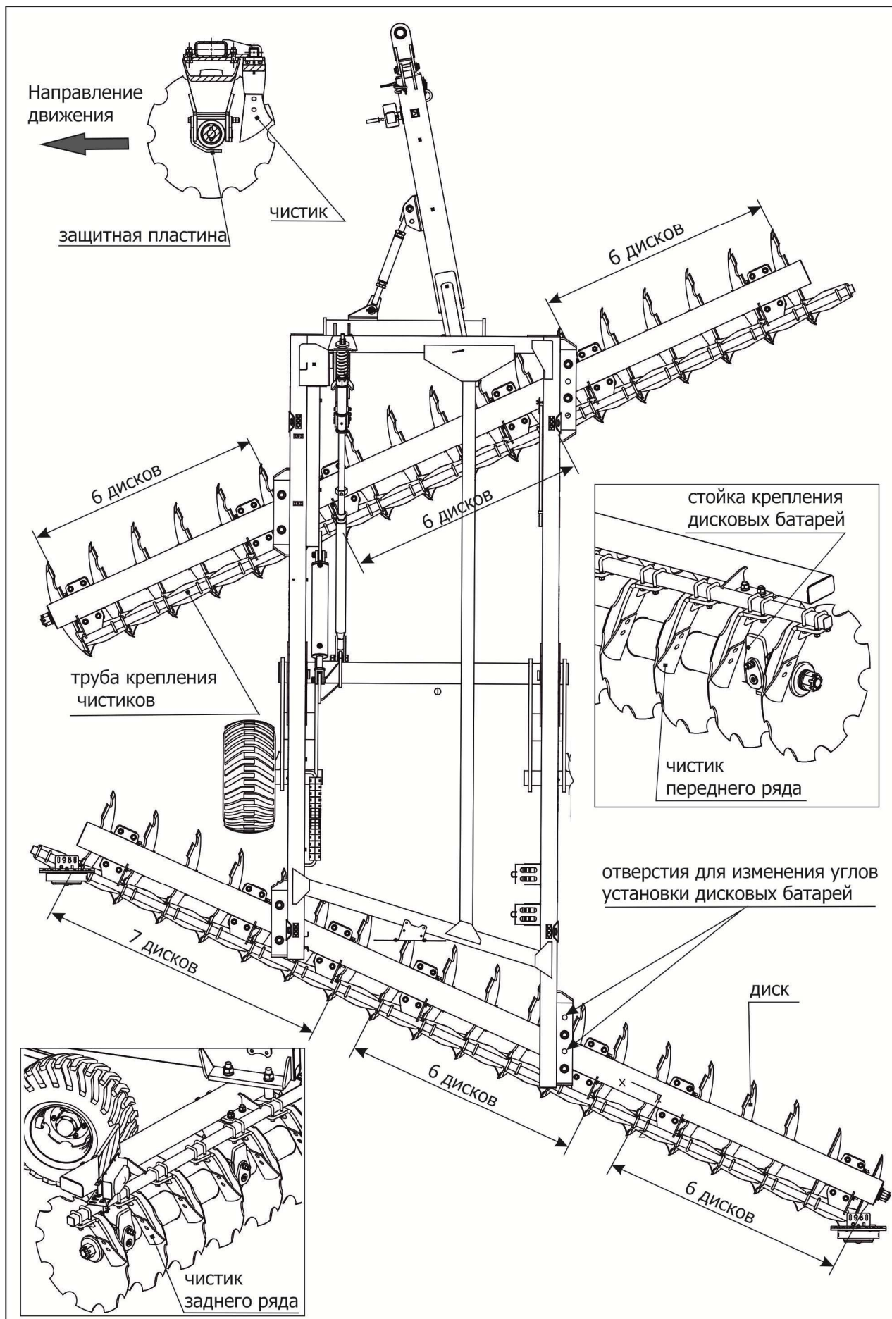
Рисунок 3.7 – Расположение дисковых батарей, чистиков
