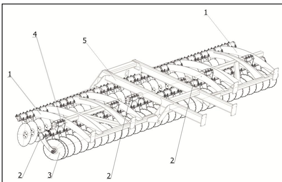
Рисунок 3.10 – Брус рабочих органов мульчировщика HD-800/800
