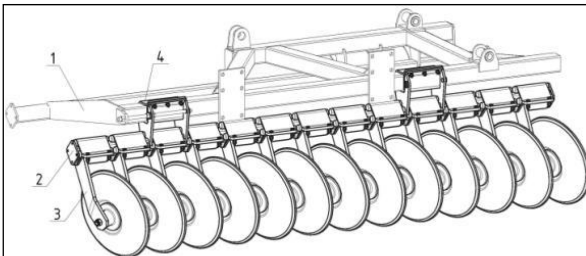
Рисунок 3.9 – Брус рабочих органов мульчировщика HD-800/600
