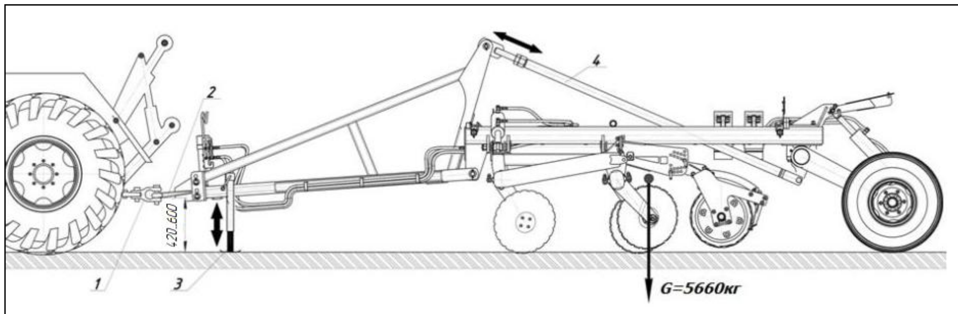
1 – прицепная серьга навески трактора; 2 – прицеп мульчировщика; 3 – домкрат; 4 – троса МД-800.24.000 Рисунок Б.1 – Схема агрегатирования мульчировщика HD-800/600 при краткосрочном и длительном хранении
