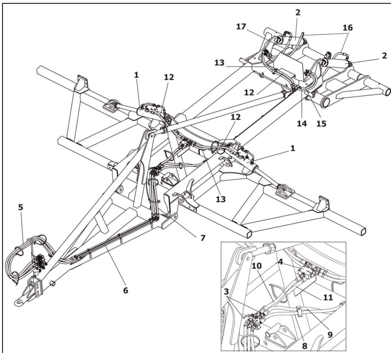
1 – гидроцилиндр подъема крыла; 2 – гидроцилиндр подъема шасси; 3 – кран шаровый; 4 – делитель потока; 5 - РВД.12.А2L.Б2L.2400.2SN ; 6 – трубопровод; 7 - РВД.12.А2L.А7L.800.2SN ; 8 - РВД.12.А2L.Б2L.1300.2SN ; 9 - РВД.12.А2L.Б2L.1320.2SN ; 10 - РВД.12.А2L.А2L.510.2SN ; 11- РВД.12.А2L.А2L.630.2SN ; 12 - РВД.12.А2L.А3L.820.2SN ТУ; 13 - РВД.12.А2L.А3L.740.2SN ; 14 - РВД.12.А2L.А3L.620.2SN ; 15 - РВД.12.А2L.А2L.510.2SN ; 16 - РВД.12.А2L.А3L.1000.2SN ; 17 - РВД.12.А2L.А3L.600.2SN Рисунок 3.13 – Гидравлическая система мульчировщика HD-800/600
