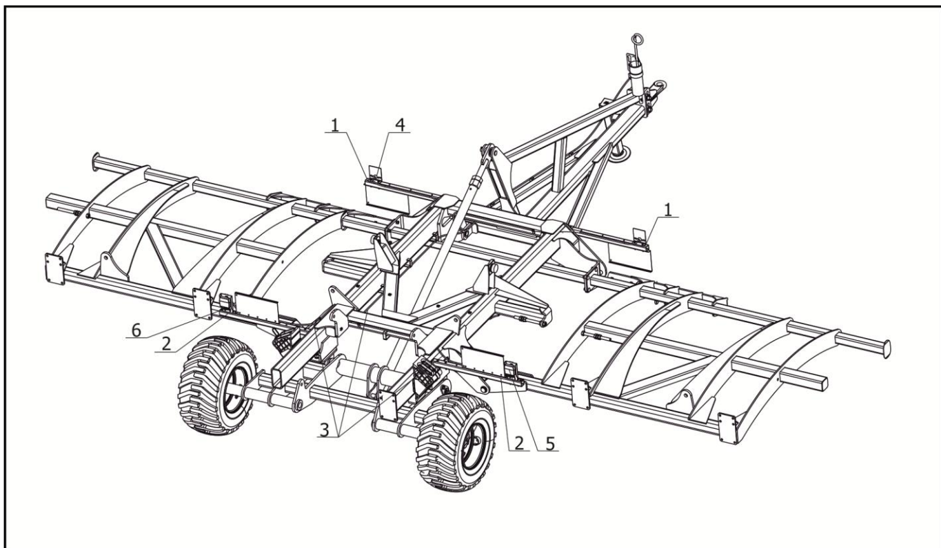
1,2 – кронштейн для фонарей; 3 – жгут электропроводки; 4 – фонарь передний; 5 – фонарь задний; 6 – световозвращатель
