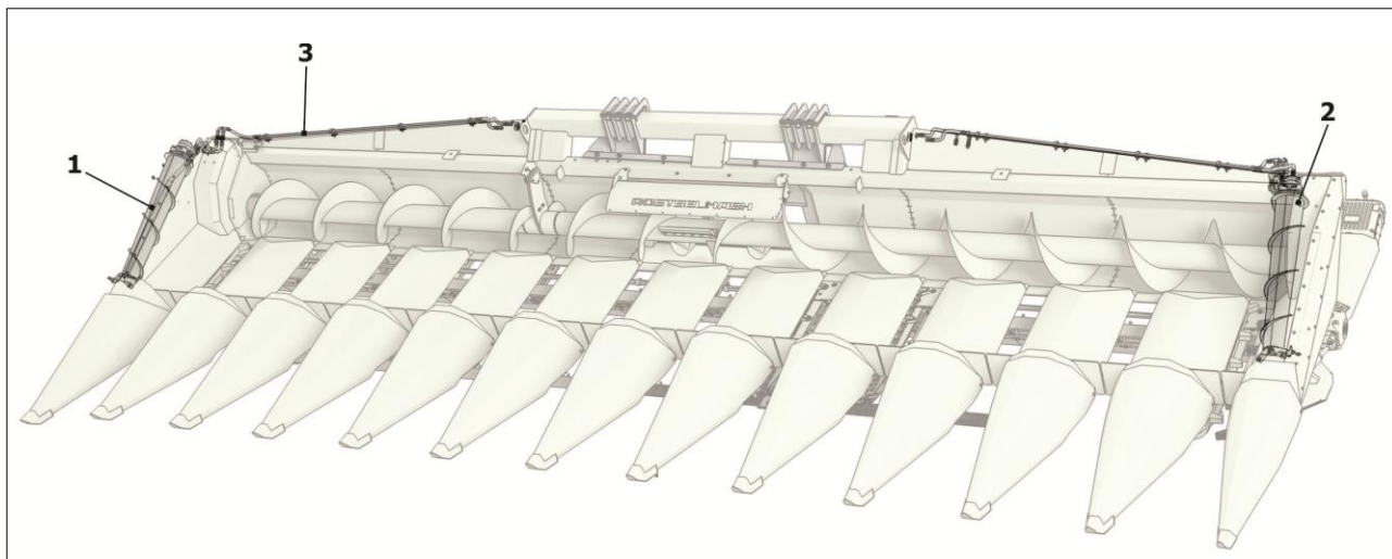
1 – Установка правого шнека; 2 – Установка левого шнека; 3 – Установка трубопроводов Рисунок 8.13 – Комплект активных делителей CS-1275.01.09.000
