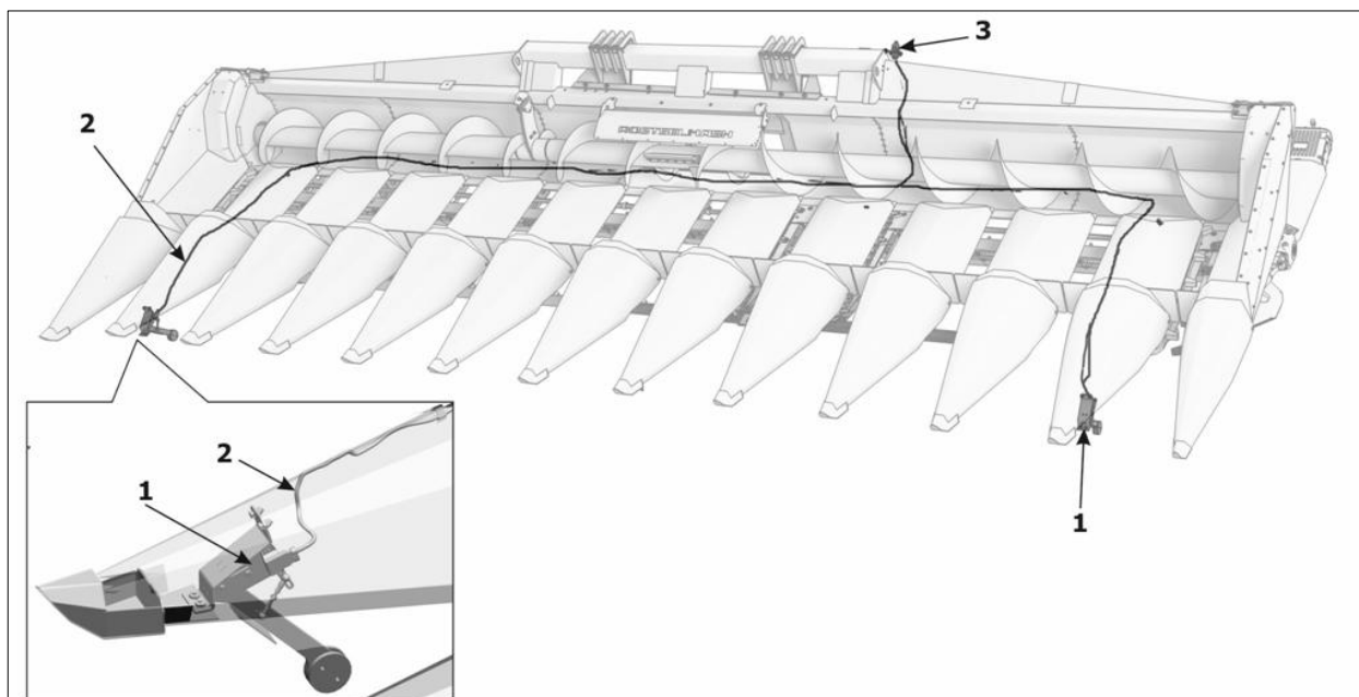
1 – Установка датчиков; 2 – Жгут; 3 – Розетка Рисунок 8.15 – Комплект датчиков CS-1275.01.08.000
