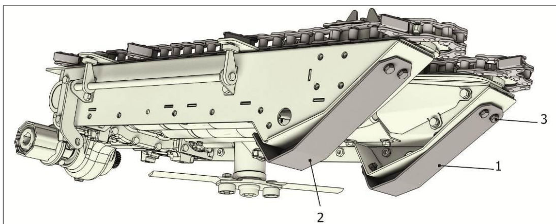
1, 2 – Подшо́ва; 3 – Болт
