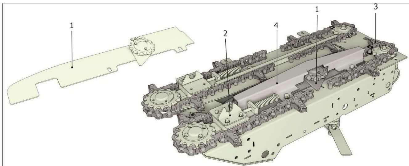
1 – Режущий аппарат CS-1275.33.01.010; 2 – Натяжник; 3 – Цепь; 4 – Успокоитель CS-1275.33.01.401 Рисунок 8.19 – Установка комплекта режущего аппарата CS-1275.33.01.000
