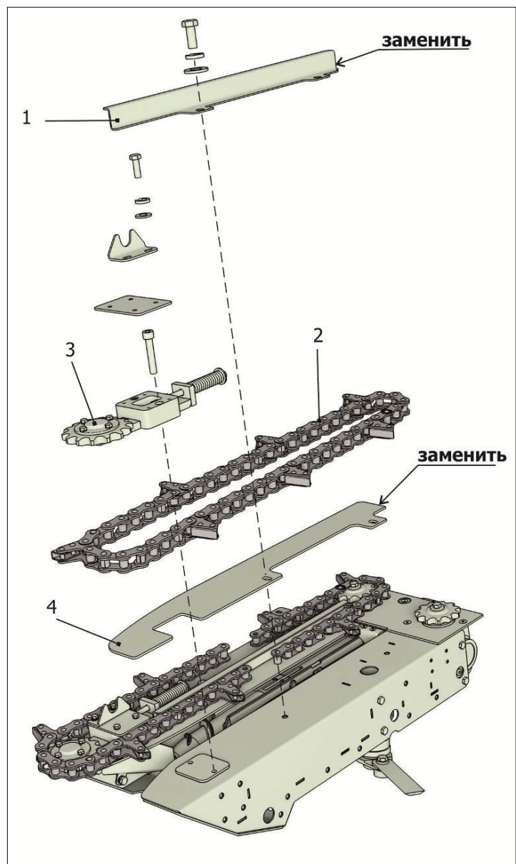
1 – Успокоитель CS-1275.01.16.424; 2 – Цепь; 3 – Натяжник; 4 – Отрывная пластина CS-1275.01.16.418 Рисунок 8.18 – Демонтаж деталей русла
