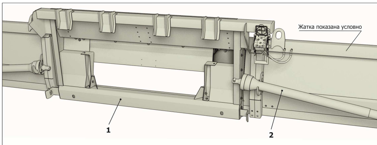
1-Рамка переходная ППК-81.63.00.000Г; 2-Вал карданный
