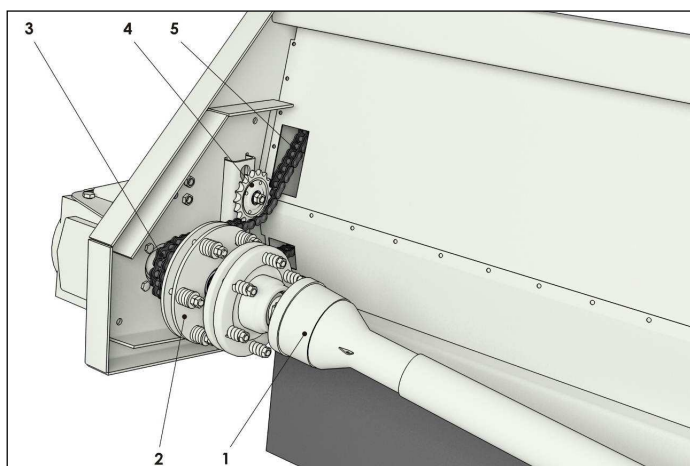
1-Карданный вал с предохранительной муфтой; 2-Предохранительная фрикционная муфта; 3-Ведущая звездочка привода шнека; 4-Натяжная звездочка; 5-Приводная цепь
