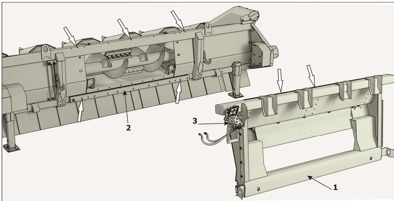
1-Нижняя балка проставки; 2- Балка каркасаятки; 3-Гидроразъем Рисунок 5.1
