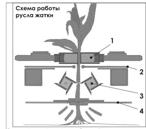
Режущие вальцы
