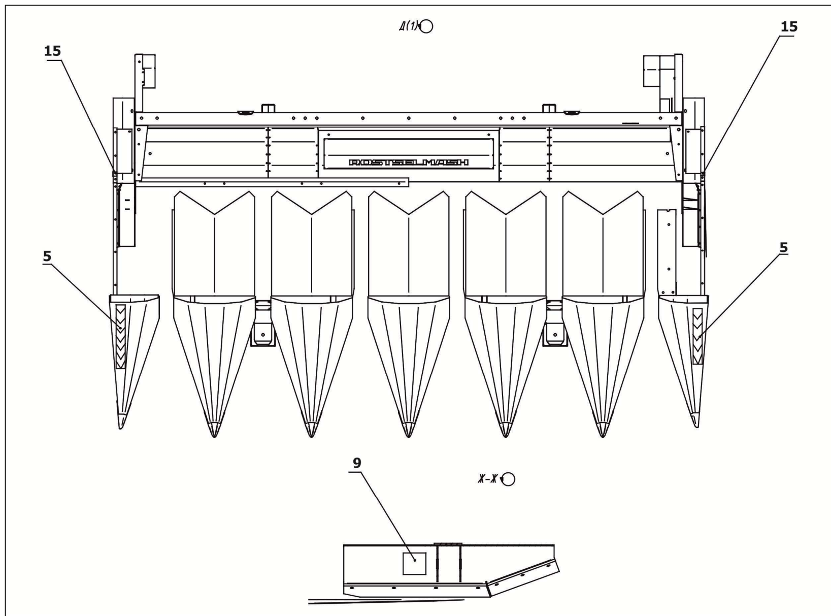
Рисунок 4.2 - Месторасположение табличек, аппликаций на приспособлении
