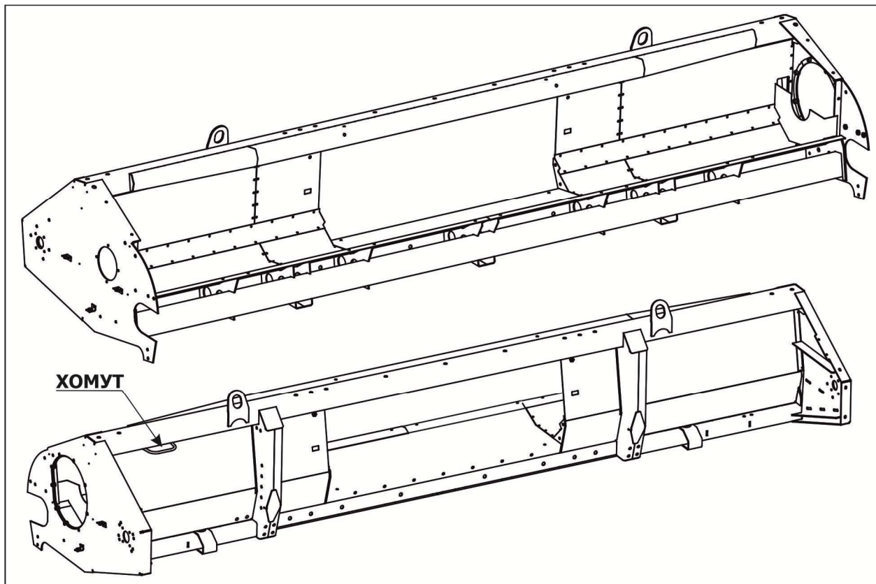
Рисунок 2.2 – Каркас жатки
