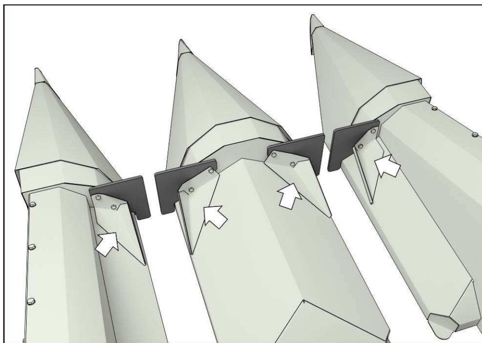
Рисунок 7.11 - Установка ловителей на капоты
