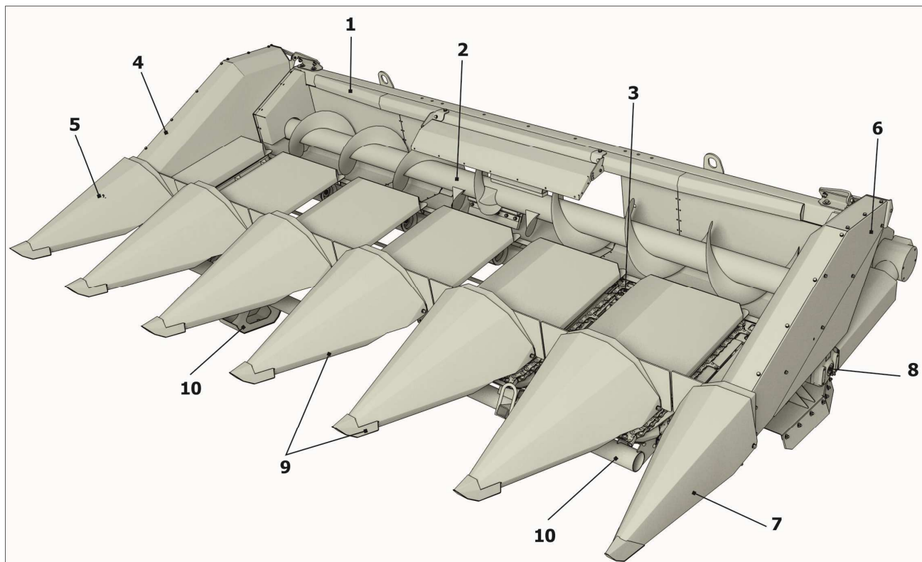
1-Каркас; 2-Шнек; 3-Русло; 4-Капот правый; 5-Делитель правый; 6-Капот левый; 7-Делитель левый; 8-Привод; 9-Делитель; 10-Траверса
