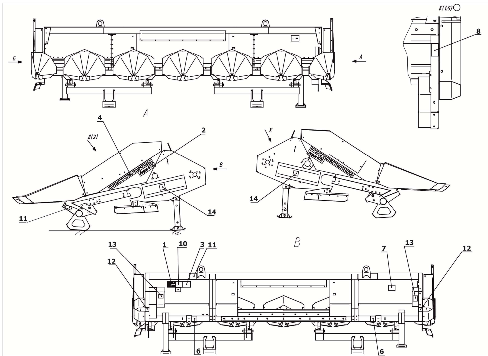
Рисунок 4.1 - Месторасположение табличек, аппликаций на приспособлении
