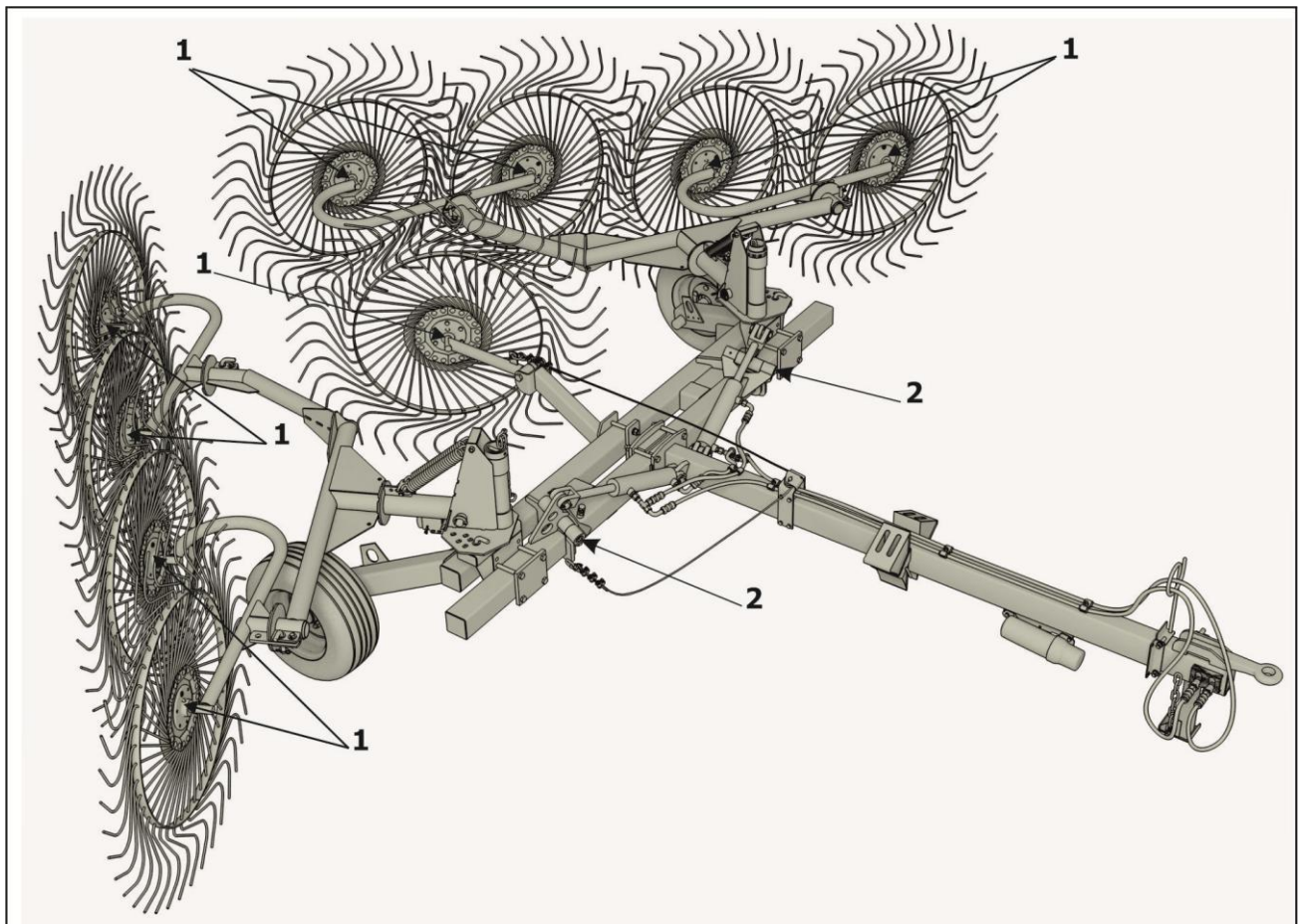
Рисунок 7.1 – Места смазки
