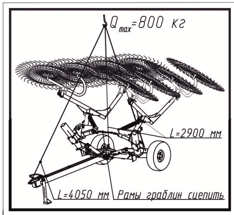
Рисунок 8.1 – Схема строповки
