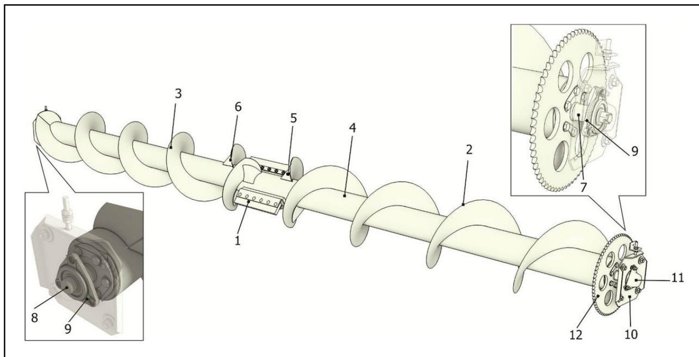
1 – Лопасть; 2 – Спираль левая; 3 – Спираль правая; 4 – Труба шнека; 5 – Виток левый; 6 – Виток правый; 7, 8 – Цапфа; 9 – Подшипниковая опора; 10 – Кронштейн; 11 – Колпачок; 12 – Звездочка
