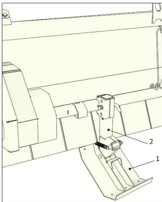
1 – Комплект приминателей стерни; 2 – Труба Рисунок 8.10
