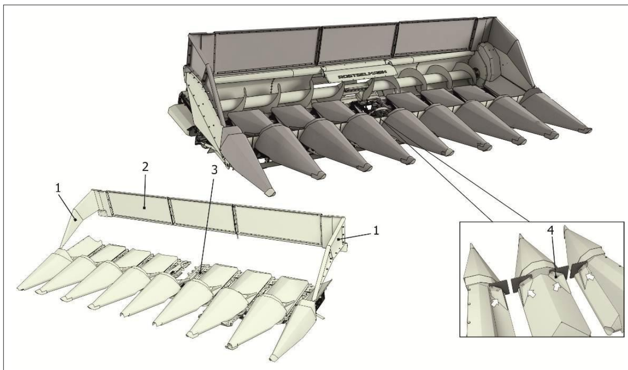
1 – Комплект увеличения бортов CS-1270.33.02.010; 2 – Комплект защитных щитков; 3 – Комплект режущего аппарата CS-1270.33.01.000; 4 – Комплект ловителей Рисунок 8.13 – Установка комплекта для уборки подсолнечника
