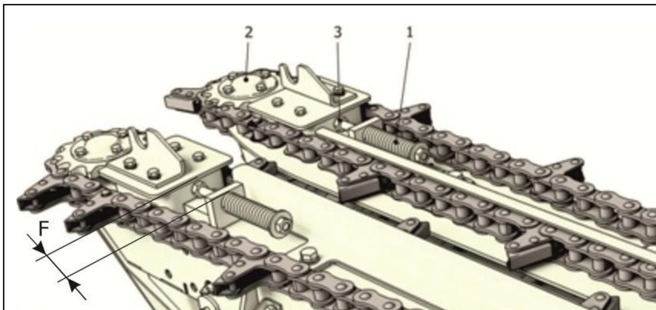
1 – Пружина; 2 – Звездочка; 3 – Гайка
