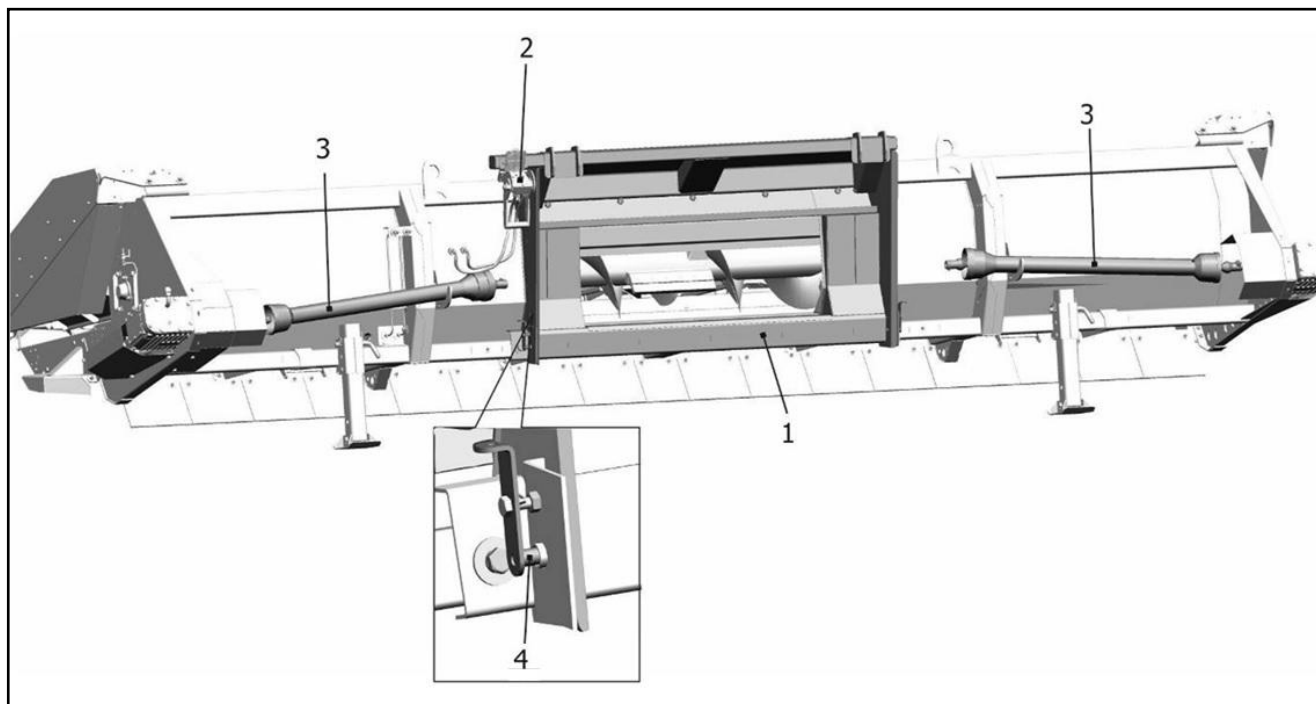
Рисунок 2.14 – RSM CS-875-47 Комплект для агрегатирования
