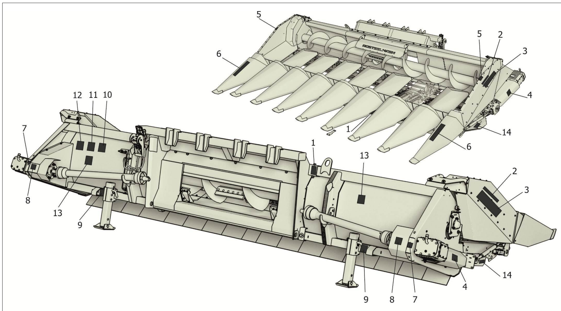
Рисунок 4.1 – Месторасположение табличек и аппликаций
