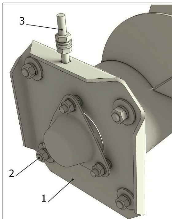
Рисунок 8.7 – Регулировка шнека
