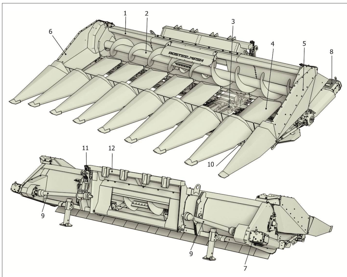
1 – Каркас; 2 – Шнек; 3 – Русло; 4 – Центральный капот с делителем; 5, 6 – Боковой капот с делителем; 7 – Редуктор боковой правый; 8 – Редуктор боковой левый; 9 – Вал карданный; 10 – Траверса; 11 – ЕГР; 12 – Комплект для агрегатирования
