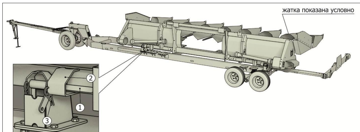
Рисунок 10.3 – Установка на тележке
