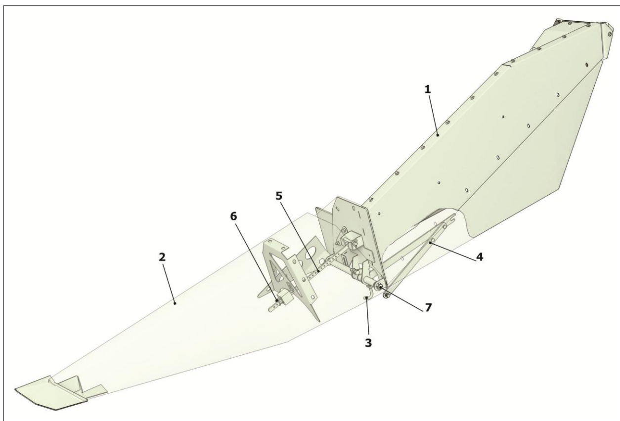
1 – Капот; 2 – Делитель; 3 – Зацеп; 4 – Фиксатор; 5 – Фиксатор; 6 – Шплинт; 7 – Шарнир
