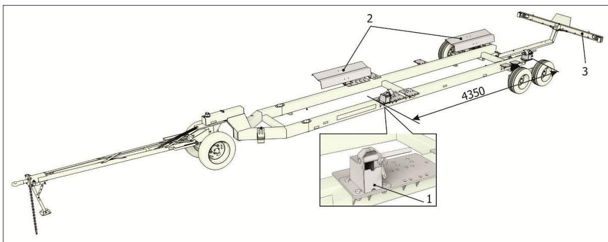
Рисунок 10.2 – Установка комплекта для транспортирования на тележке
