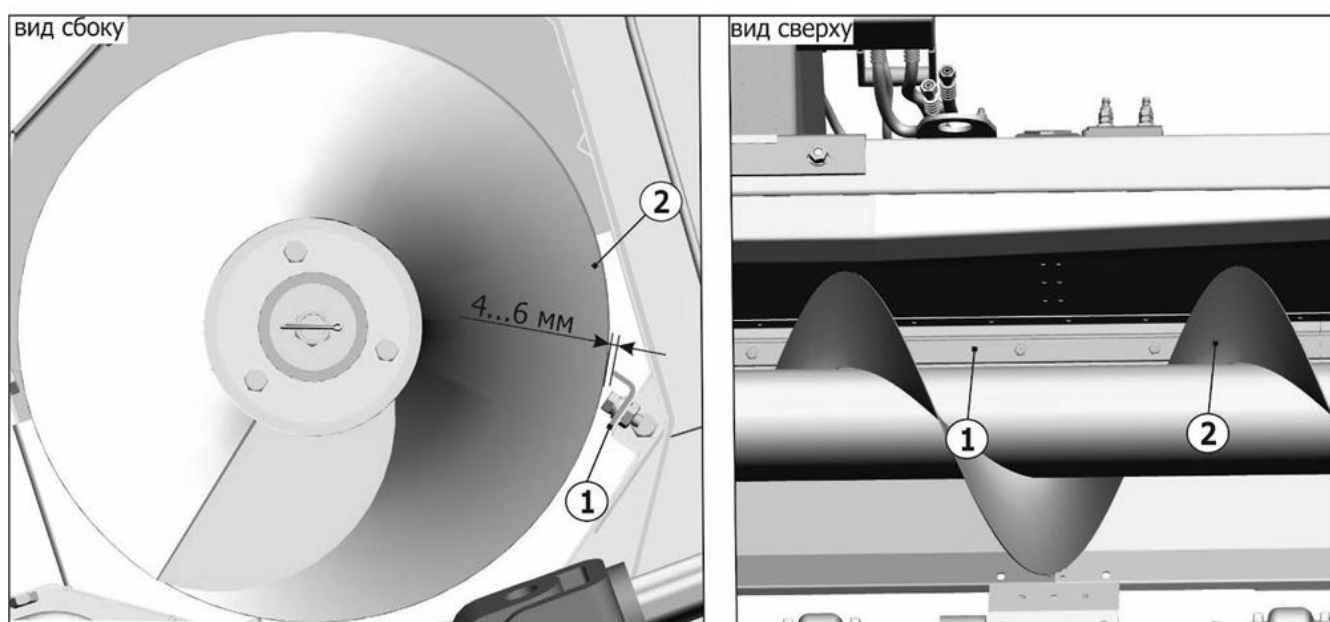
Рисунок 8.8 – Чистик шнека
