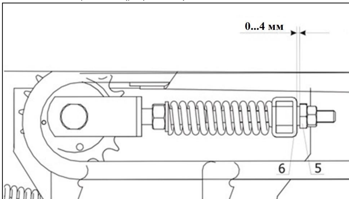
Рисунок 2.12 – Автоматическое натяжение транспортеров стеблей
