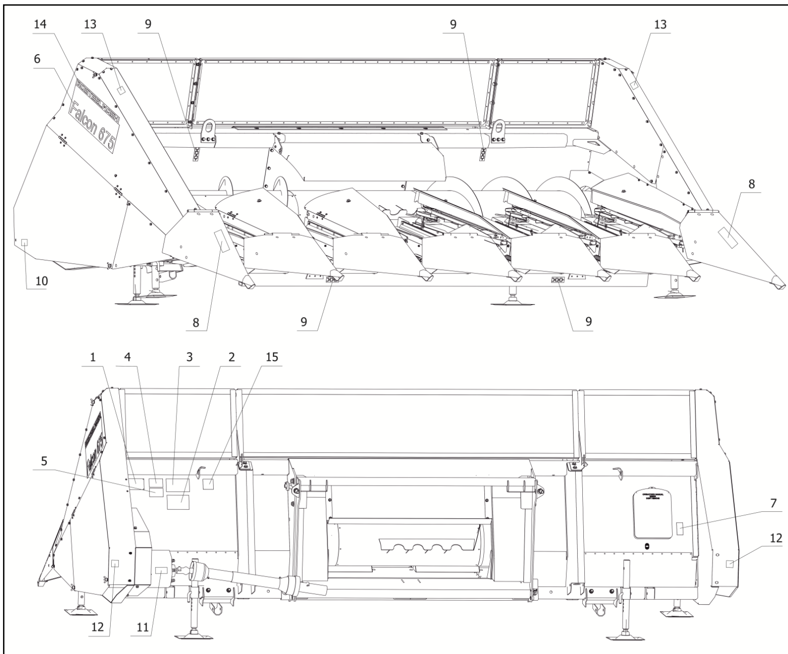
Рисунок 4.2 – Месторасположение табличек и аппликаций на приспособлении ПСП-675
