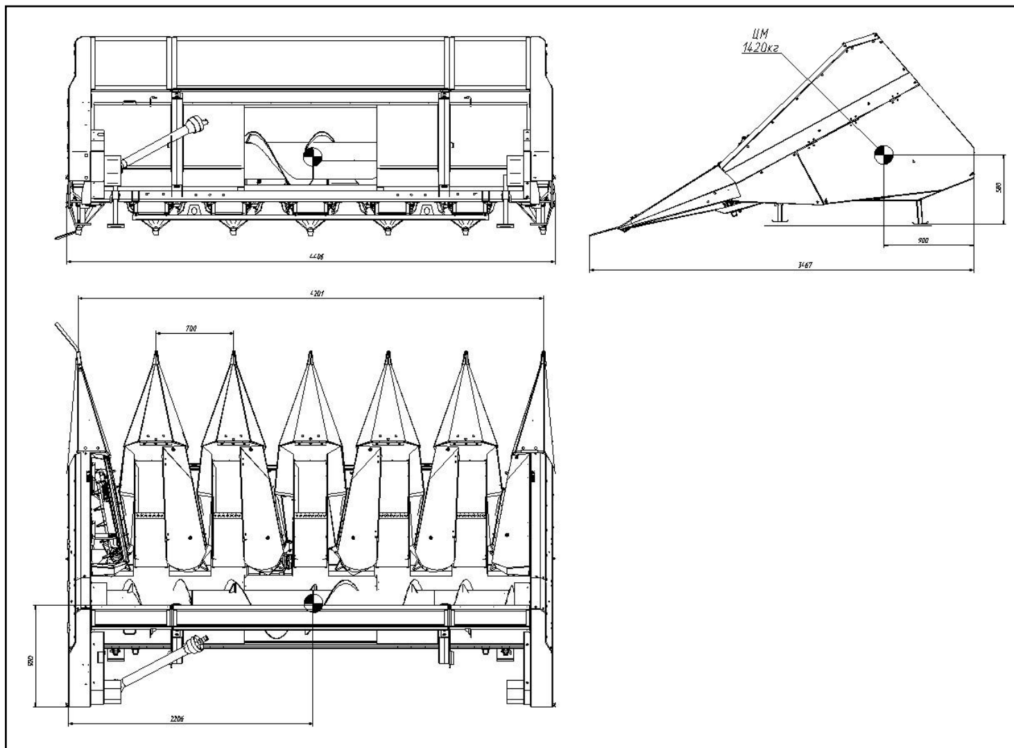
Рисунок Г.1 – Габаритные размеры приспособления ПСП-670 и расположение центра масс
