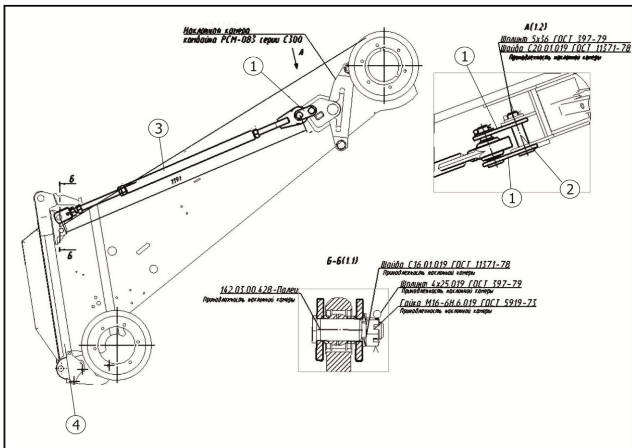
1 – Ушко; 2 – 2-ось; 3 – Тяга; 4 – Рамка
