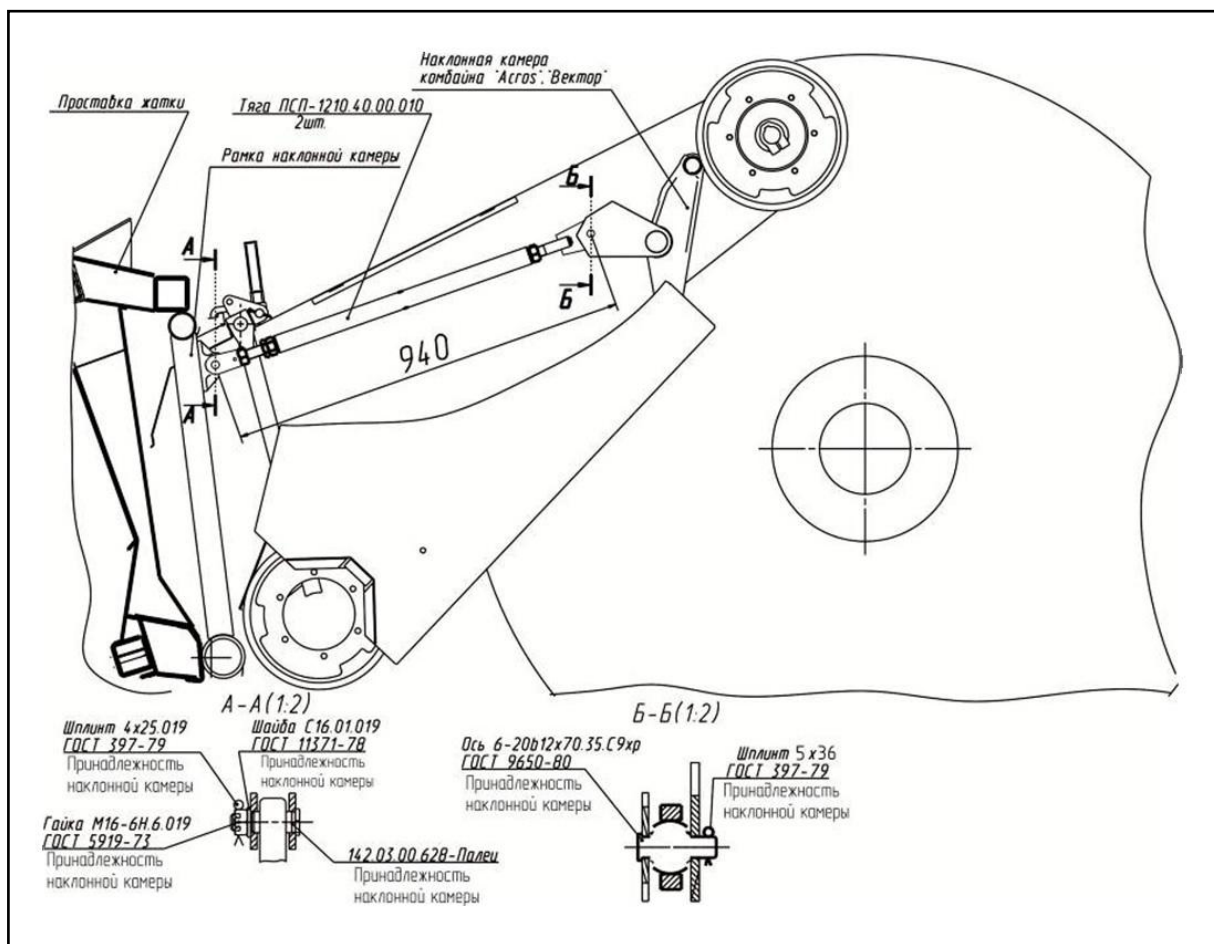
Рисунок 6.4 – Установка тяг на наклонную камеру комбайнов «ACROS»
