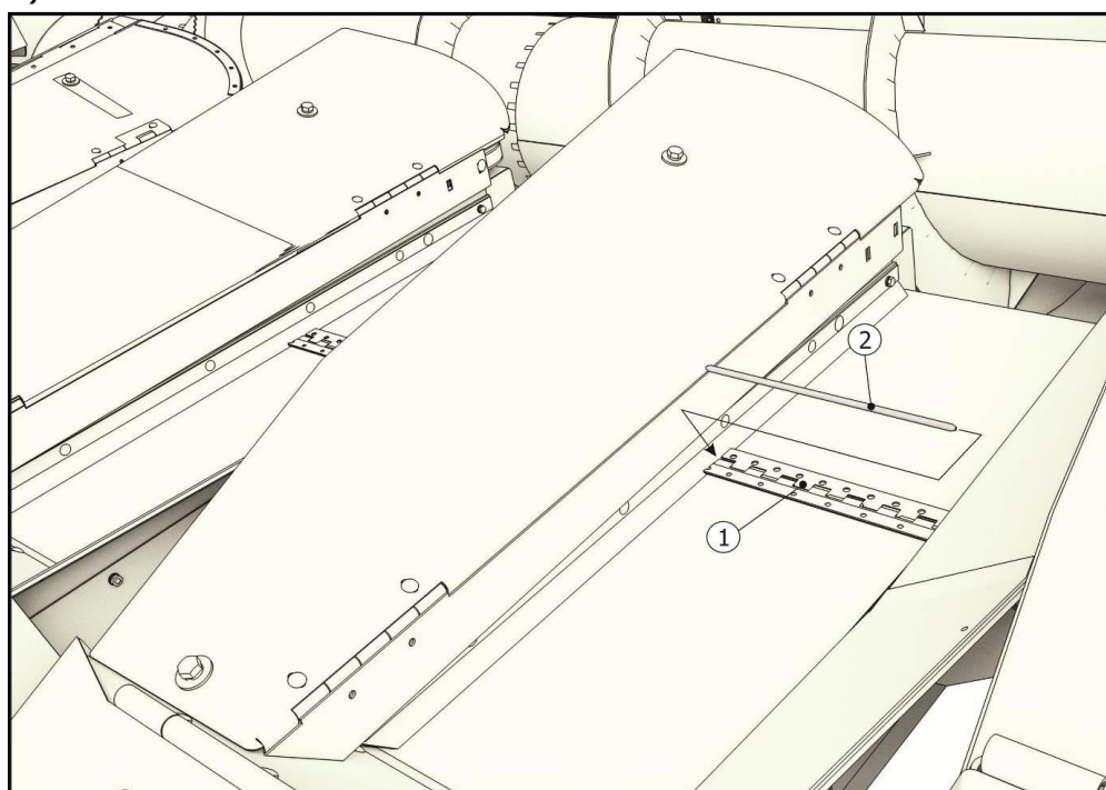
1 – Петля ПСХ-01.462; 2 – Ось ПСП-810.01.01.601
