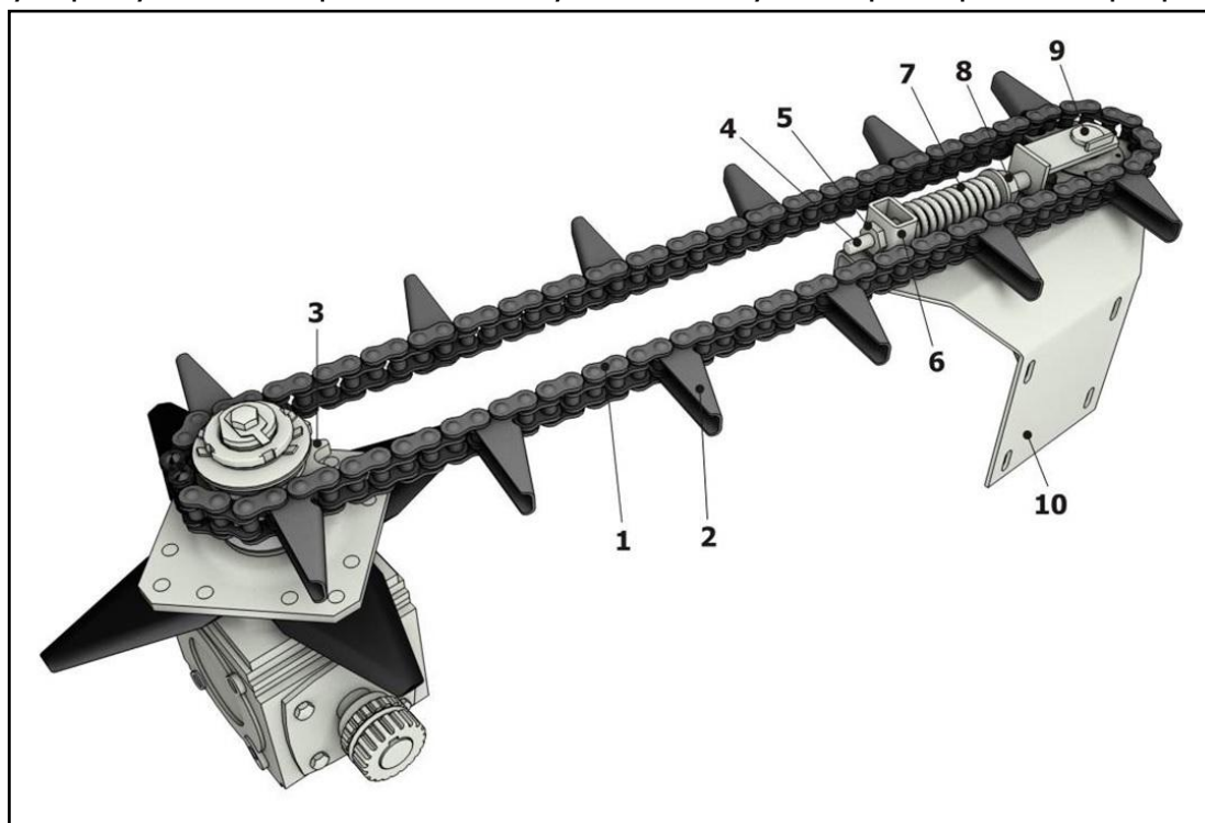
Рисунок 2.11 – Транспортер стеблей
