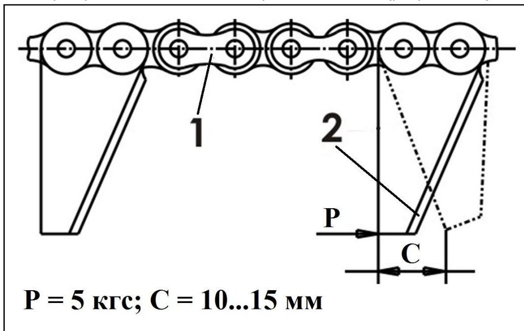
Рисунок 2.13 – Контроль натяжения транспортеров стеблей
