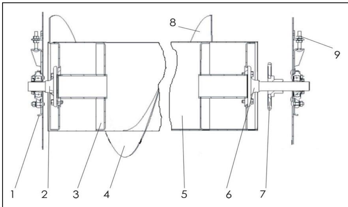
1 – Пластина подвижная; 2 – Цапфа правая; 3 – Диск; 4 – Спираль правая; 5 – Труба шнека; 6 – Цапфа левая; 7 – Звездочка привода; 8 – Спираль левая; 9 – Тяга регулировочная
