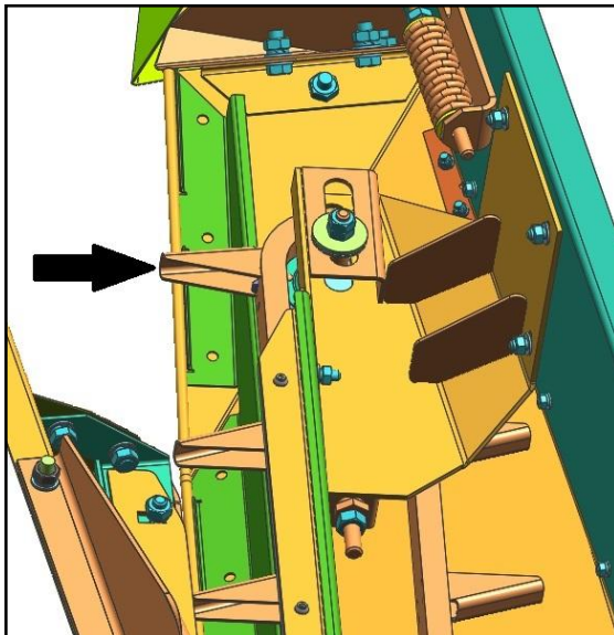
Рисунок 2.3 – Транспортер стеблей
