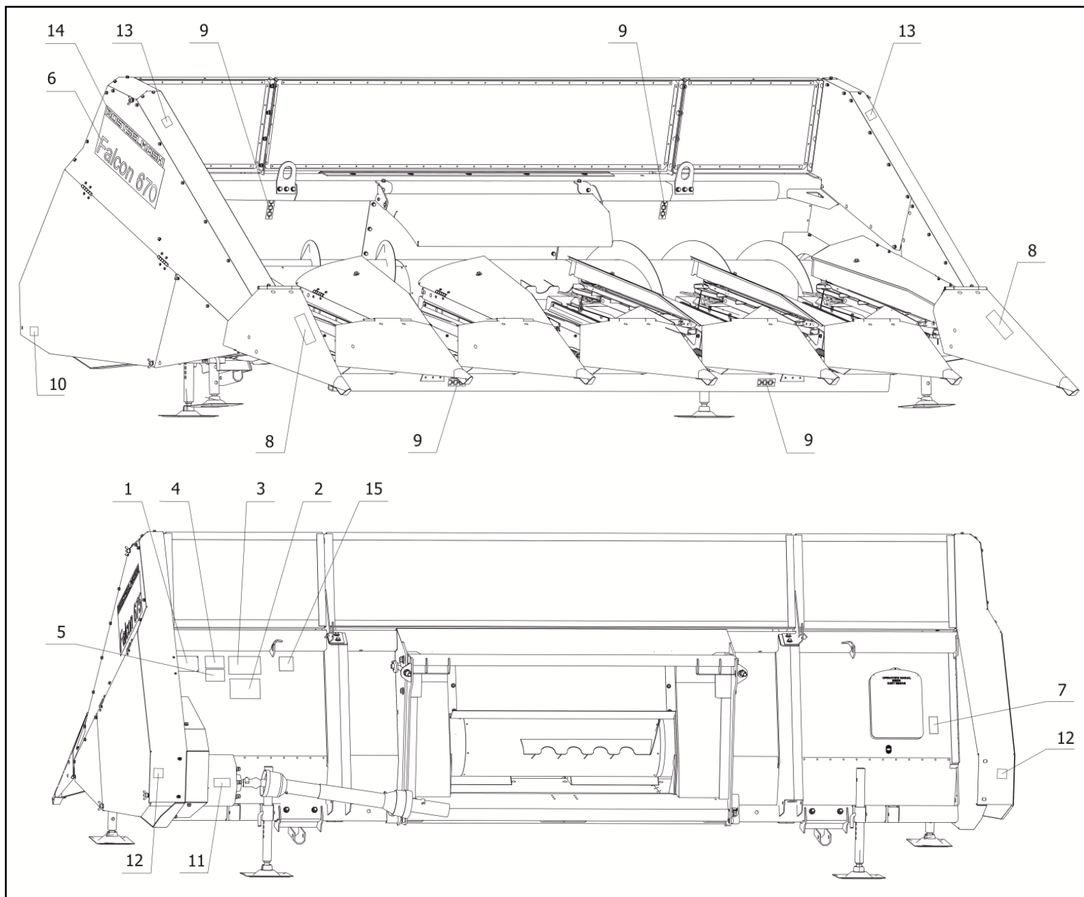
Рисунок 4.1 – Месторасположение табличек и аппликаций на приспособлении ПСП-670
