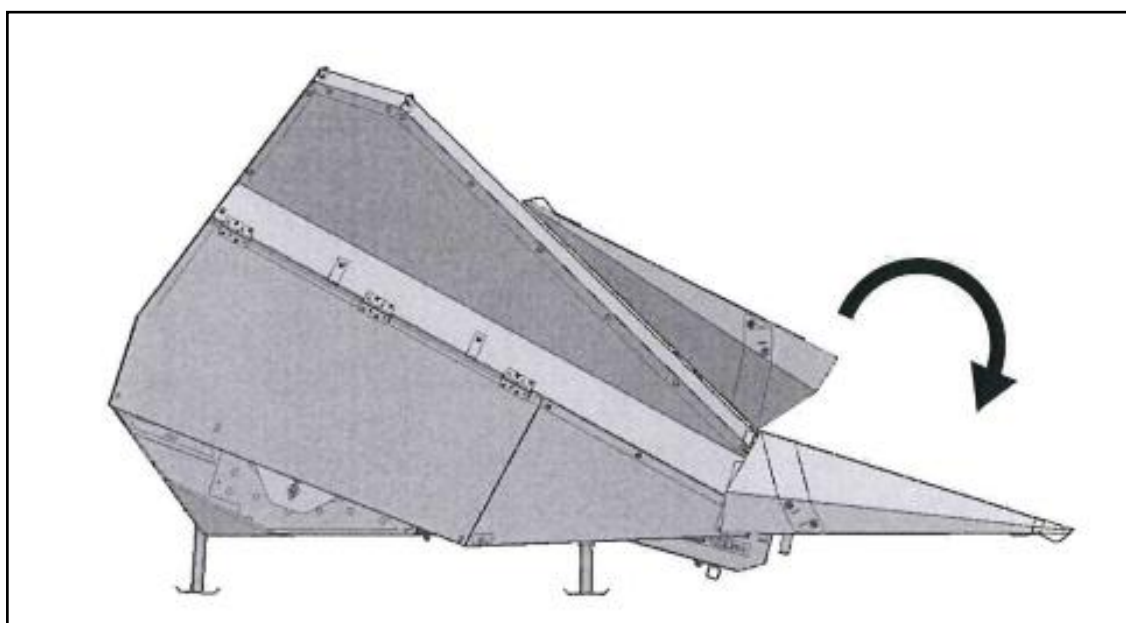
Рисунок 2.6 – Перевод боковых делителей в транспортное положение
