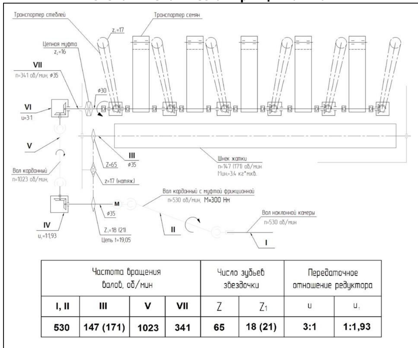
Рисунок А.1 – Схема кинематическая принципиальная
