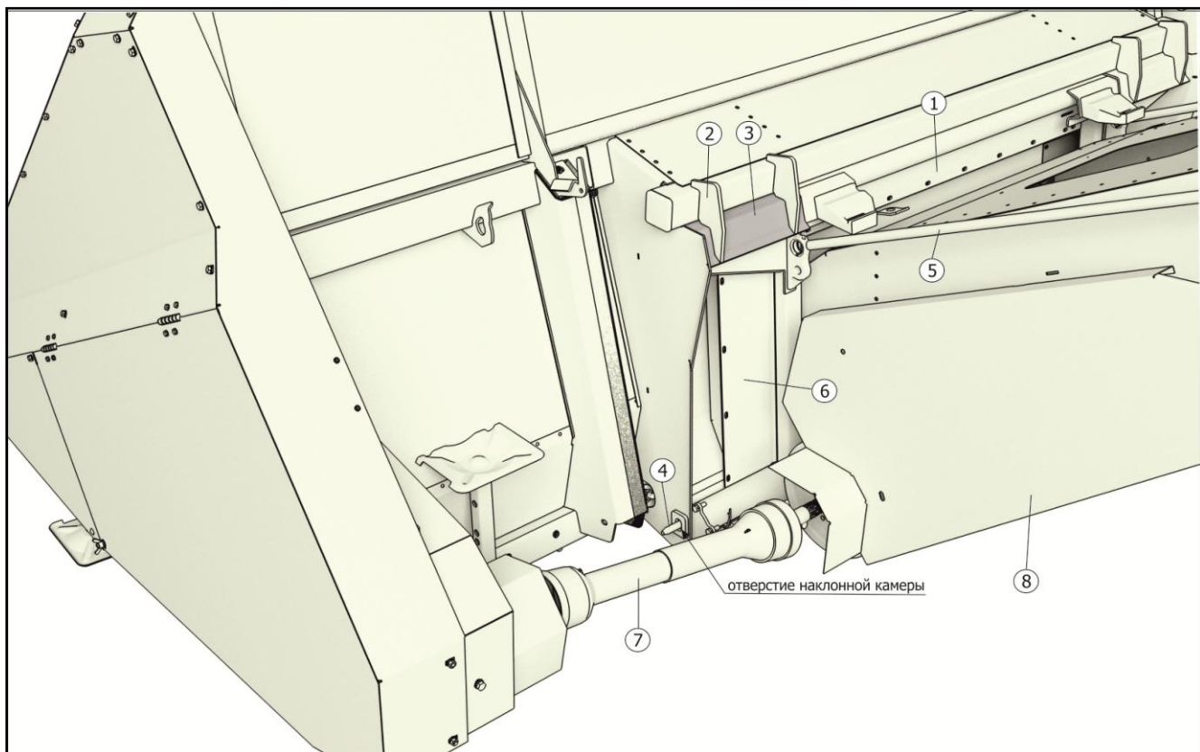
1 – Верхняя труба наклонной камеры; 2 – Зацеп; 3 – Ловители жатки; 4 – Штырь наклонной камеры; 5 – Тяга; 6 – Рамка наклонной камеры; 7 – Карданный вал; 8 – Корпус наклонной камеры
