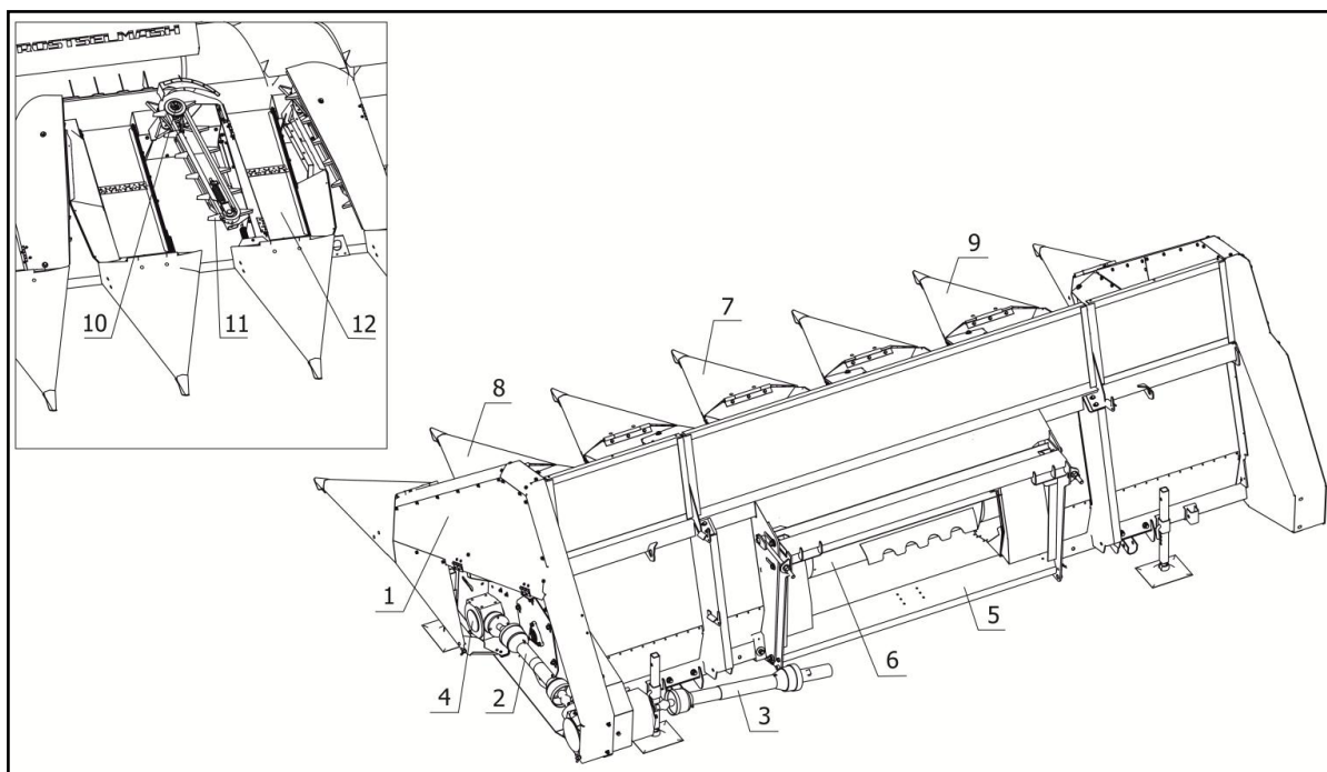
1 – Корпус жатки; 2 – Карданный вал боковой; 3 – Карданный вал с предохранительной муфтой; 4 – Боковой редуктор; 5 – Переходная рамка; 6 – Шнек; 7 – Лифтер центральный; 8 – Лифтер левый; 9 – Лифтер правый; 10 – Режущий аппарат; 11 – Транспортёр стеблей; 12 – Транспортёр семян
