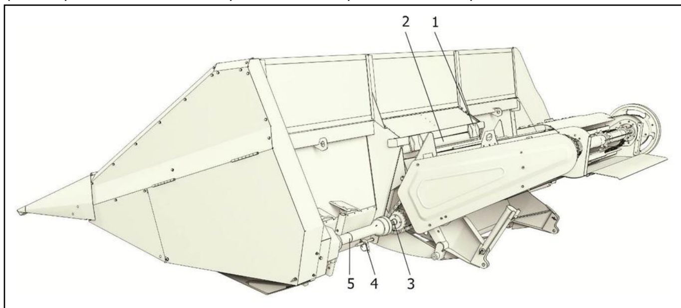
1 – Верхняя труба; 2 – Ловитель; 3 – Переходник; 4 – Фиксатор; 5 – Карданный вал
