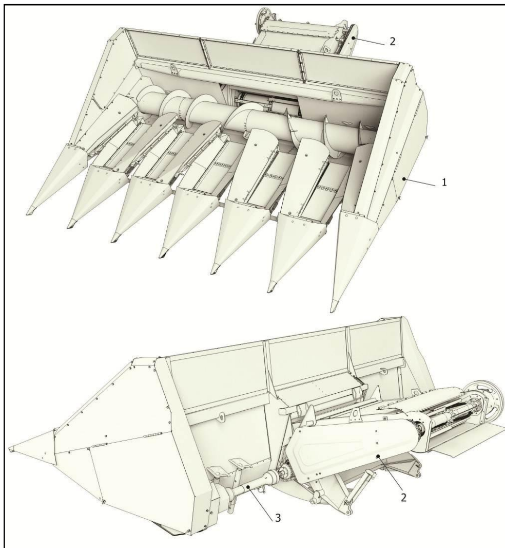
1 – Жатка; 2 – Наклонная камера; 3 – Карданный вал
