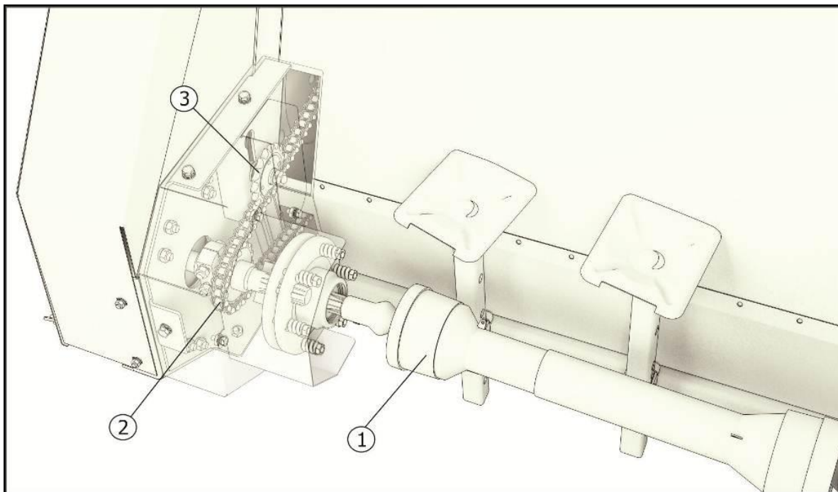
1 – Карданный вал; 2 – Цепь; 3 – Натяжная звездочка
