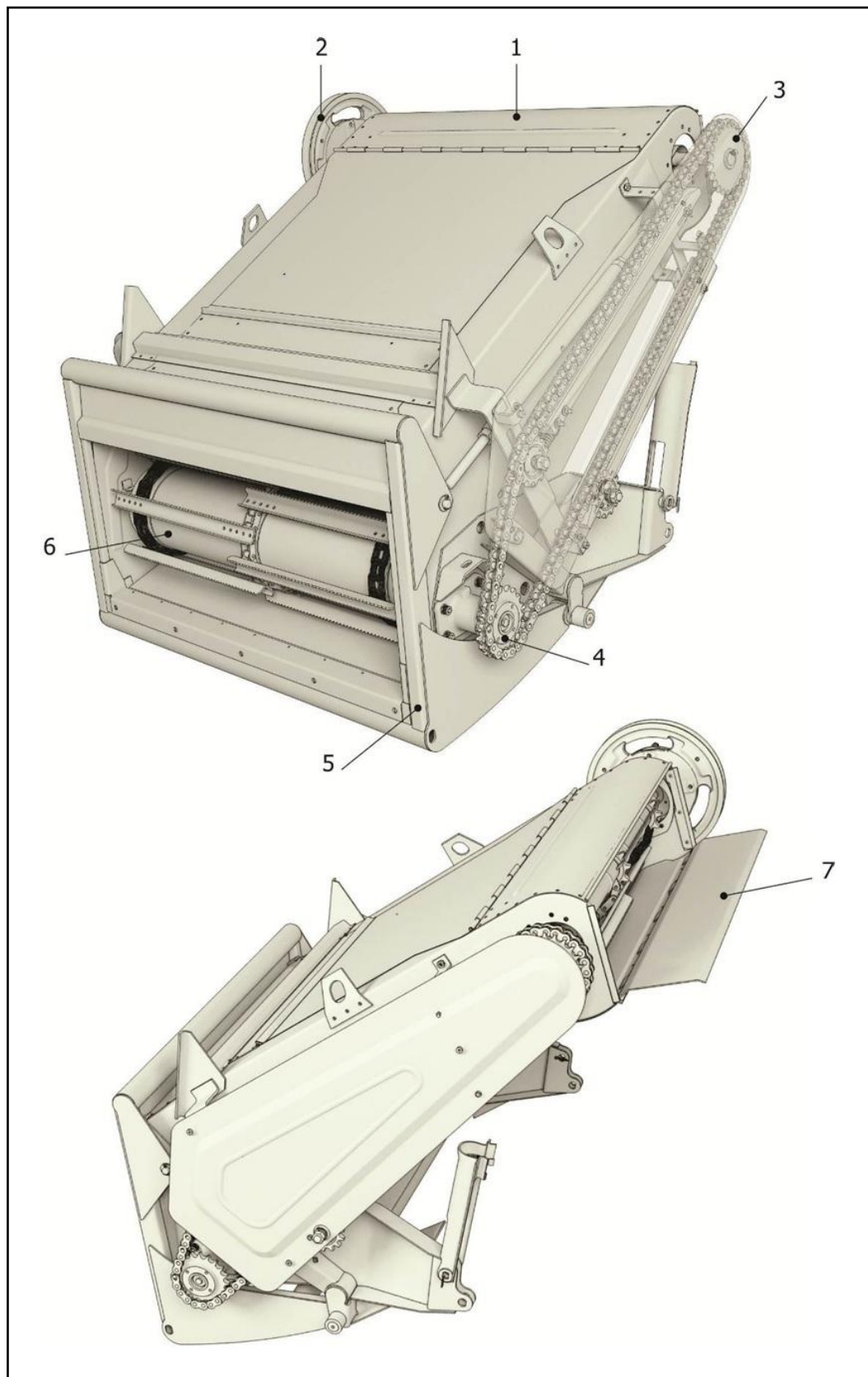
1 – Корпус; 2 – Шкив; 3 – Звездочка; 4 – Вал; 5 – Рамка; 6 – Транспортер Рисунок 6.8 – Вид наклонной камеры после доработки по комплекту ППК-41.20.07.000-01
