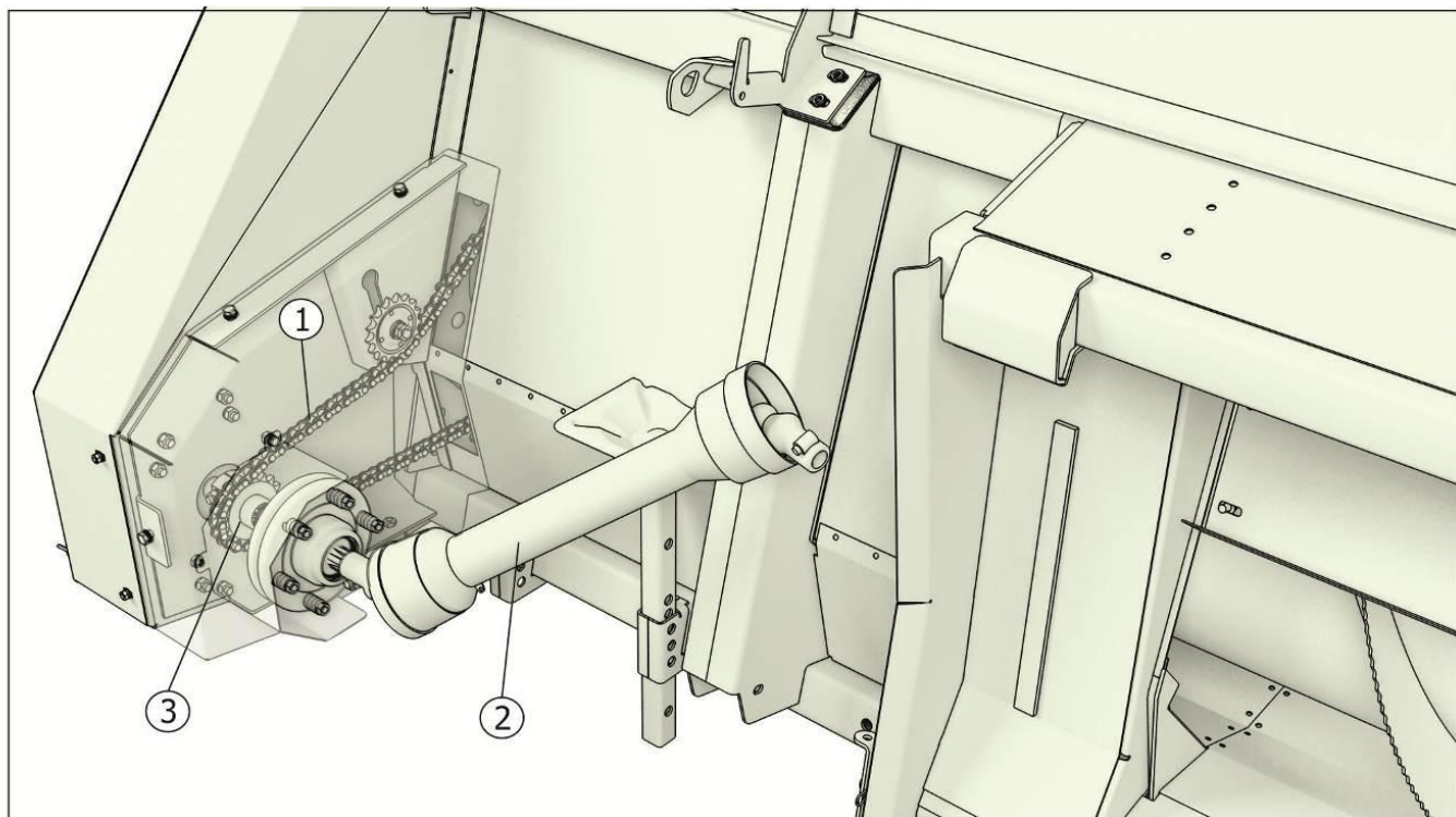
1 – Цепь; 2 – Карданный вал; 3 – Натяжная звездочка
