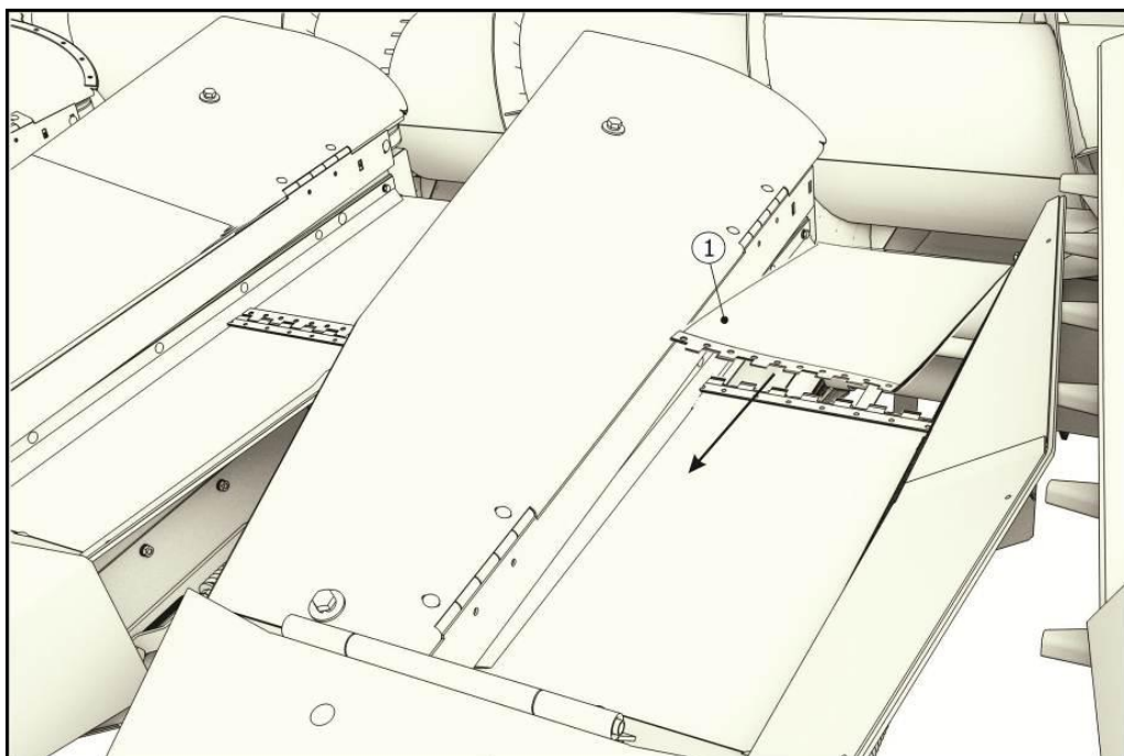
1 – Лента Рисунок 6.11
