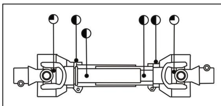
Рисунок 8.2 – Места и периодичность смазки карданного вала
