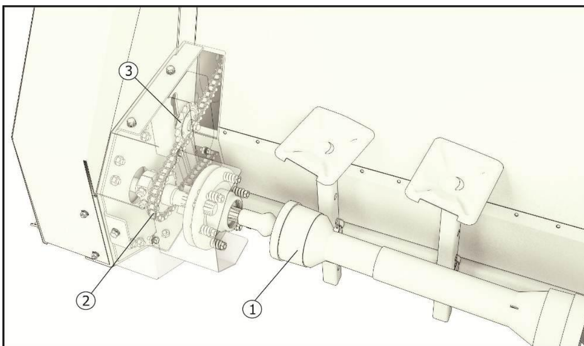
1 – Карданный вал; 2 – Цепь; 3 – Натяжная звездочка
