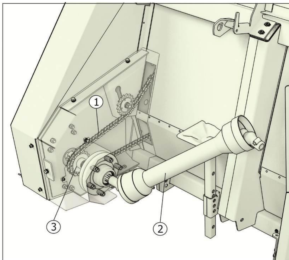
1 – Цепь; 2 – Карданный вал; 3 – Натяжная звездочка
