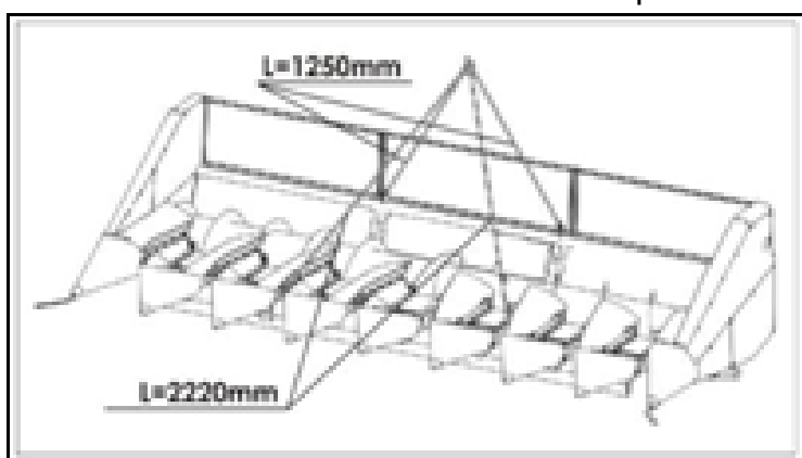
Рисунок 9.1 – Схема строповки
