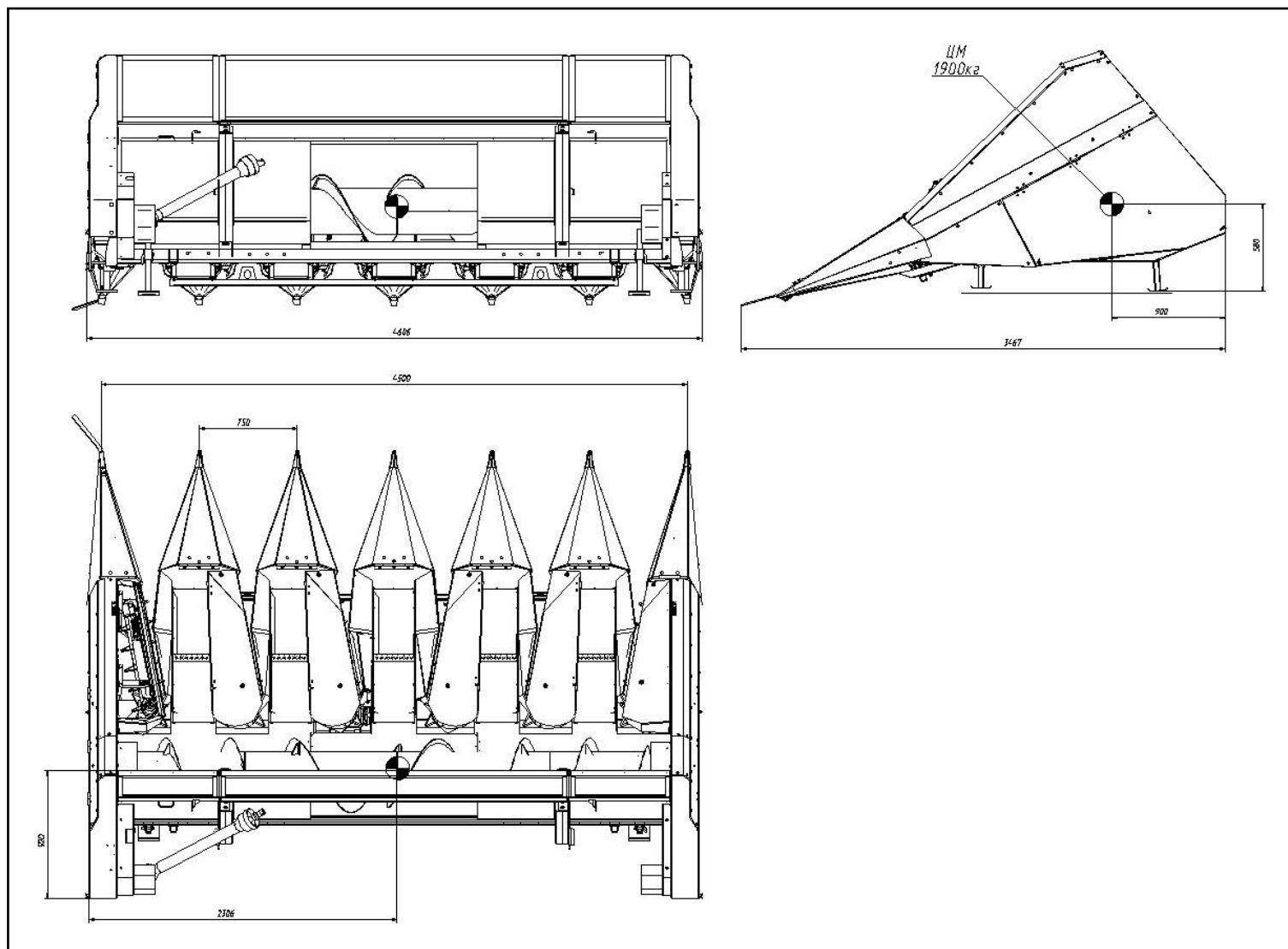
Рисунок Г.2 – Габаритные размеры приспособления ПСП-675 и расположение центра масс
