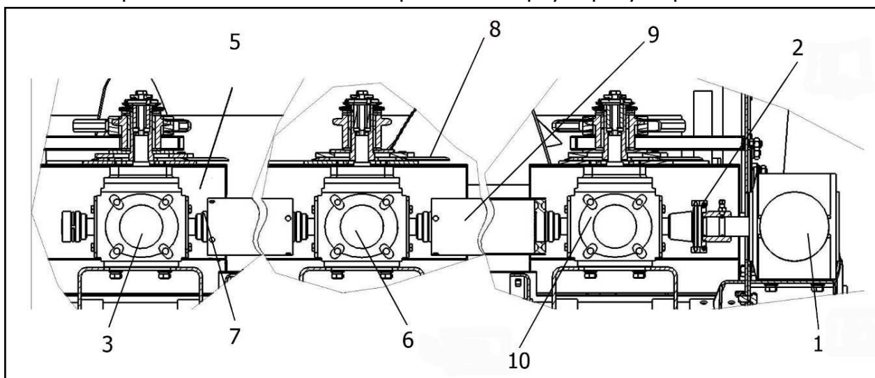
1 – Угловой редуктор; 2 – Цепная муфта; 3, 6, 10 – Конический редуктор; 5 – Кожух защитный; 7 – Муфта шлицевая; 8 – Противорежущая пластина; 9 – Валик транспортера семян
