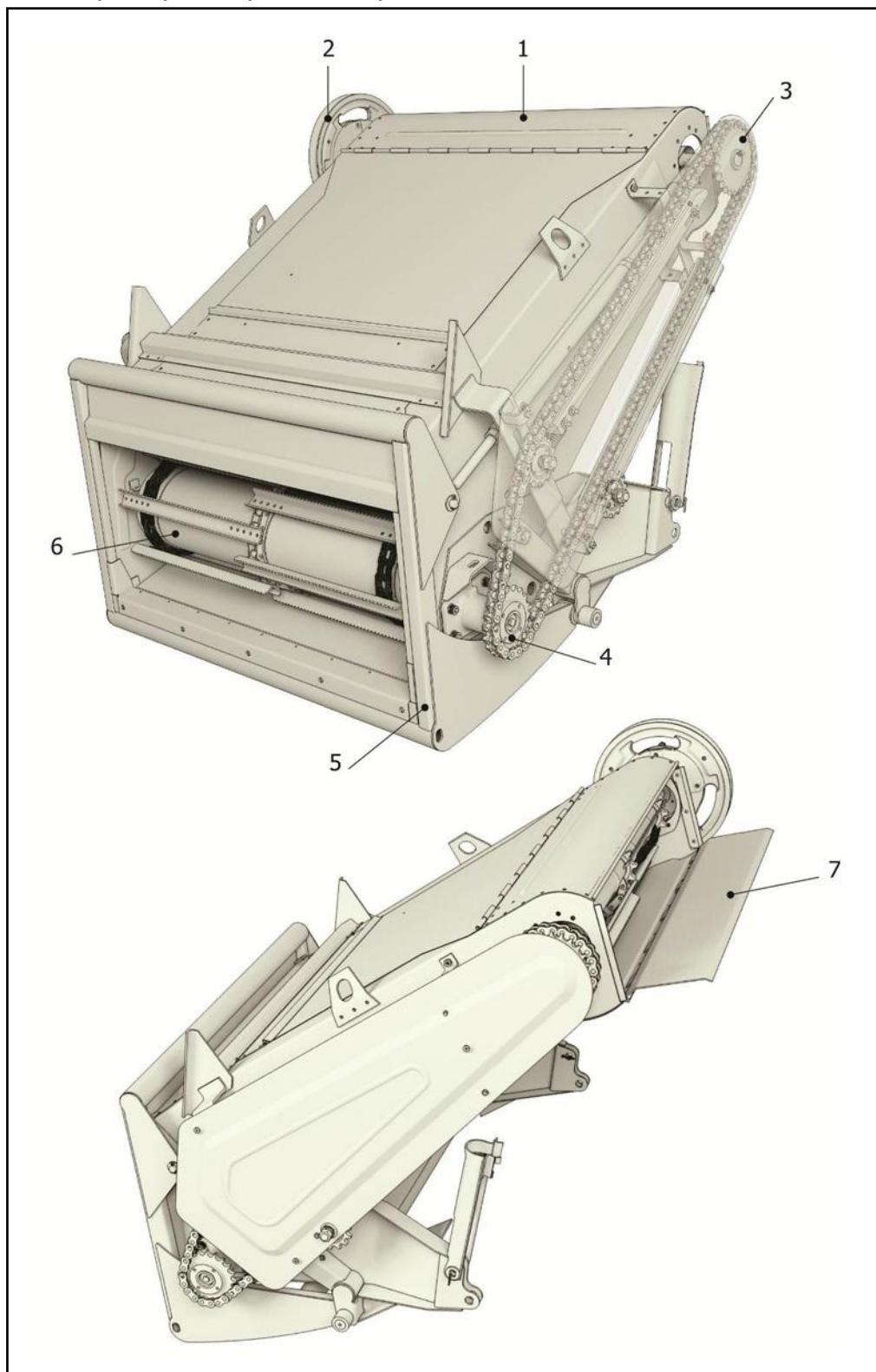
1 – Корпус; 2 – Шкив; 3 – Звездочка; 4 – Вал; 5 – Рамка; 6 – Транспортер
