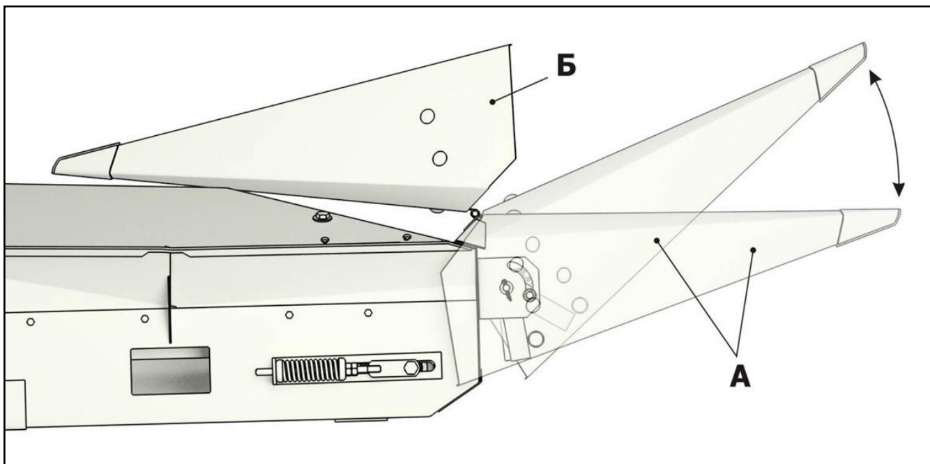
Рисунок 2.10 – Положения делителя
