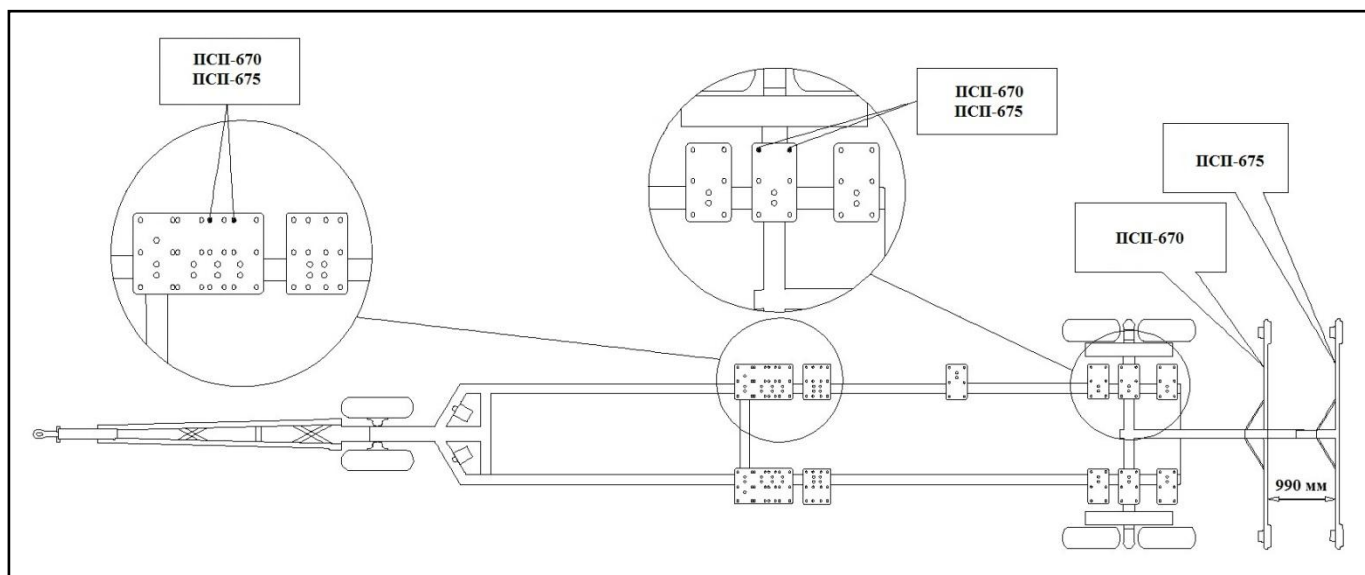
Рисунок 9.3 – Установка опор приспособления ПСП-670
