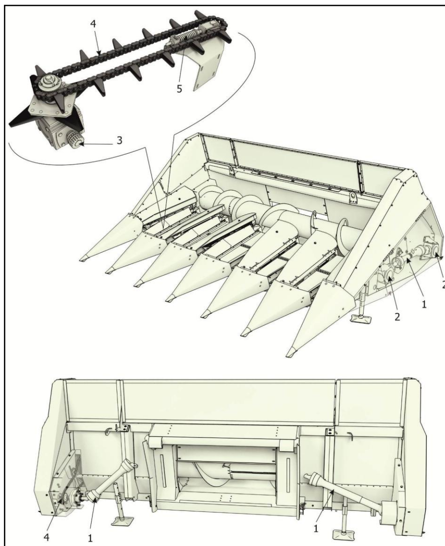
Рисунок 8.1 – Места смазки приспособления
