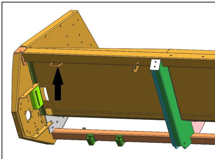
Рисунок 2.2 – Хомут
