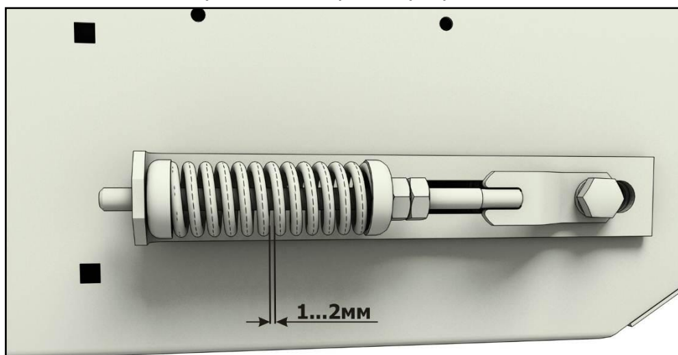
Рисунок 2.15 – Контроль натяжения транспортеров стеблей
