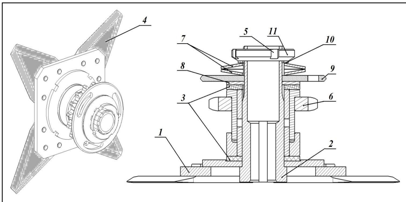
1 – Диск ножевой; 2 – Втулка шлицевая; 3 – Фрикционная накладка; 4 – Нож; 5 – Шайба стопорная; 6 – Звездочка транспортера стеблей; 7 – Тарельчатая пружина; 8, 9 – Шайба упорная; 10 – Шайба; 11 – Гайка
