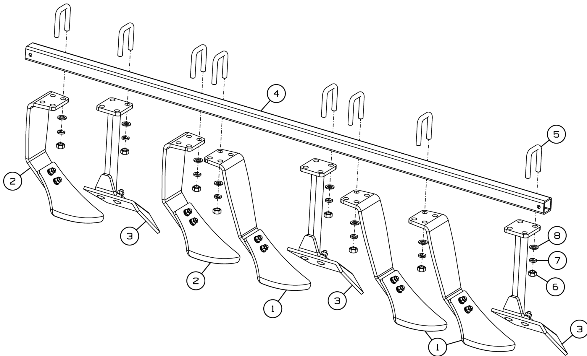
Рисунок 23 - Секция чистиков ДХ-1080.04.010А
