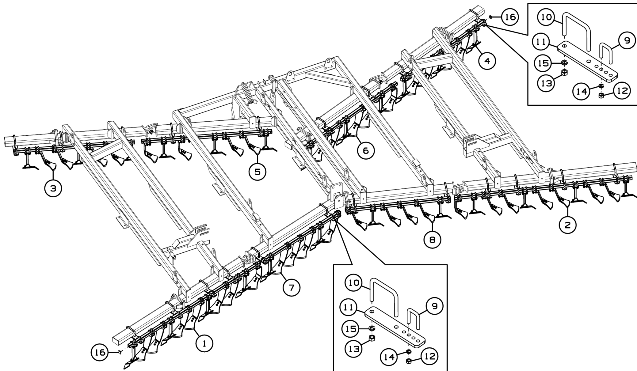
Рисунок 18 - Установка чистиков ДХ-880.04.000
