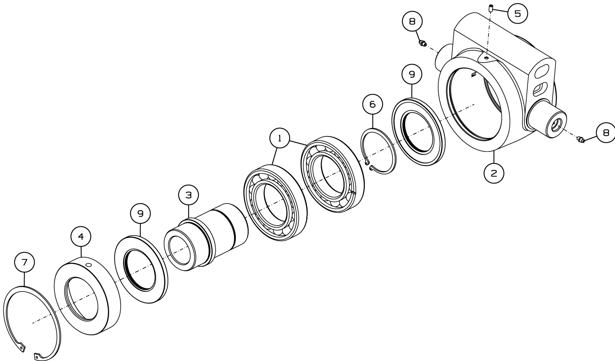
Рисунок 17 - Подшипниковая опора ДХ-1080.03.110
