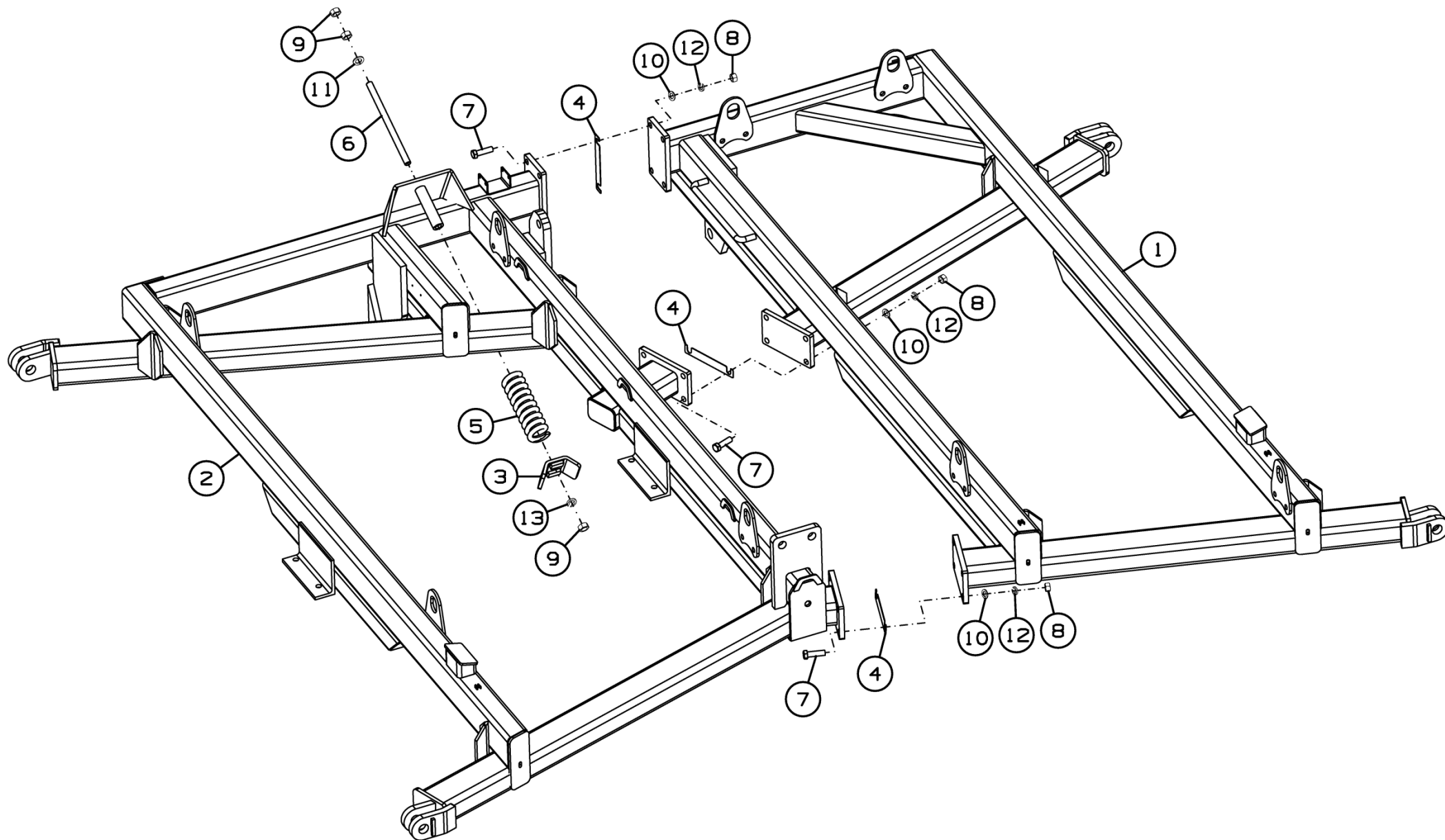
Рисунок 3 - Рама ДХ-1080.01.000
