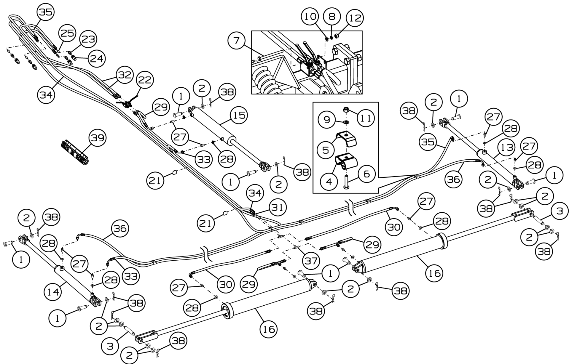
Рисунок 8 - Установка гидрооборудования ДХ-1080.12.000А-01
