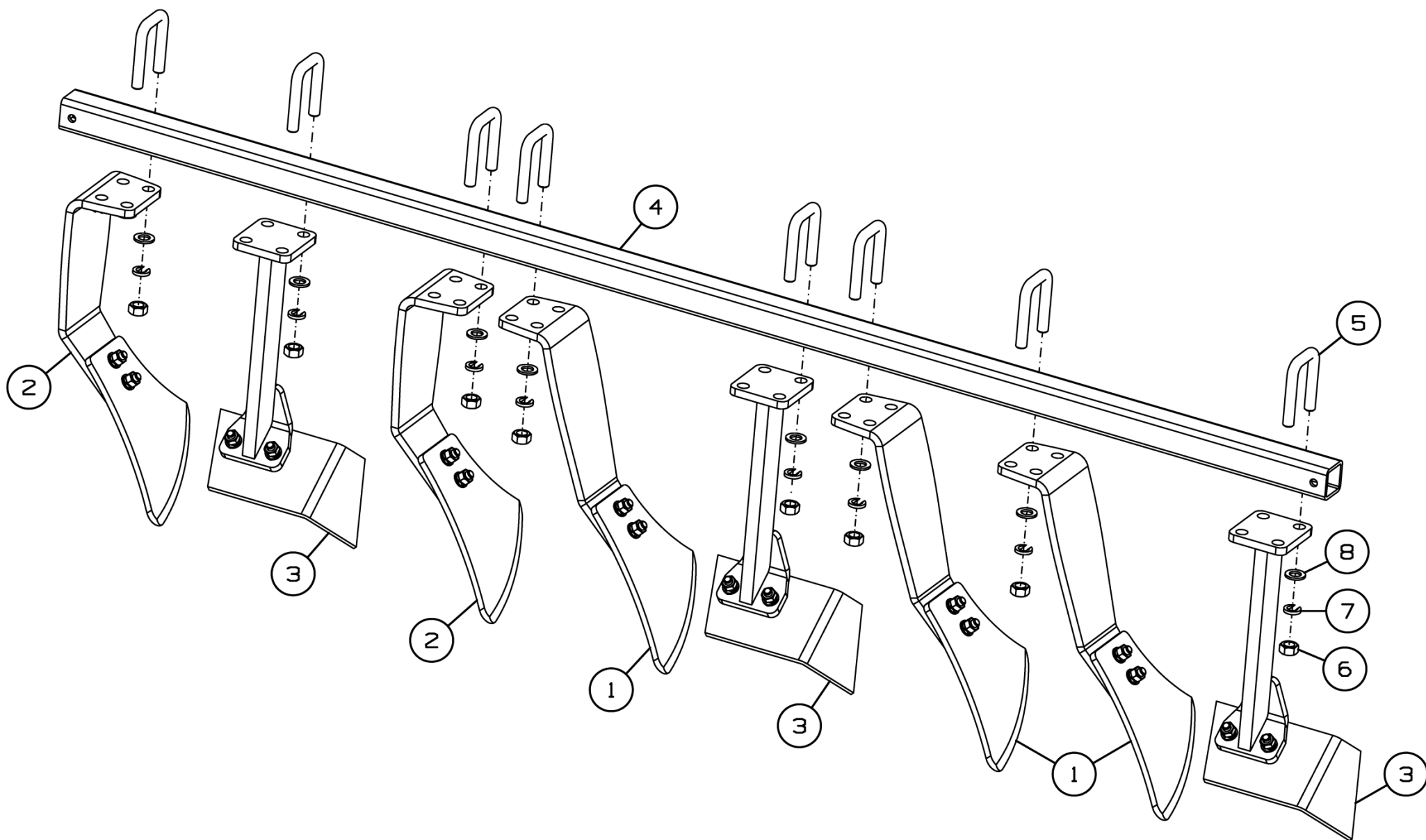
Рисунок 24 - Секция чистиков ДХ-1080.04.020А
