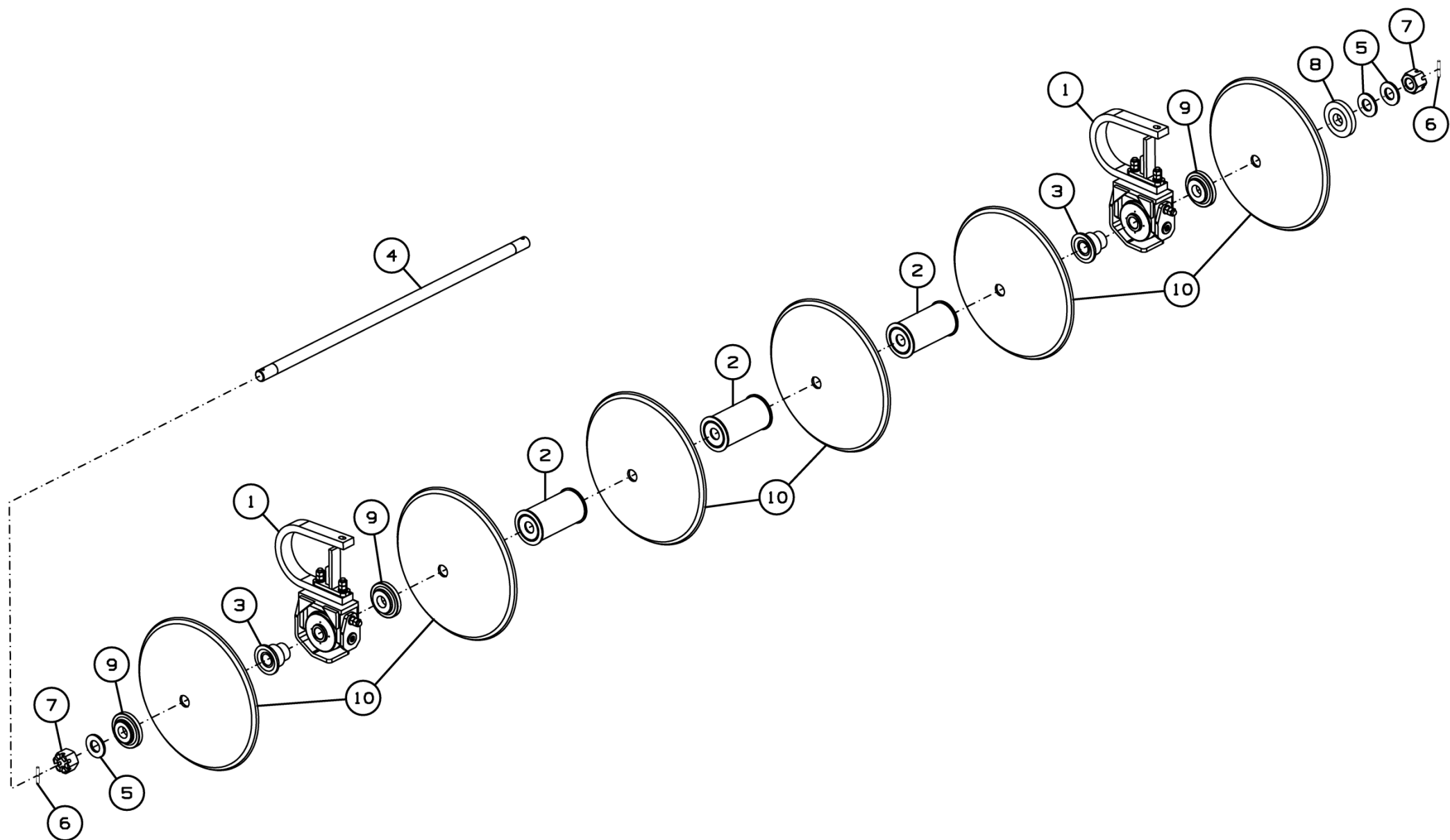
Рисунок 14 - Батарея ДХ-1080.03.030А
