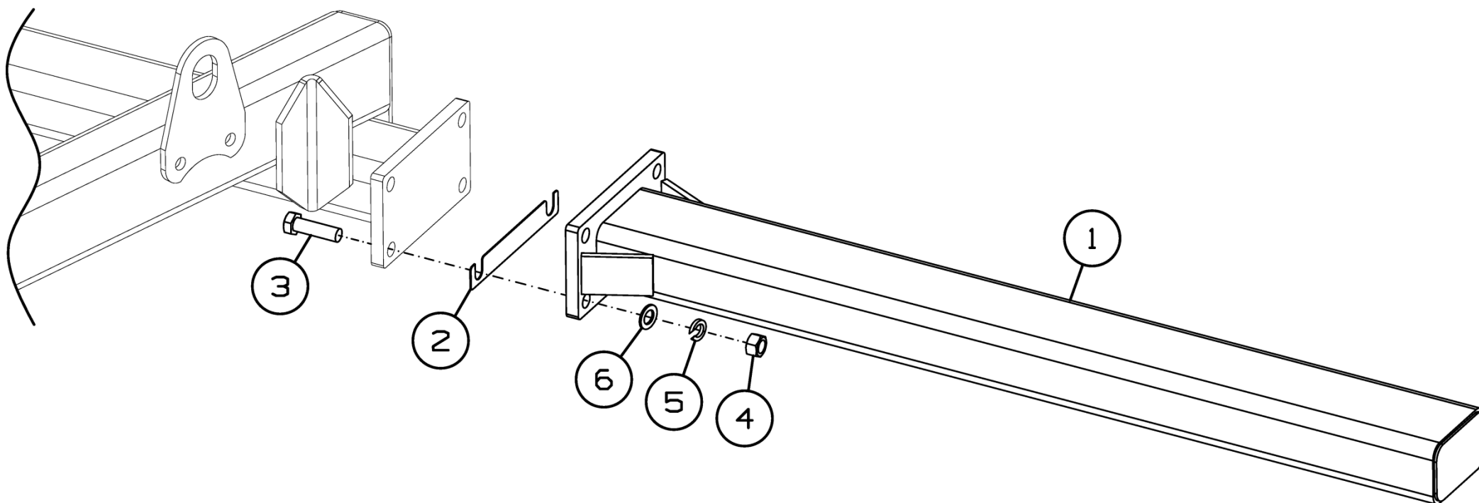
Рисунок 5 - Удлинитель рамы ДХ-880.06.010
