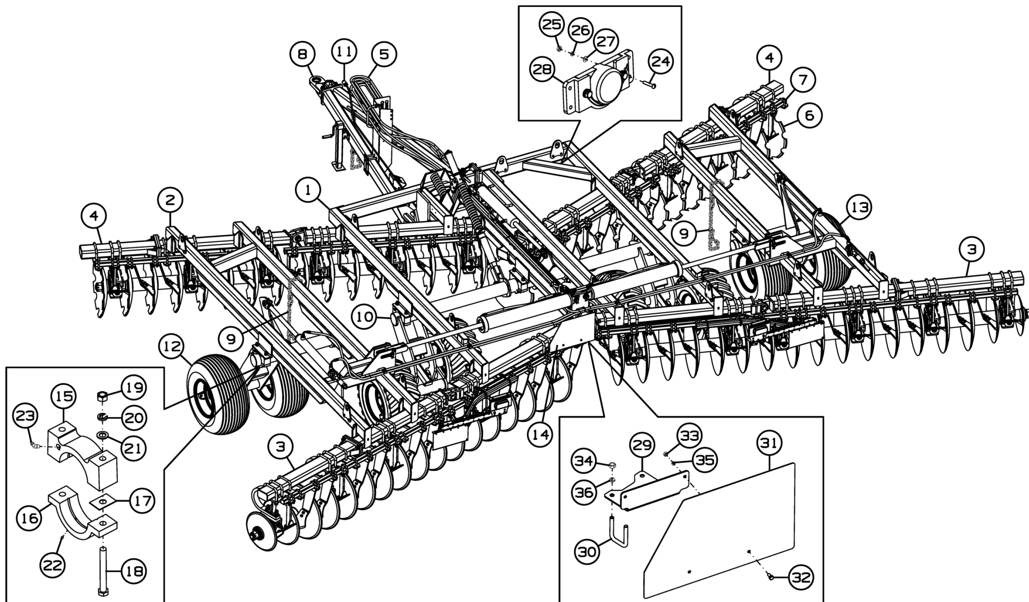
Рисунок 1 - Борона дисковая tandemная ДХ-880.00.000
