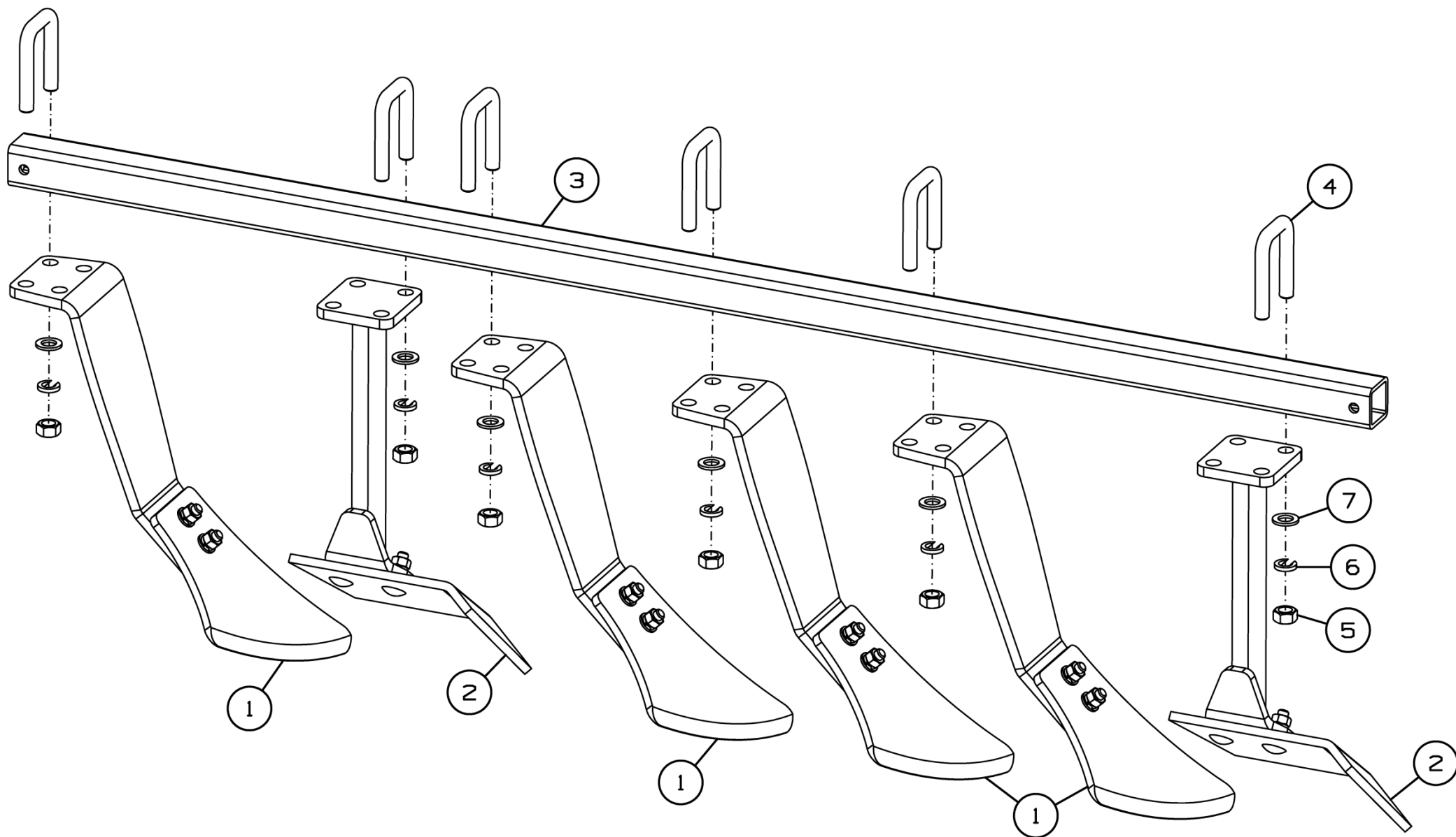
Рисунок 26 - Секция чистиков ДХ-1080.04.040А
