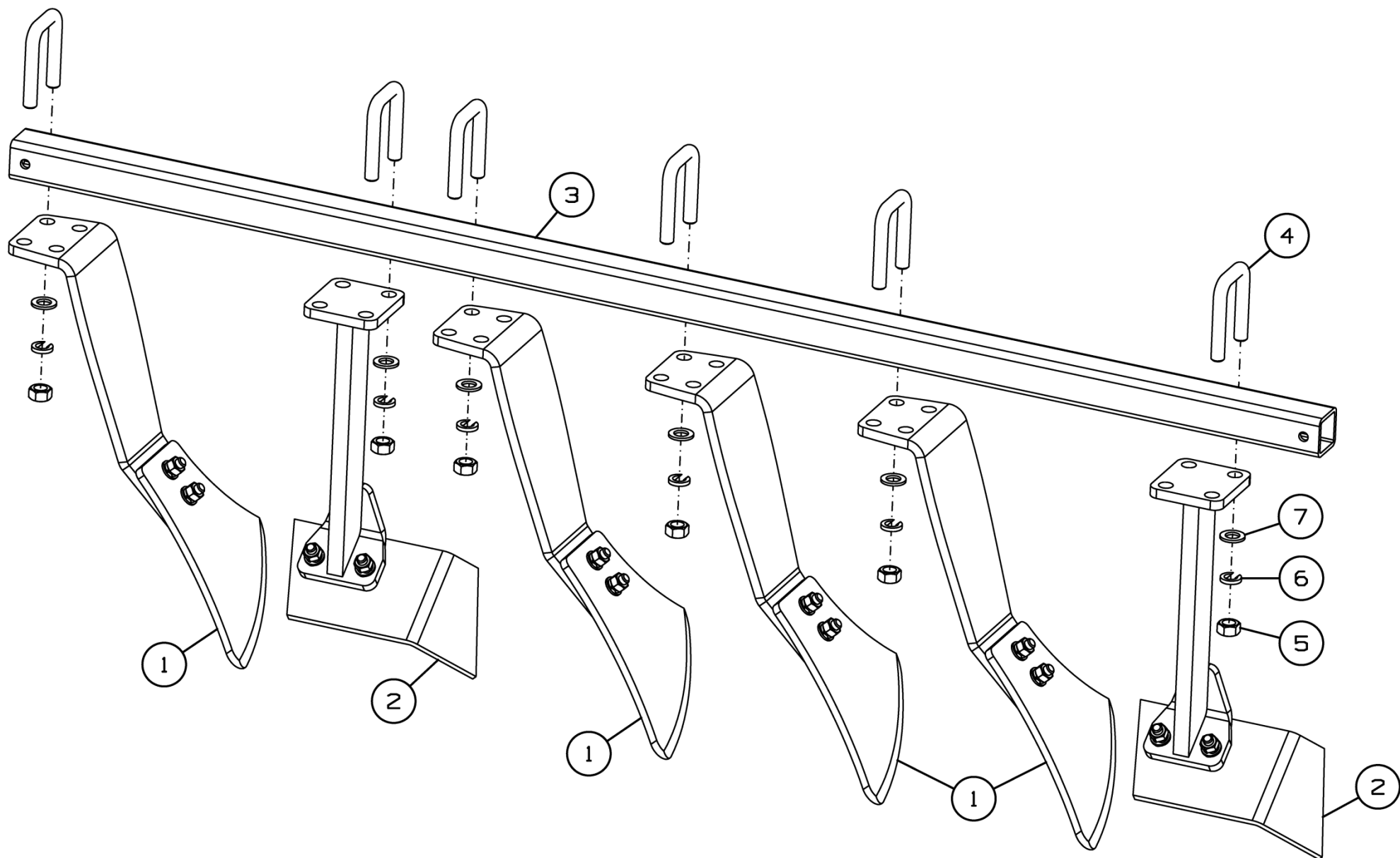
Рисунок 25 - Секция чистиков ДХ-1080.04.030А
