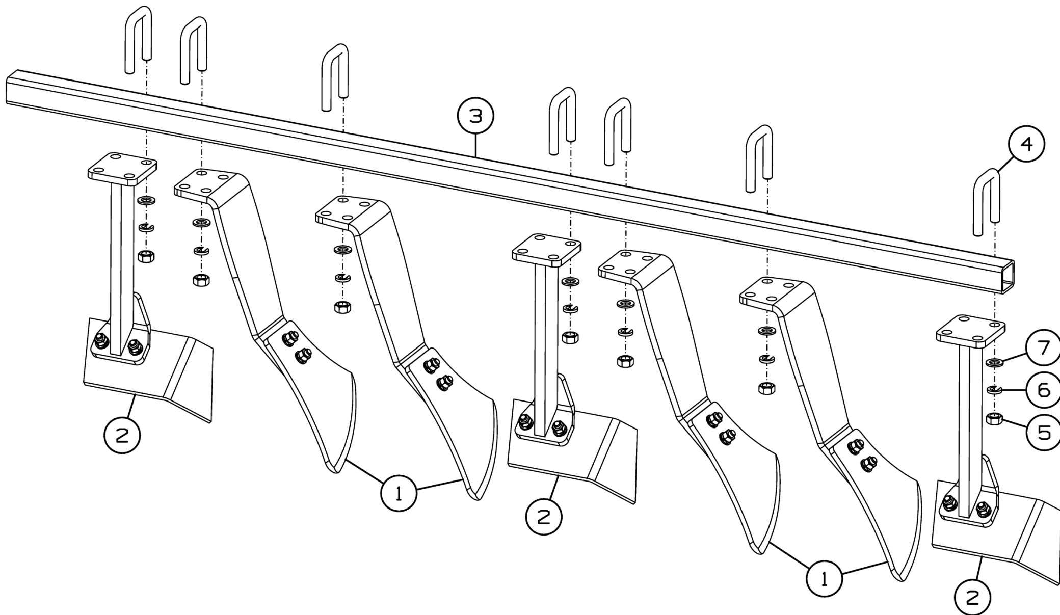
Рисунок 22 - Секция чистиков ДХ-880.04.040А
