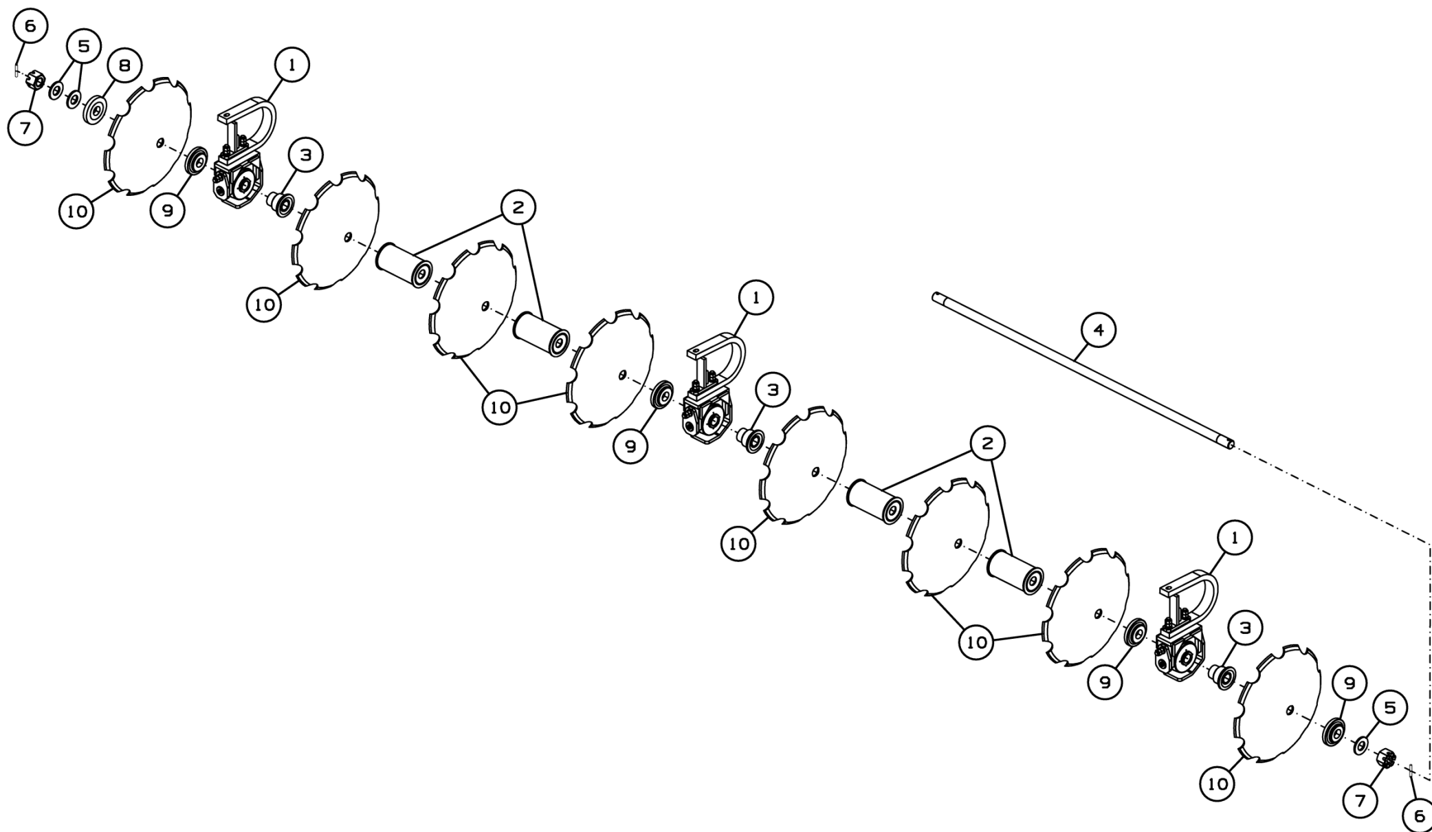
Рисунок 12 - Батарея ДХ-1080.03.010А
