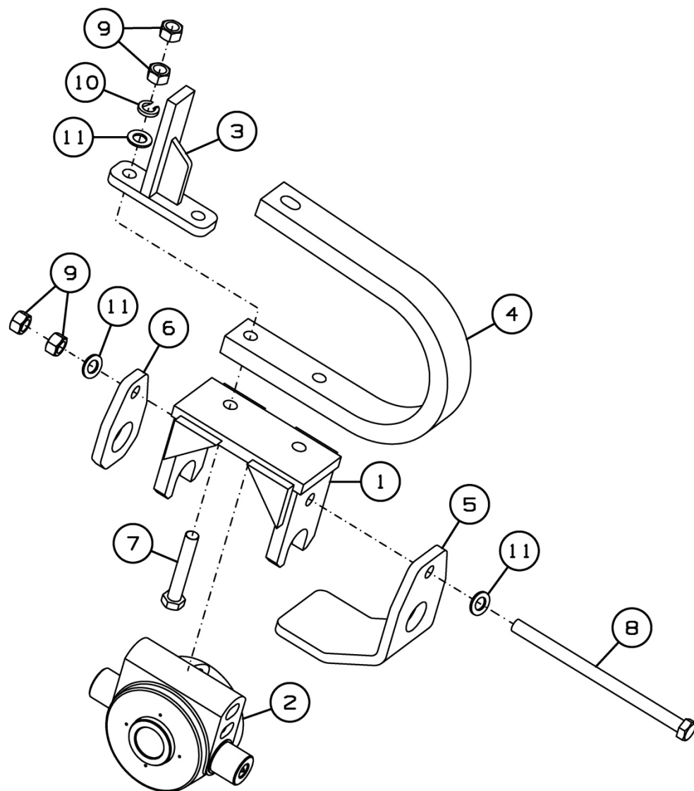
Рисунок 16 - Стойка ДХ-1080.03.800 и ДХ-1080.03.800-01
