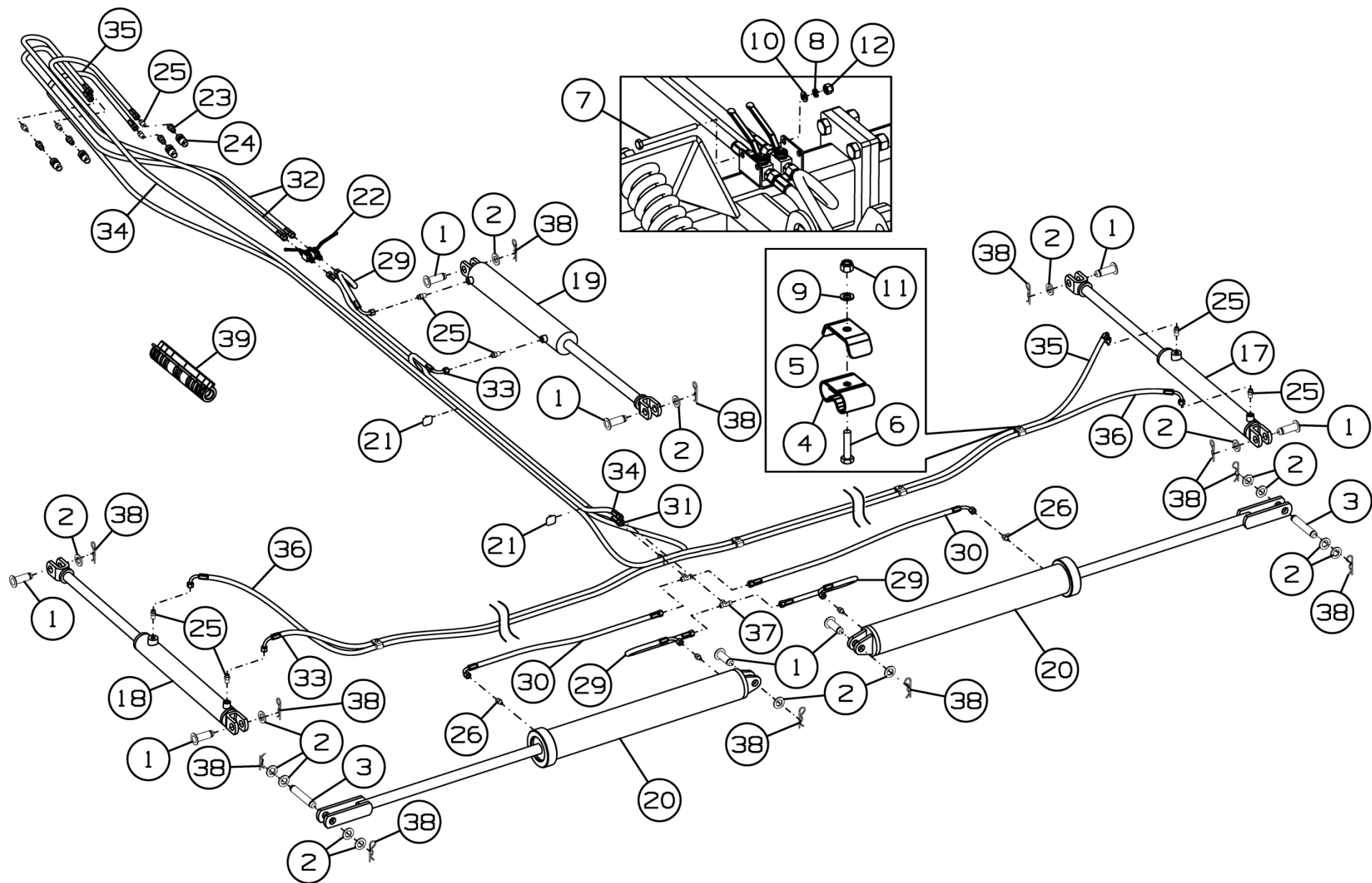
Рисунок 7 - Установка гидрооборудования ДХ-1080.12.000А
