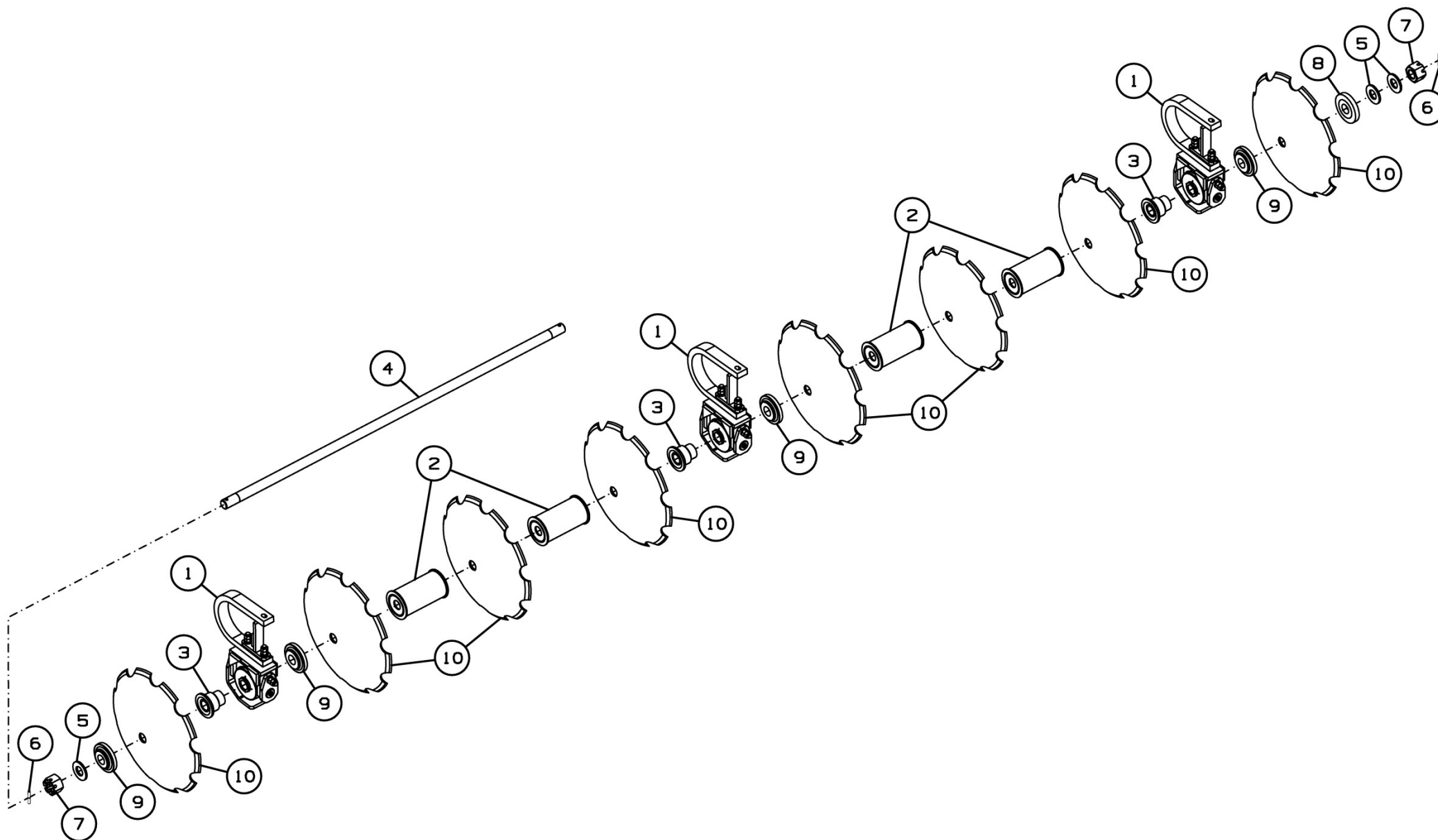
Рисунок 13 - Батарея ДХ-1080.03.020А
