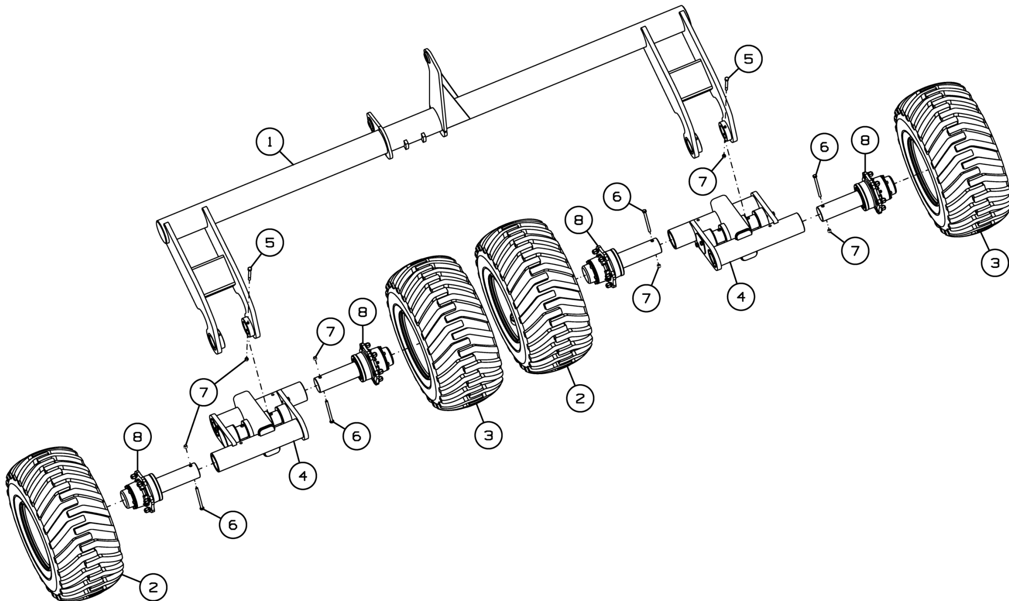
Рисунок 33 - Шасси ДХ-1080.08.000
