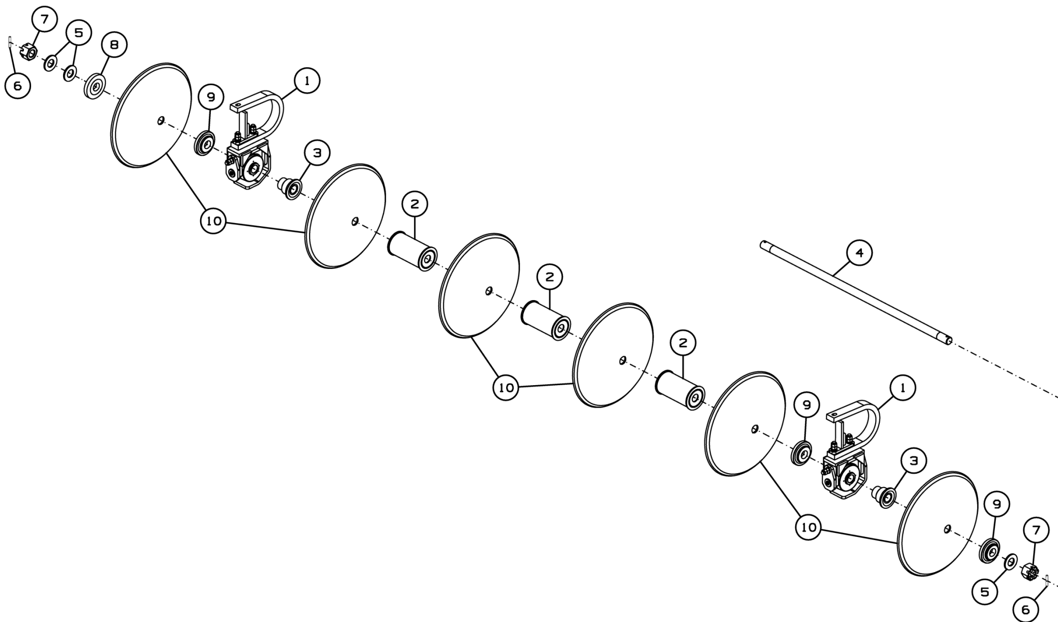
Рисунок 15 - Батарея ДХ-1080.03.040А
