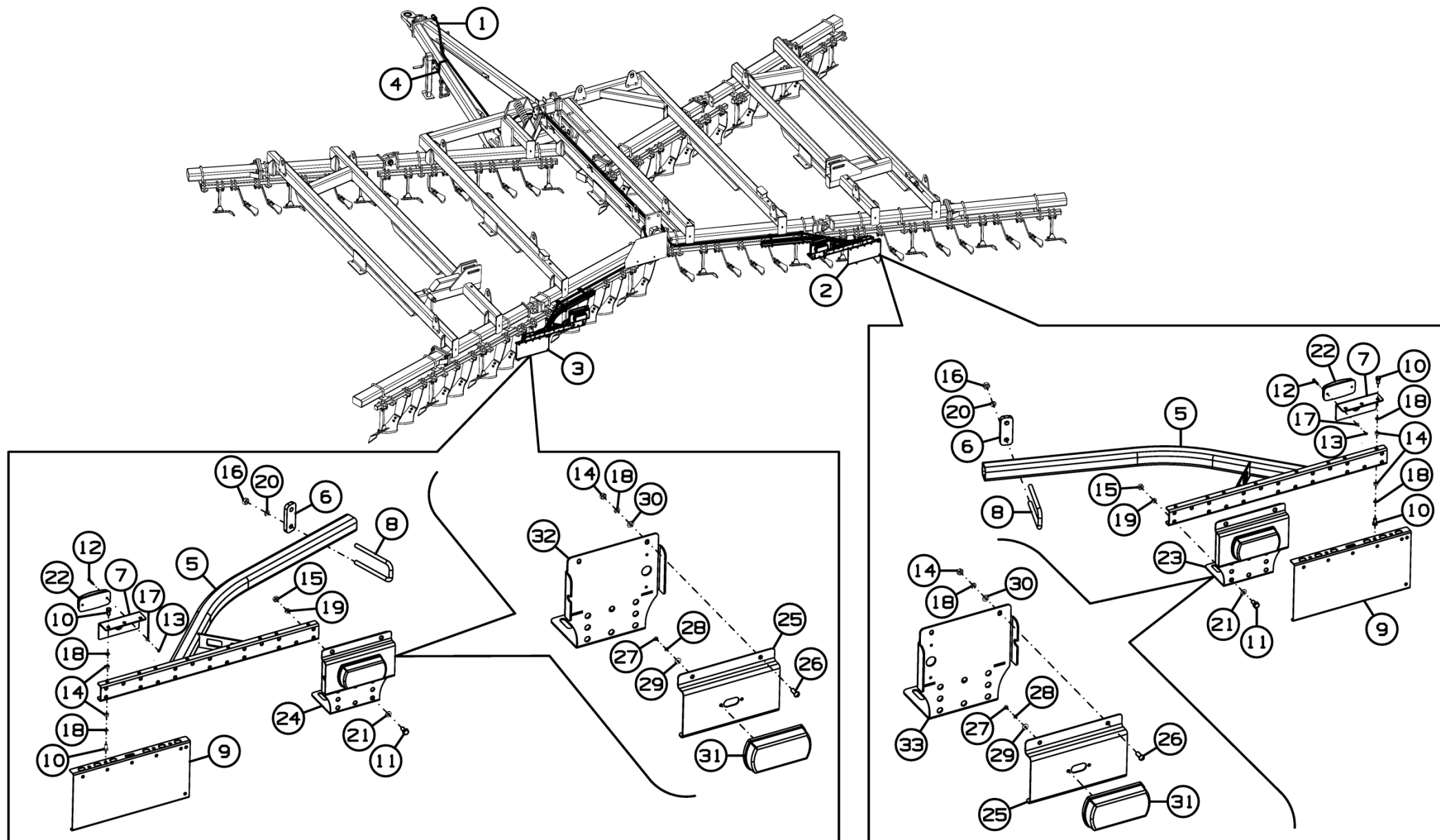
Рисунок 38 - Коммуникации электрические ДХ-1080.10.000А
