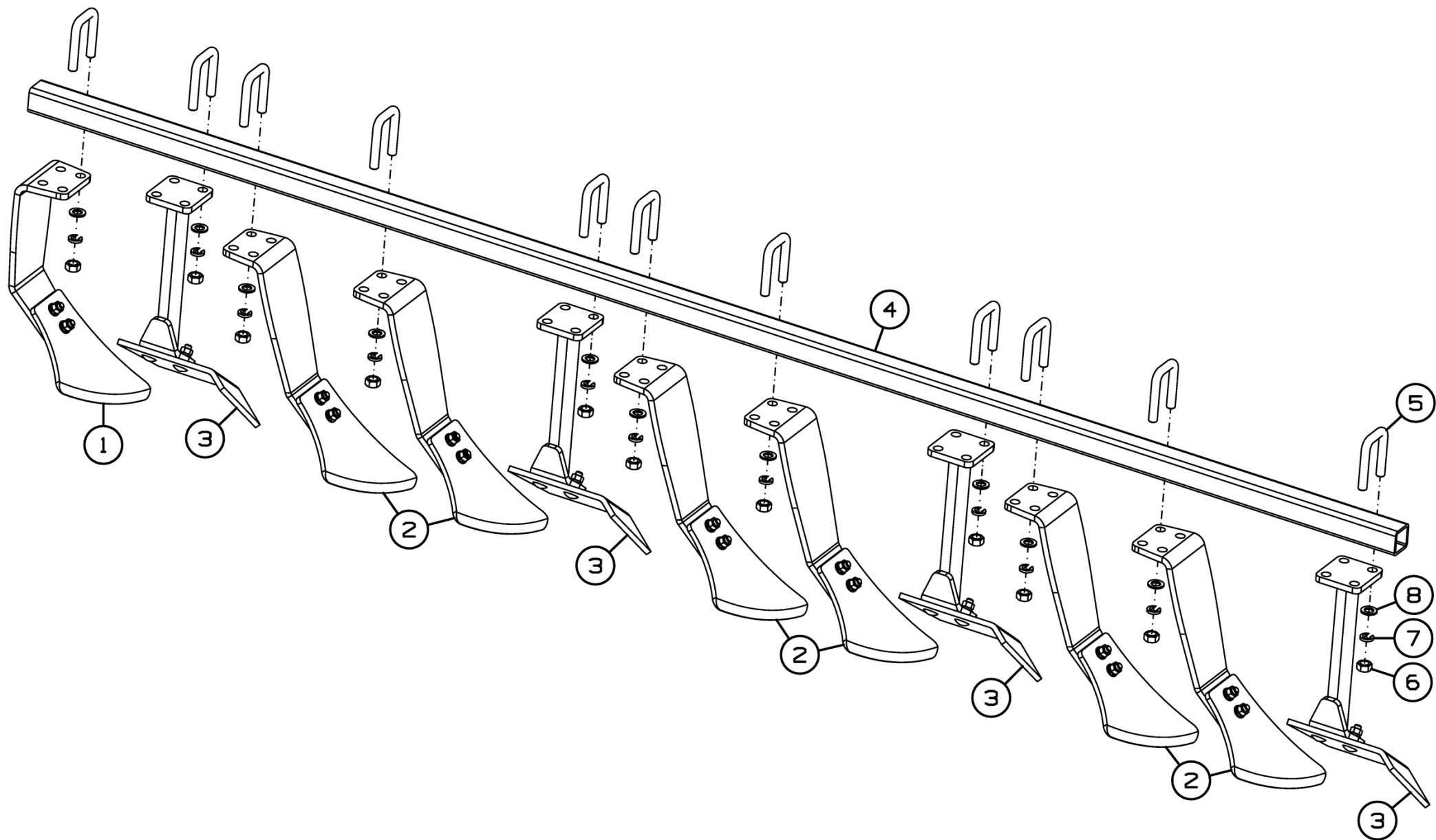
Рисунок 20 - Секция чистиков ДХ-880.04.020А
