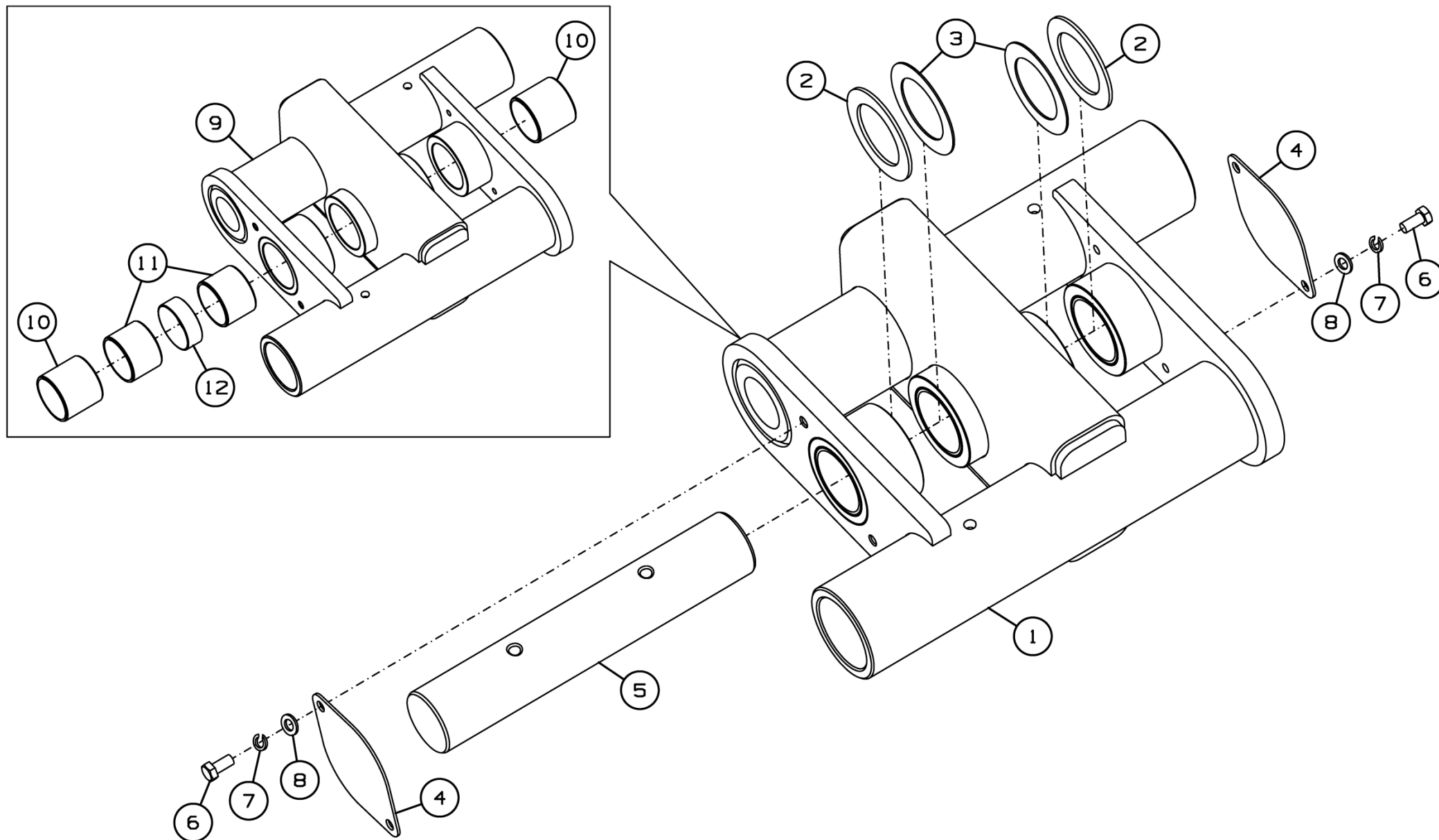
Рисунок 35 - Балансир в сборе ДХ-1080.08.100Б
