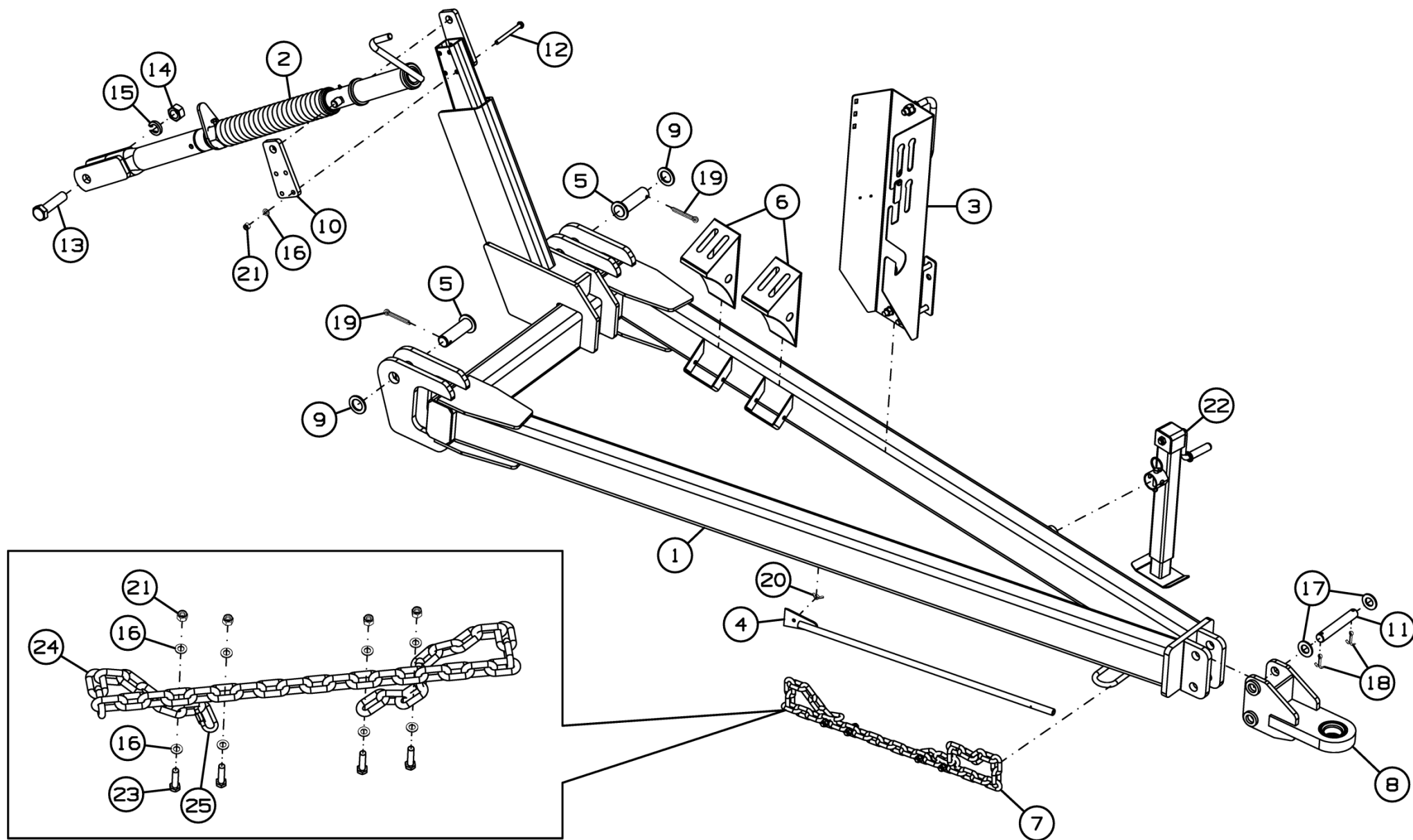
Рисунок 30 - Сница ДХ-1080.05.000А
