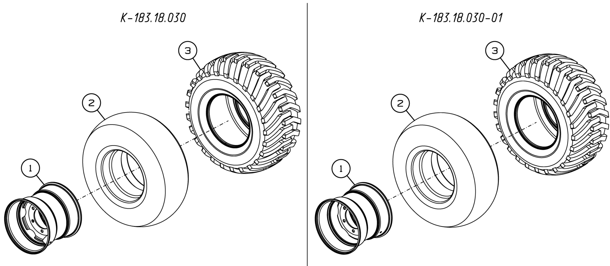
Рисунок 34 - Колесо в сборе К-183.18.030 и К-183.18.030-01
