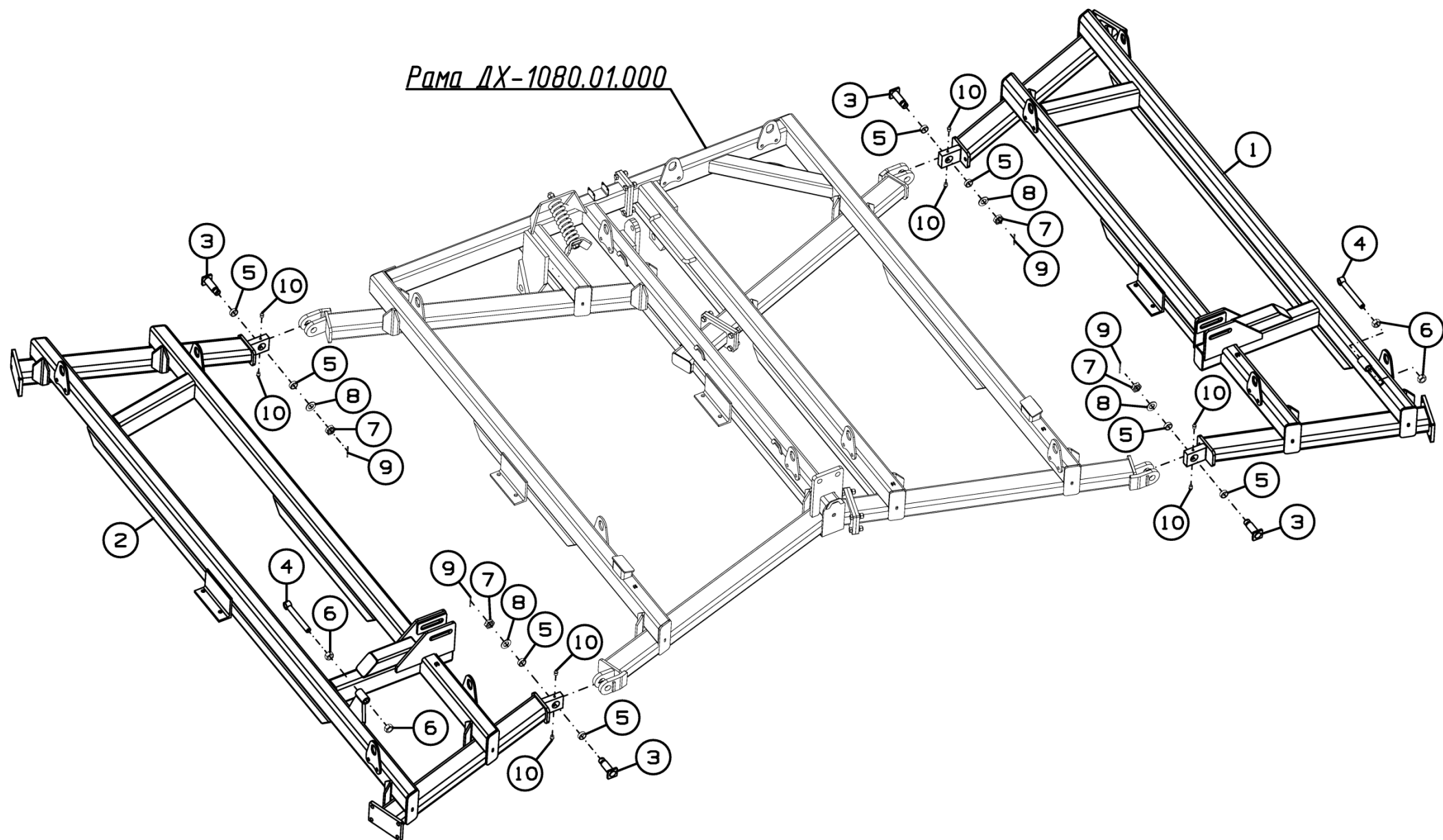
Рисунок 4 – Установка секций ДХ-880.02.000
