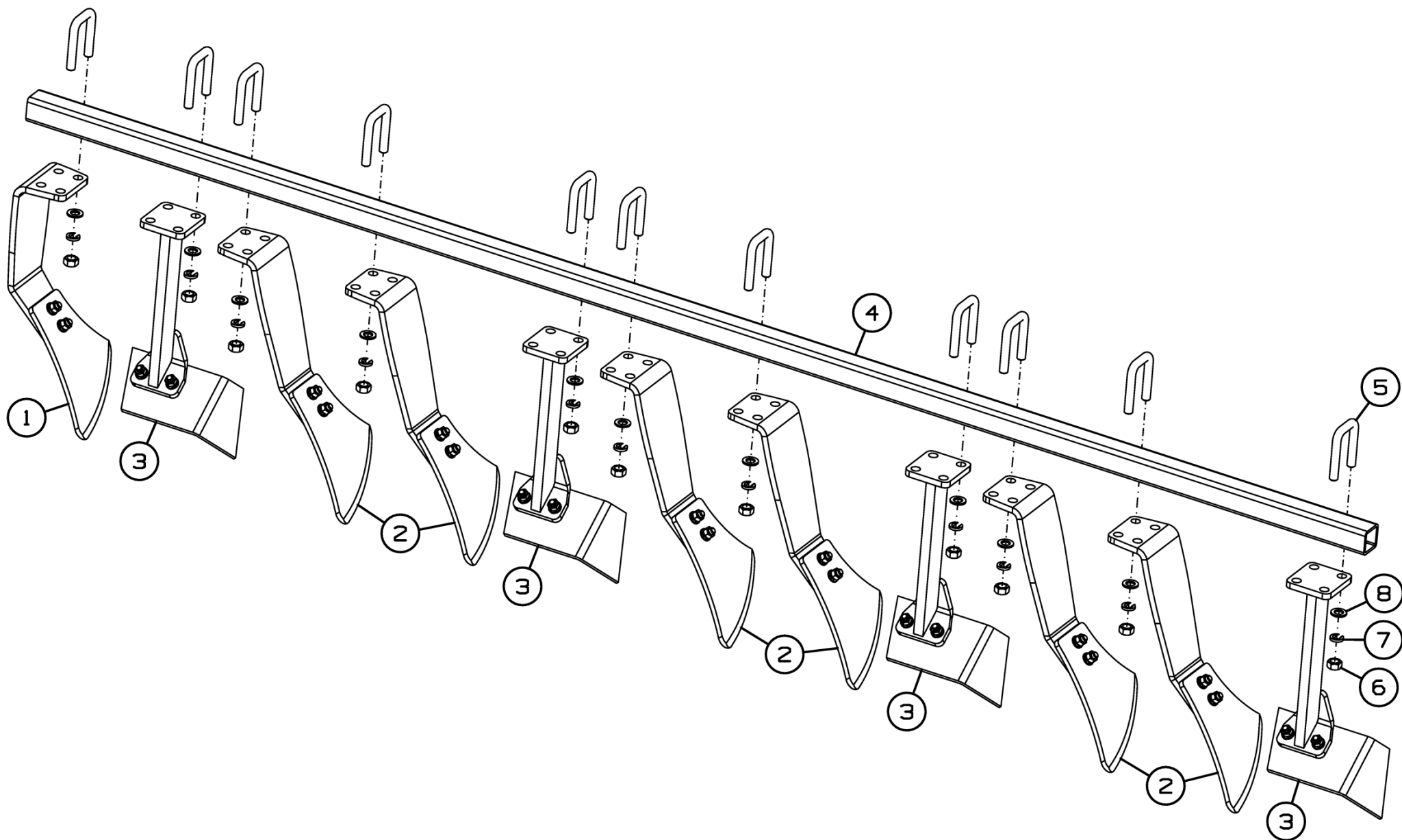
Рисунок 19 - Секция чистиков ДХ-880.04.010А
