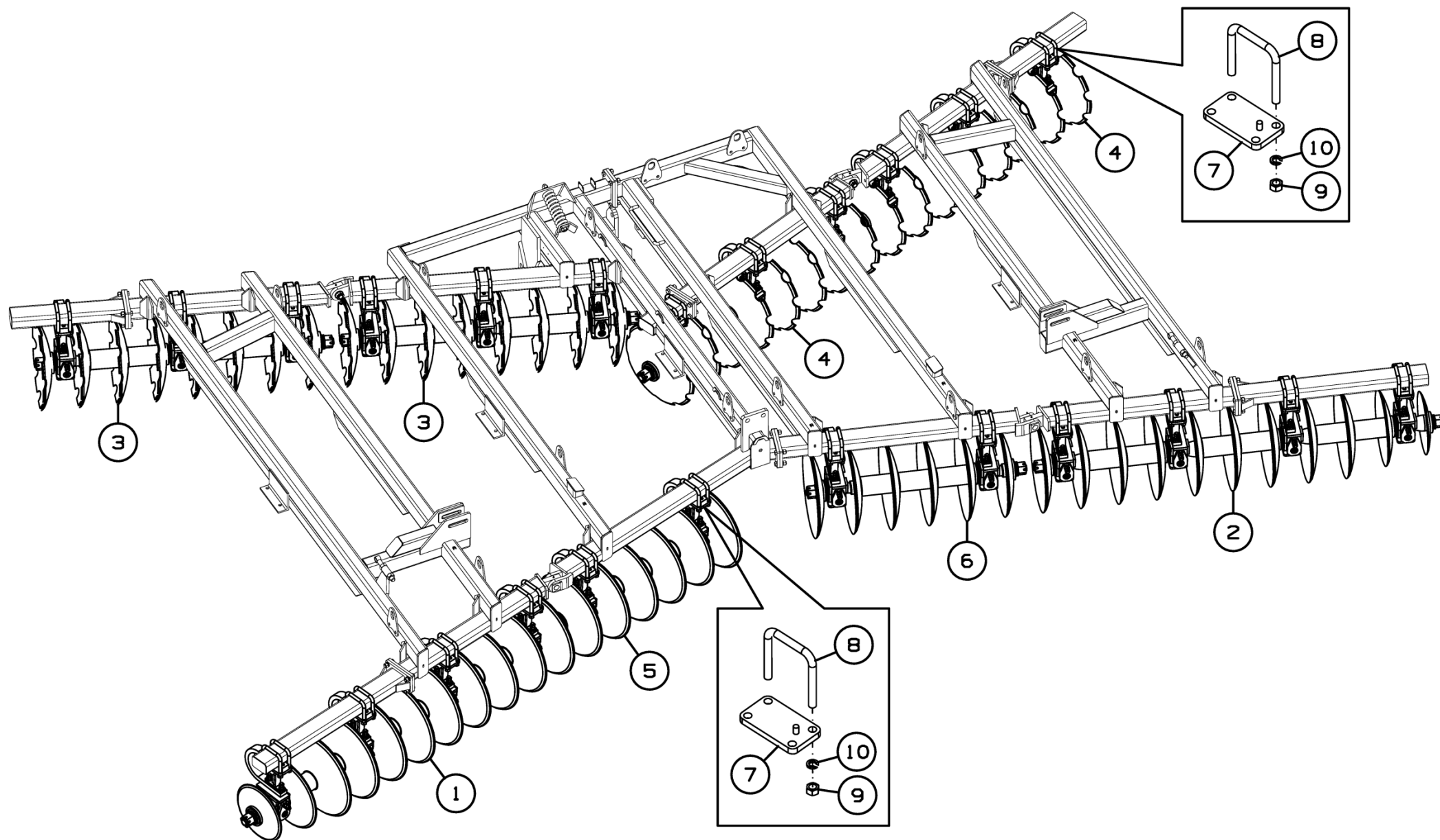
Рисунок 9 - Установка дисковых батарей ДХ-880.03.000 (общий вид)
