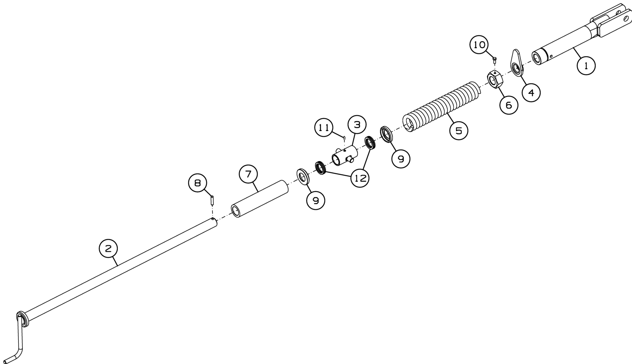
Рисунок 31 - Регулятор горизонта ДХ-1080.05.100
