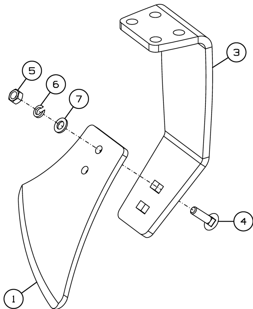
Рисунок 28 - Чистик ДХ-1080.04.320 и ДХ-1080.04.320-01
