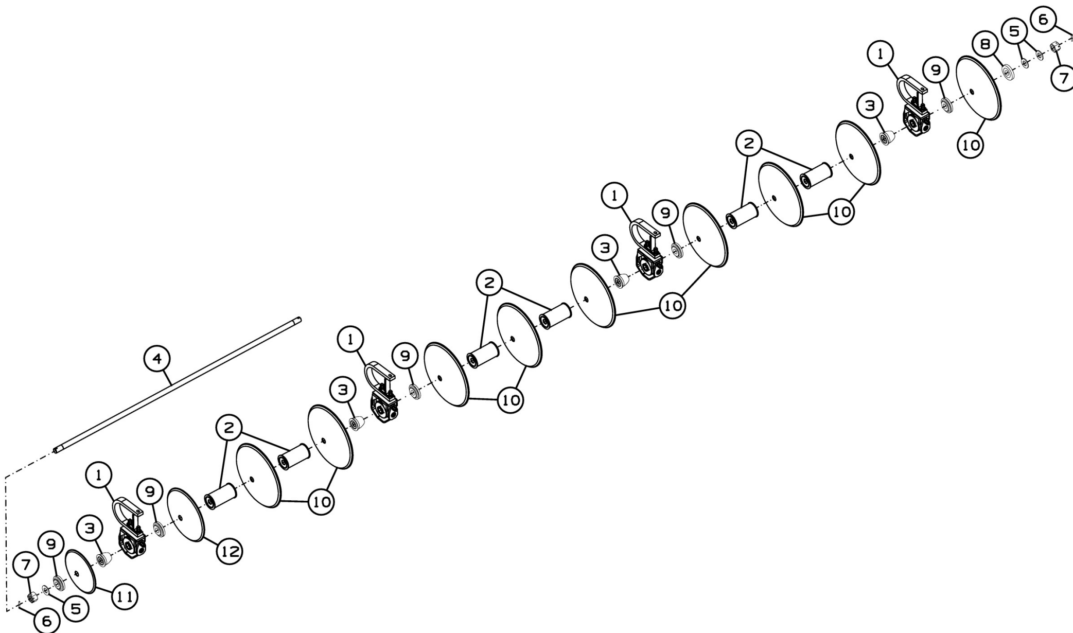
Рисунок 10 - Батарея ДХ-880.03.010А
