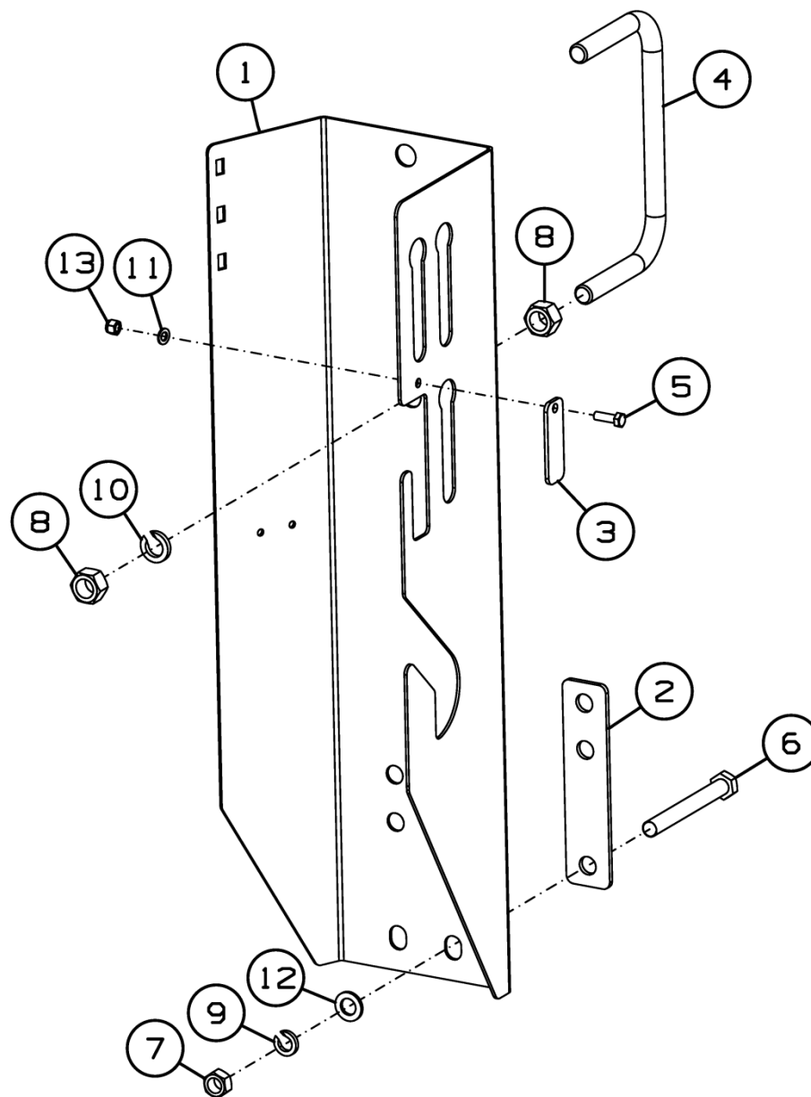
Рисунок 32 – Кронштейн ДХ-1080.05.180
