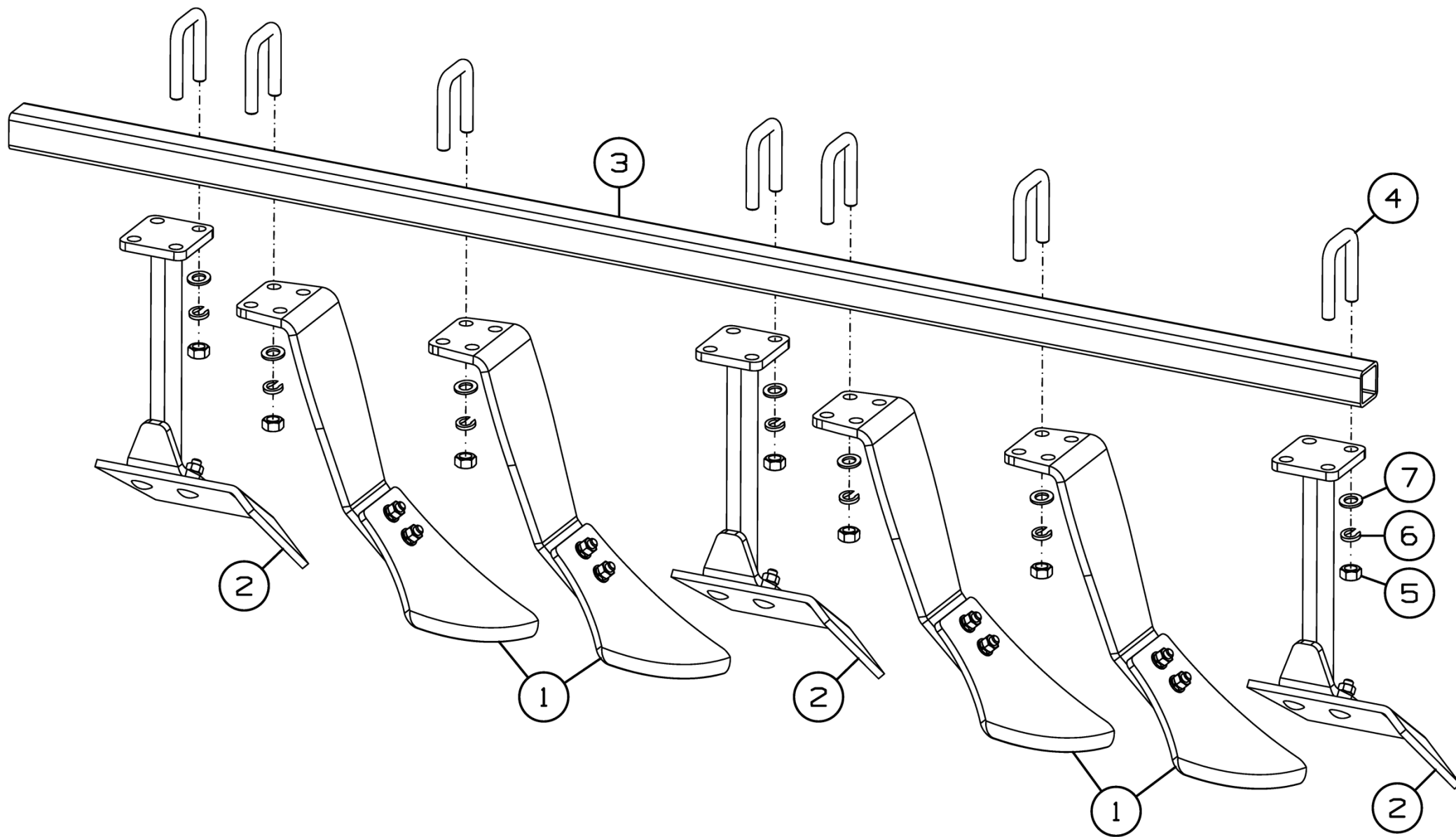
Рисунок 21 - Секция чистиков ДХ-880.04.030А
