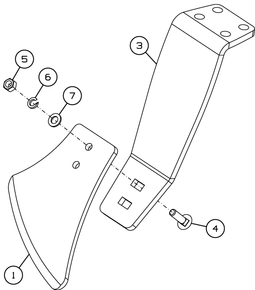
Рисунок 27 - Чистик ДХ-1080.04.310 и ДХ-1080.04.310-01
