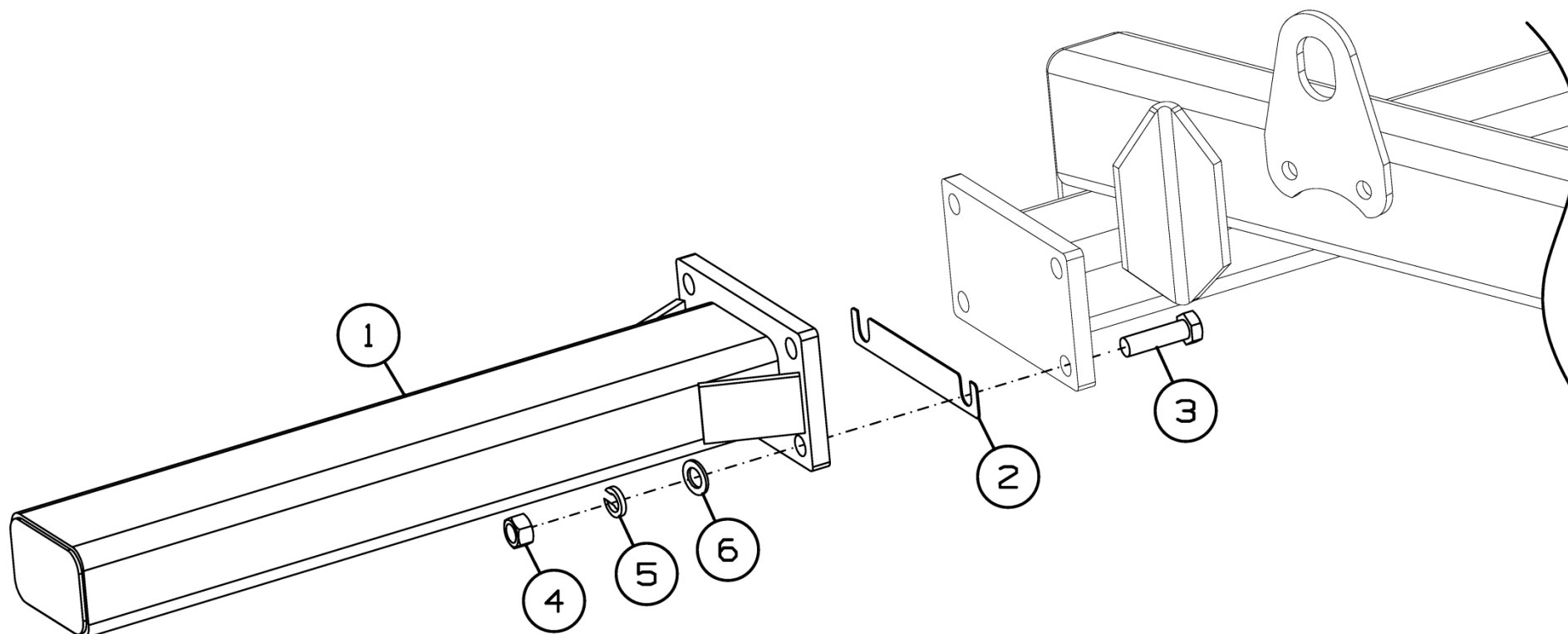
Рисунок 6 - Удлинитель рамы ДХ-880.06.020
